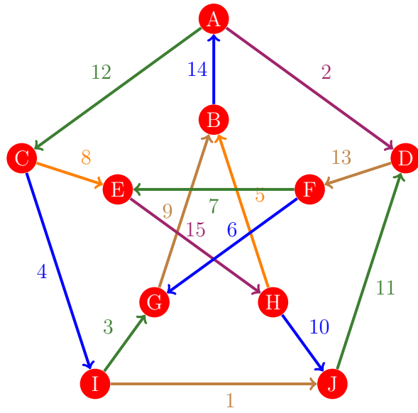
Figura 1076: Flujo 1068 de la gráfica de Petersen
