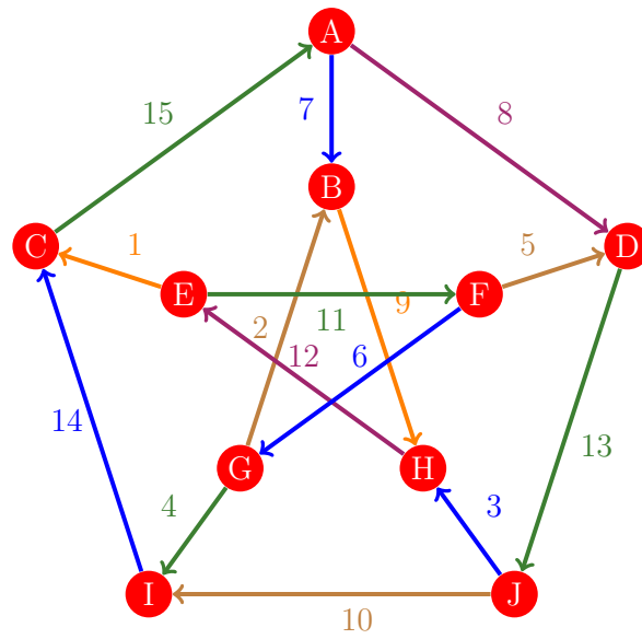
Figura 568: Flujo 560 de la gráfica de Petersen
