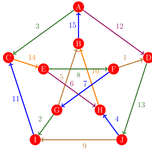
Figura 1131: Flujo 1123 de la gráfica de Petersen
