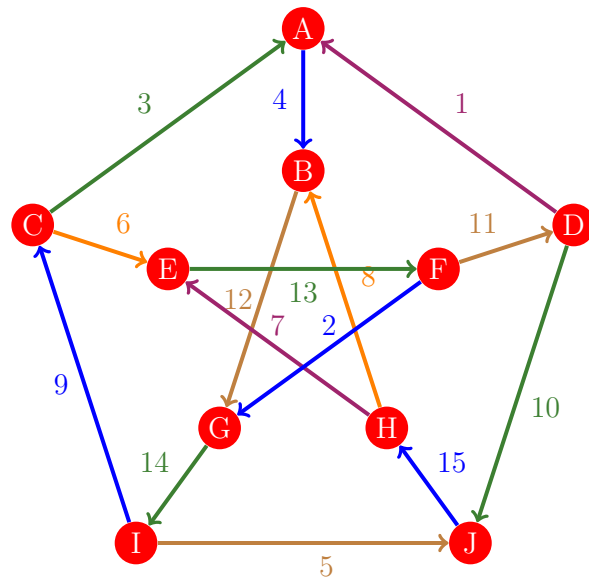
Figura 292: Flujo 284 de la gráfica de Petersen
