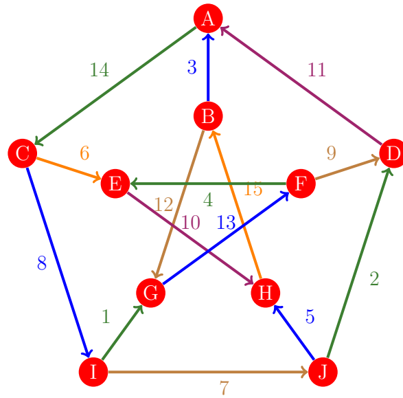
Figura 205: Flujo 197 de la gráfica de Petersen
