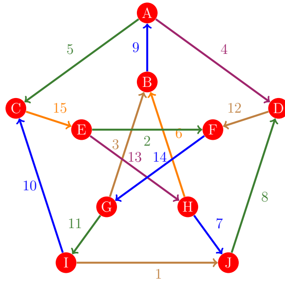
Figura 667: Flujo 659 de la gráfica de Petersen
