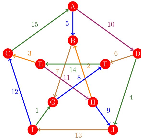
Figura 403: Flujo 395 de la gráfica de Petersen
