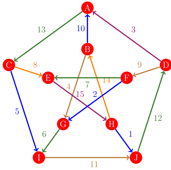
Figura 757: Flujo 749 de la gráfica de Petersen
