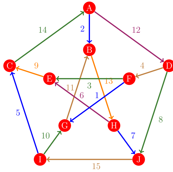
Figura 163: Flujo 155 de la gráfica de Petersen
