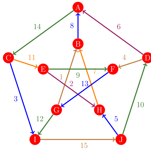
Figura 604: Flujo 596 de la gráfica de Petersen
