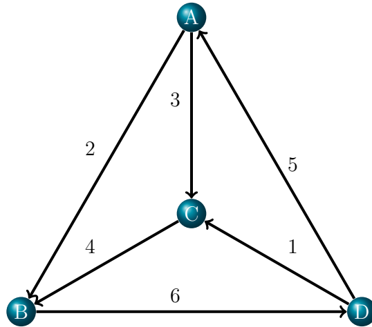
Figura 2: Flujo elegante en una gráfica.
