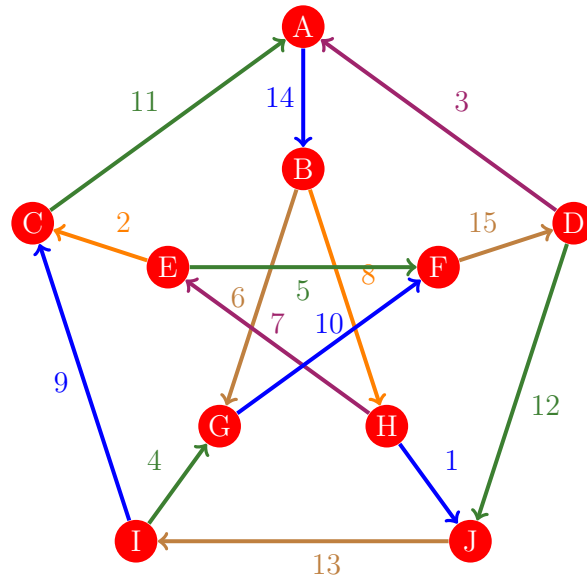
Figura 1111: Flujo 1103 de la gráfica de Petersen
