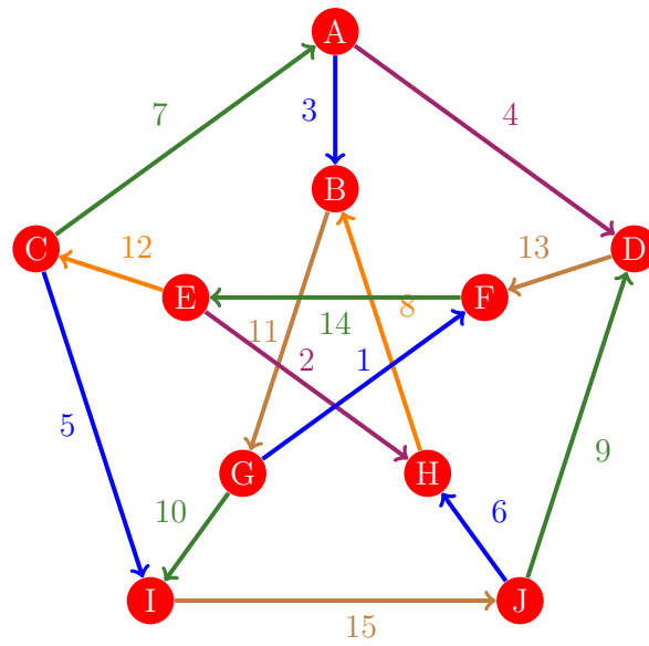
Figura 220: Flujo 212 de la gráfica de Petersen
