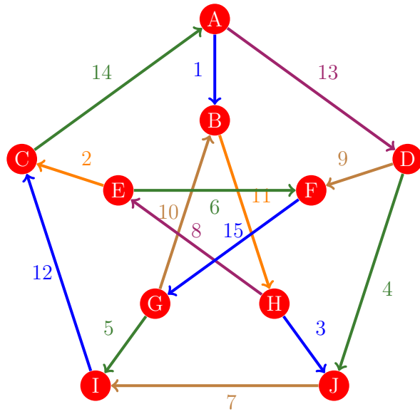
Figura 83: Flujo 75 de la gráfica de Petersen
