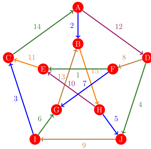
Figura 164: Flujo 156 de la gráfica de Petersen
