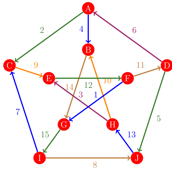
Figura 290: Flujo 282 de la gráfica de Petersen
