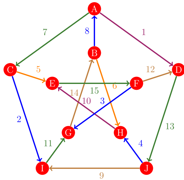
Figura 590: Flujo 582 de la gráfica de Petersen
