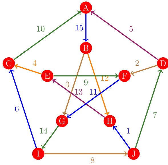
Figura 1193: Flujo 1185 de la gráfica de Petersen
