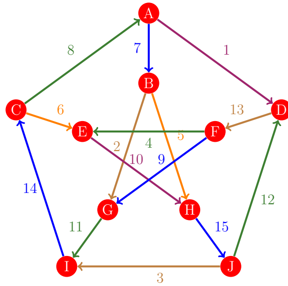
Figura 551: Flujo 543 de la gráfica de Petersen
