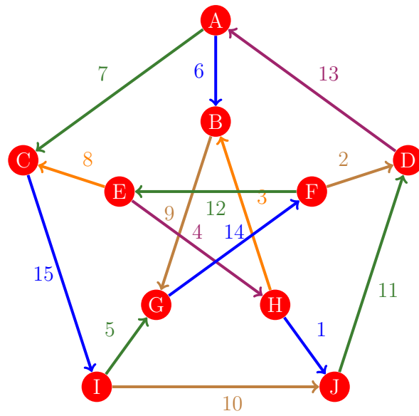
Figura 464: Flujo 456 de la gráfica de Petersen
