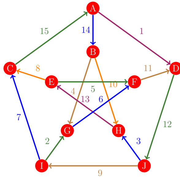
Figura 1127: Flujo 1119 de la gráfica de Petersen
