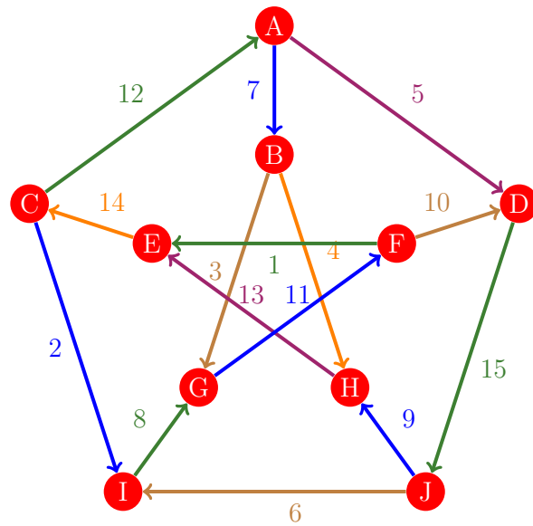
Figura 560: Flujo 552 de la gráfica de Petersen
