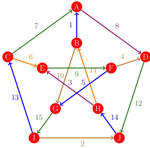
Figura 13: Flujo 5 de la gráfica de Petersen
