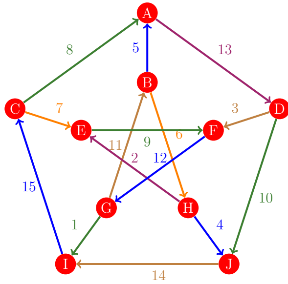
Figura 340: Flujo 332 de la gráfica de Petersen
