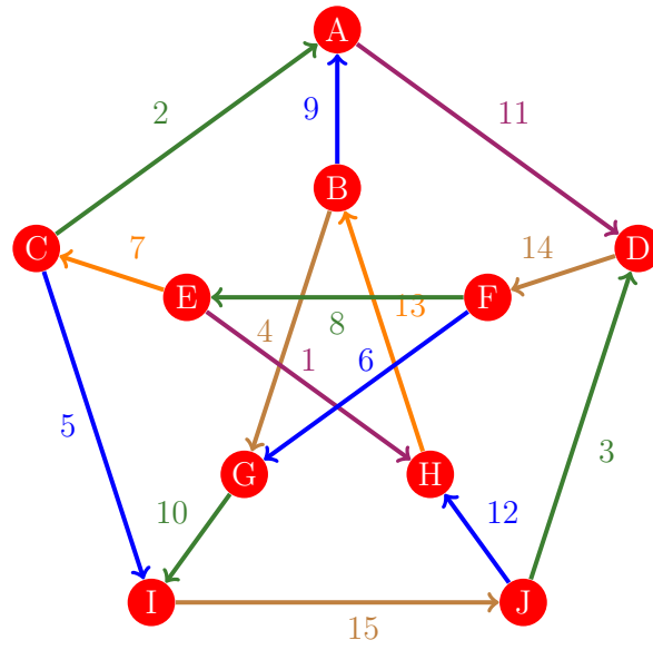
Figura 649: Flujo 641 de la gráfica de Petersen
