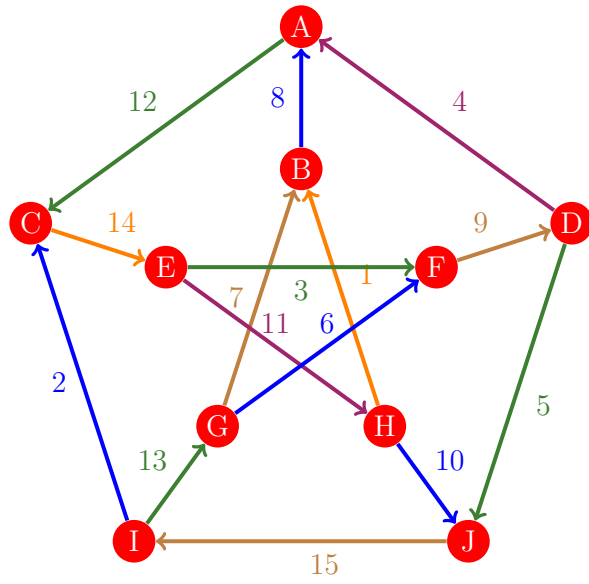
Figura 597: Flujo 589 de la gráfica de Petersen
