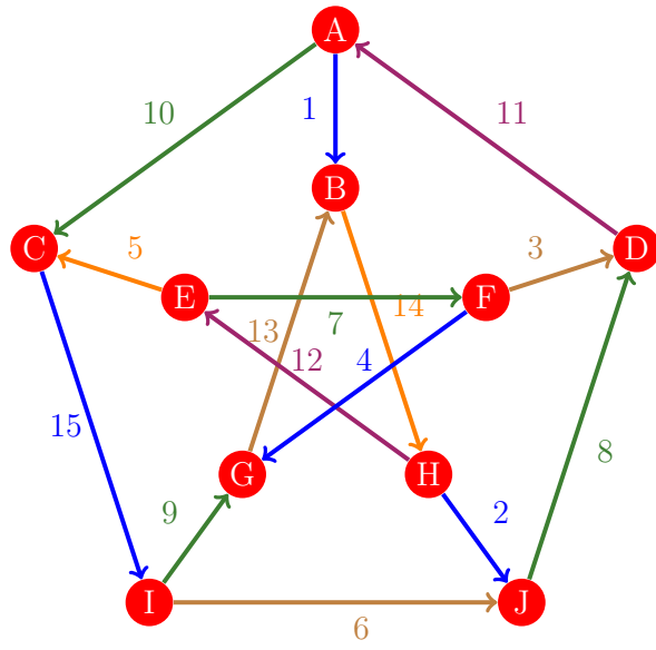
Figura 65: Flujo 57 de la gráfica de Petersen
