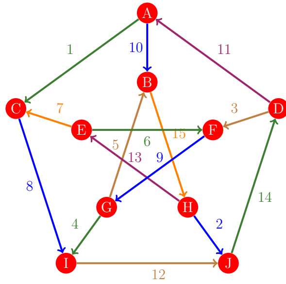
Figura 785: Flujo 777 de la gráfica de Petersen
