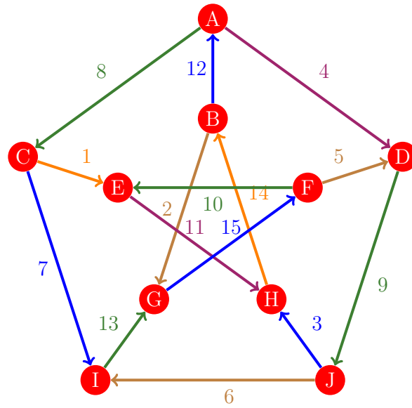
Figura 907: Flujo 899 de la gráfica de Petersen
