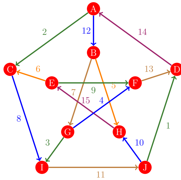
Figura 932: Flujo 924 de la gráfica de Petersen
