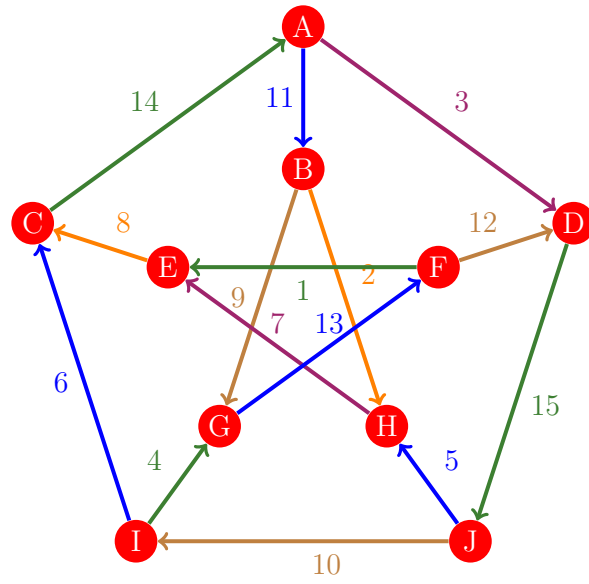
Figura 885: Flujo 877 de la gráfica de Petersen
