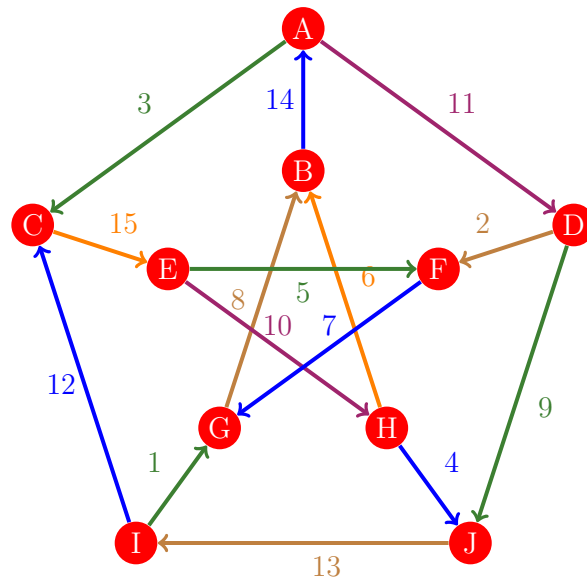
Figura 1056: Flujo 1048 de la gráfica de Petersen
