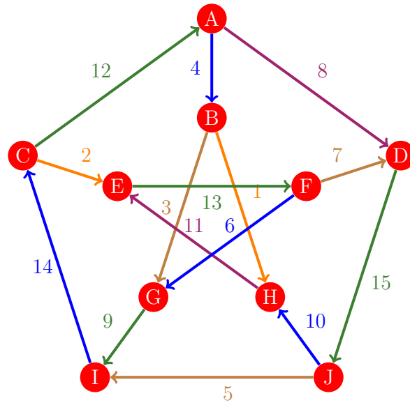
Figura 321: Flujo 313 de la gráfica de Petersen
