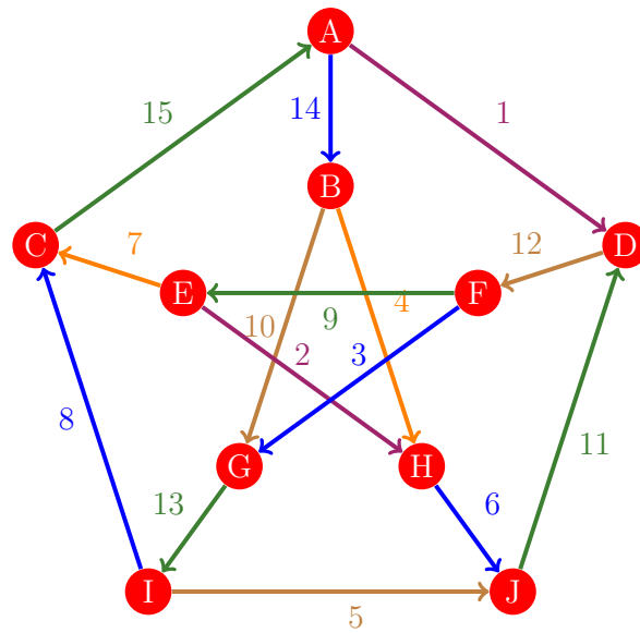
Figura 1128: Flujo 1120 de la gráfica de Petersen
