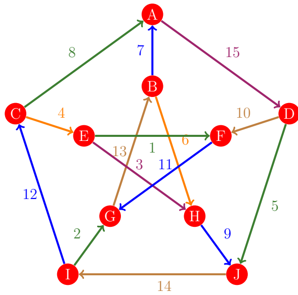
Figura 512: Flujo 504 de la gráfica de Petersen
