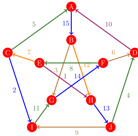
Figura 1178: Flujo 1170 de la gráfica de Petersen
