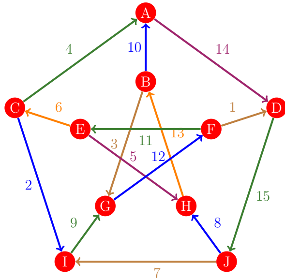
Figura 732: Flujo 724 de la gráfica de Petersen
