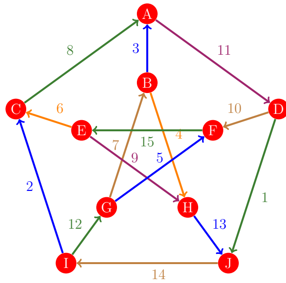
Figura 182: Flujo 174 de la gráfica de Petersen
