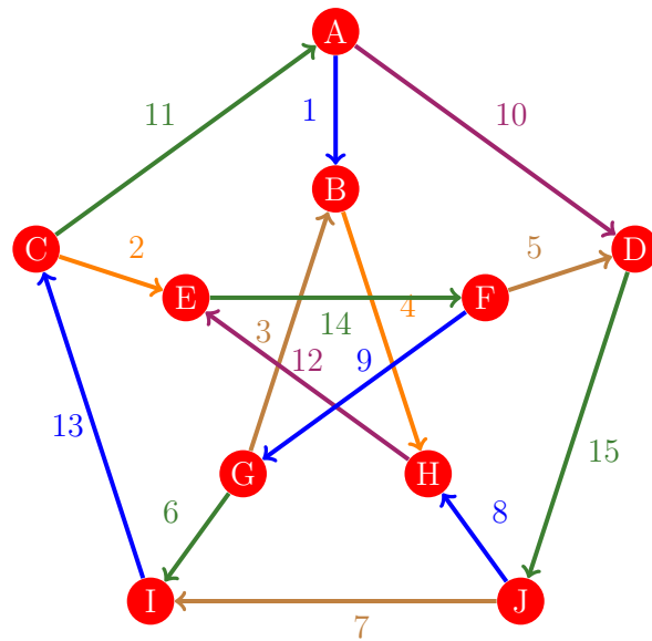
Figura 70: Flujo 62 de la gráfica de Petersen
