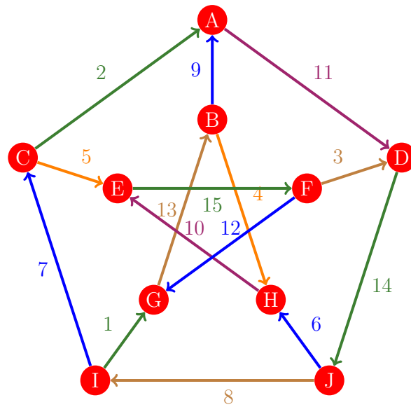
Figura 650: Flujo 642 de la gráfica de Petersen
