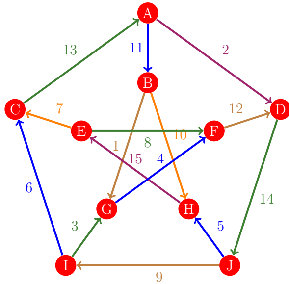
Figura 884: Flujo 876 de la gráfica de Petersen
