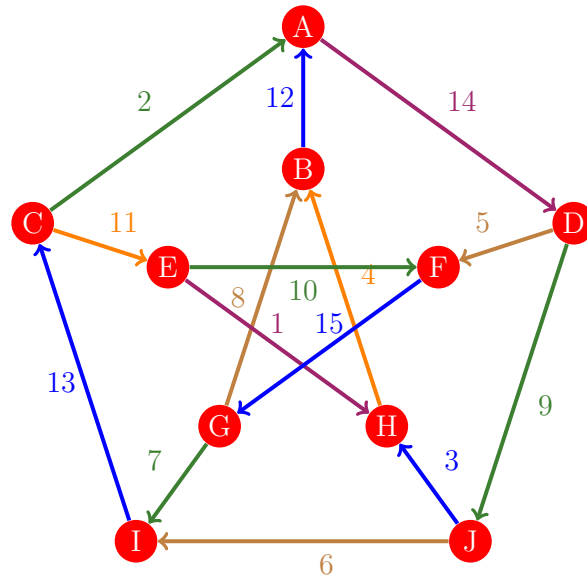
Figura 893: Flujo 885 de la gráfica de Petersen
