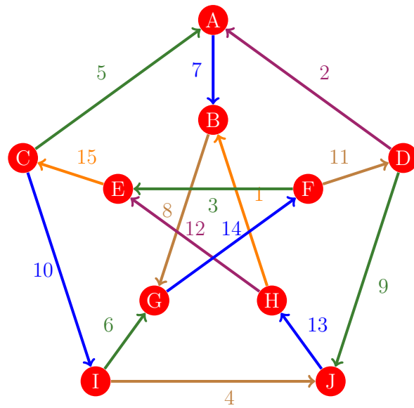
Figura 538: Flujo 530 de la gráfica de Petersen
