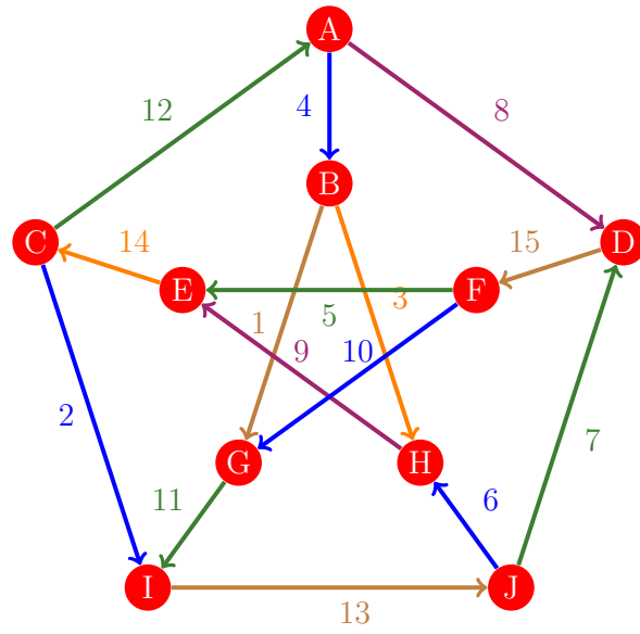
Figura 319: Flujo 311 de la gráfica de Petersen
