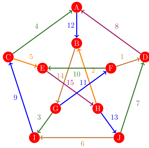
Figura 942: Flujo 934 de la gráfica de Petersen
