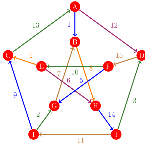
Figura 79: Flujo 71 de la gráfica de Petersen
