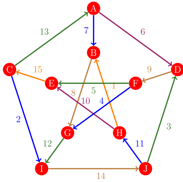
Figura 563: Flujo 555 de la gráfica de Petersen
