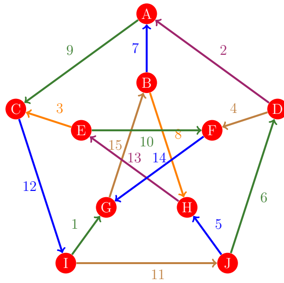
Figura 518: Flujo 510 de la gráfica de Petersen
