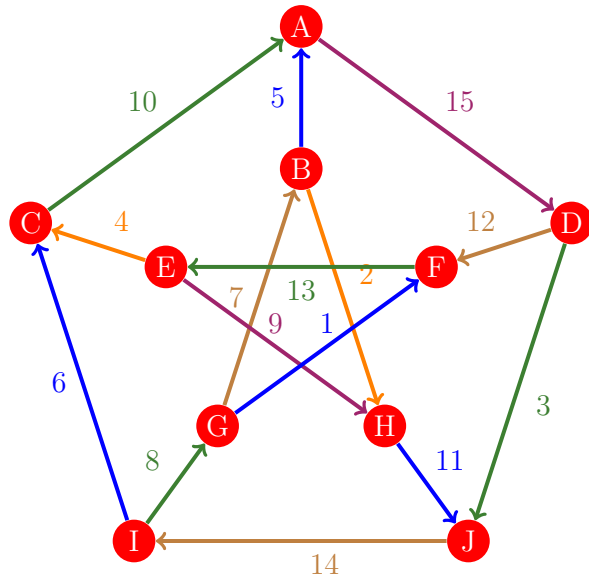
Figura 346: Flujo 338 de la gráfica de Petersen
