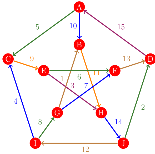
Figura 778: Flujo 770 de la gráfica de Petersen
