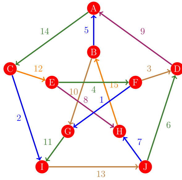
Figura 359: Flujo 351 de la gráfica de Petersen
