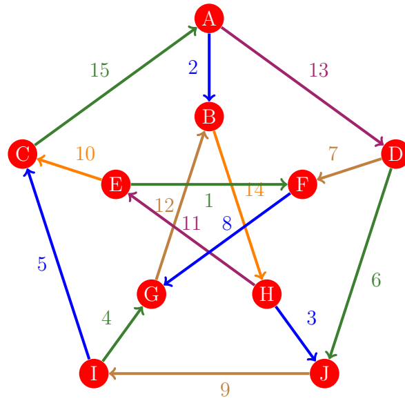
Figura 167: Flujo 159 de la gráfica de Petersen
