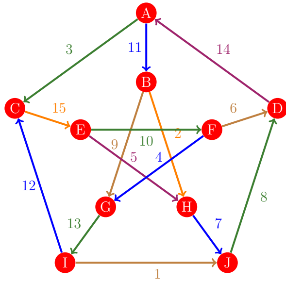
Figura 855: Flujo 847 de la gráfica de Petersen
