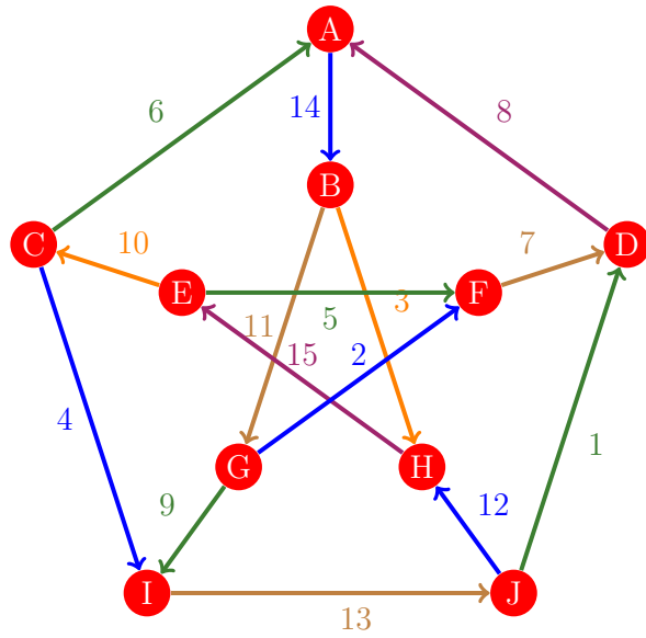
Figura 1104: Flujo 1096 de la gráfica de Petersen
