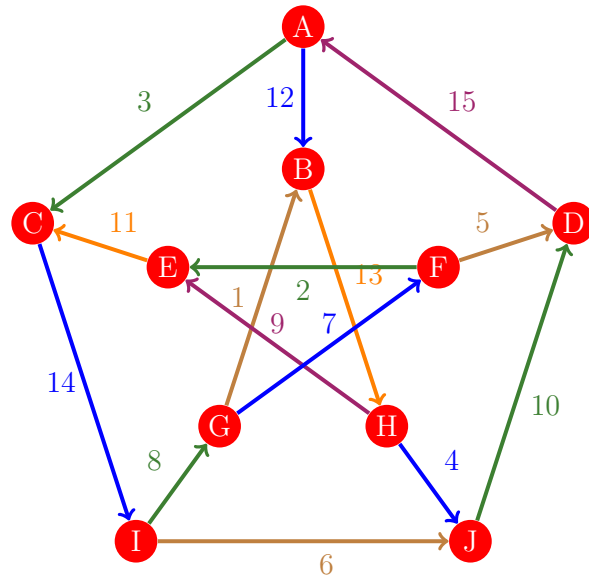
Figura 937: Flujo 929 de la gráfica de Petersen
