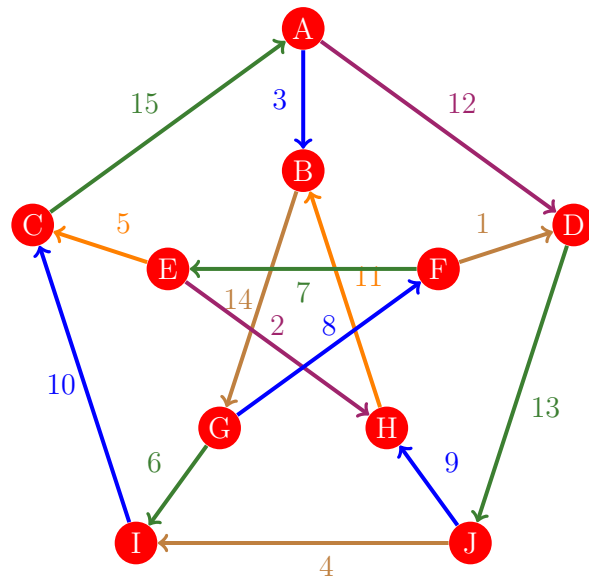
Figura 248: Flujo 240 de la gráfica de Petersen
