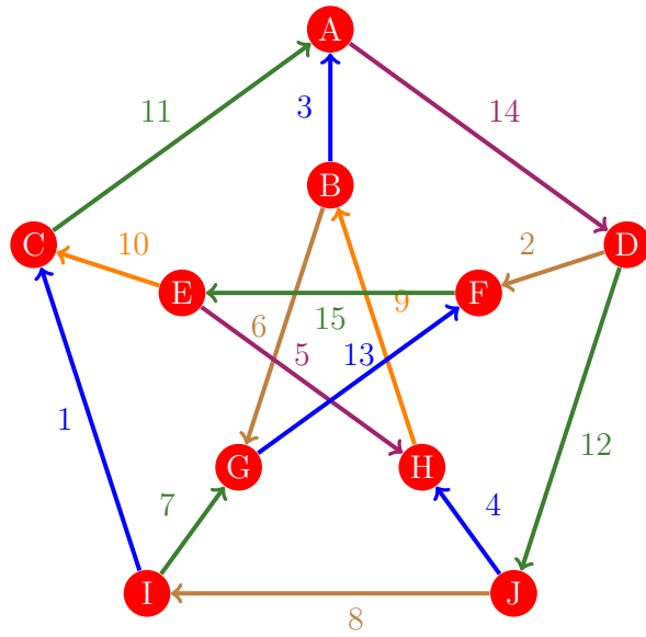
Figura 191: Flujo 183 de la gráfica de Petersen
