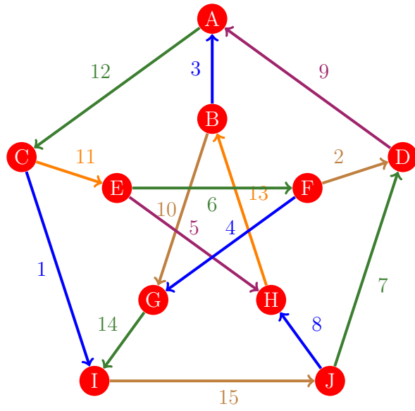
Figura 199: Flujo 191 de la gráfica de Petersen
