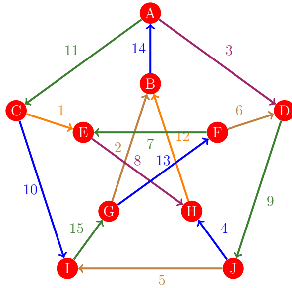
Figura 1073: Flujo 1065 de la gráfica de Petersen
