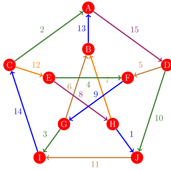
Figura 969: Flujo 961 de la gráfica de Petersen
