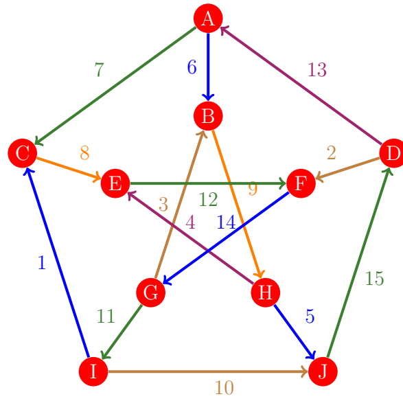
Figura 465: Flujo 457 de la gráfica de Petersen
