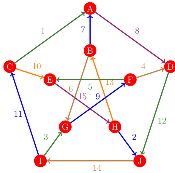
Figura 506: Flujo 498 de la gráfica de Petersen
