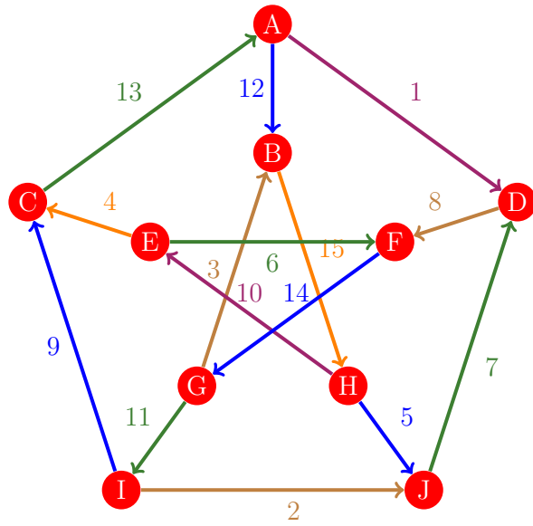
Figura 959: Flujo 951 de la gráfica de Petersen
