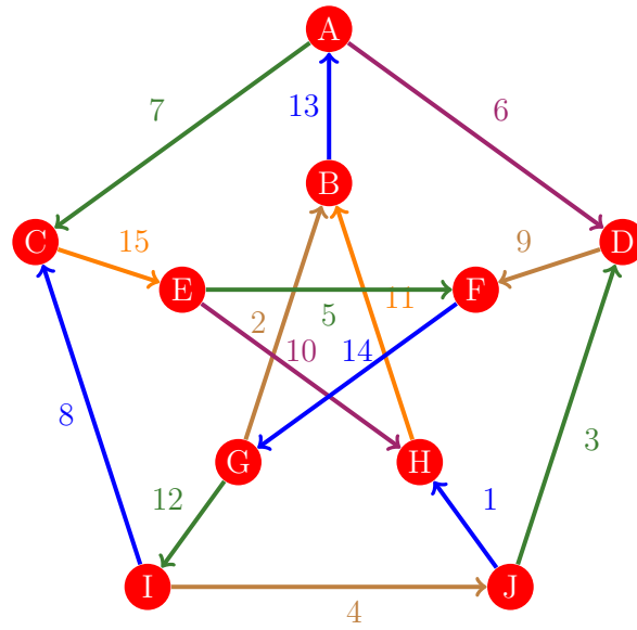
Figura 985: Flujo 977 de la gráfica de Petersen
