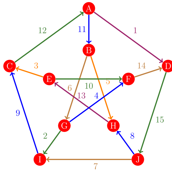
Figura 882: Flujo 874 de la gráfica de Petersen
