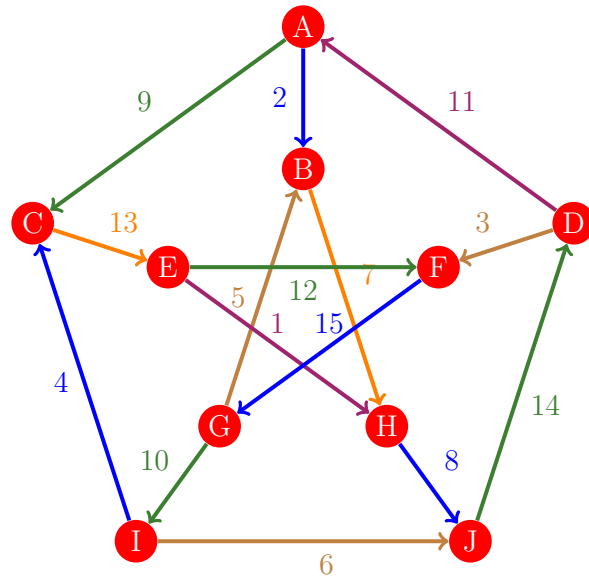
Figura 145: Flujo 137 de la gráfica de Petersen
