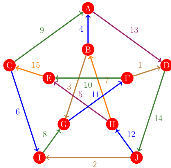
Figura 272: Flujo 264 de la gráfica de Petersen
