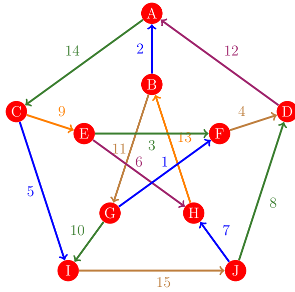
Figura 123: Flujo 115 de la gráfica de Petersen
