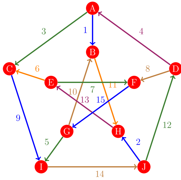
Figura 49: Flujo 41 de la gráfica de Petersen
