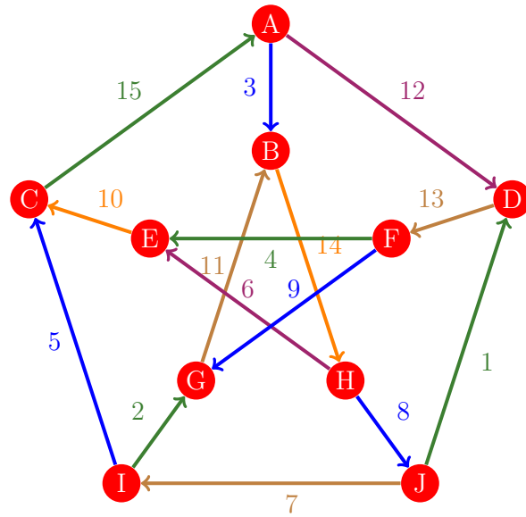
Figura 247: Flujo 239 de la gráfica de Petersen
