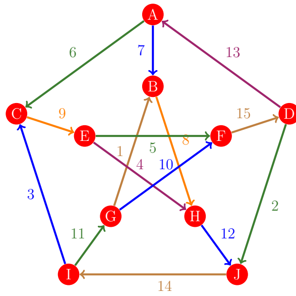
Figura 541: Flujo 533 de la gráfica de Petersen
