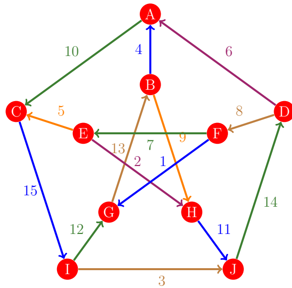
Figura 278: Flujo 270 de la gráfica de Petersen
