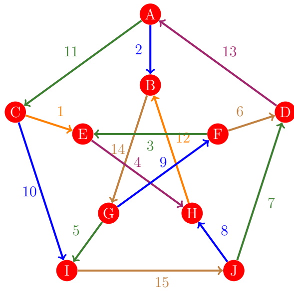
Figura 150: Flujo 142 de la gráfica de Petersen
