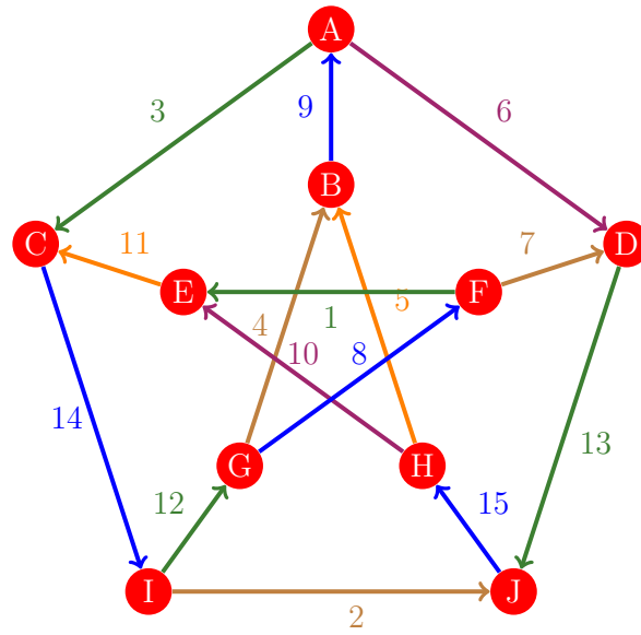
Figura 655: Flujo 647 de la gráfica de Petersen
