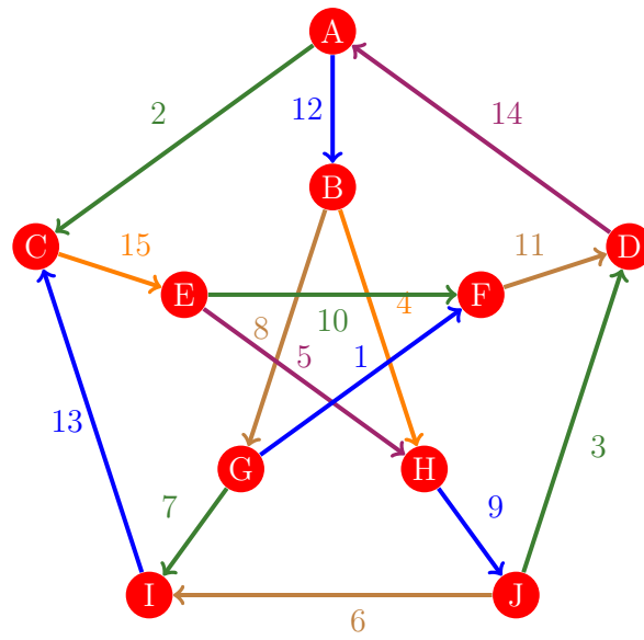
Figura 934: Flujo 926 de la gráfica de Petersen
