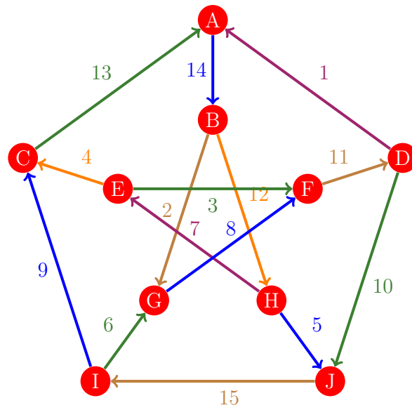
Figura 1122: Flujo 1114 de la gráfica de Petersen
