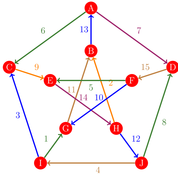
Figura 983: Flujo 975 de la gráfica de Petersen
