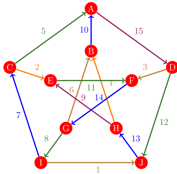
Figura 736: Flujo 728 de la gráfica de Petersen
