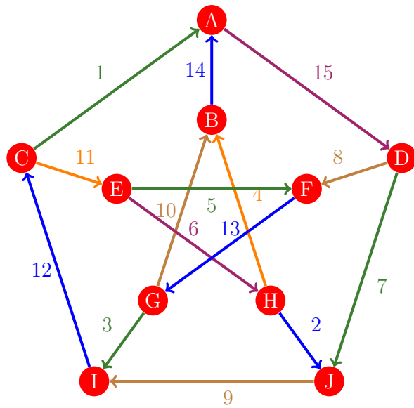
Figura 1084: Flujo 1076 de la gráfica de Petersen
