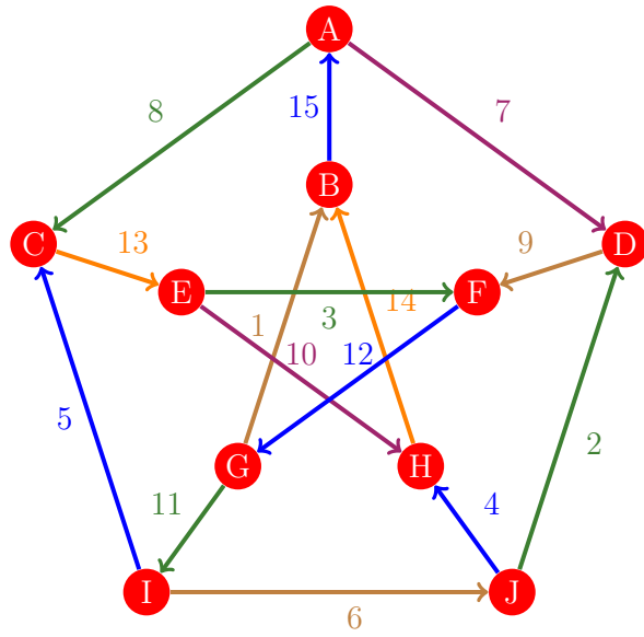
Figura 1150: Flujo 1142 de la gráfica de Petersen
