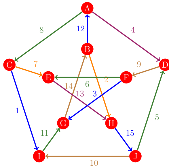
Figura 910: Flujo 902 de la gráfica de Petersen
