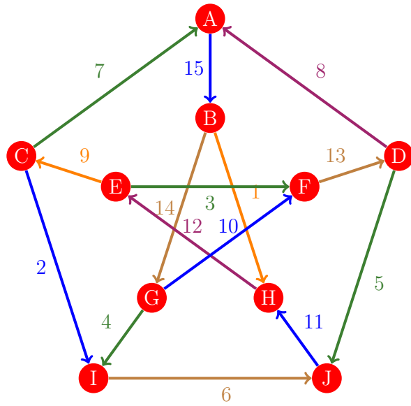
Figura 1185: Flujo 1177 de la gráfica de Petersen
