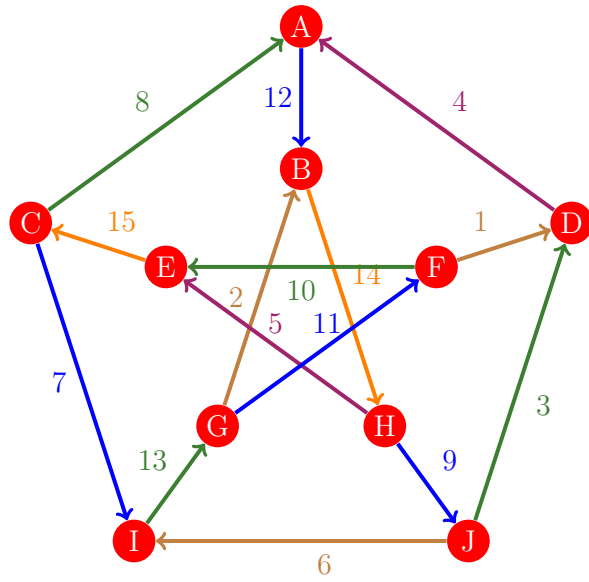
Figura 948: Flujo 940 de la gráfica de Petersen
