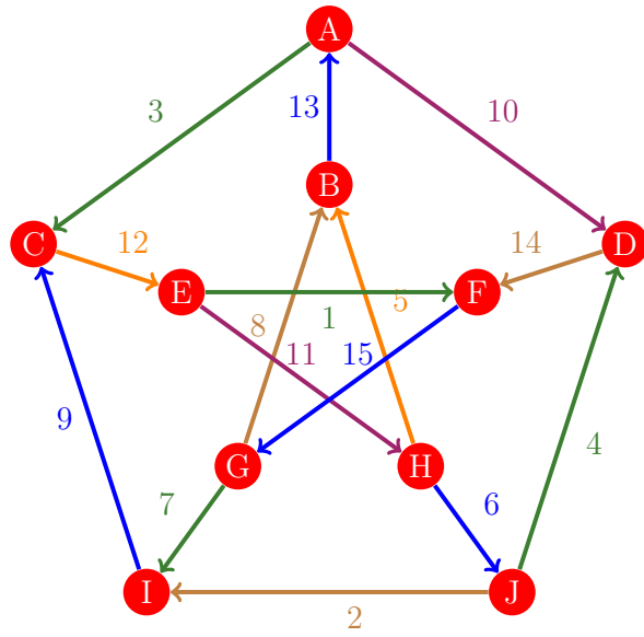
Figura 974: Flujo 966 de la gráfica de Petersen
