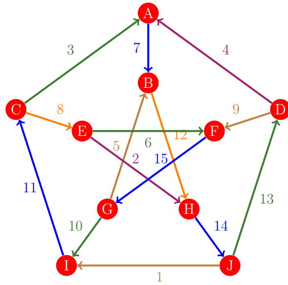
Figura 533: Flujo 525 de la gráfica de Petersen
