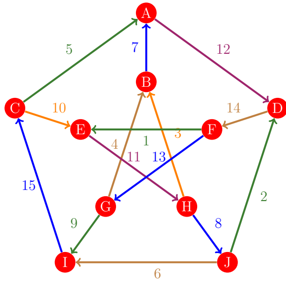
Figura 497: Flujo 489 de la gráfica de Petersen
