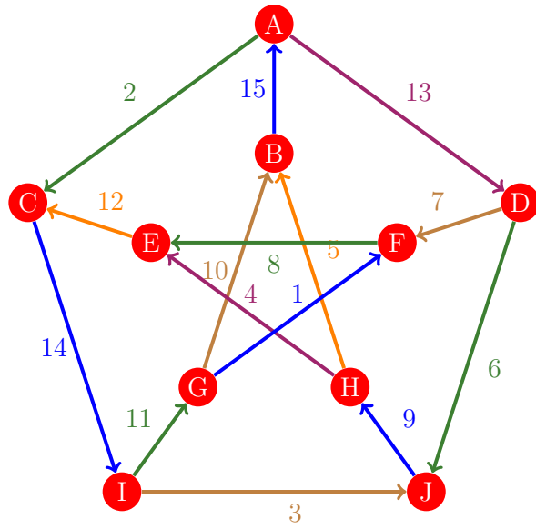
Figura 1130: Flujo 1122 de la gráfica de Petersen
