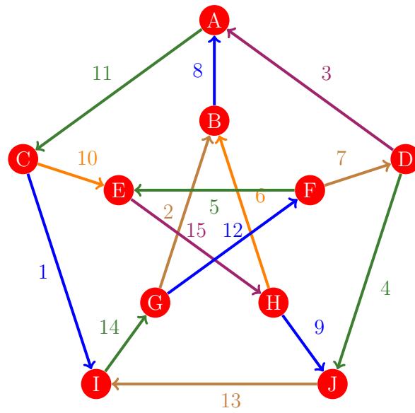
Figura 596: Flujo 588 de la gráfica de Petersen
