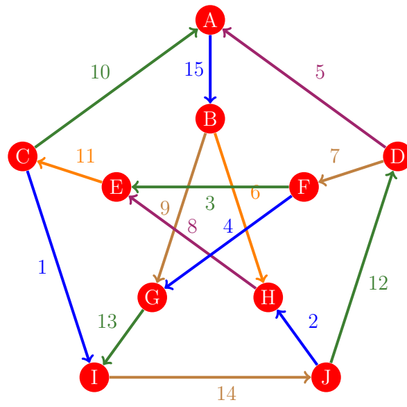
Figura 1197: Flujo 1189 de la gráfica de Petersen
