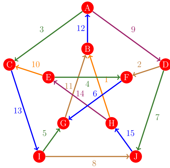
Figura 897: Flujo 889 de la gráfica de Petersen
