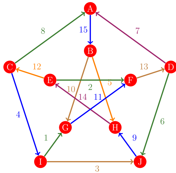
Figura 1188: Flujo 1180 de la gráfica de Petersen
