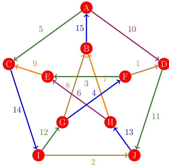
Figura 1136: Flujo 1128 de la gráfica de Petersen
