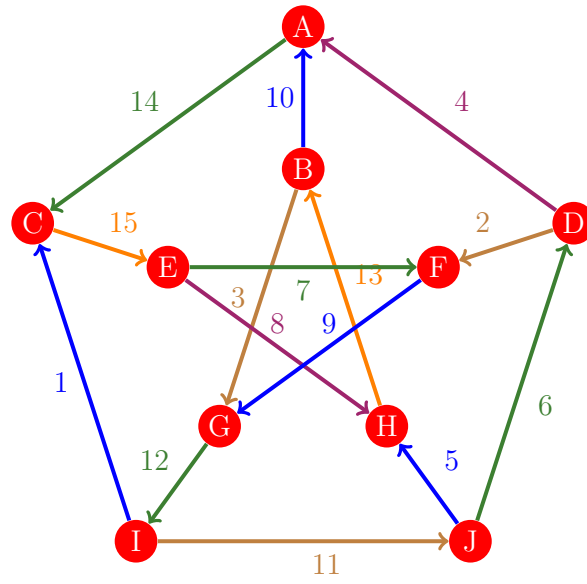
Figura 759: Flujo 751 de la gráfica de Petersen
