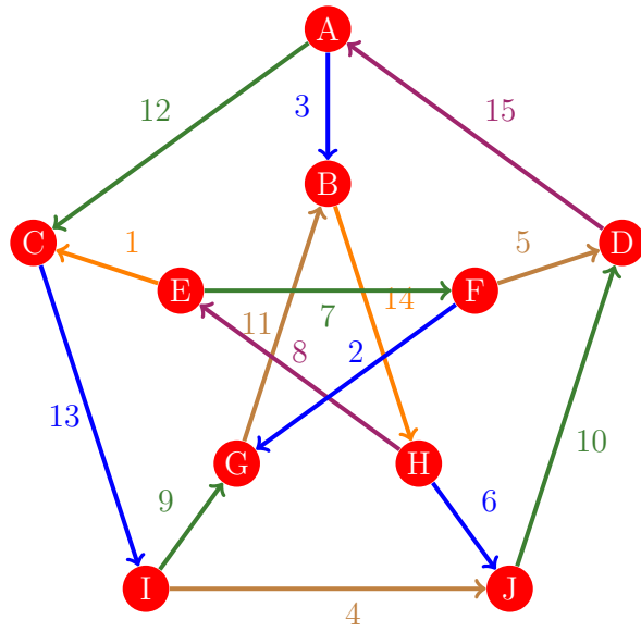
Figura 239: Flujo 231 de la gráfica de Petersen
