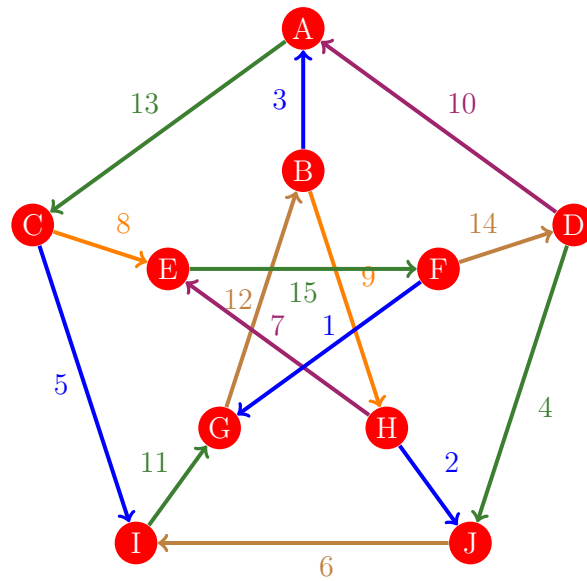
Figura 202: Flujo 194 de la gráfica de Petersen
