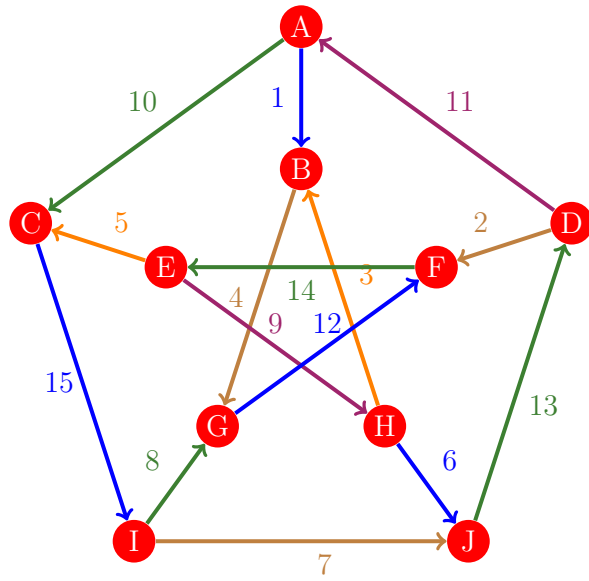
Figura 61: Flujo 53 de la gráfica de Petersen
