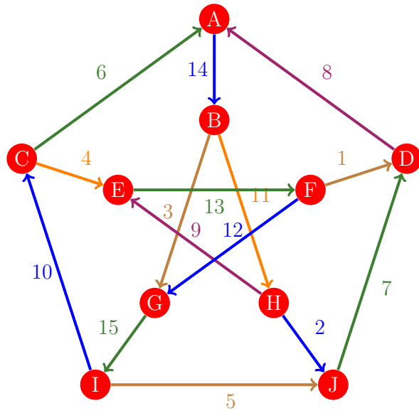
Figura 1103: Flujo 1095 de la gráfica de Petersen
