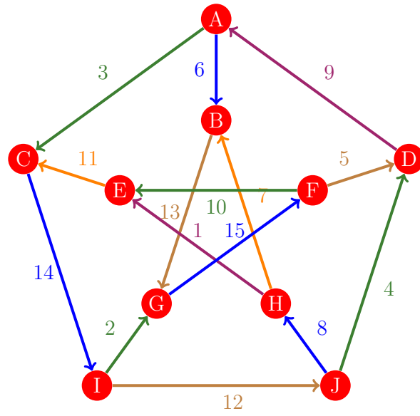
Figura 455: Flujo 447 de la gráfica de Petersen
