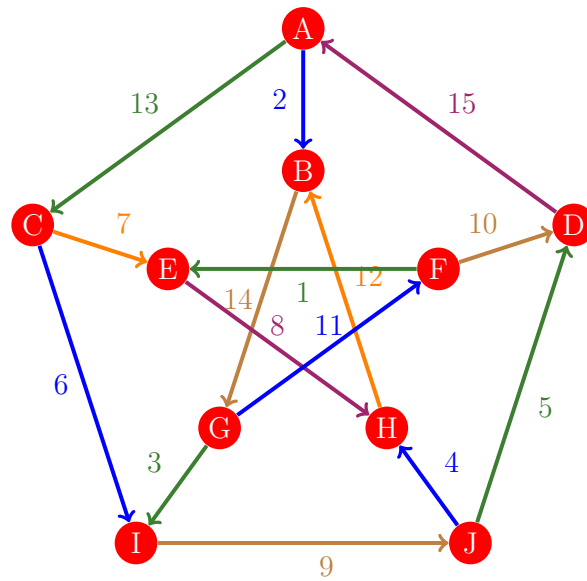
Figura 160: Flujo 152 de la gráfica de Petersen
