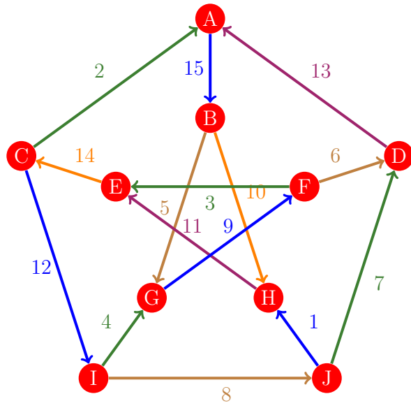
Figura 1169: Flujo 1161 de la gráfica de Petersen
