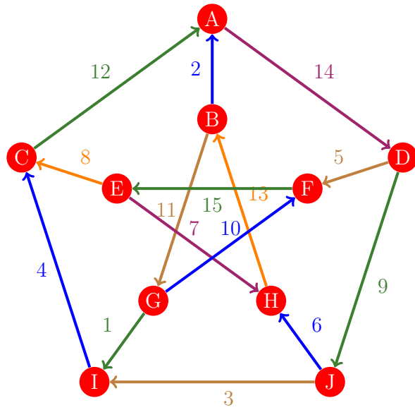
Figura 113: Flujo 105 de la gráfica de Petersen
