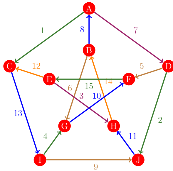
Figura 592: Flujo 584 de la gráfica de Petersen
