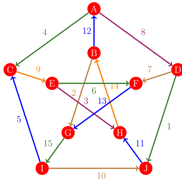
Figura 900: Flujo 892 de la gráfica de Petersen
