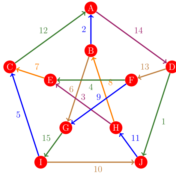
Figura 111: Flujo 103 de la gráfica de Petersen
