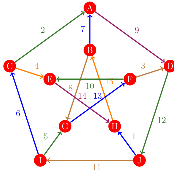
Figura 489: Flujo 481 de la gráfica de Petersen
