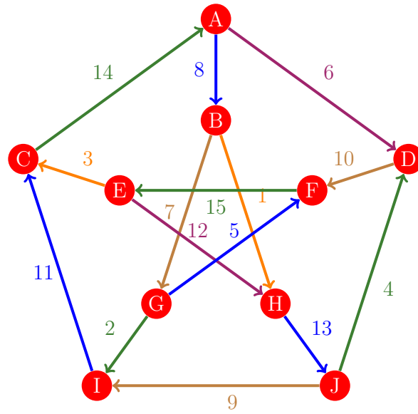
Figura 643: Flujo 635 de la gráfica de Petersen
