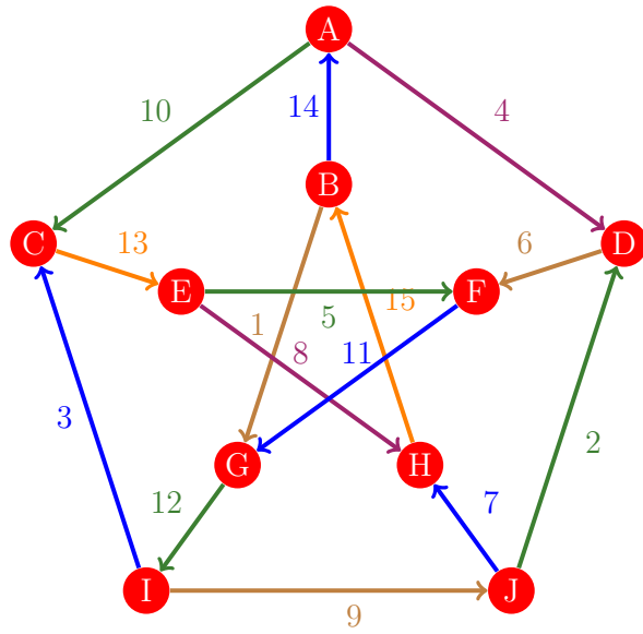
Figura 1069: Flujo 1061 de la gráfica de Petersen
