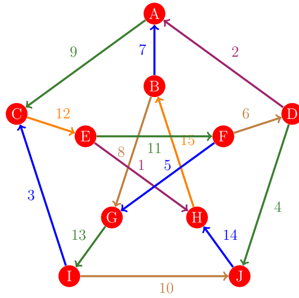
Figura 517: Flujo 509 de la gráfica de Petersen
