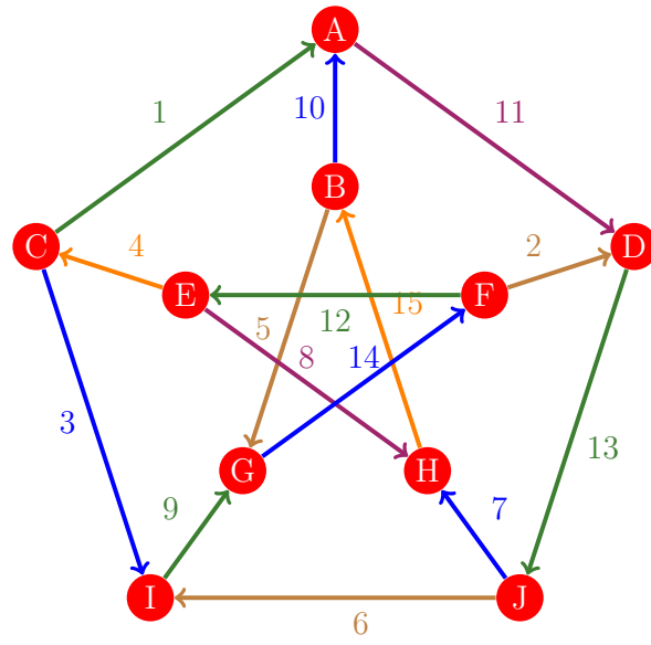
Figura 747: Flujo 739 de la gráfica de Petersen
