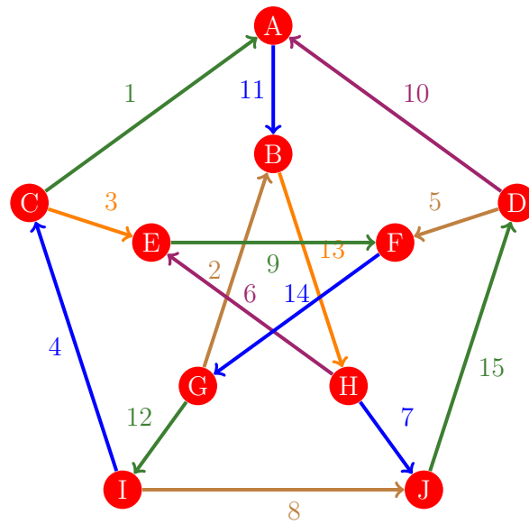
Figura 876: Flujo 868 de la gráfica de Petersen
