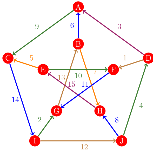
Figura 435: Flujo 427 de la gráfica de Petersen
