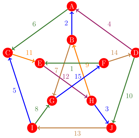
Figura 95: Flujo 87 de la gráfica de Petersen
