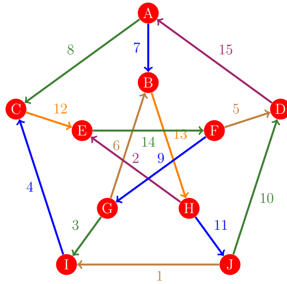
Figura 553: Flujo 545 de la gráfica de Petersen
