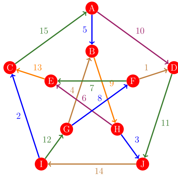
Figura 401: Flujo 393 de la gráfica de Petersen
