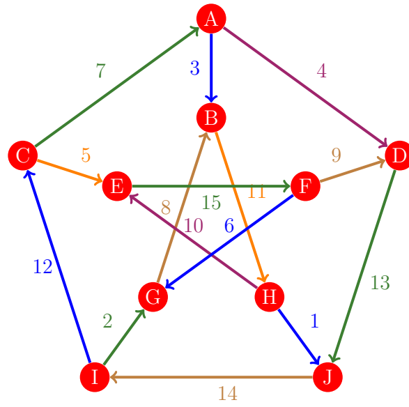
Figura 219: Flujo 211 de la gráfica de Petersen
