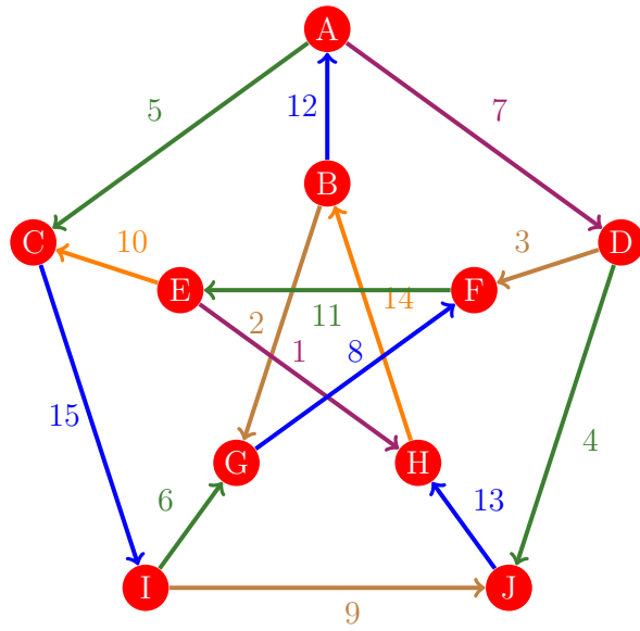
Figura 903: Flujo 895 de la gráfica de Petersen
