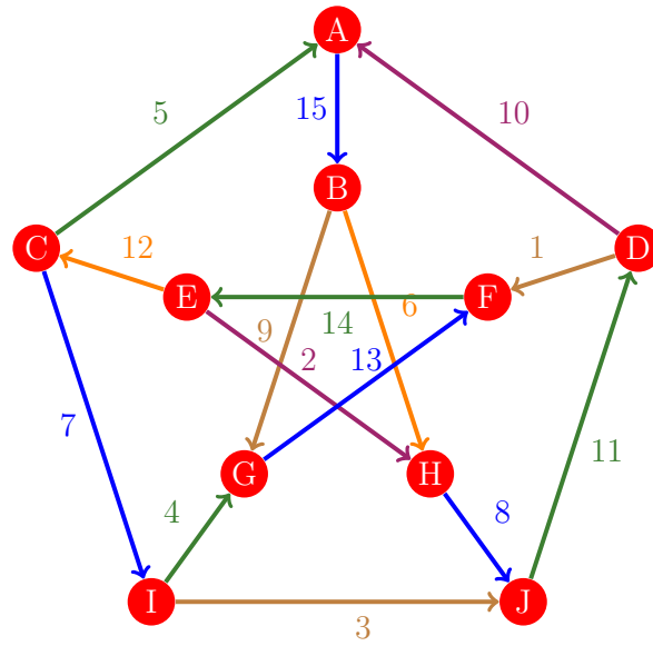
Figura 1177: Flujo 1169 de la gráfica de Petersen
