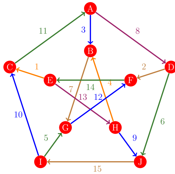
Figura 232: Flujo 224 de la gráfica de Petersen
