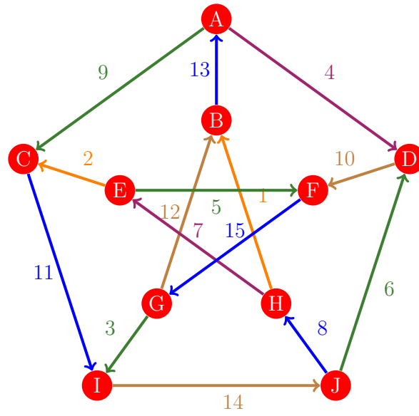
Figura 991: Flujo 983 de la gráfica de Petersen
