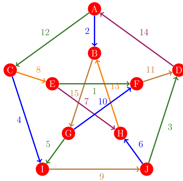
Figura 156: Flujo 148 de la gráfica de Petersen
