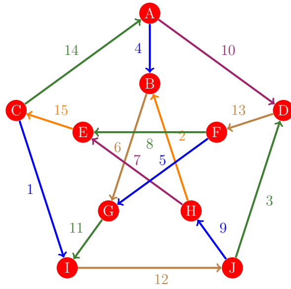
Figura 327: Flujo 319 de la gráfica de Petersen
