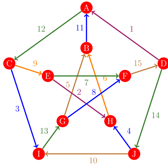
Figura 841: Flujo 833 de la gráfica de Petersen
