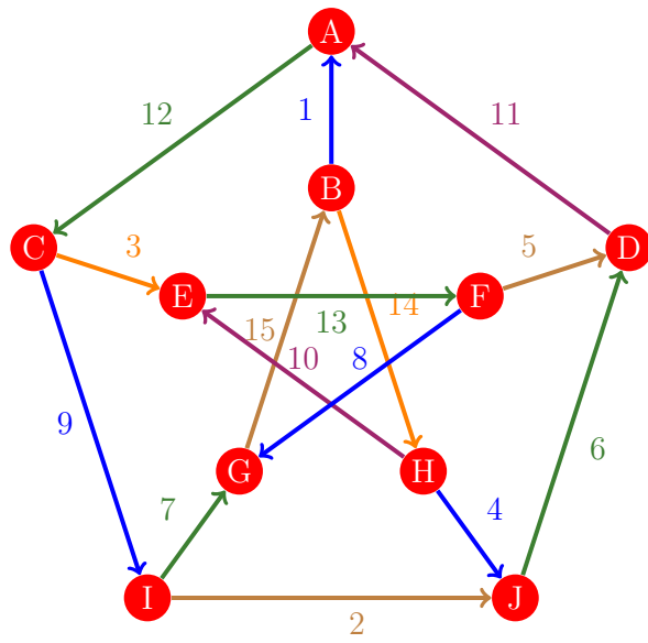
Figura 38: Flujo 30 de la gráfica de Petersen
