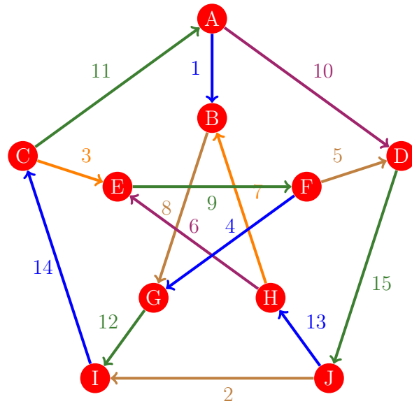
Figura 69: Flujo 61 de la gráfica de Petersen
