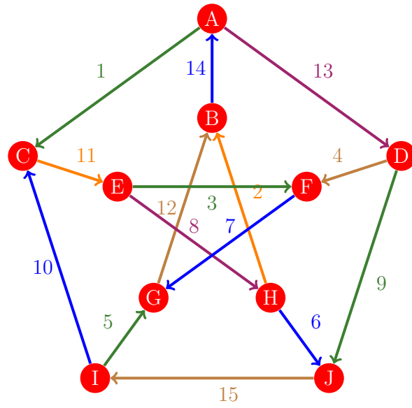
Figura 1085: Flujo 1077 de la gráfica de Petersen
