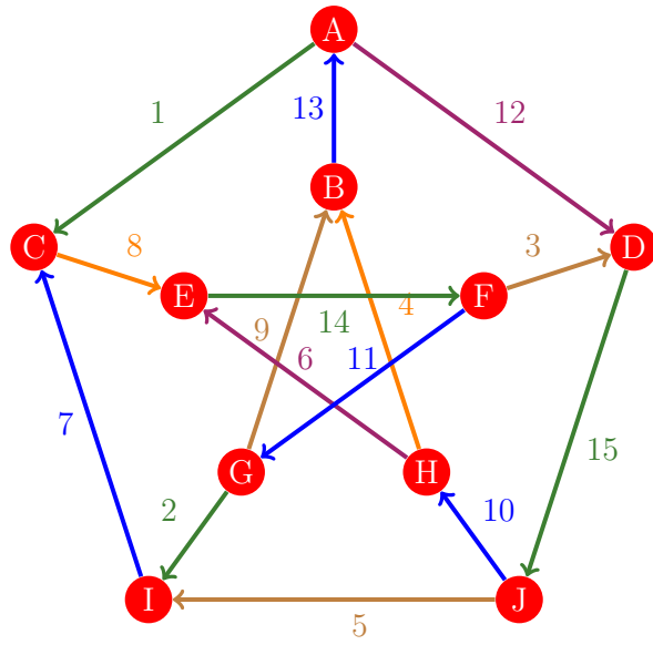
Figura 1004: Flujo 996 de la gráfica de Petersen
