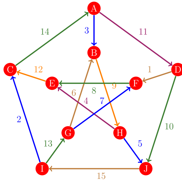
Figura 243: Flujo 235 de la gráfica de Petersen
