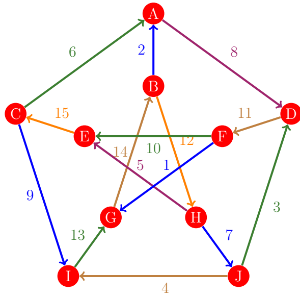
Figura 94: Flujo 86 de la gráfica de Petersen
