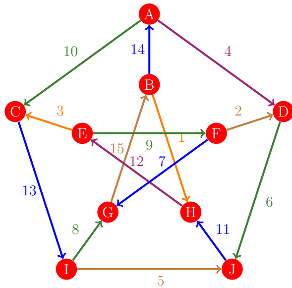
Figura 1070: Flujo 1062 de la gráfica de Petersen
