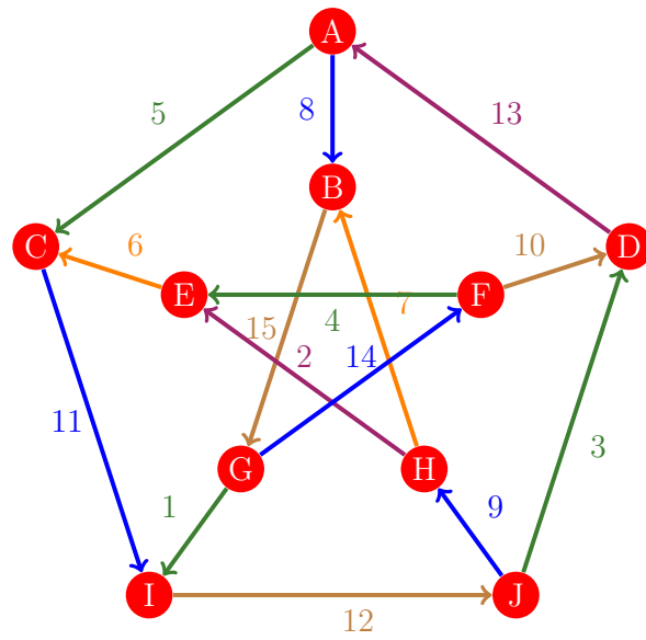
Figura 618: Flujo 610 de la gráfica de Petersen
