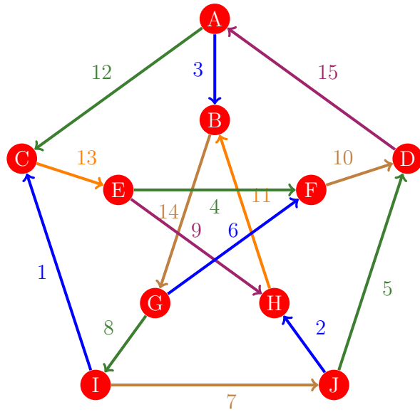
Figura 240: Flujo 232 de la gráfica de Petersen
