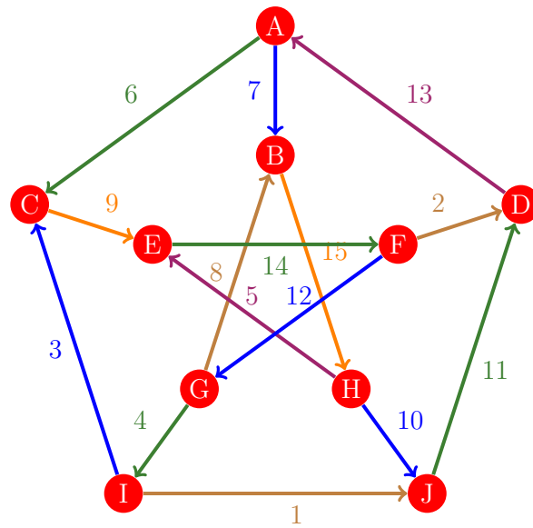
Figura 542: Flujo 534 de la gráfica de Petersen
