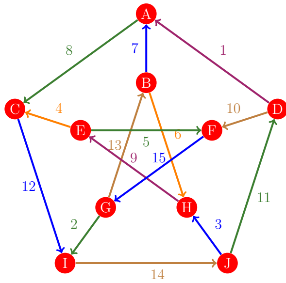
Figura 516: Flujo 508 de la gráfica de Petersen
