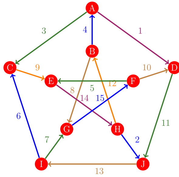
Figura 253: Flujo 245 de la gráfica de Petersen
