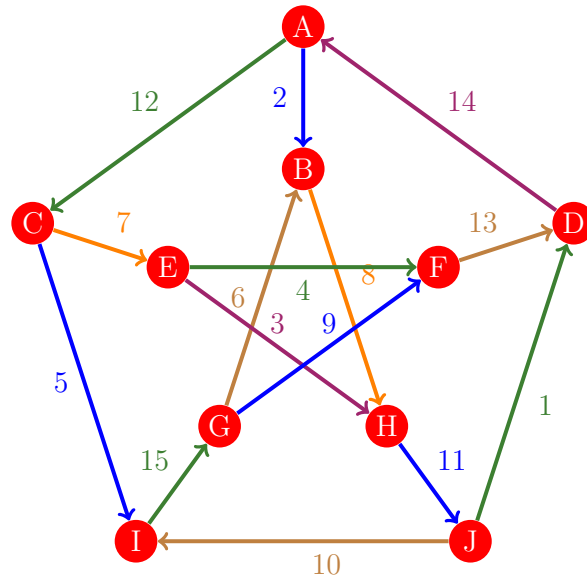
Figura 151: Flujo 143 de la gráfica de Petersen
