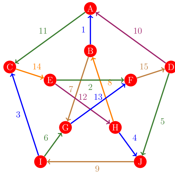
Figura 30: Flujo 22 de la gráfica de Petersen
