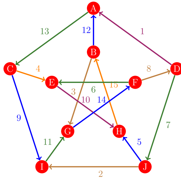
Figura 919: Flujo 911 de la gráfica de Petersen
