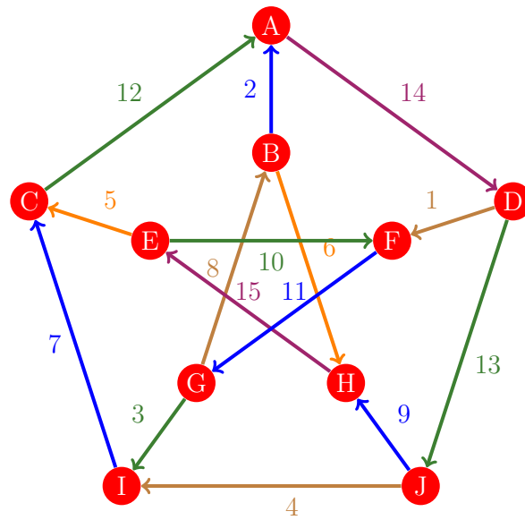
Figura 112: Flujo 104 de la gráfica de Petersen
