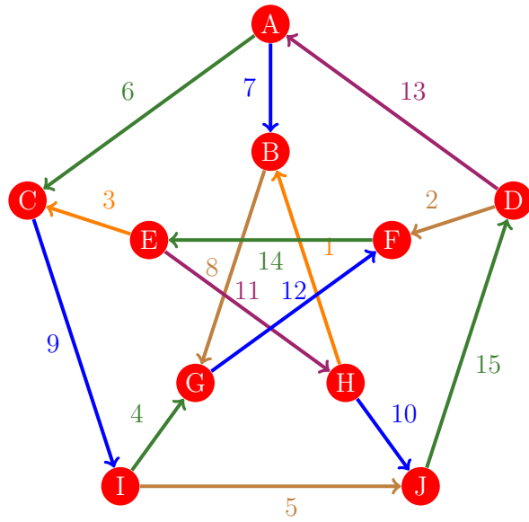
Figura 543: Flujo 535 de la gráfica de Petersen
