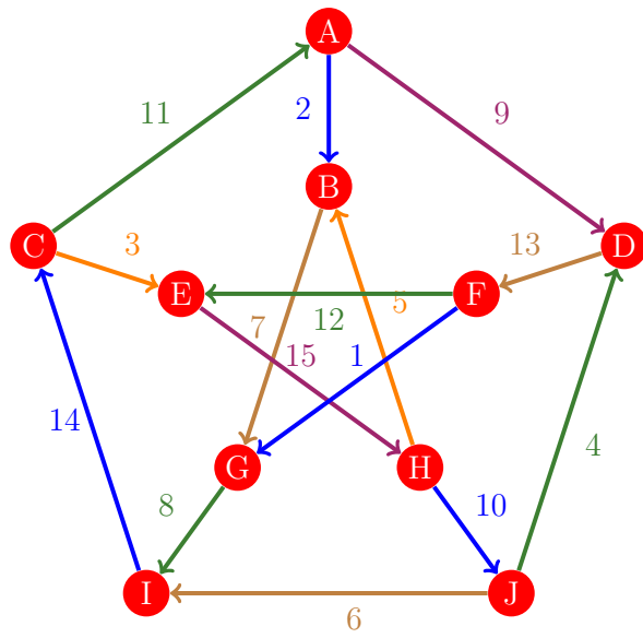
Figura 148: Flujo 140 de la gráfica de Petersen
