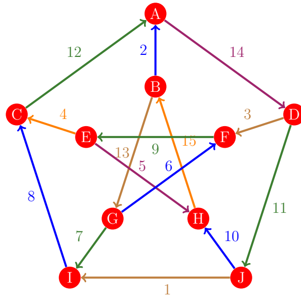
Figura 115: Flujo 107 de la gráfica de Petersen
