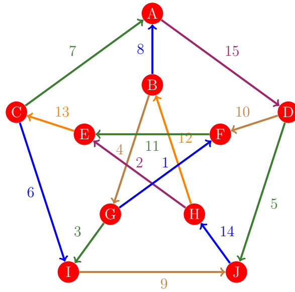
Figura 583: Flujo 575 de la gráfica de Petersen
