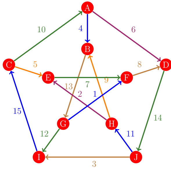
Figura 316: Flujo 308 de la gráfica de Petersen
