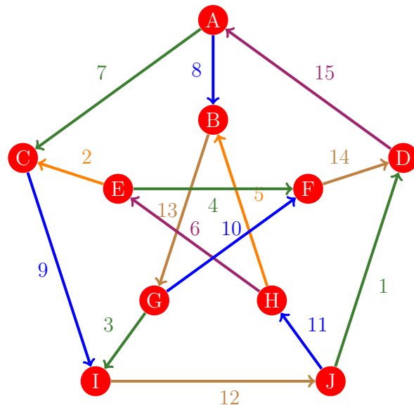
Figura 630: Flujo 622 de la gráfica de Petersen
