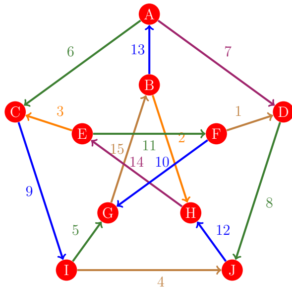
Figura 984: Flujo 976 de la gráfica de Petersen
