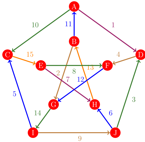
Figura 828: Flujo 820 de la gráfica de Petersen
