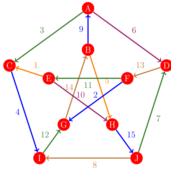
Figura 658: Flujo 650 de la gráfica de Petersen
