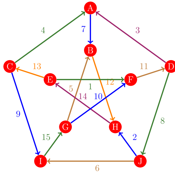
Figura 535: Flujo 527 de la gráfica de Petersen
