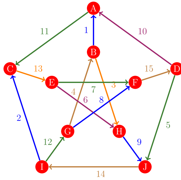
Figura 29: Flujo 21 de la gráfica de Petersen
