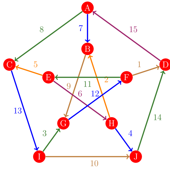
Figura 555: Flujo 547 de la gráfica de Petersen
