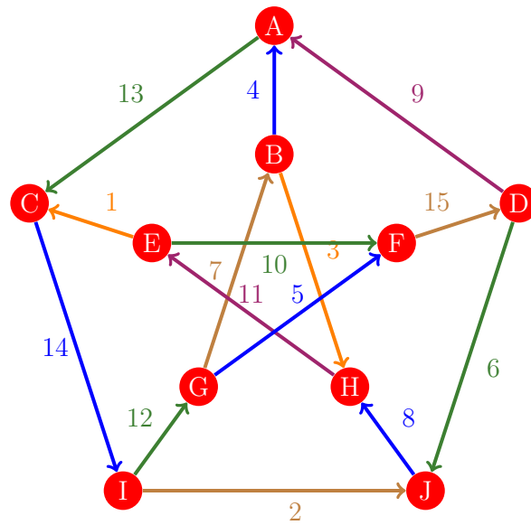
Figura 284: Flujo 276 de la gráfica de Petersen
