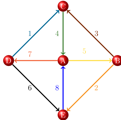
Figura 6: Gráfica G = (5, 8) con flujo elegante.
