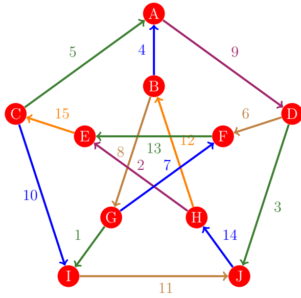
Figura 257: Flujo 249 de la gráfica de Petersen
