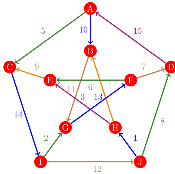
Figura 780: Flujo 772 de la gráfica de Petersen
