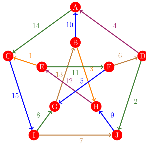
Figura 760: Flujo 752 de la gráfica de Petersen
