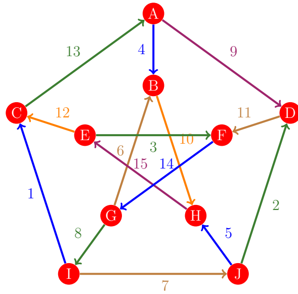
Figura 323: Flujo 315 de la gráfica de Petersen
