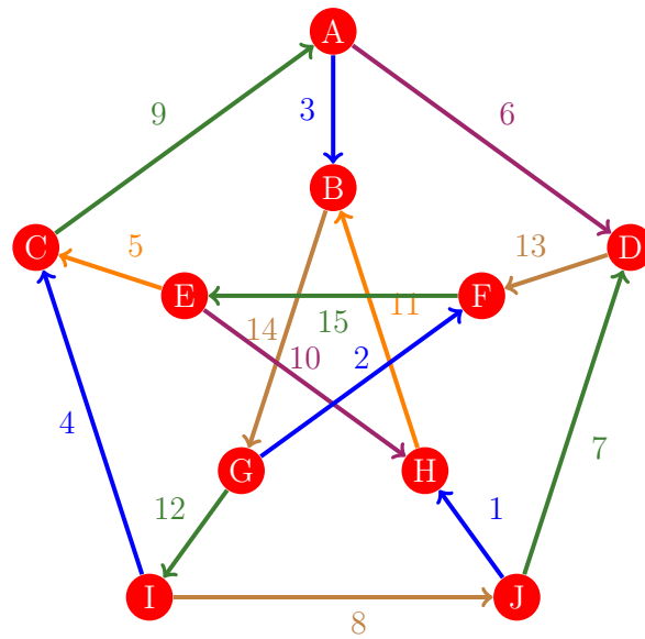
Figura 226: Flujo 218 de la gráfica de Petersen
