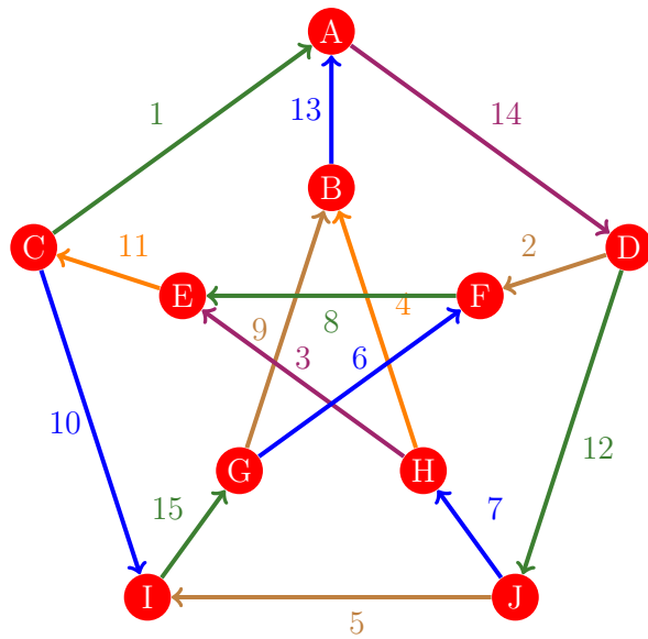
Figura 1002: Flujo 994 de la gráfica de Petersen
