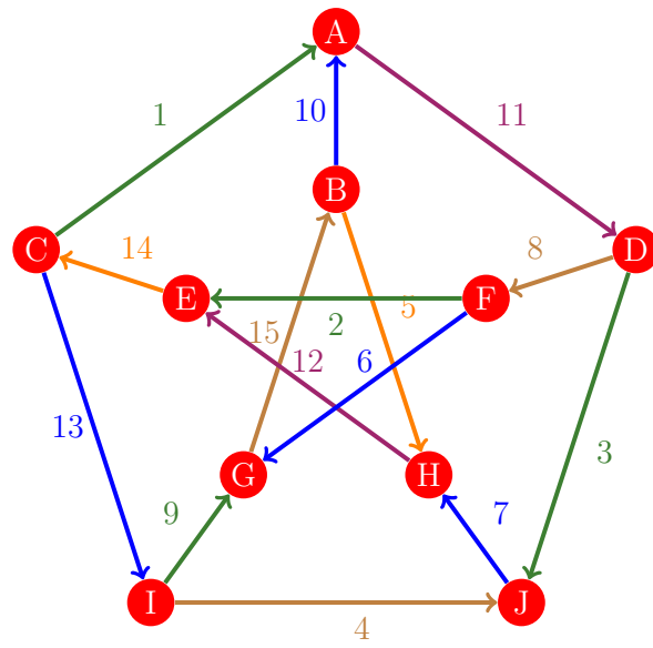
Figura 750: Flujo 742 de la gráfica de Petersen
