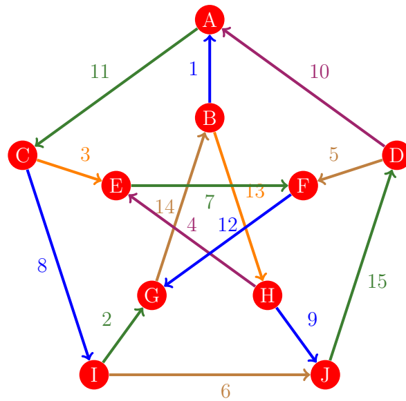
Figura 34: Flujo 26 de la gráfica de Petersen
