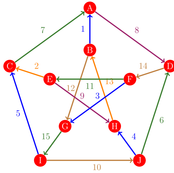
Figura 15: Flujo 7 de la gráfica de Petersen
