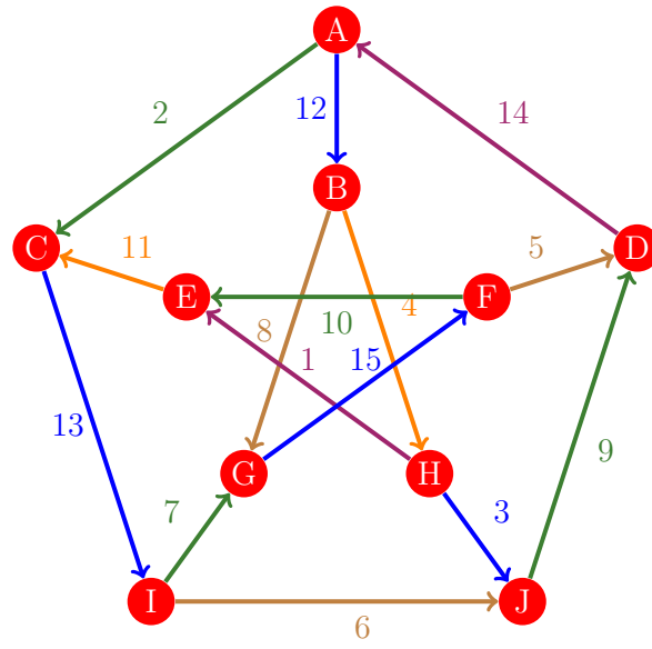
Figura 933: Flujo 925 de la gráfica de Petersen
