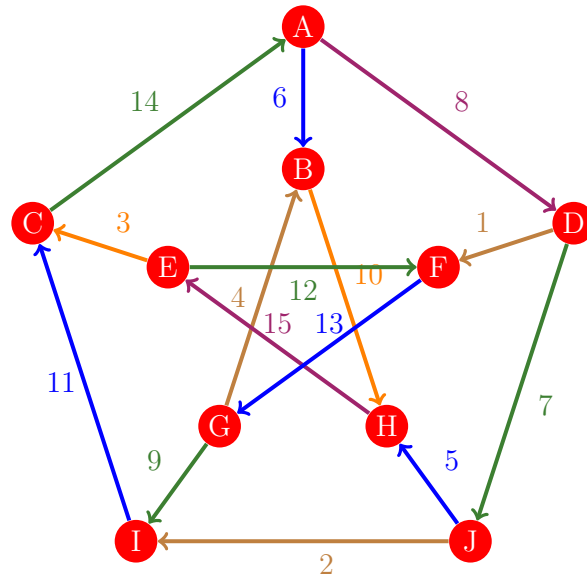
Figura 485: Flujo 477 de la gráfica de Petersen
