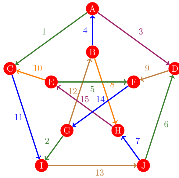
Figura 256: Flujo 248 de la gráfica de Petersen
