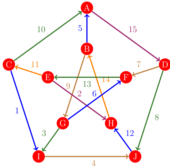
Figura 349: Flujo 341 de la gráfica de Petersen
