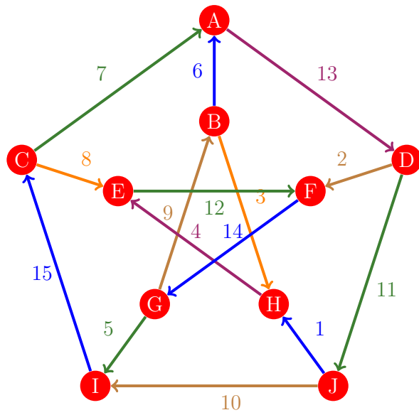
Figura 424: Flujo 416 de la gráfica de Petersen
