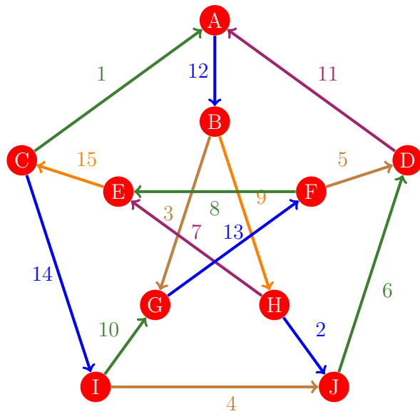
Figura 956: Flujo 948 de la gráfica de Petersen
