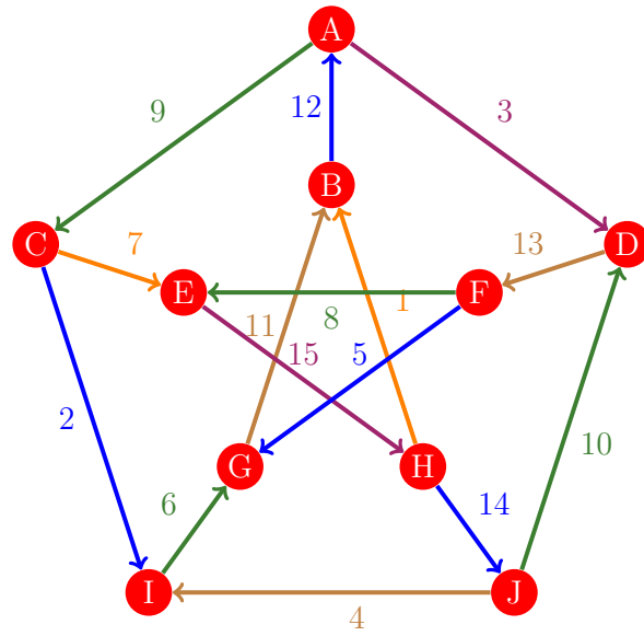
Figura 911: Flujo 903 de la gráfica de Petersen
