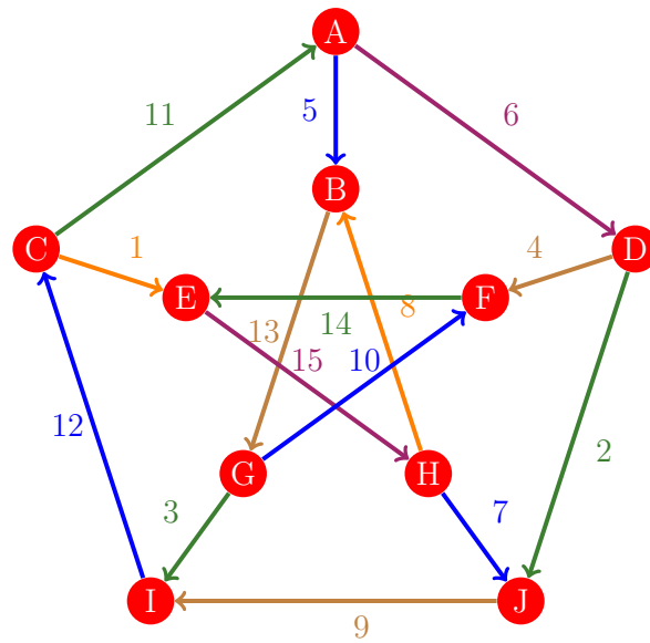
Figura 394: Flujo 386 de la gráfica de Petersen
