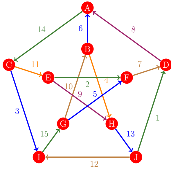
Figura 446: Flujo 438 de la gráfica de Petersen
