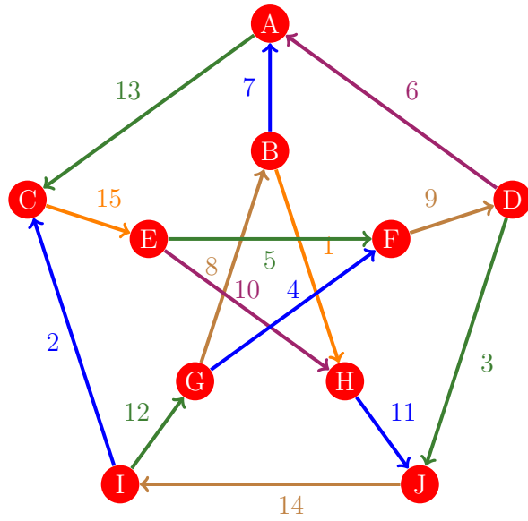
Figura 522: Flujo 514 de la gráfica de Petersen
