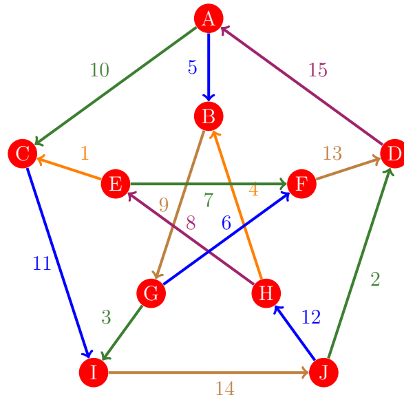
Figura 389: Flujo 381 de la gráfica de Petersen
