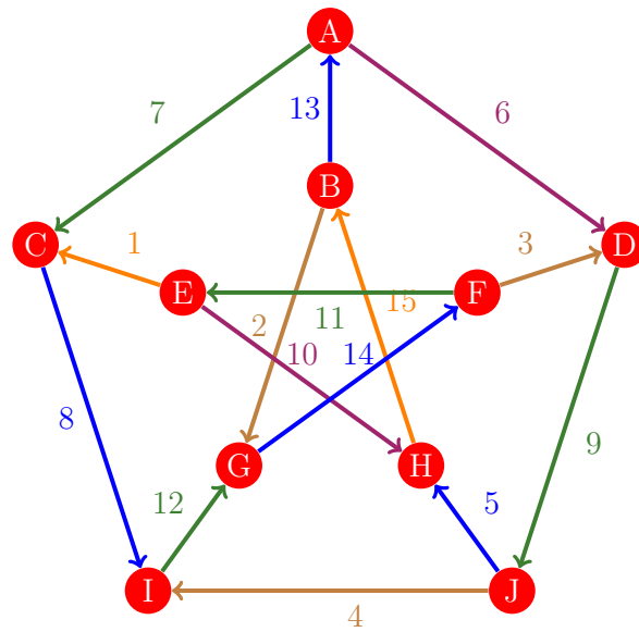
Figura 986: Flujo 978 de la gráfica de Petersen
