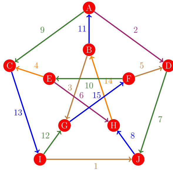
Figura 825: Flujo 817 de la gráfica de Petersen
