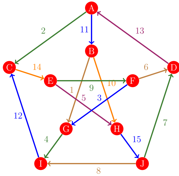
Figura 852: Flujo 844 de la gráfica de Petersen
