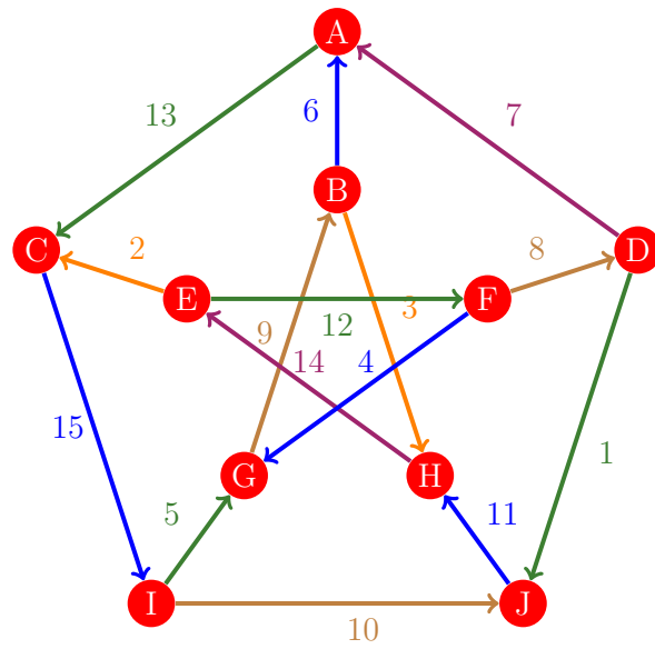
Figura 444: Flujo 436 de la gráfica de Petersen
