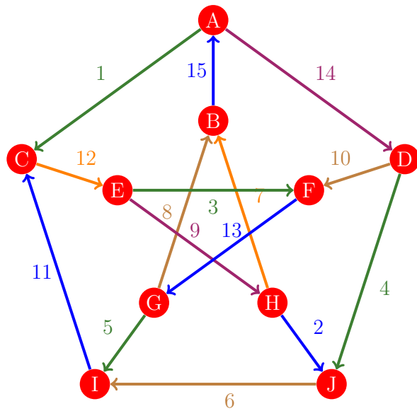
Figura 1168: Flujo 1160 de la gráfica de Petersen
