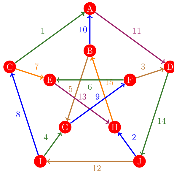
Figura 745: Flujo 737 de la gráfica de Petersen
