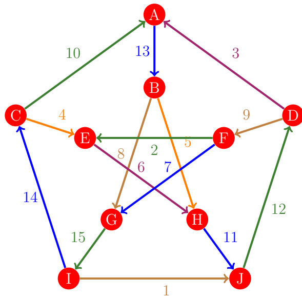
Figura 1036: Flujo 1028 de la gráfica de Petersen
