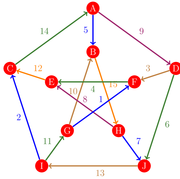
Figura 399: Flujo 391 de la gráfica de Petersen
