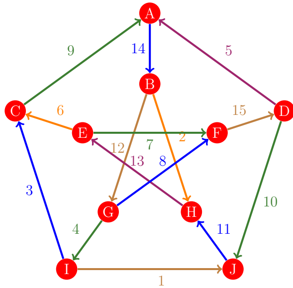
Figura 1108: Flujo 1100 de la gráfica de Petersen
