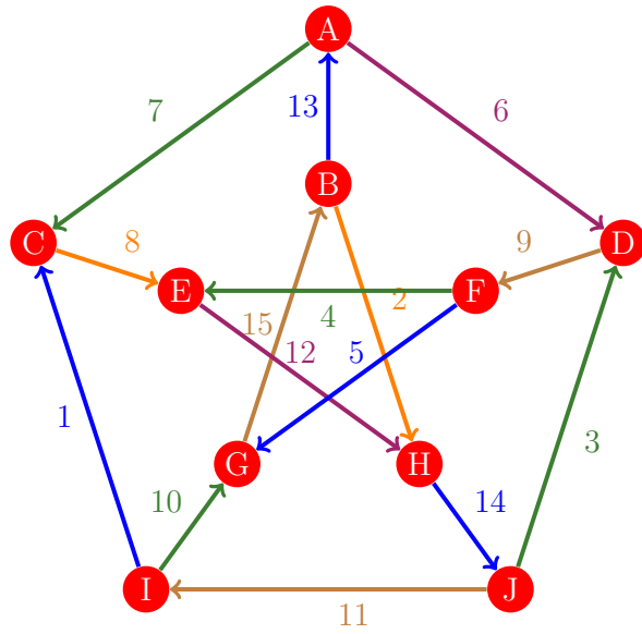
Figura 988: Flujo 980 de la gráfica de Petersen
