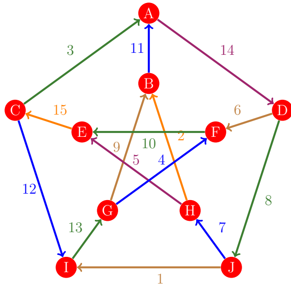
Figura 813: Flujo 805 de la gráfica de Petersen
