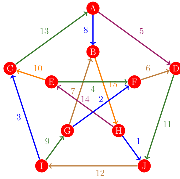
Figura 641: Flujo 633 de la gráfica de Petersen
