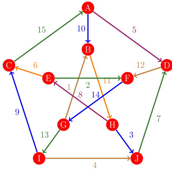
Figura 803: Flujo 795 de la gráfica de Petersen
