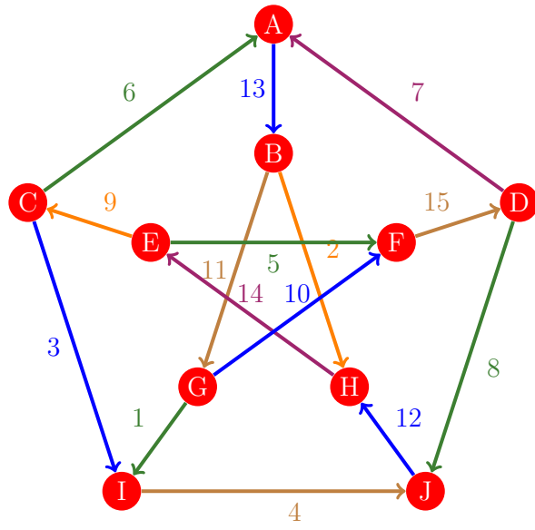
Figura 1023: Flujo 1015 de la gráfica de Petersen
