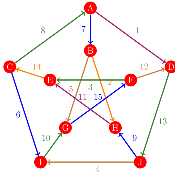
Figura 549: Flujo 541 de la gráfica de Petersen
