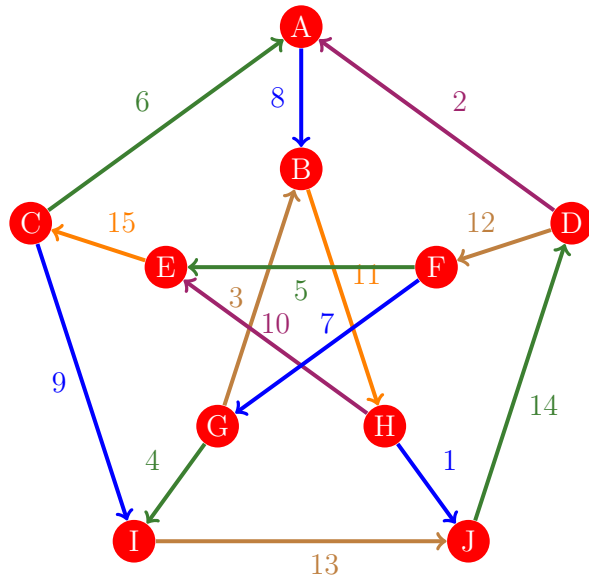
Figura 619: Flujo 611 de la gráfica de Petersen
