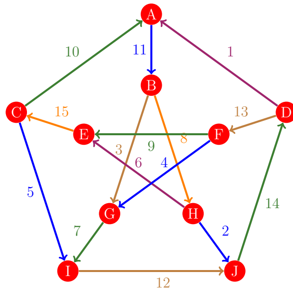
Figura 870: Flujo 862 de la gráfica de Petersen
