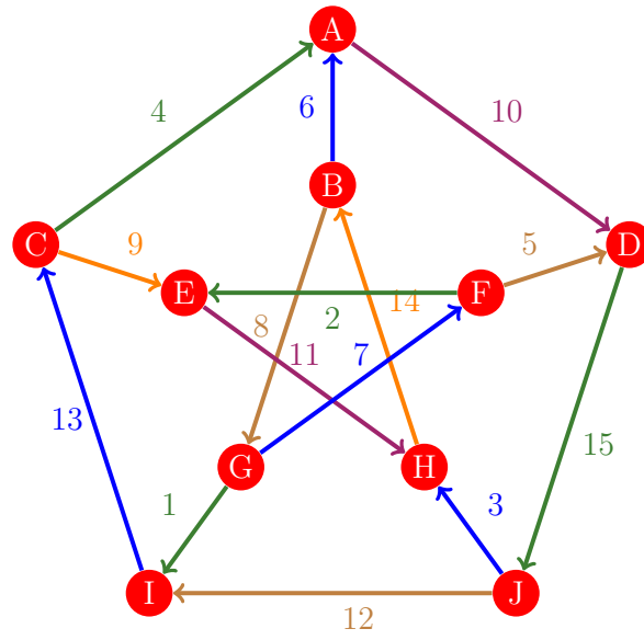
Figura 417: Flujo 409 de la gráfica de Petersen
