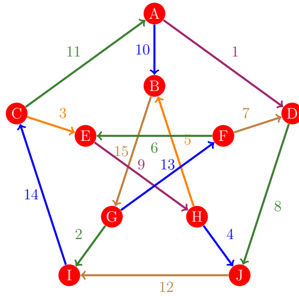
Figura 795: Flujo 787 de la gráfica de Petersen
