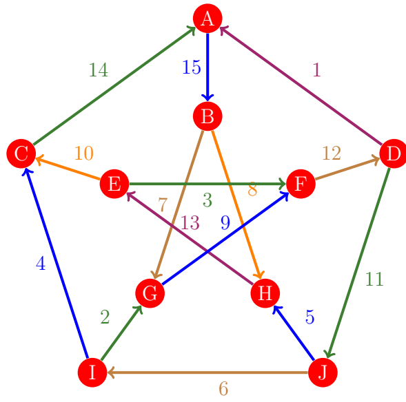
Figura 1205: Flujo 1197 de la gráfica de Petersen
