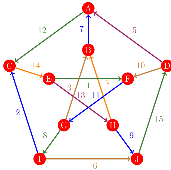
Figura 520: Flujo 512 de la gráfica de Petersen
