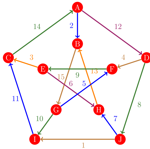
Figura 166: Flujo 158 de la gráfica de Petersen
