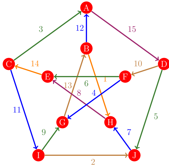
Figura 896: Flujo 888 de la gráfica de Petersen
