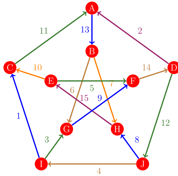
Figura 1037: Flujo 1029 de la gráfica de Petersen
