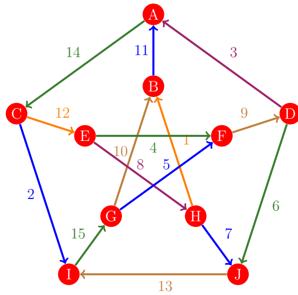
Figura 846: Flujo 838 de la gráfica de Petersen
