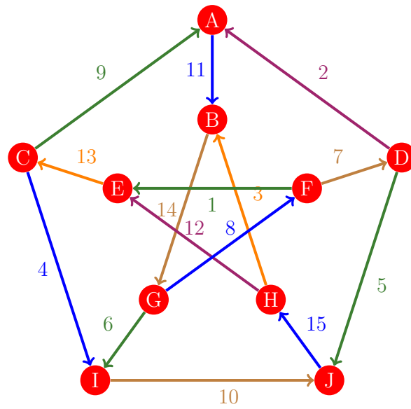
Figura 866: Flujo 858 de la gráfica de Petersen
