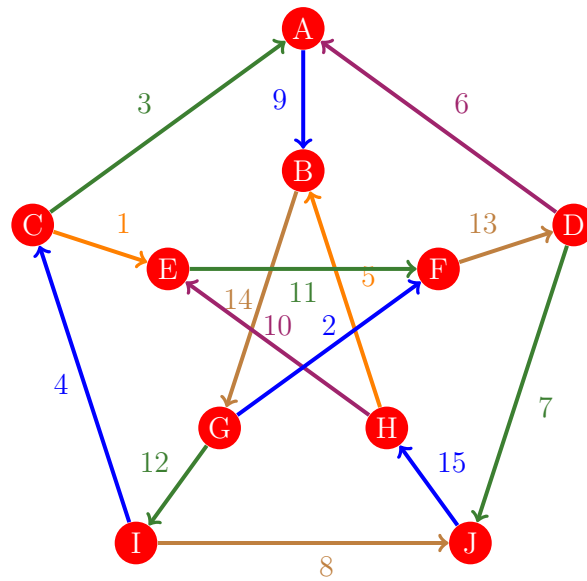
Figura 696: Flujo 688 de la gráfica de Petersen
