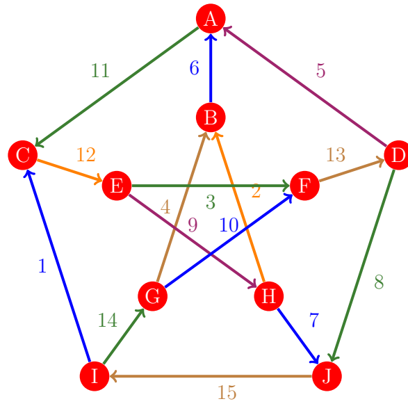
Figura 439: Flujo 431 de la gráfica de Petersen
