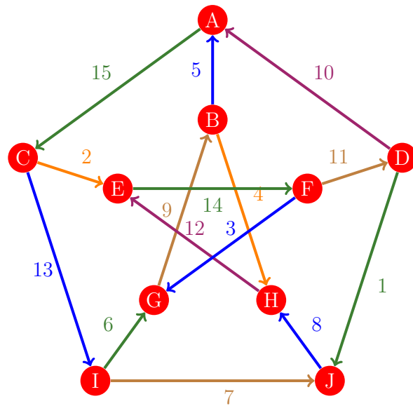
Figura 364: Flujo 356 de la gráfica de Petersen
