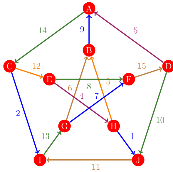
Figura 686: Flujo 678 de la gráfica de Petersen
