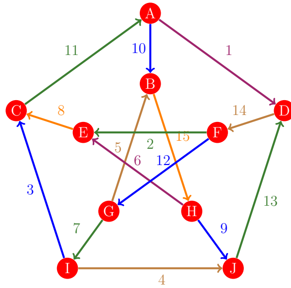
Figura 791: Flujo 783 de la gráfica de Petersen
