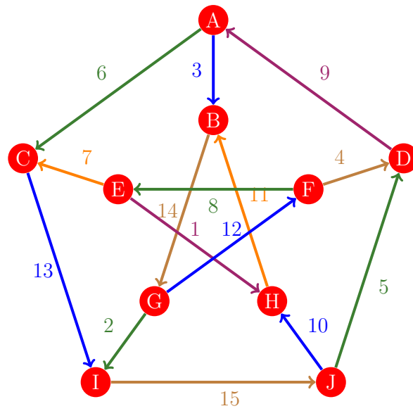
Figura 218: Flujo 210 de la gráfica de Petersen
