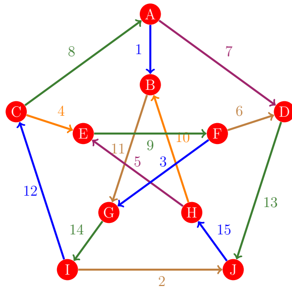
Figura 58: Flujo 50 de la gráfica de Petersen
