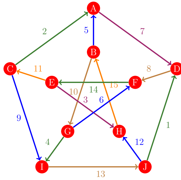
Figura 329: Flujo 321 de la gráfica de Petersen
