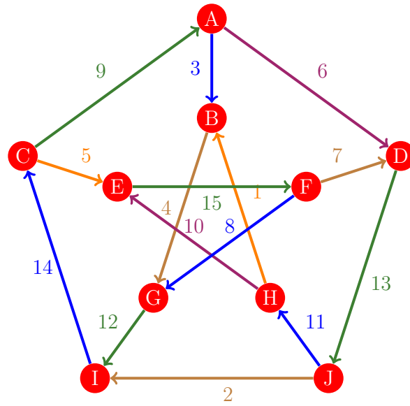
Figura 223: Flujo 215 de la gráfica de Petersen
