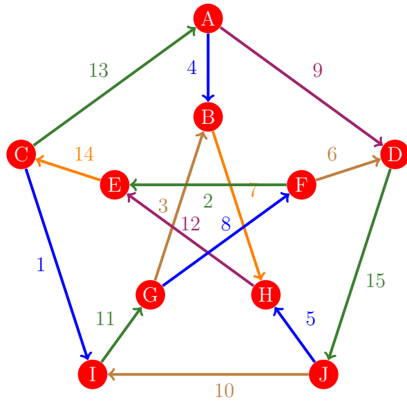
Figura 325: Flujo 317 de la gráfica de Petersen
