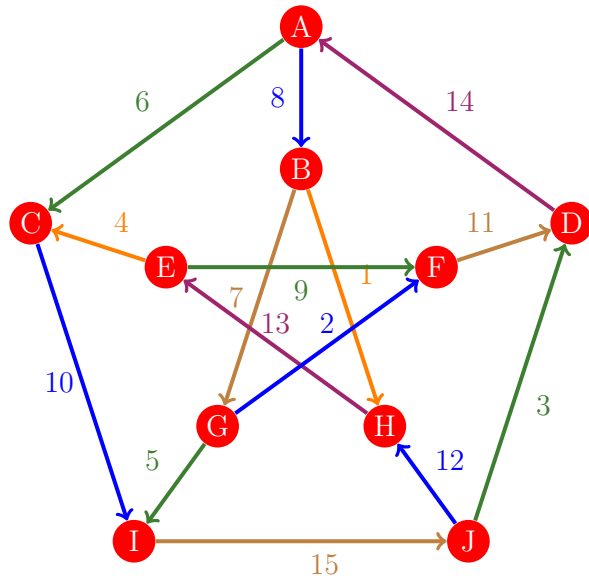
Figura 621: Flujo 613 de la gráfica de Petersen
