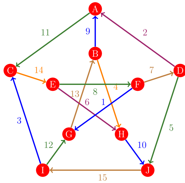
Figura 678: Flujo 670 de la gráfica de Petersen
