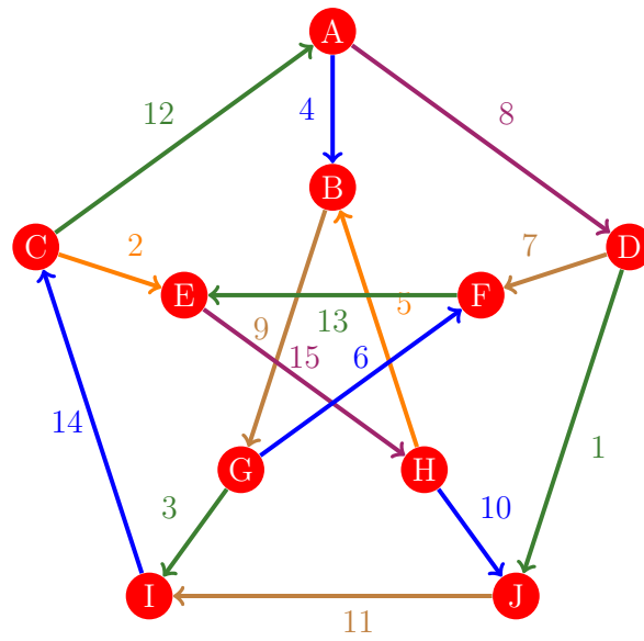
Figura 322: Flujo 314 de la gráfica de Petersen
