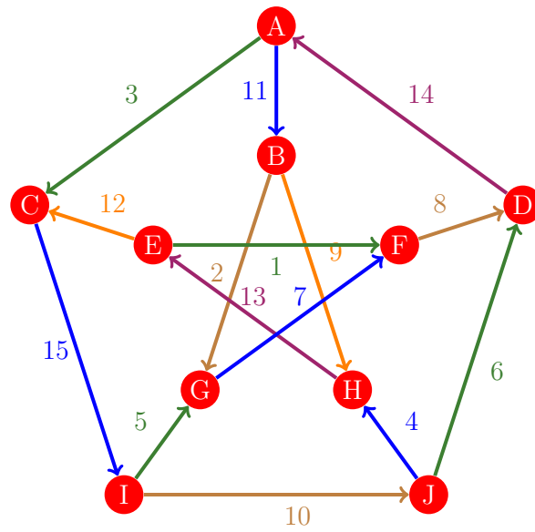
Figura 858: Flujo 850 de la gráfica de Petersen
