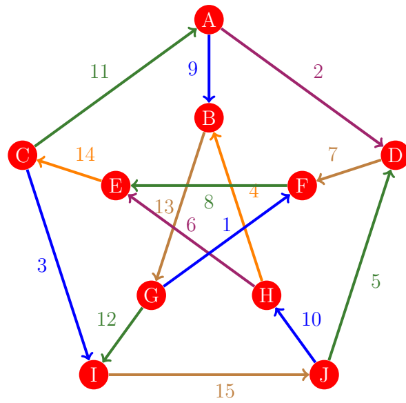
Figura 718: Flujo 710 de la gráfica de Petersen
