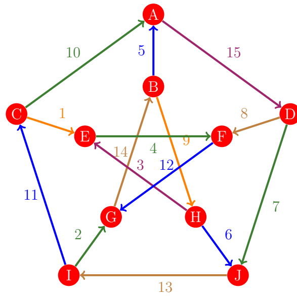
Figura 352: Flujo 344 de la gráfica de Petersen
