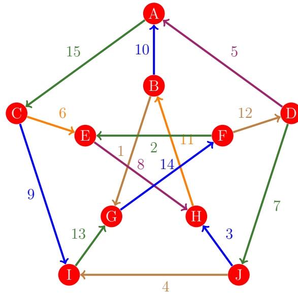
Figura 763: Flujo 755 de la gráfica de Petersen
