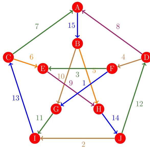
Figura 1184: Flujo 1176 de la gráfica de Petersen
