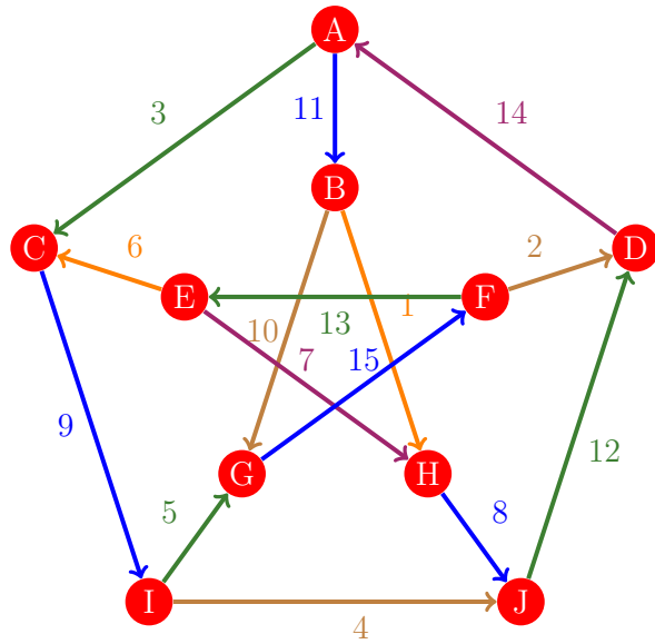
Figura 856: Flujo 848 de la gráfica de Petersen
