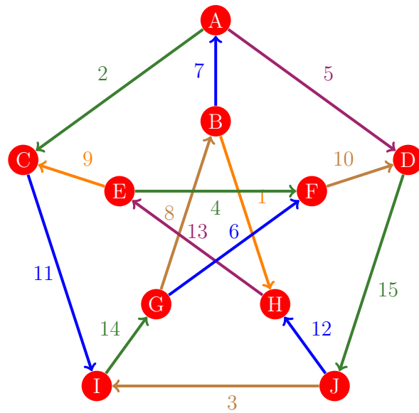
Figura 492: Flujo 484 de la gráfica de Petersen
