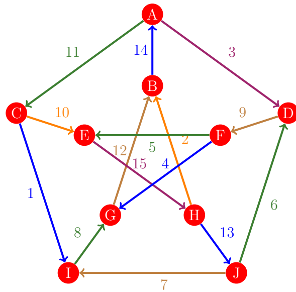
Figura 1074: Flujo 1066 de la gráfica de Petersen
