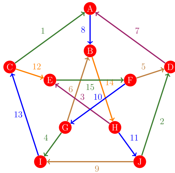
Figura 632: Flujo 624 de la gráfica de Petersen
