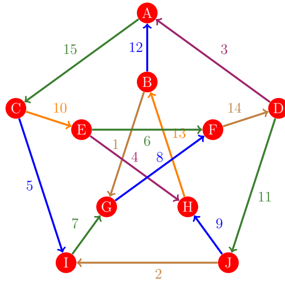
Figura 927: Flujo 919 de la gráfica de Petersen
