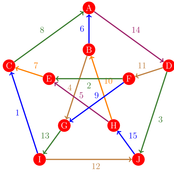
Figura 427: Flujo 419 de la gráfica de Petersen
