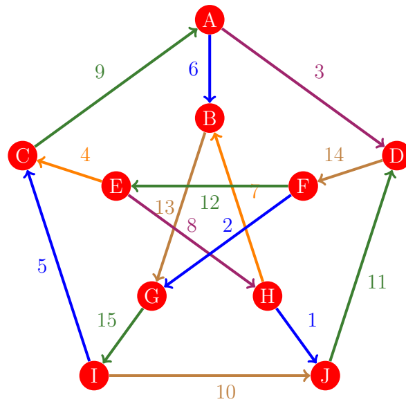
Figura 474: Flujo 466 de la gráfica de Petersen
