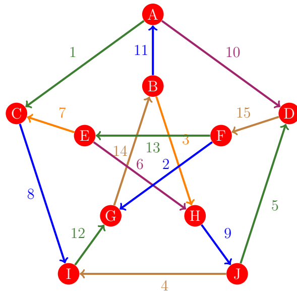
Figura 840: Flujo 832 de la gráfica de Petersen
