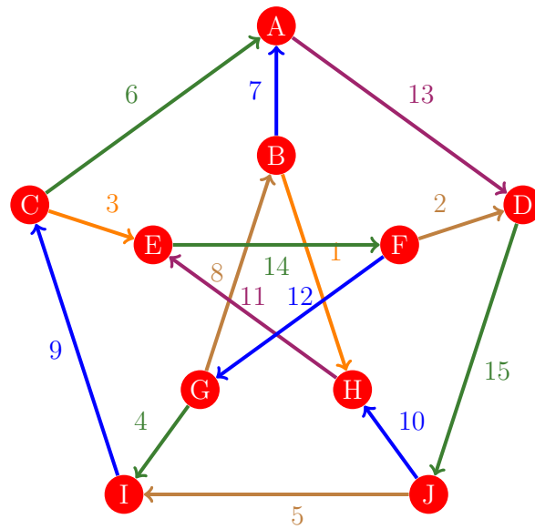
Figura 502: Flujo 494 de la gráfica de Petersen
