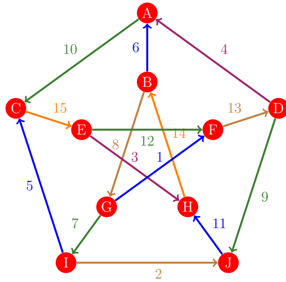
Figura 437: Flujo 429 de la gráfica de Petersen
