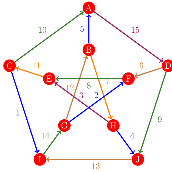
Figura 351: Flujo 343 de la gráfica de Petersen
