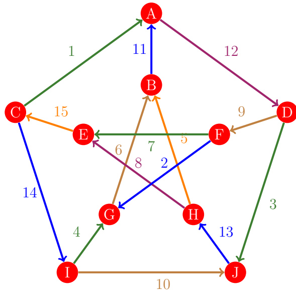
Figura 834: Flujo 826 de la gráfica de Petersen
