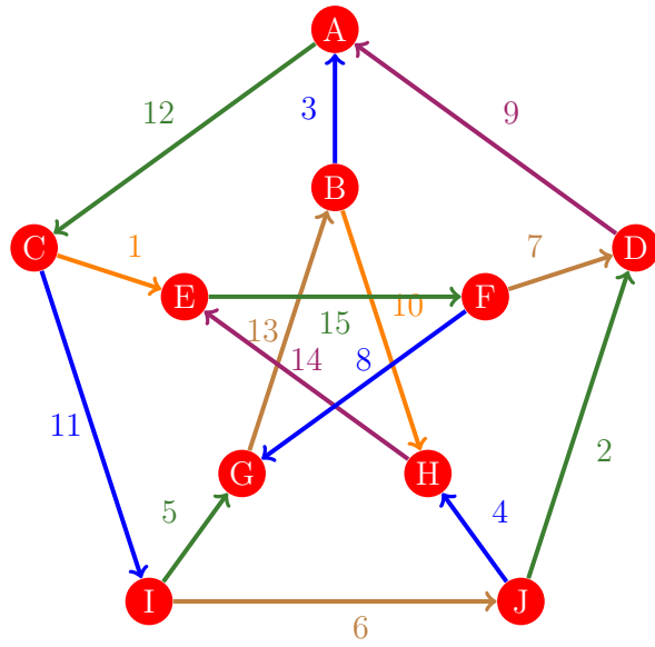
Figura 200: Flujo 192 de la gráfica de Petersen
