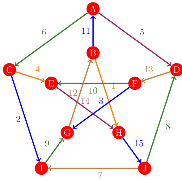
Figura 822: Flujo 814 de la gráfica de Petersen
