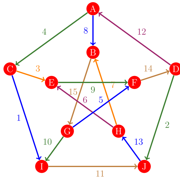
Figura 616: Flujo 608 de la gráfica de Petersen
