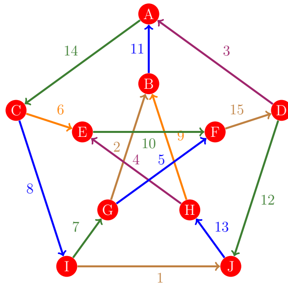
Figura 848: Flujo 840 de la gráfica de Petersen
