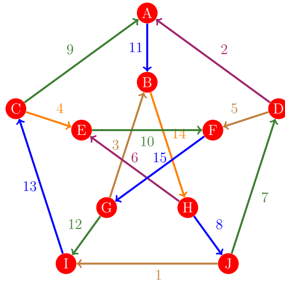
Figura 865: Flujo 857 de la gráfica de Petersen
