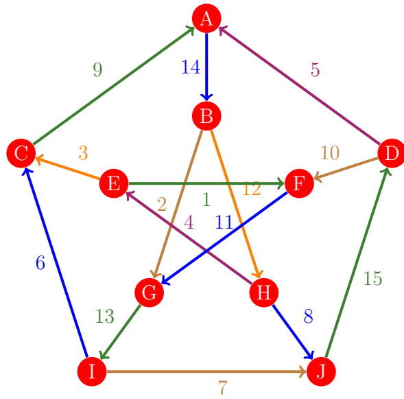
Figura 1107: Flujo 1099 de la gráfica de Petersen
