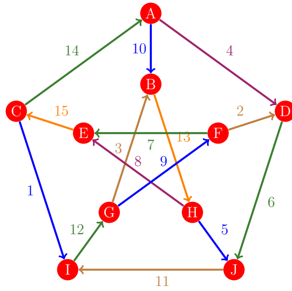
Figura 799: Flujo 791 de la gráfica de Petersen
