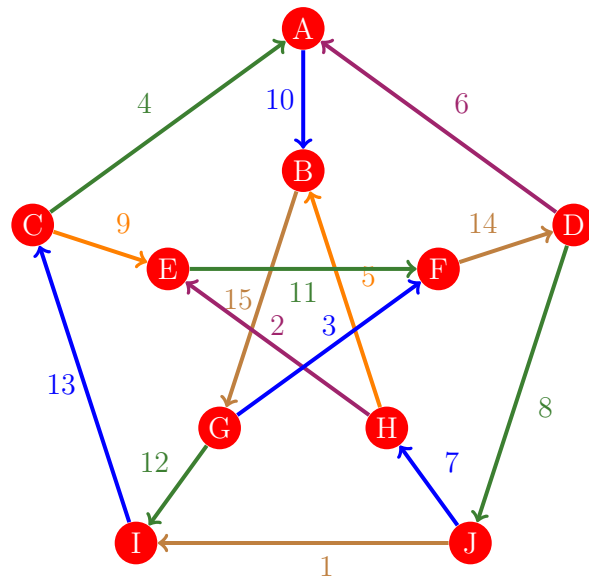
Figura 772: Flujo 764 de la gráfica de Petersen
