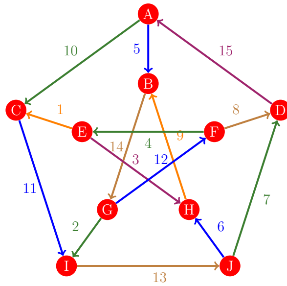
Figura 392: Flujo 384 de la gráfica de Petersen
