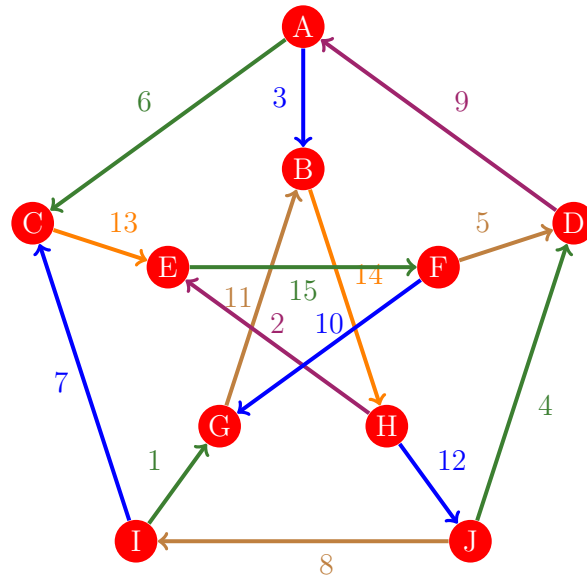
Figura 217: Flujo 209 de la gráfica de Petersen
