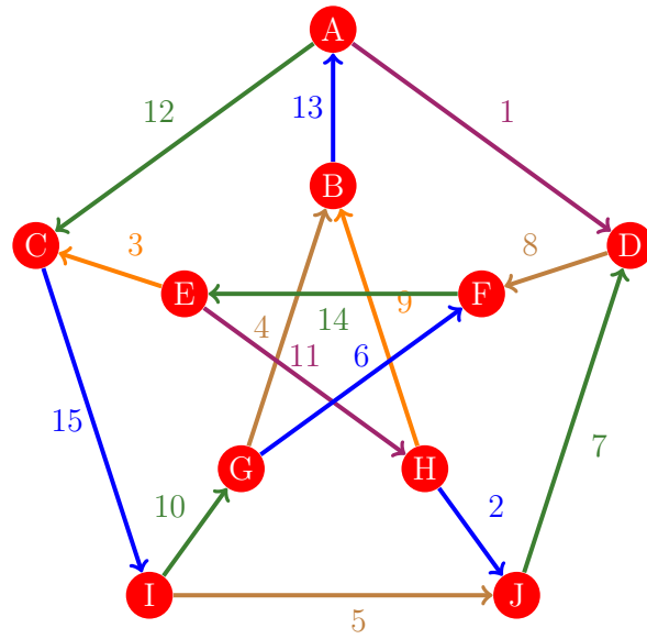
Figura 999: Flujo 991 de la gráfica de Petersen
