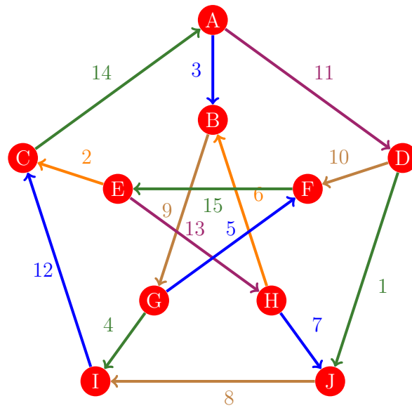
Figura 244: Flujo 236 de la gráfica de Petersen
