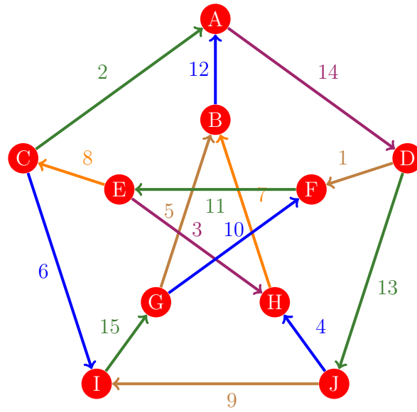
Figura 891: Flujo 883 de la gráfica de Petersen
