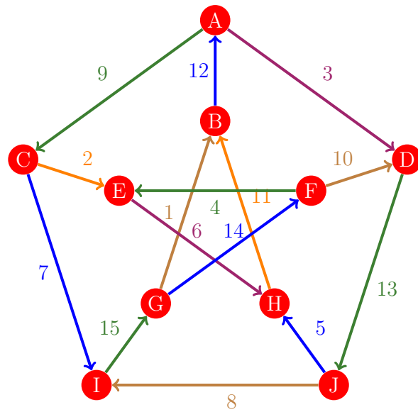
Figura 912: Flujo 904 de la gráfica de Petersen
