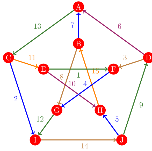
Figura 523: Flujo 515 de la gráfica de Petersen
