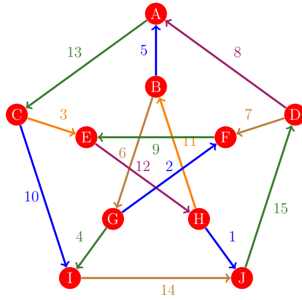
Figura 357: Flujo 349 de la gráfica de Petersen
