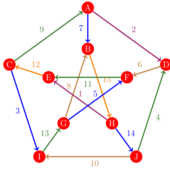
Figura 557: Flujo 549 de la gráfica de Petersen
