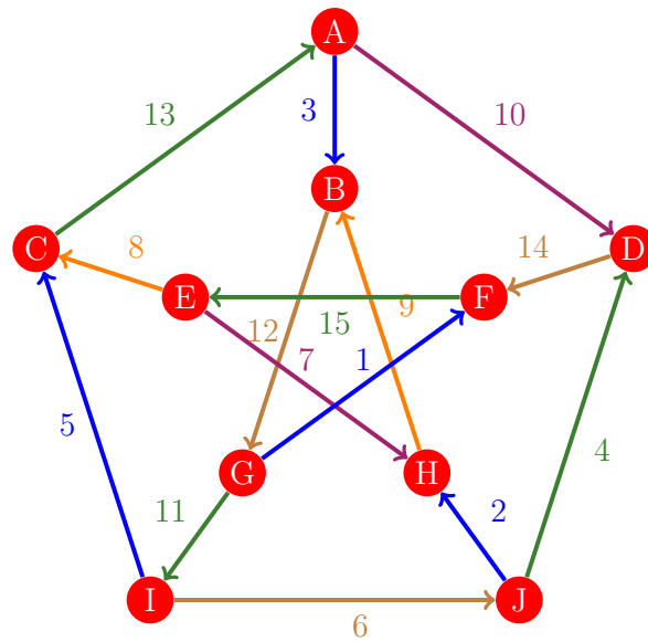
Figura 242: Flujo 234 de la gráfica de Petersen
