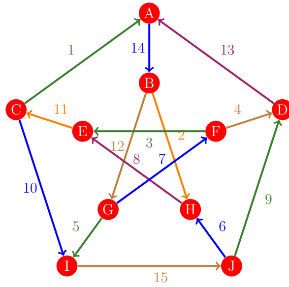
Figura 1123: Flujo 1115 de la gráfica de Petersen
