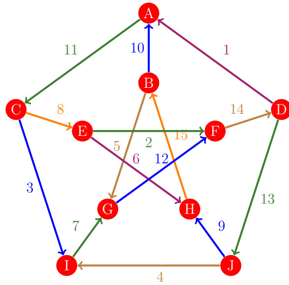
Figura 751: Flujo 743 de la gráfica de Petersen
