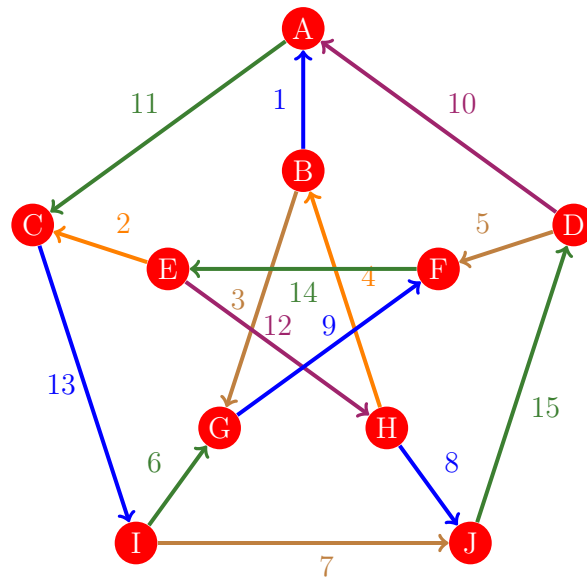
Figura 32: Flujo 24 de la gráfica de Petersen
