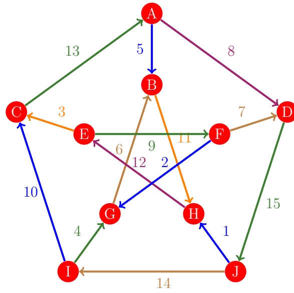
Figura 397: Flujo 389 de la gráfica de Petersen
