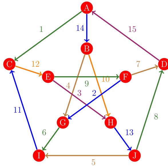
Figura 1125: Flujo 1117 de la gráfica de Petersen
