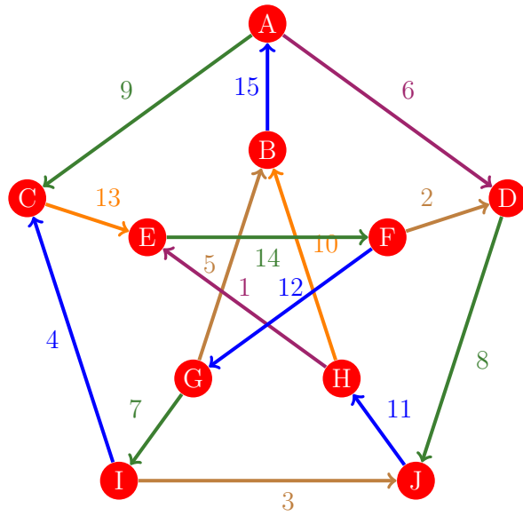
Figura 1151: Flujo 1143 de la gráfica de Petersen
