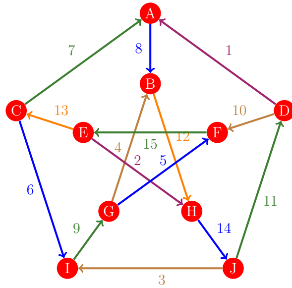
Figura 623: Flujo 615 de la gráfica de Petersen
