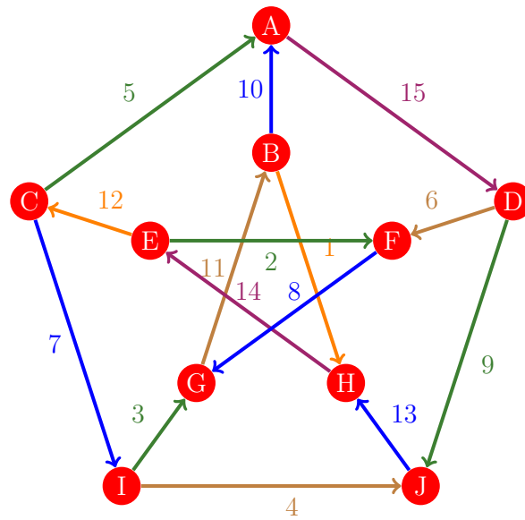
Figura 742: Flujo 734 de la gráfica de Petersen
