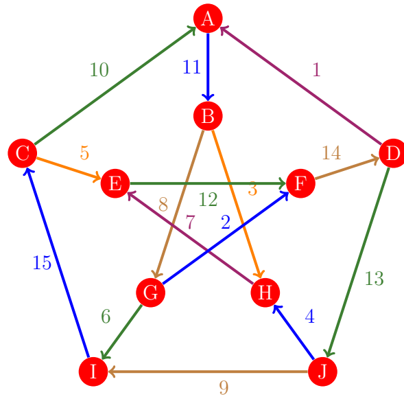
Figura 867: Flujo 859 de la gráfica de Petersen
