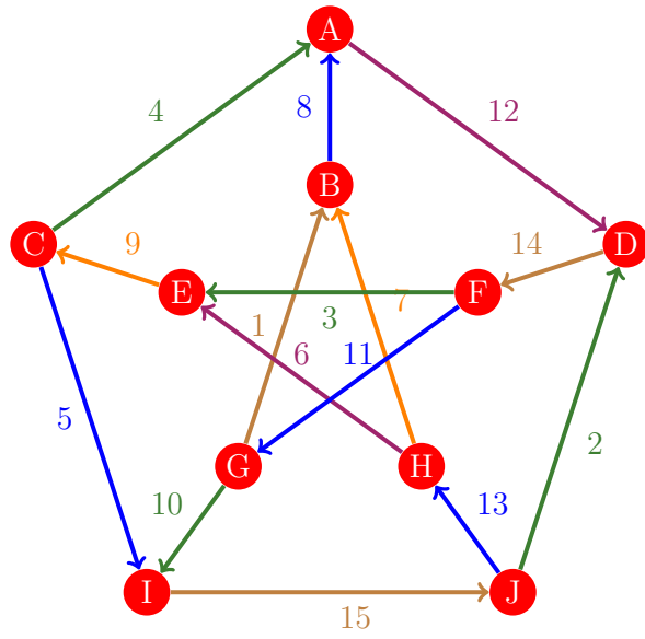
Figura 575: Flujo 567 de la gráfica de Petersen
