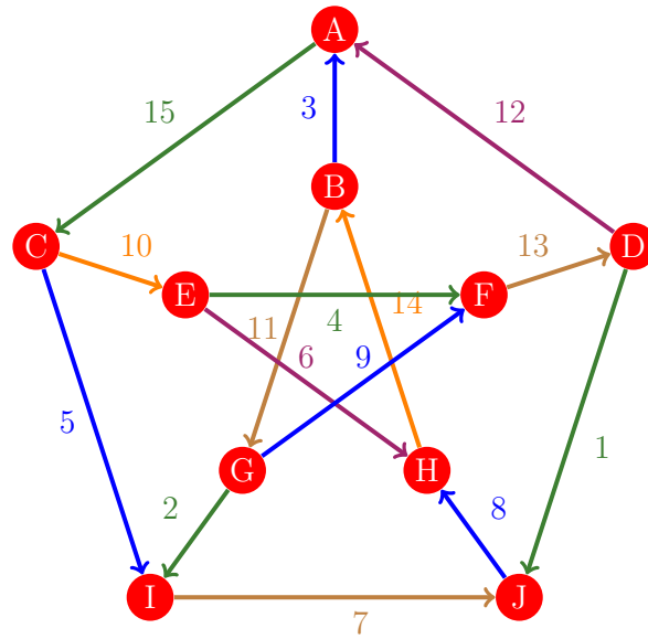
Figura 207: Flujo 199 de la gráfica de Petersen
