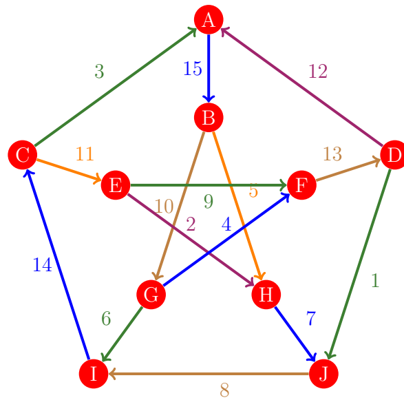
Figura 1172: Flujo 1164 de la gráfica de Petersen
