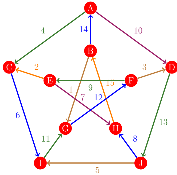
Figura 1059: Flujo 1051 de la gráfica de Petersen
