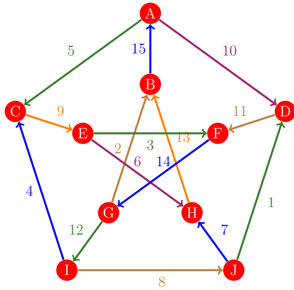
Figura 1133: Flujo 1125 de la gráfica de Petersen
