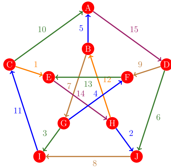
Figura 347: Flujo 339 de la gráfica de Petersen
