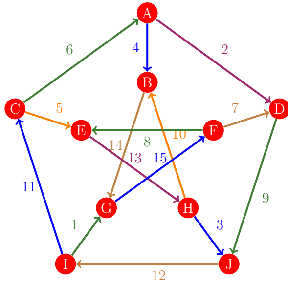
Figura 300: Flujo 292 de la gráfica de Petersen
