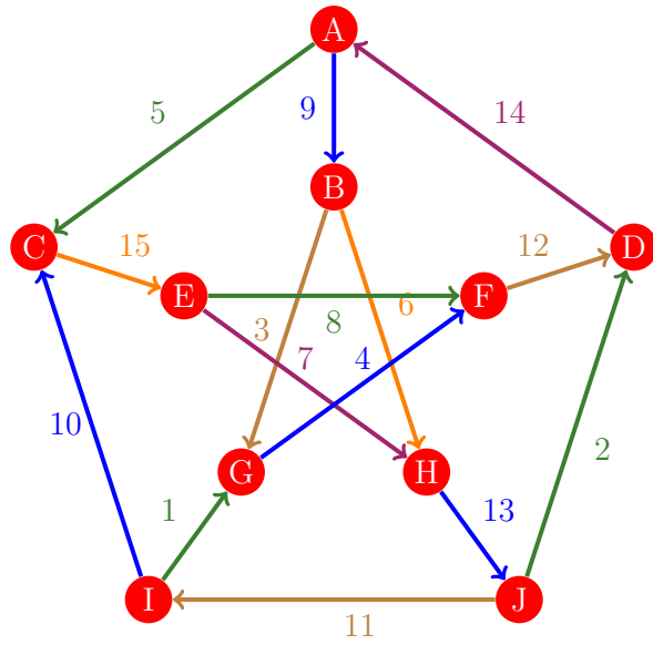
Figura 708: Flujo 700 de la gráfica de Petersen
