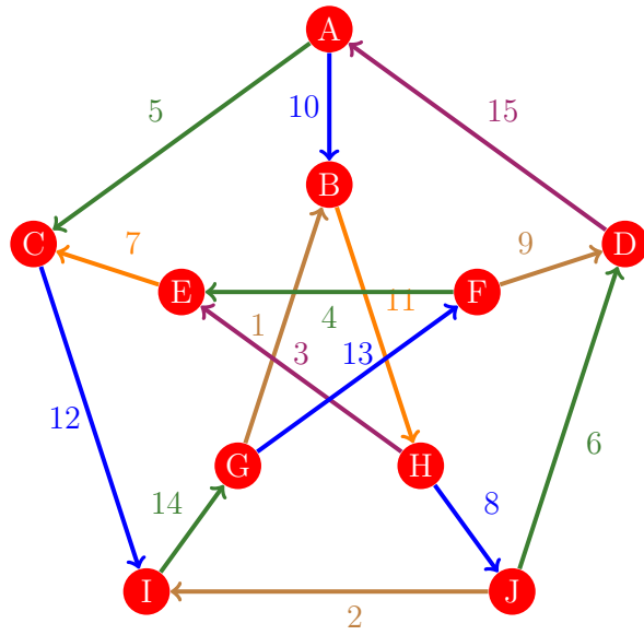
Figura 777: Flujo 769 de la gráfica de Petersen
