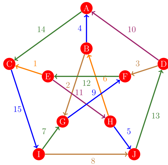
Figura 288: Flujo 280 de la gráfica de Petersen
