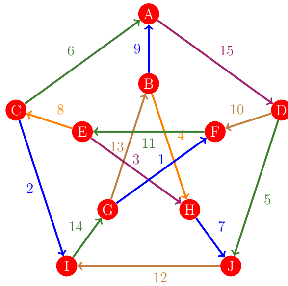
Figura 670: Flujo 662 de la gráfica de Petersen
