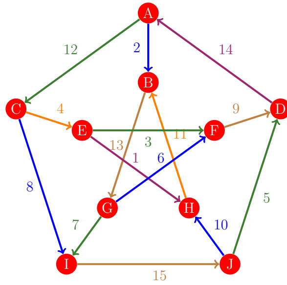
Figura 155: Flujo 147 de la gráfica de Petersen
