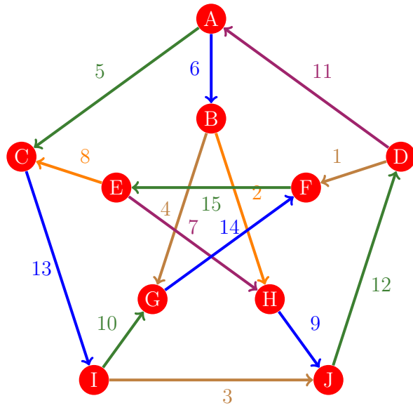
Figura 461: Flujo 453 de la gráfica de Petersen
