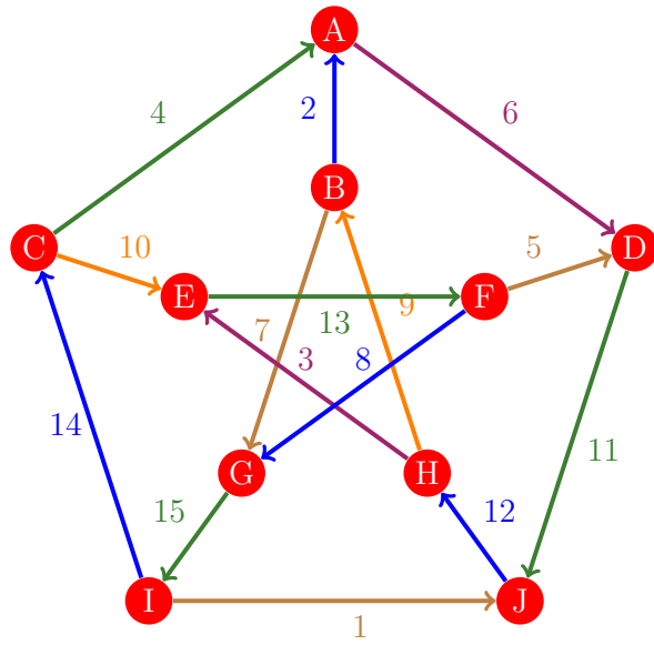
Figura 89: Flujo 81 de la gráfica de Petersen
