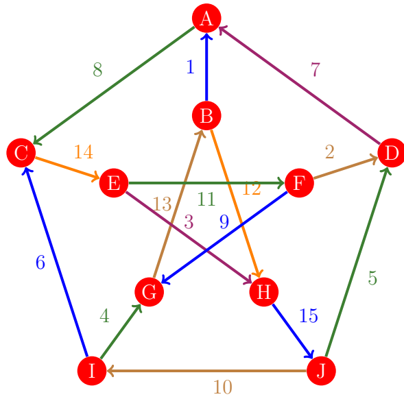
Figura 20: Flujo 12 de la gráfica de Petersen
