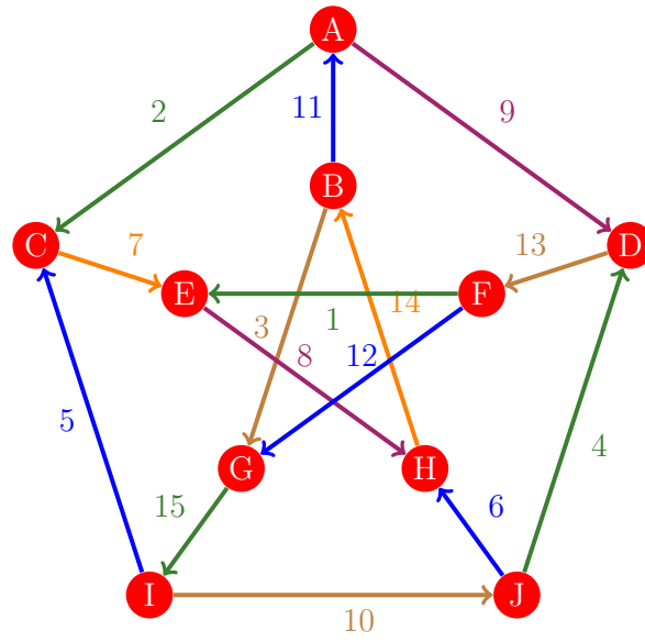
Figura 811: Flujo 803 de la gráfica de Petersen
