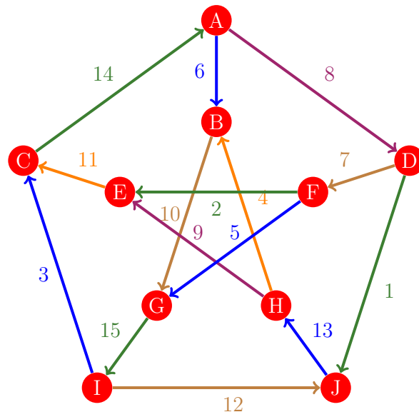
Figura 486: Flujo 478 de la gráfica de Petersen
