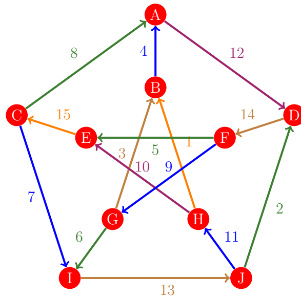
Figura 268: Flujo 260 de la gráfica de Petersen
