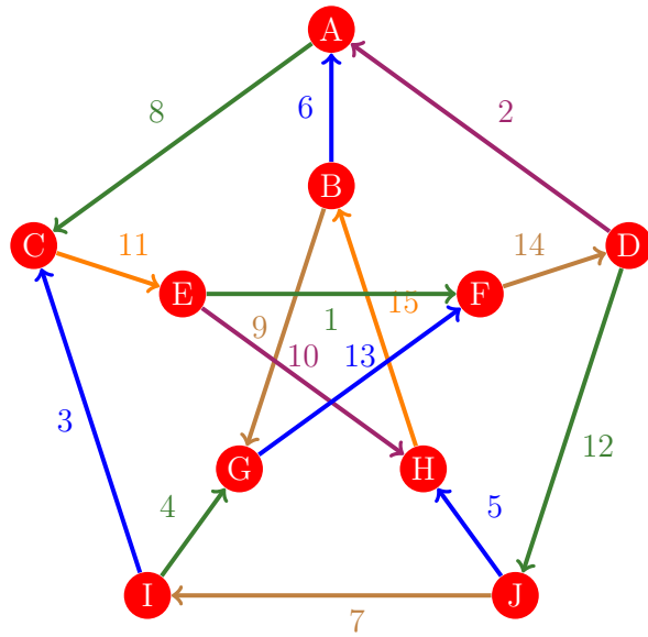
Figura 429: Flujo 421 de la gráfica de Petersen
