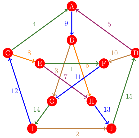
Figura 699: Flujo 691 de la gráfica de Petersen
