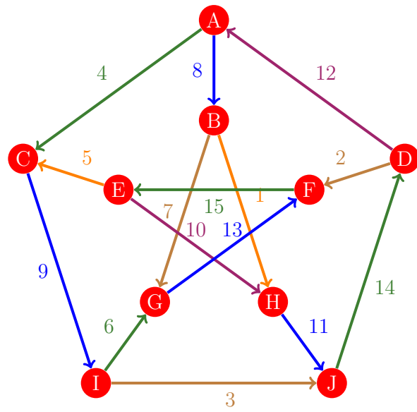
Figura 614: Flujo 606 de la gráfica de Petersen
