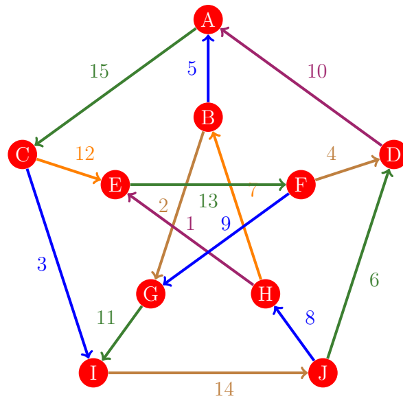
Figura 368: Flujo 360 de la gráfica de Petersen
