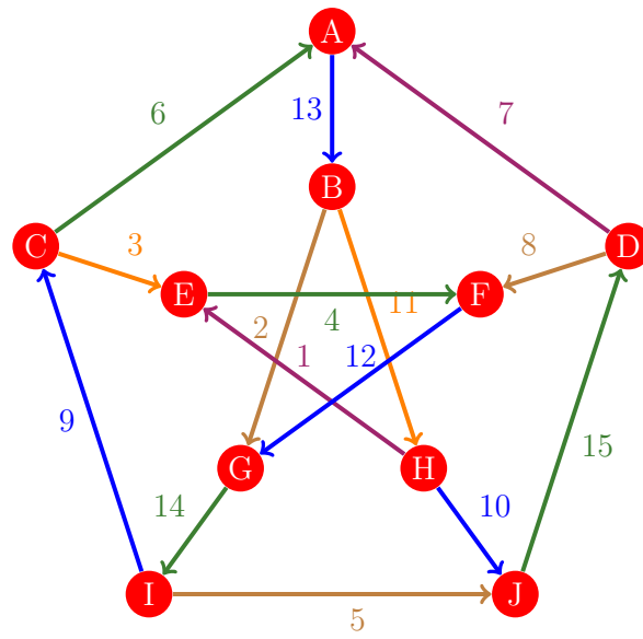
Figura 1022: Flujo 1014 de la gráfica de Petersen
