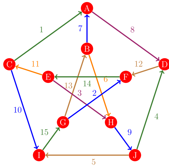
Figura 508: Flujo 500 de la gráfica de Petersen
