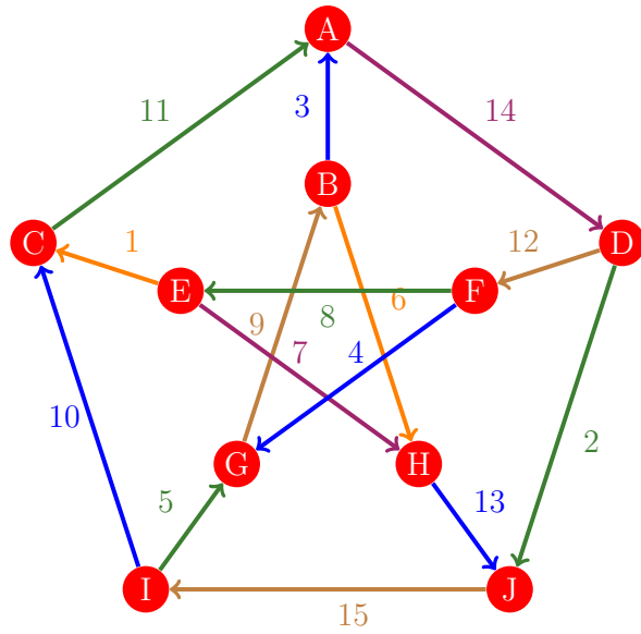
Figura 192: Flujo 184 de la gráfica de Petersen
