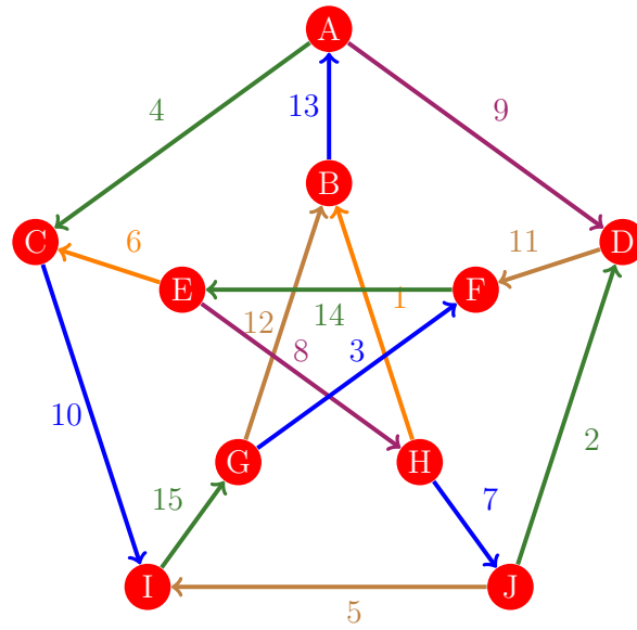
Figura 975: Flujo 967 de la gráfica de Petersen
