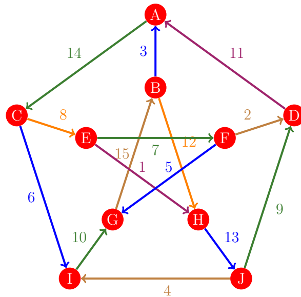
Figura 206: Flujo 198 de la gráfica de Petersen
