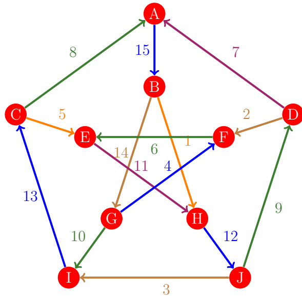
Figura 1189: Flujo 1181 de la gráfica de Petersen
