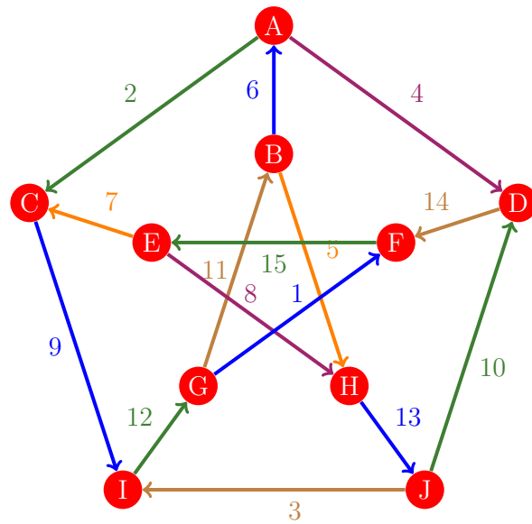
Figura 412: Flujo 404 de la gráfica de Petersen
