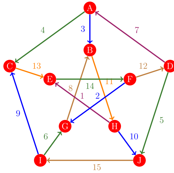
Figura 213: Flujo 205 de la gráfica de Petersen
