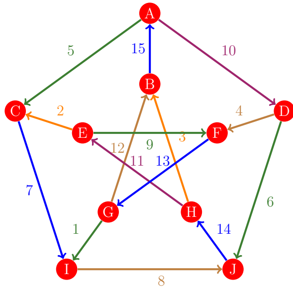
Figura 1139: Flujo 1131 de la gráfica de Petersen
