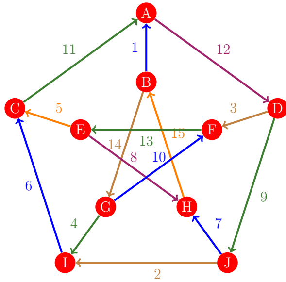
Figura 27: Flujo 19 de la gráfica de Petersen
