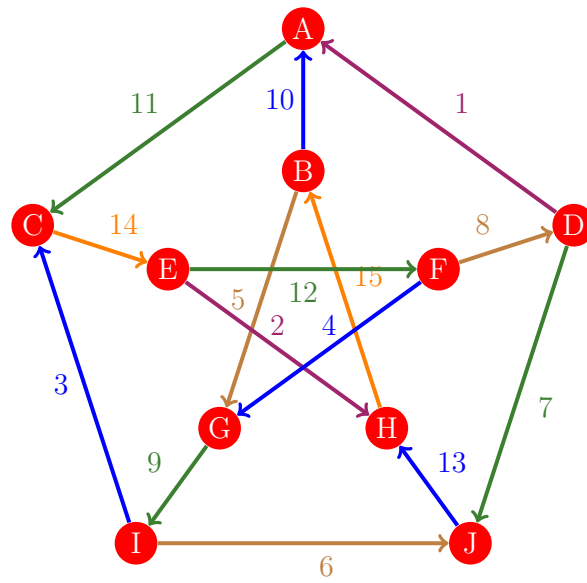
Figura 753: Flujo 745 de la gráfica de Petersen
