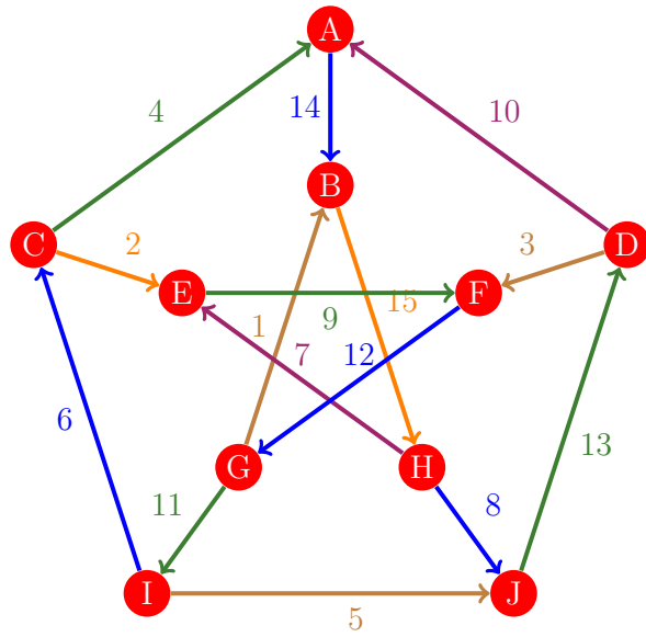
Figura 1099: Flujo 1091 de la gráfica de Petersen
