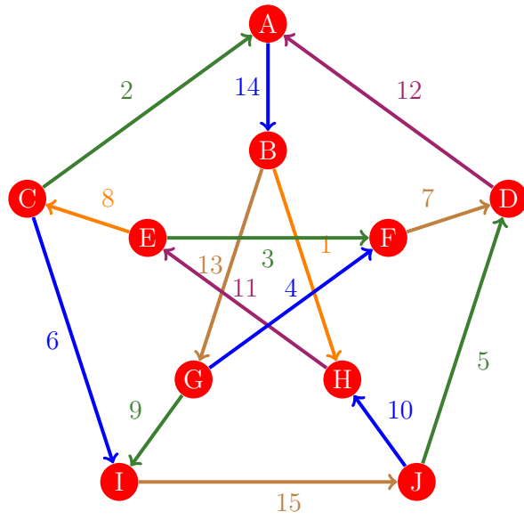
Figura 1093: Flujo 1085 de la gráfica de Petersen
