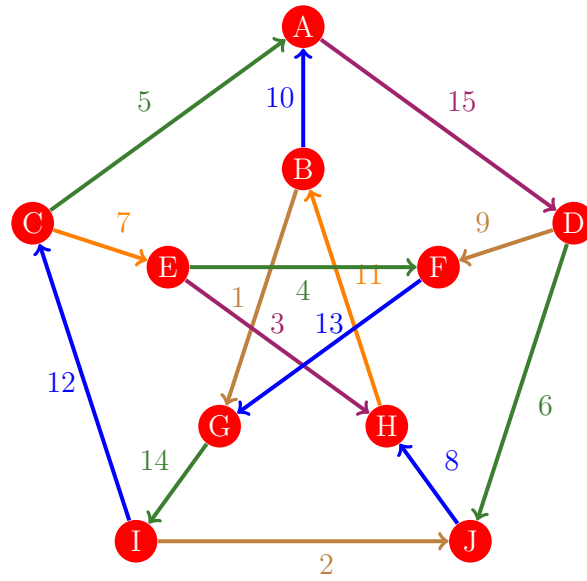
Figura 737: Flujo 729 de la gráfica de Petersen
