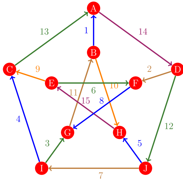
Figura 40: Flujo 32 de la gráfica de Petersen
