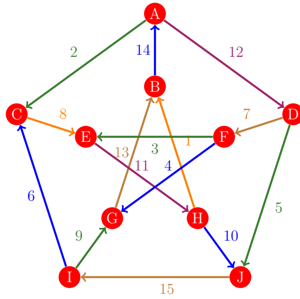
Figura 1053: Flujo 1045 de la gráfica de Petersen
