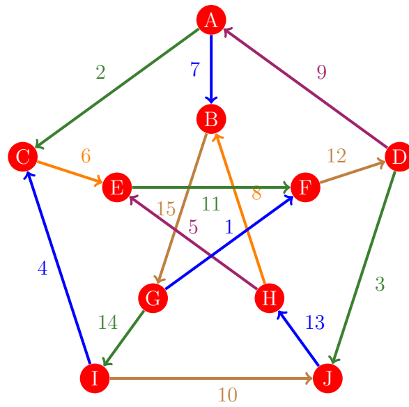
Figura 532: Flujo 524 de la gráfica de Petersen
