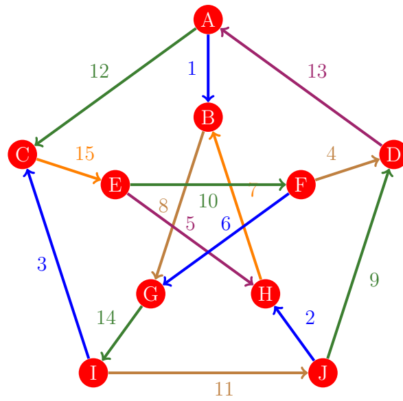
Figura 78: Flujo 70 de la gráfica de Petersen
