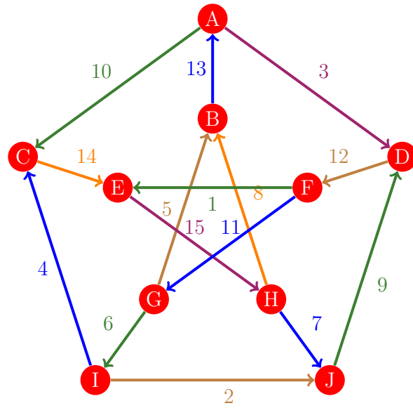
Figura 995: Flujo 987 de la gráfica de Petersen
