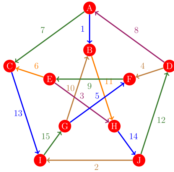
Figura 53: Flujo 45 de la gráfica de Petersen
