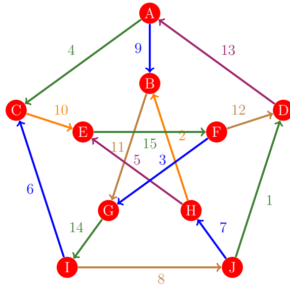
Figura 703: Flujo 695 de la gráfica de Petersen
