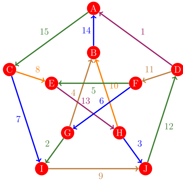
Figura 1087: Flujo 1079 de la gráfica de Petersen
