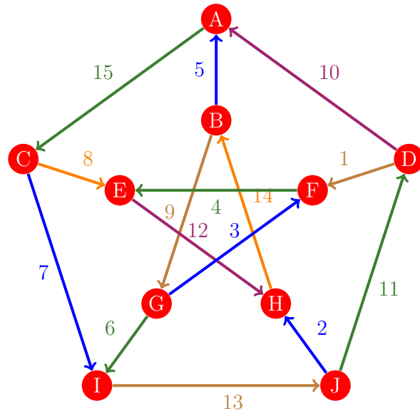
Figura 365: Flujo 357 de la gráfica de Petersen
