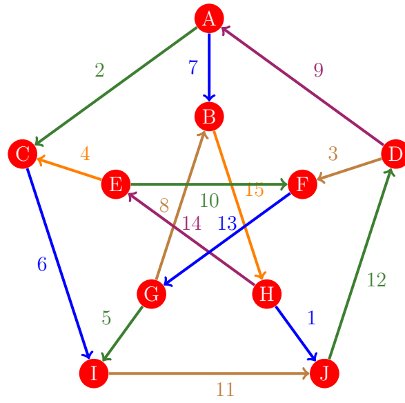
Figura 531: Flujo 523 de la gráfica de Petersen
