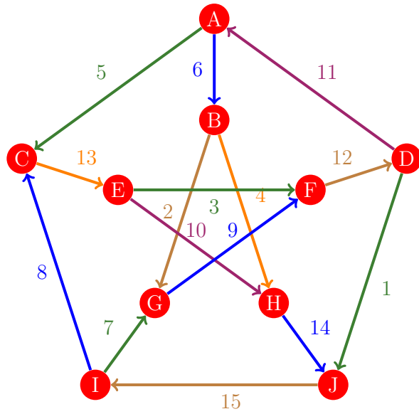
Figura 462: Flujo 454 de la gráfica de Petersen
