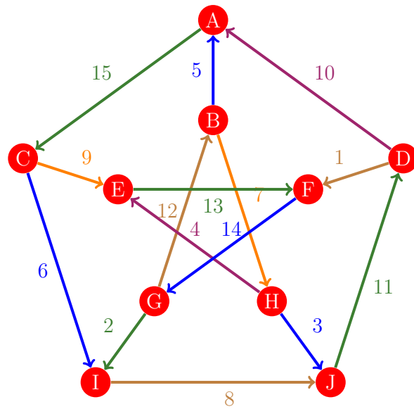
Figura 366: Flujo 358 de la gráfica de Petersen
