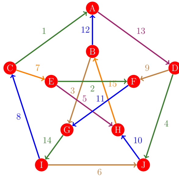
Figura 915: Flujo 907 de la gráfica de Petersen
