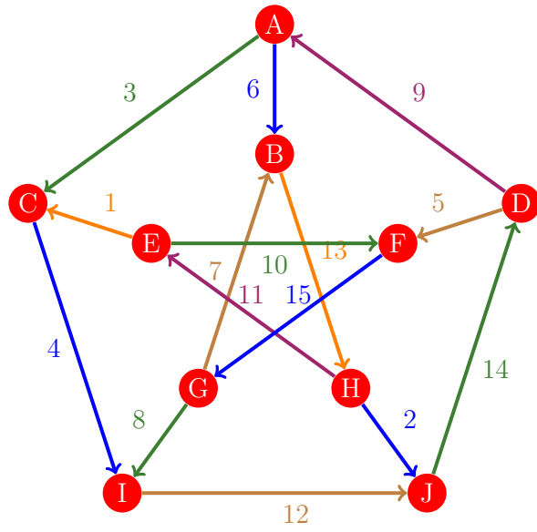
Figura 453: Flujo 445 de la gráfica de Petersen
