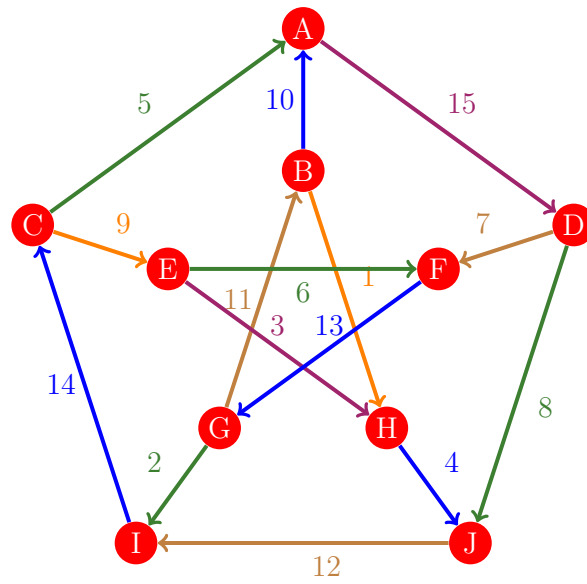
Figura 740: Flujo 732 de la gráfica de Petersen
