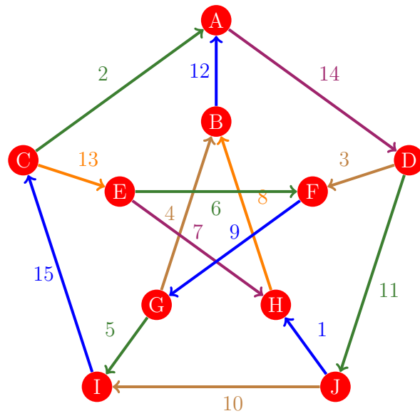
Figura 890: Flujo 882 de la gráfica de Petersen
