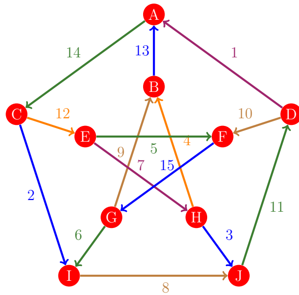
Figura 1006: Flujo 998 de la gráfica de Petersen
