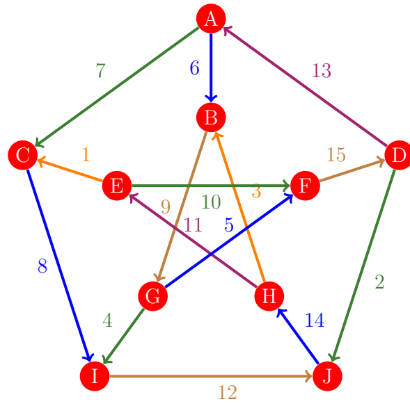
Figura 463: Flujo 455 de la gráfica de Petersen
