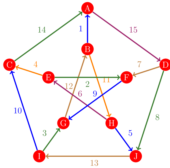
Figura 44: Flujo 36 de la gráfica de Petersen
