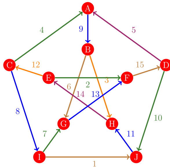
Figura 700: Flujo 692 de la gráfica de Petersen
