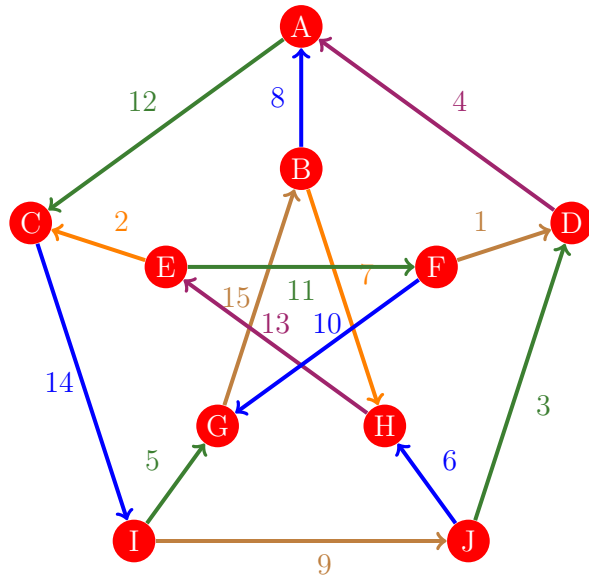
Figura 600: Flujo 592 de la gráfica de Petersen
