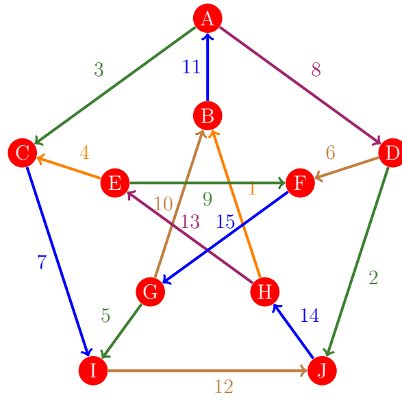
Figura 817: Flujo 809 de la gráfica de Petersen
