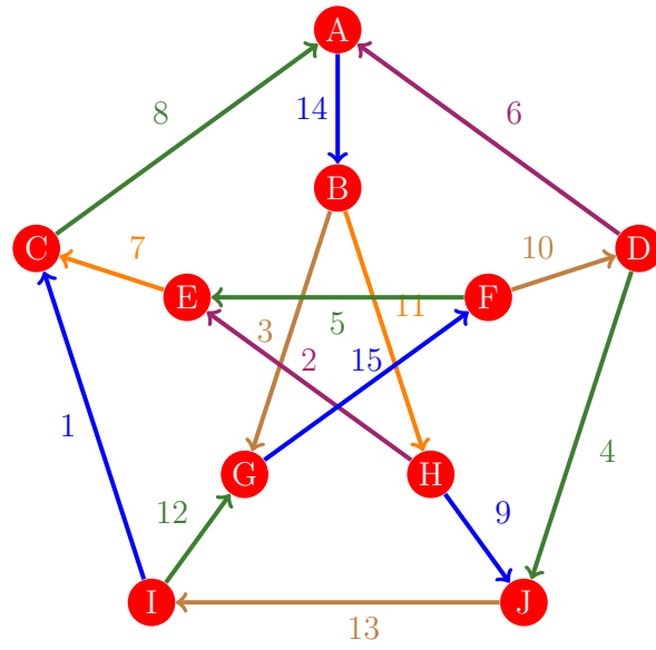
Figura 1105: Flujo 1097 de la gráfica de Petersen
