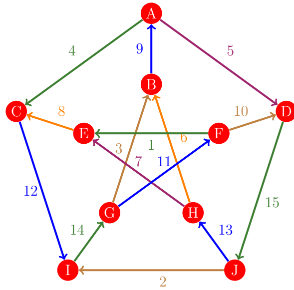
Figura 663: Flujo 655 de la gráfica de Petersen
