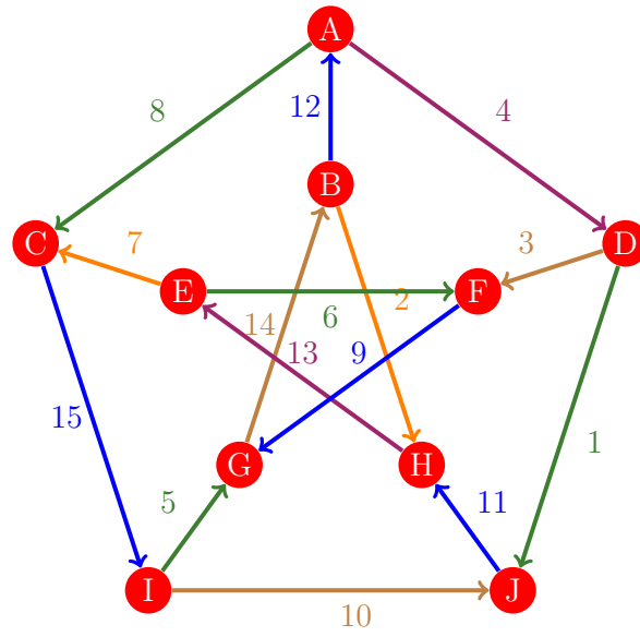
Figura 909: Flujo 901 de la gráfica de Petersen
