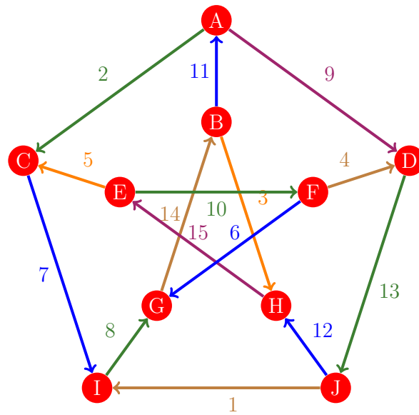
Figura 812: Flujo 804 de la gráfica de Petersen
