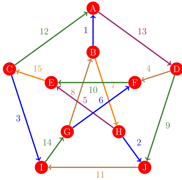
Figura 36: Flujo 28 de la gráfica de Petersen
