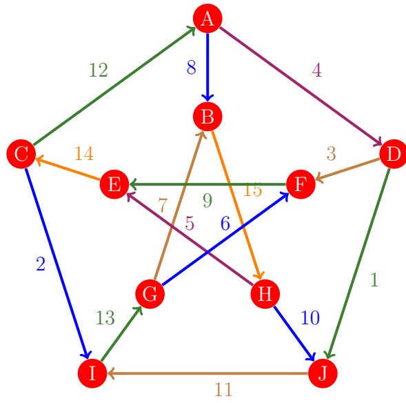
Figura 637: Flujo 629 de la gráfica de Petersen
