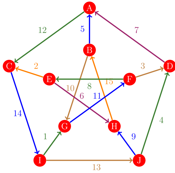
Figura 355: Flujo 347 de la gráfica de Petersen
