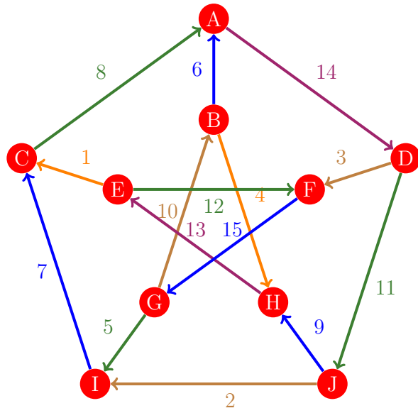
Figura 428: Flujo 420 de la gráfica de Petersen
