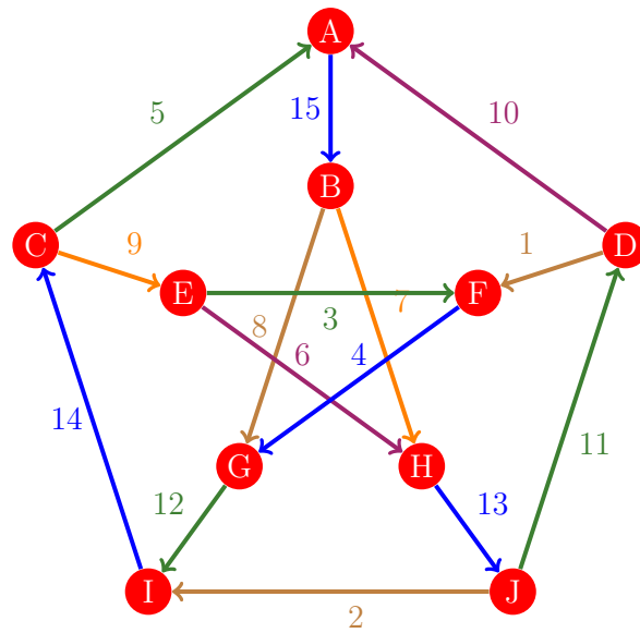
Figura 1176: Flujo 1168 de la gráfica de Petersen
