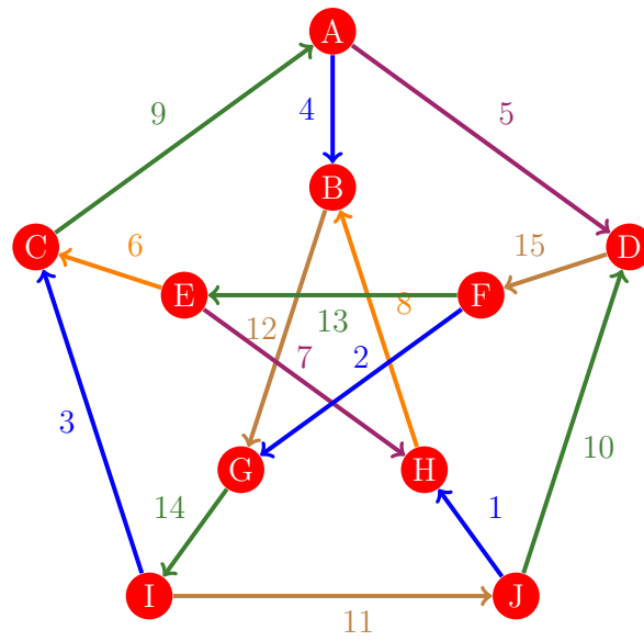
Figura 310: Flujo 302 de la gráfica de Petersen
