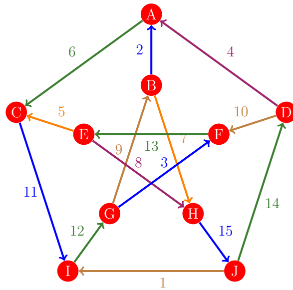
Figura 96: Flujo 88 de la gráfica de Petersen
