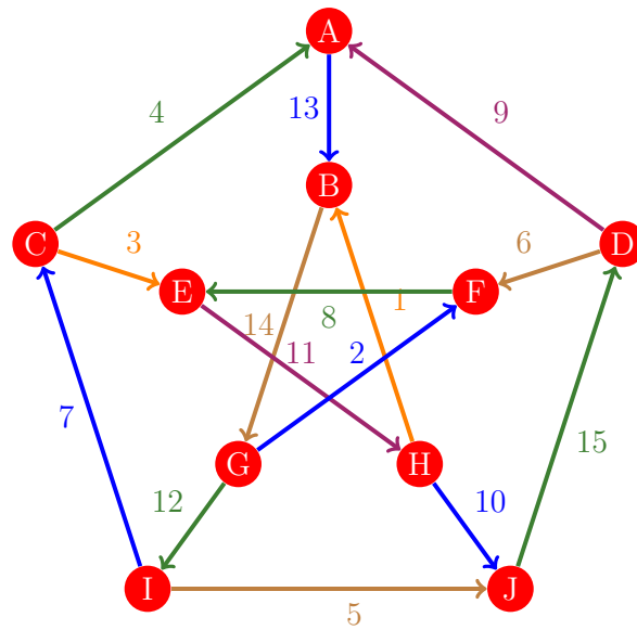
Figura 1018: Flujo 1010 de la gráfica de Petersen
