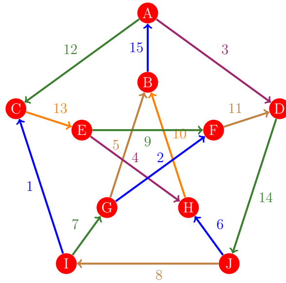
Figura 1161: Flujo 1153 de la gráfica de Petersen
