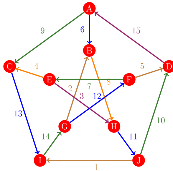
Figura 476: Flujo 468 de la gráfica de Petersen
