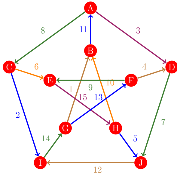
Figura 824: Flujo 816 de la gráfica de Petersen
