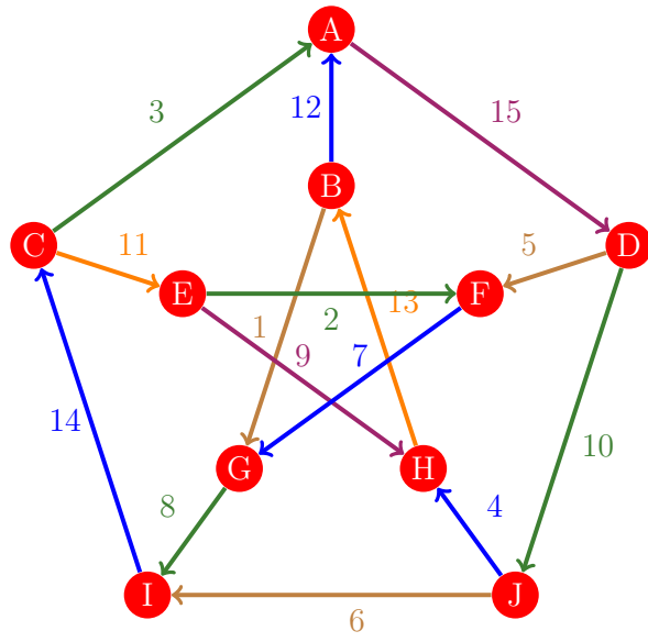
Figura 895: Flujo 887 de la gráfica de Petersen
