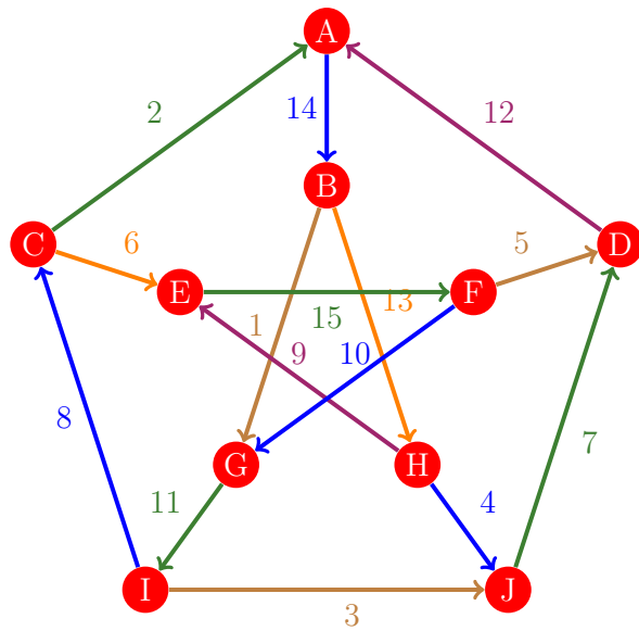
Figura 1094: Flujo 1086 de la gráfica de Petersen
