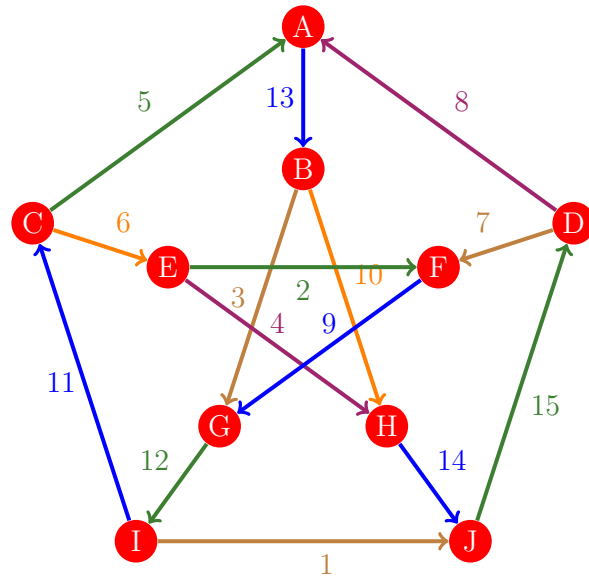
Figura 1019: Flujo 1011 de la gráfica de Petersen
