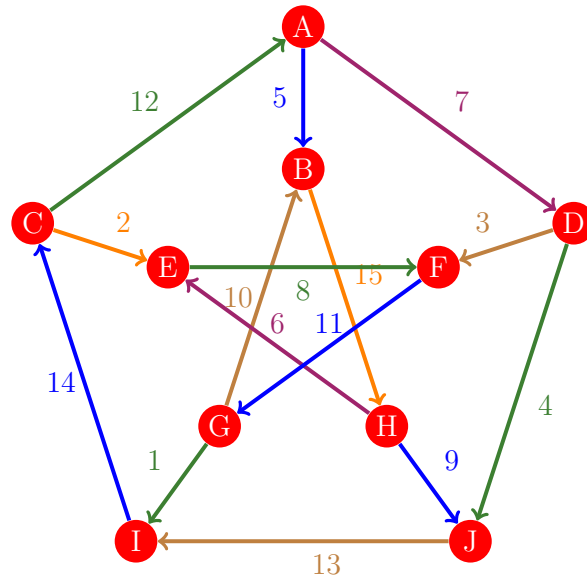
Figura 395: Flujo 387 de la gráfica de Petersen
