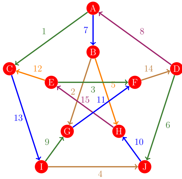
Figura 547: Flujo 539 de la gráfica de Petersen
