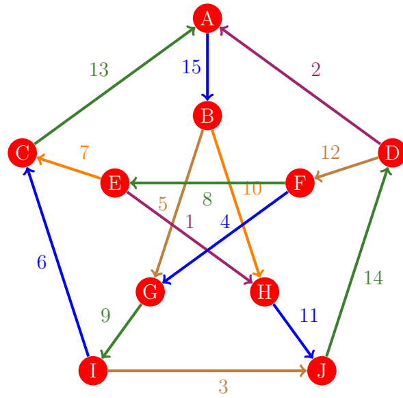
Figura 1203: Flujo 1195 de la gráfica de Petersen
