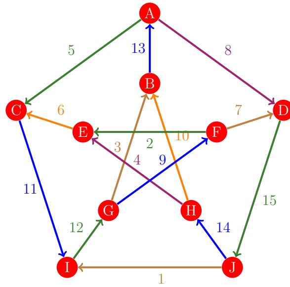
Figura 979: Flujo 971 de la gráfica de Petersen
