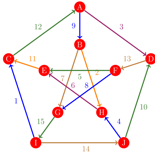
Figura 719: Flujo 711 de la gráfica de Petersen
