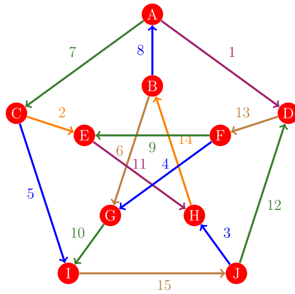
Figura 588: Flujo 580 de la gráfica de Petersen
