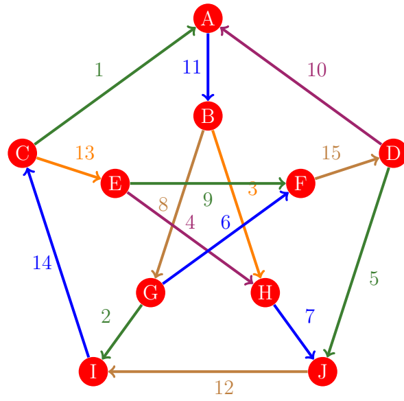
Figura 873: Flujo 865 de la gráfica de Petersen
