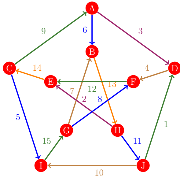
Figura 472: Flujo 464 de la gráfica de Petersen
