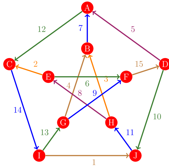
Figura 519: Flujo 511 de la gráfica de Petersen
