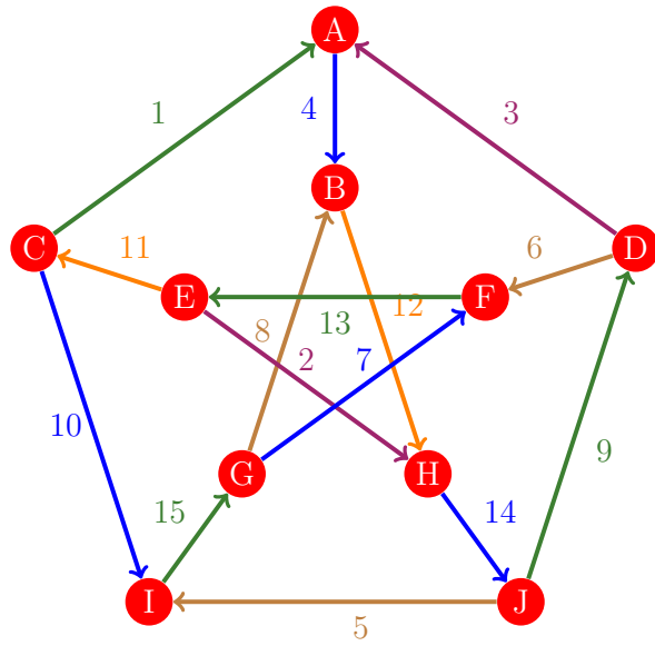
Figura 295: Flujo 287 de la gráfica de Petersen
