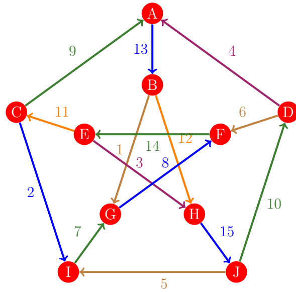
Figura 1033: Flujo 1025 de la gráfica de Petersen
