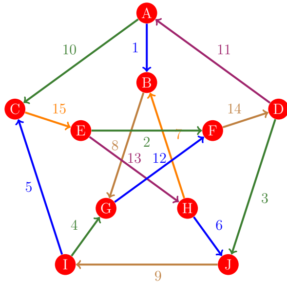
Figura 63: Flujo 55 de la gráfica de Petersen
