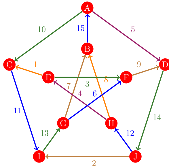
Figura 1155: Flujo 1147 de la gráfica de Petersen
