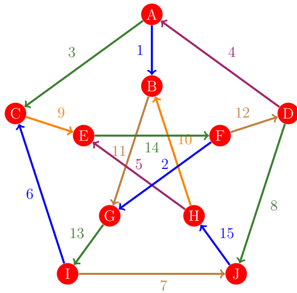
Figura 50: Flujo 42 de la gráfica de Petersen
