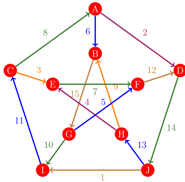
Figura 468: Flujo 460 de la gráfica de Petersen
