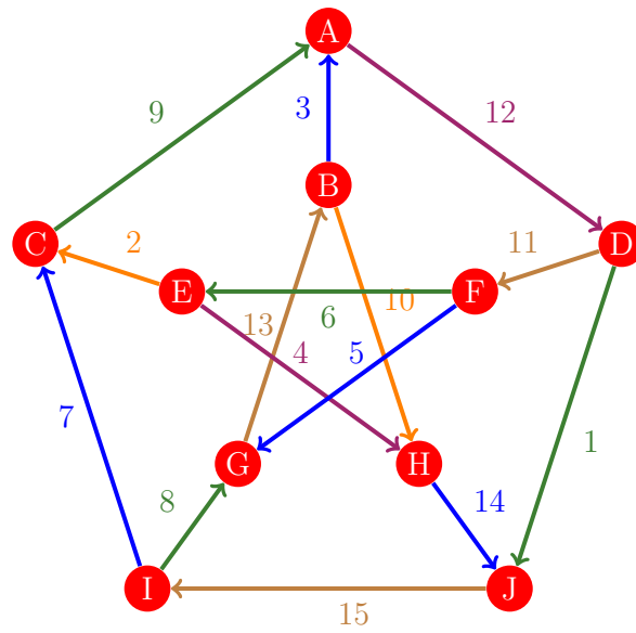
Figura 184: Flujo 176 de la gráfica de Petersen
