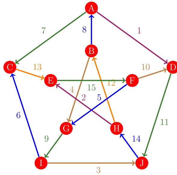
Figura 587: Flujo 579 de la gráfica de Petersen
