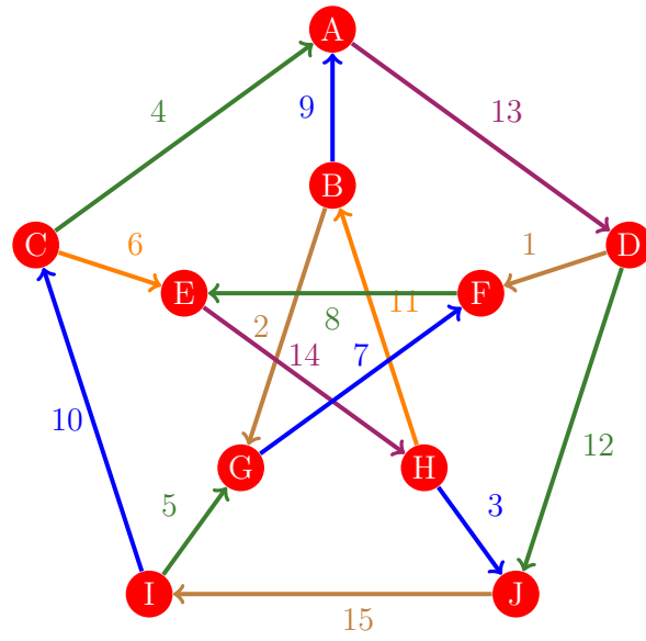
Figura 659: Flujo 651 de la gráfica de Petersen
