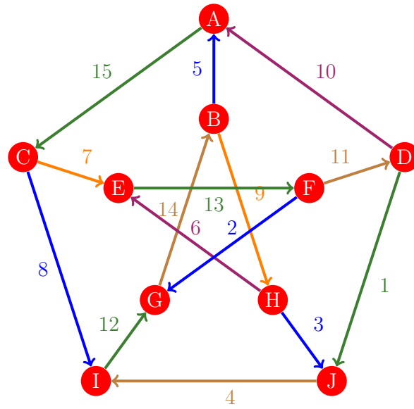
Figura 367: Flujo 359 de la gráfica de Petersen
