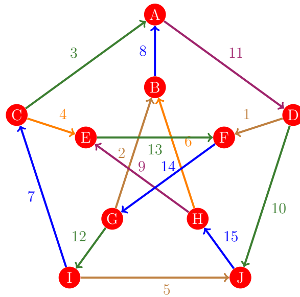
Figura 572: Flujo 564 de la gráfica de Petersen
