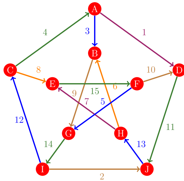
Figura 212: Flujo 204 de la gráfica de Petersen
