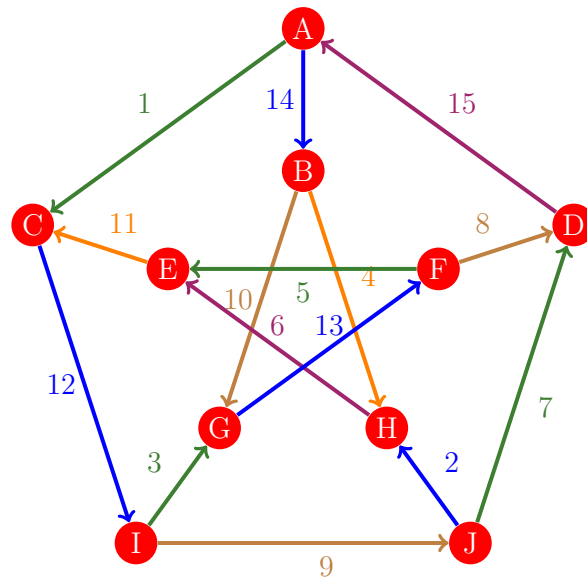
Figura 1126: Flujo 1118 de la gráfica de Petersen
