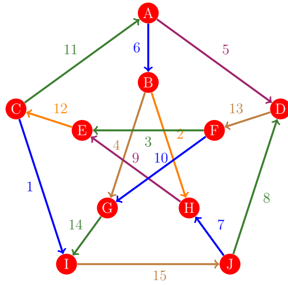
Figura 479: Flujo 471 de la gráfica de Petersen
