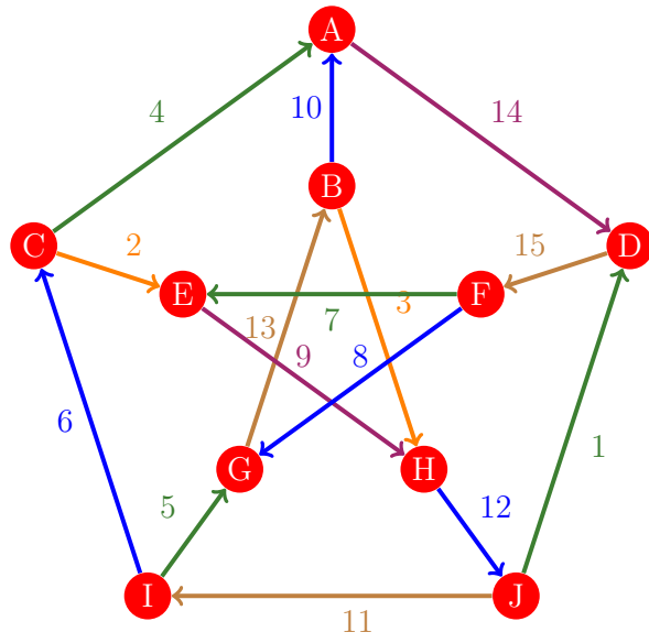
Figura 731: Flujo 723 de la gráfica de Petersen
