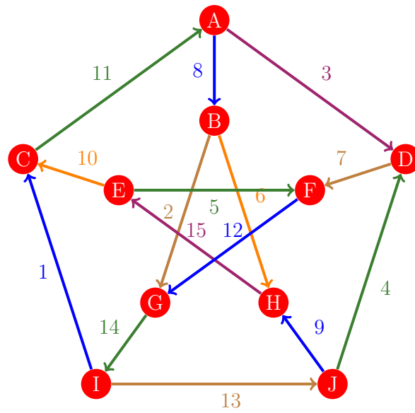
Figura 636: Flujo 628 de la gráfica de Petersen
