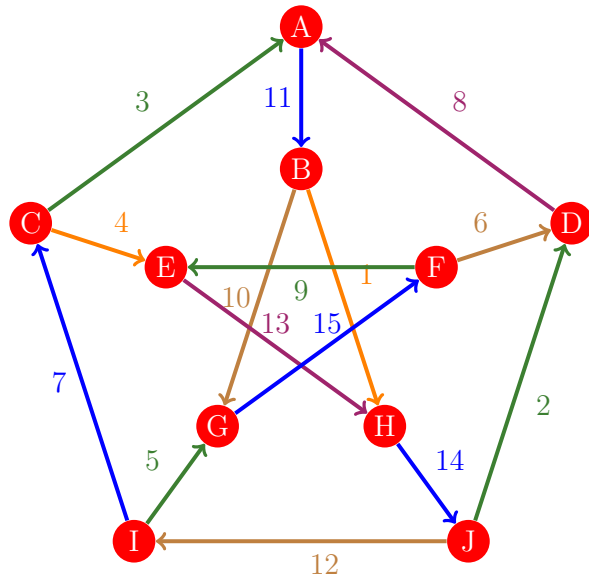
Figura 853: Flujo 845 de la gráfica de Petersen
