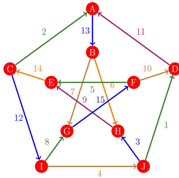
Figura 1010: Flujo 1002 de la gráfica de Petersen
