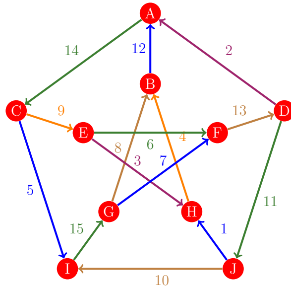
Figura 925: Flujo 917 de la gráfica de Petersen
