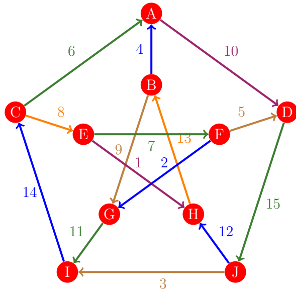
Figura 259: Flujo 251 de la gráfica de Petersen
