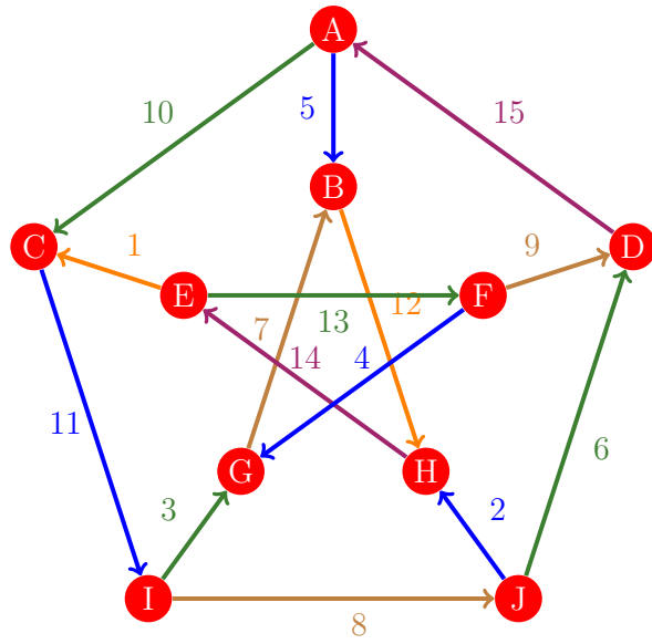
Figura 386: Flujo 378 de la gráfica de Petersen
