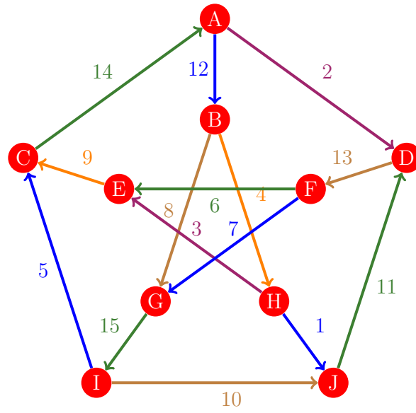
Figura 965: Flujo 957 de la gráfica de Petersen
