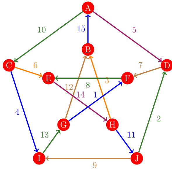
Figura 1159: Flujo 1151 de la gráfica de Petersen
