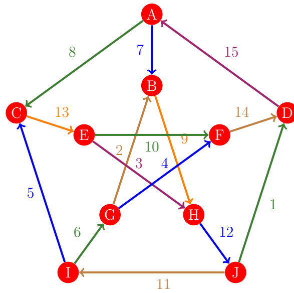
Figura 554: Flujo 546 de la gráfica de Petersen
