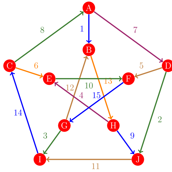
Figura 59: Flujo 51 de la gráfica de Petersen
