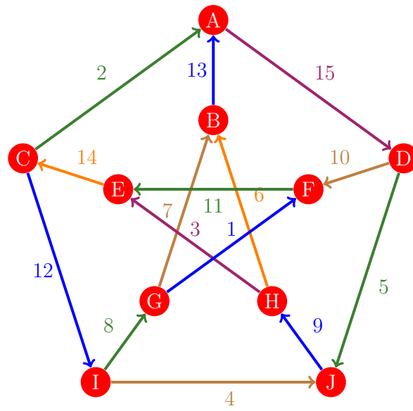
Figura 970: Flujo 962 de la gráfica de Petersen
