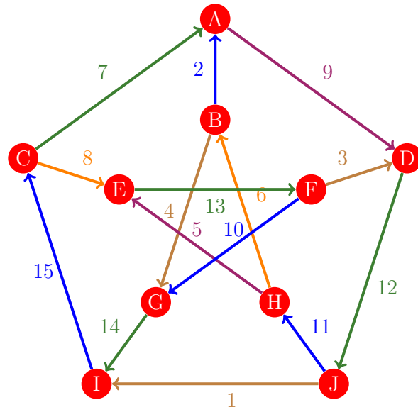
Figura 97: Flujo 89 de la gráfica de Petersen
