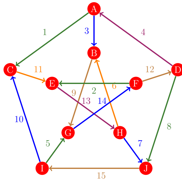
Figura 210: Flujo 202 de la gráfica de Petersen
