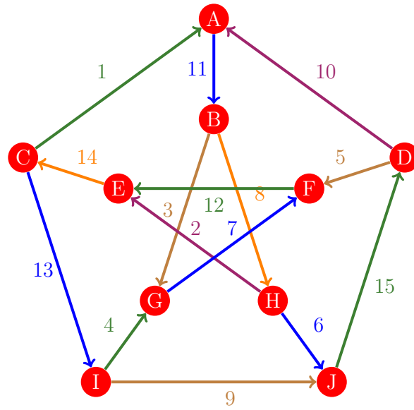
Figura 875: Flujo 867 de la gráfica de Petersen
