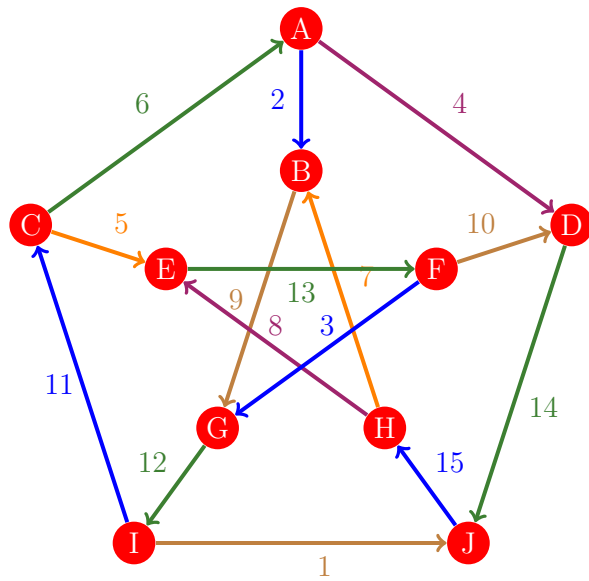
Figura 134: Flujo 126 de la gráfica de Petersen
