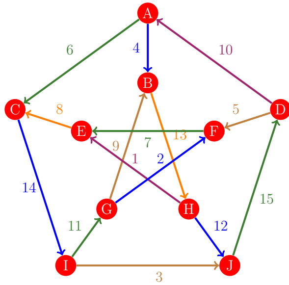
Figura 301: Flujo 293 de la gráfica de Petersen
