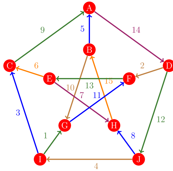
Figura 341: Flujo 333 de la gráfica de Petersen
