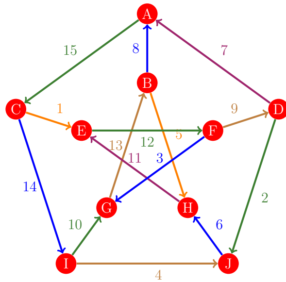
Figura 608: Flujo 600 de la gráfica de Petersen
