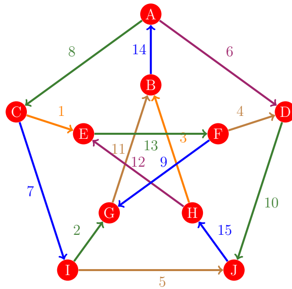
Figura 1066: Flujo 1058 de la gráfica de Petersen
