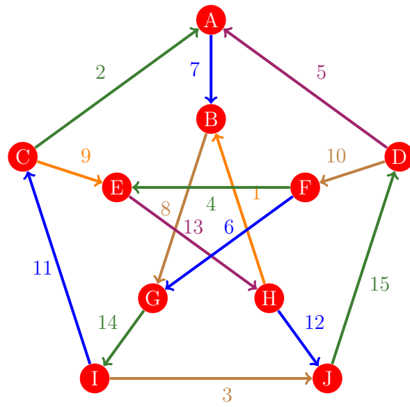
Figura 530: Flujo 522 de la gráfica de Petersen
