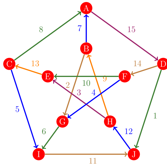
Figura 510: Flujo 502 de la gráfica de Petersen
