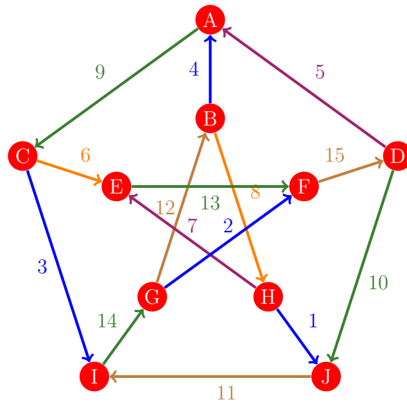
Figura 274: Flujo 266 de la gráfica de Petersen
