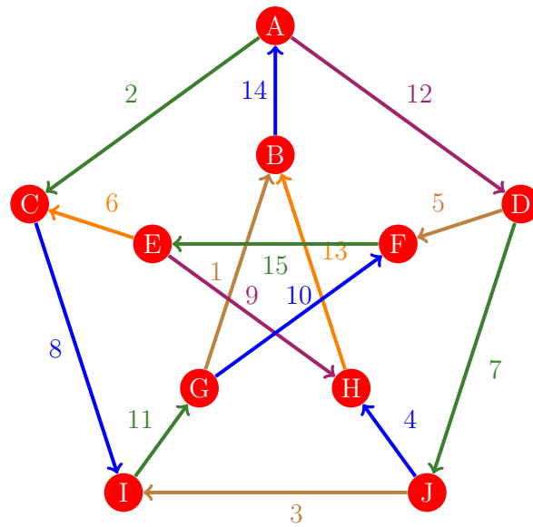
Figura 1054: Flujo 1046 de la gráfica de Petersen
