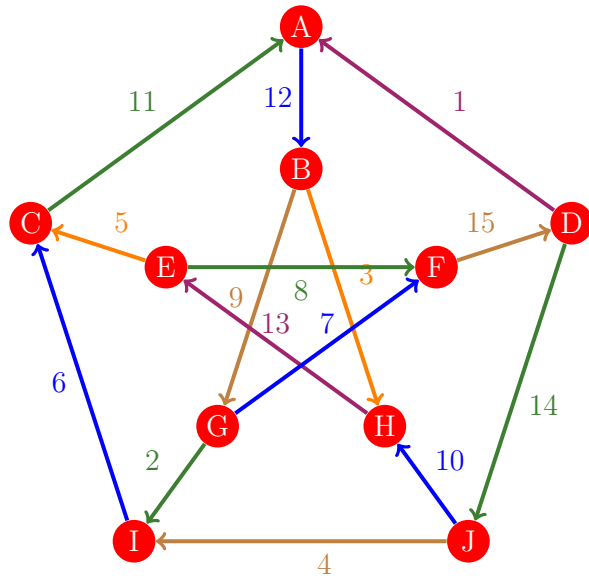
Figura 953: Flujo 945 de la gráfica de Petersen
