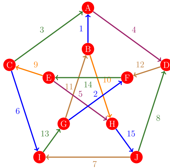
Figura 10: Flujo 2 de la gráfica de Petersen
