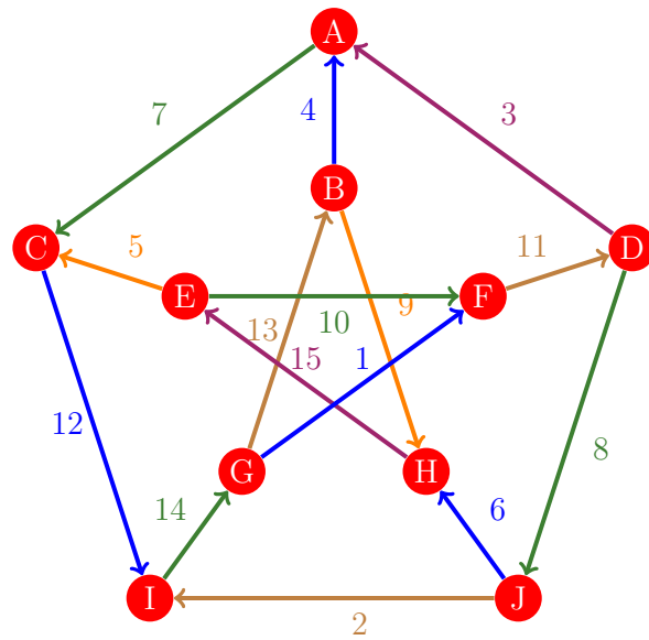
Figura 264: Flujo 256 de la gráfica de Petersen
