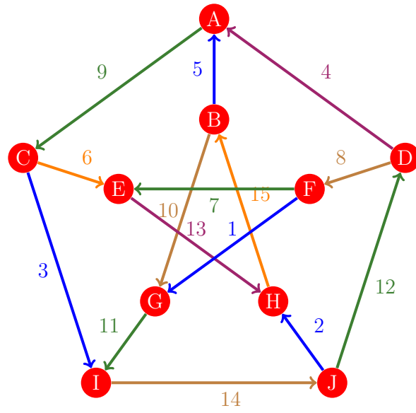
Figura 343: Flujo 335 de la gráfica de Petersen
