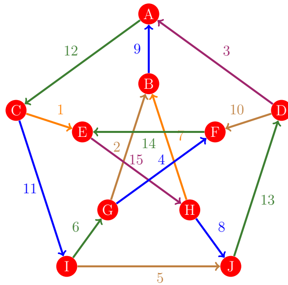
Figura 680: Flujo 672 de la gráfica de Petersen
