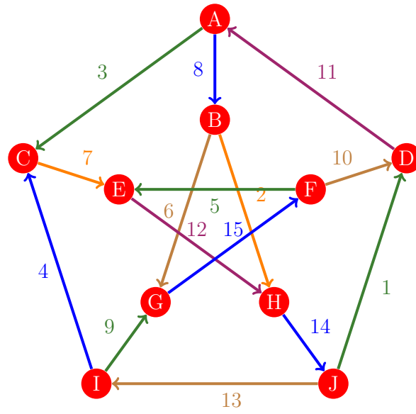
Figura 611: Flujo 603 de la gráfica de Petersen
