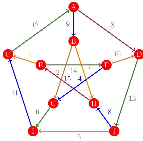
Figura 720: Flujo 712 de la gráfica de Petersen
