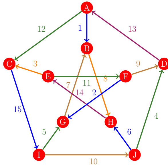
Figura 77: Flujo 69 de la gráfica de Petersen
