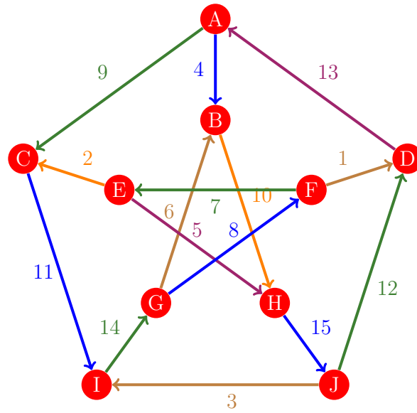
Figura 311: Flujo 303 de la gráfica de Petersen
