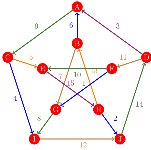
Figura 433: Flujo 425 de la gráfica de Petersen
