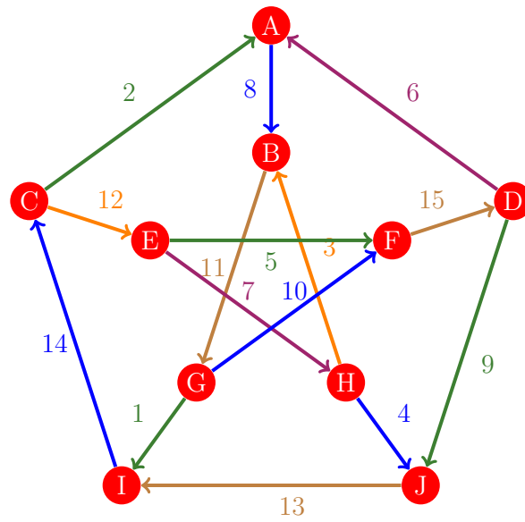
Figura 610: Flujo 602 de la gráfica de Petersen
