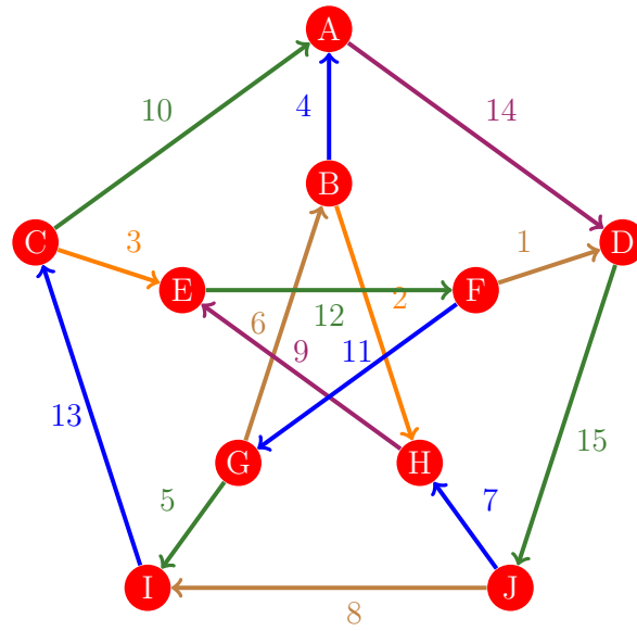
Figura 275: Flujo 267 de la gráfica de Petersen
