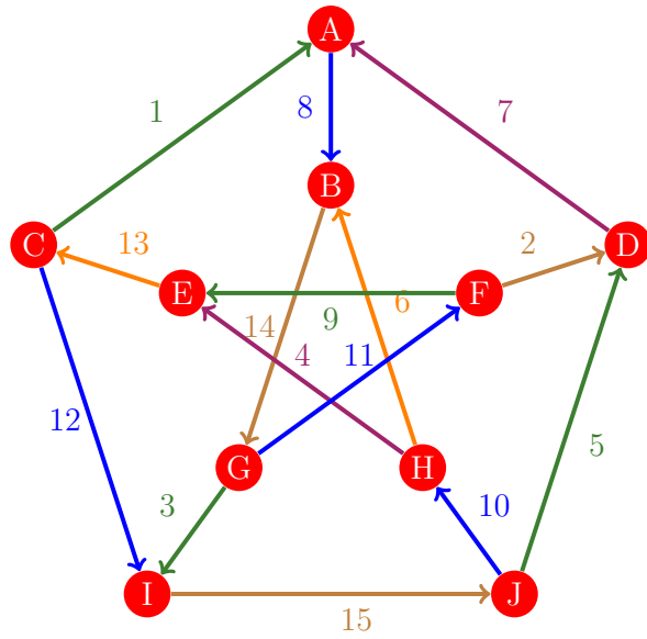
Figura 634: Flujo 626 de la gráfica de Petersen
