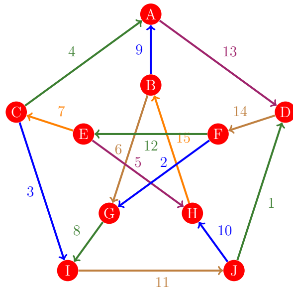
Figura 660: Flujo 652 de la gráfica de Petersen
