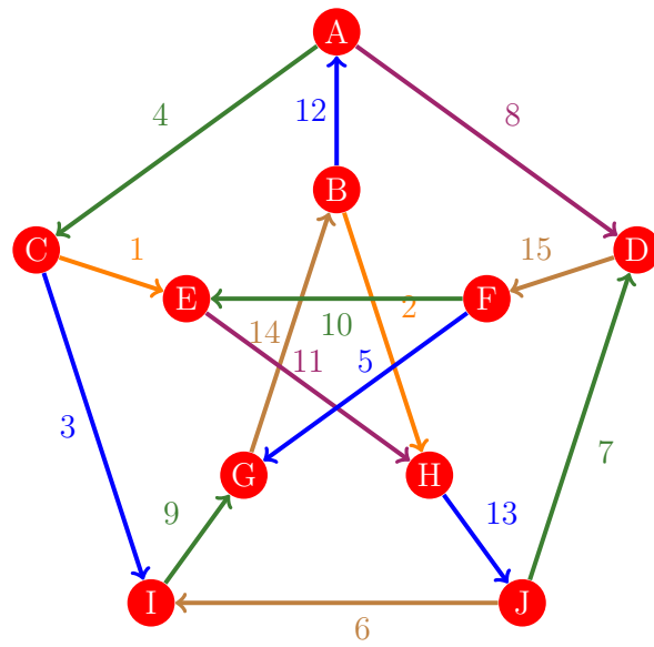
Figura 901: Flujo 893 de la gráfica de Petersen
