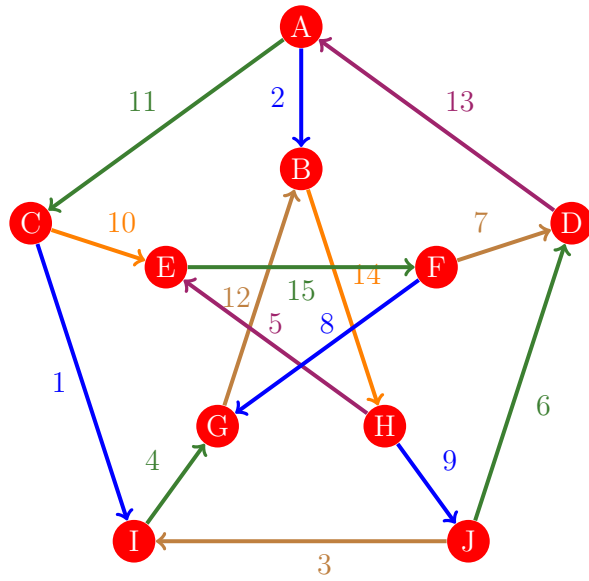
Figura 149: Flujo 141 de la gráfica de Petersen
