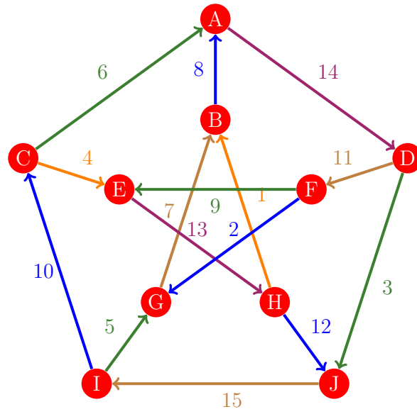
Figura 579: Flujo 571 de la gráfica de Petersen
