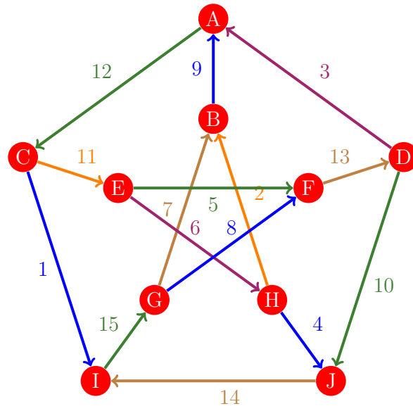
Figura 679: Flujo 671 de la gráfica de Petersen
