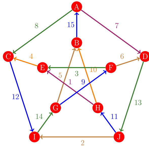
Figura 1147: Flujo 1139 de la gráfica de Petersen
