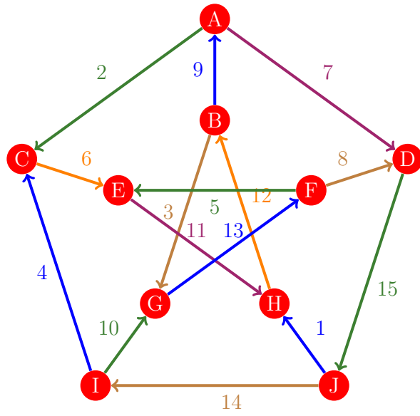
Figura 651: Flujo 643 de la gráfica de Petersen
