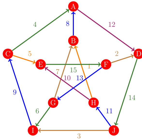
Figura 573: Flujo 565 de la gráfica de Petersen
