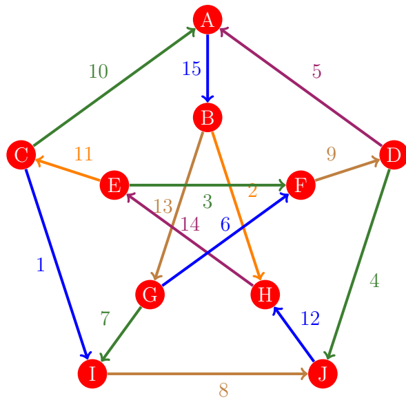
Figura 1200: Flujo 1192 de la gráfica de Petersen
