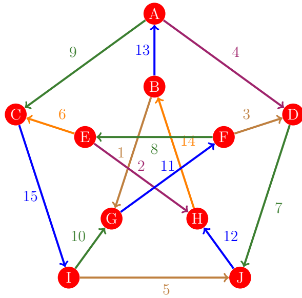
Figura 993: Flujo 985 de la gráfica de Petersen
