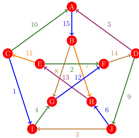
Figura 1196: Flujo 1188 de la gráfica de Petersen
