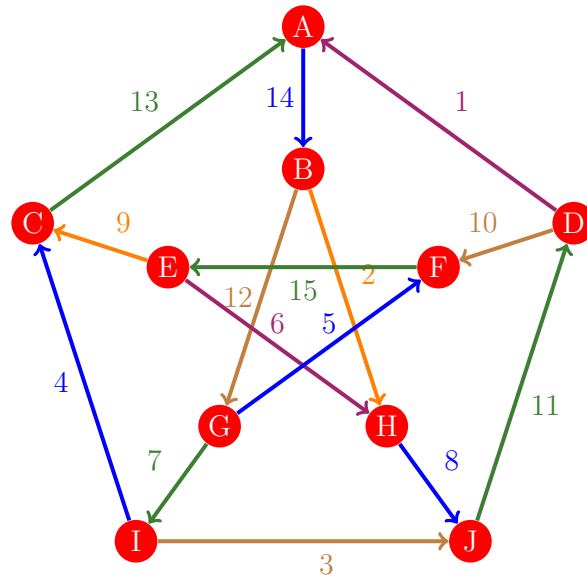
Figura 1121: Flujo 1113 de la gráfica de Petersen
