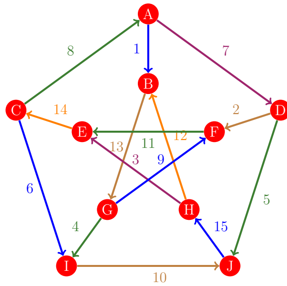
Figura 60: Flujo 52 de la gráfica de Petersen
