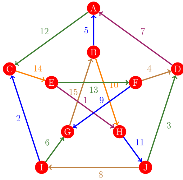
Figura 356: Flujo 348 de la gráfica de Petersen
