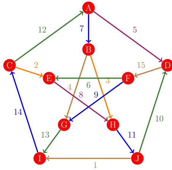
Figura 559: Flujo 551 de la gráfica de Petersen
