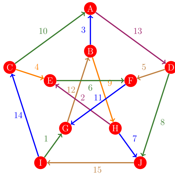
Figura 190: Flujo 182 de la gráfica de Petersen
