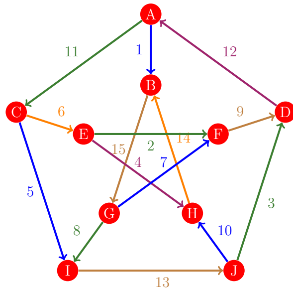
Figura 74: Flujo 66 de la gráfica de Petersen
