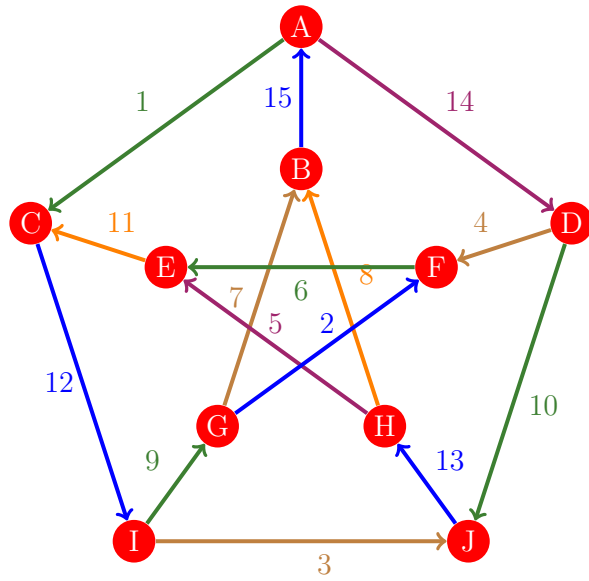
Figura 1167: Flujo 1159 de la gráfica de Petersen
