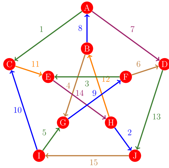
Figura 591: Flujo 583 de la gráfica de Petersen
