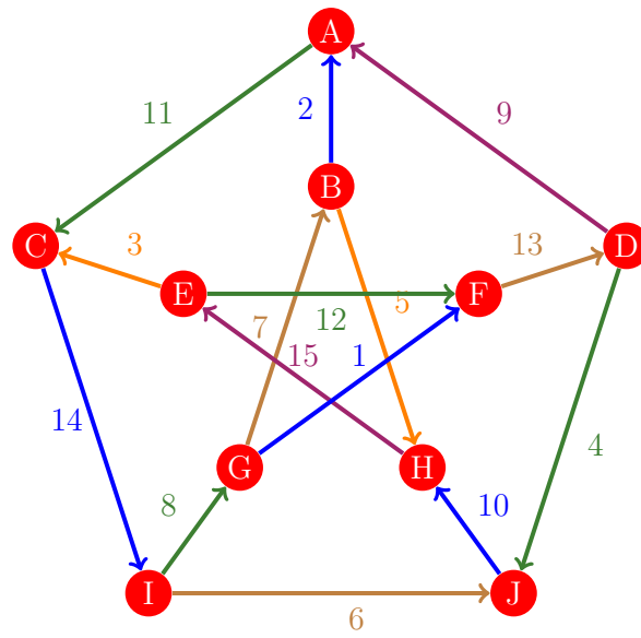
Figura 110: Flujo 102 de la gráfica de Petersen
