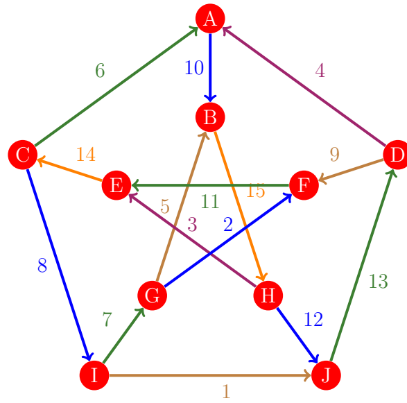
Figura 783: Flujo 775 de la gráfica de Petersen
