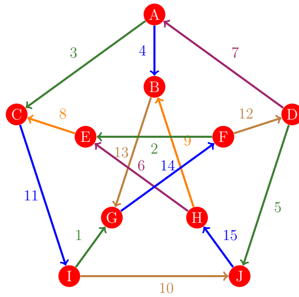
Figura 294: Flujo 286 de la gráfica de Petersen
