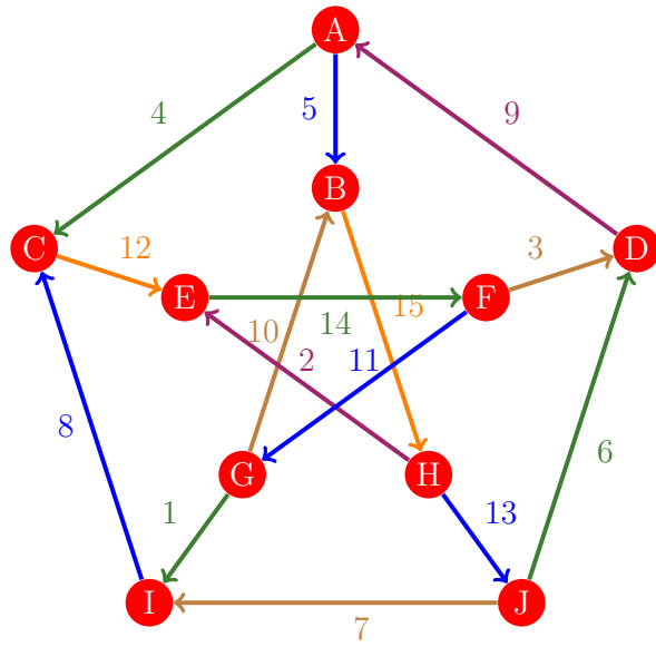
Figura 371: Flujo 363 de la gráfica de Petersen
