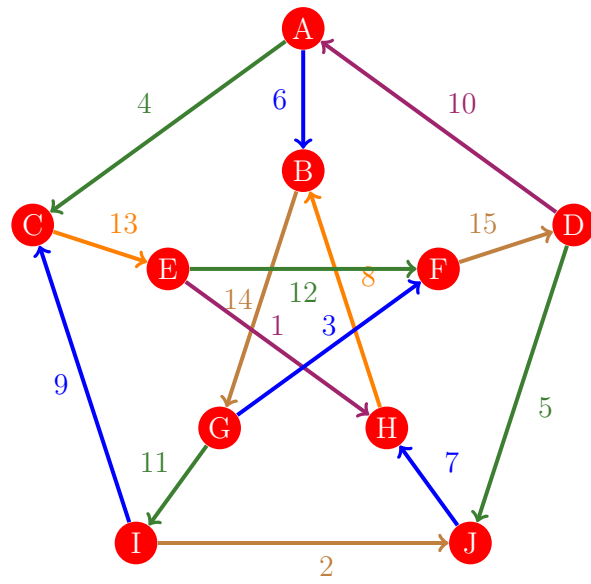
Figura 460: Flujo 452 de la gráfica de Petersen
