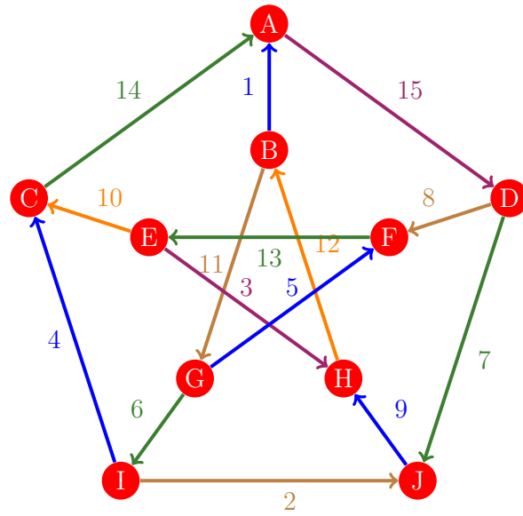
Figura 43: Flujo 35 de la gráfica de Petersen
