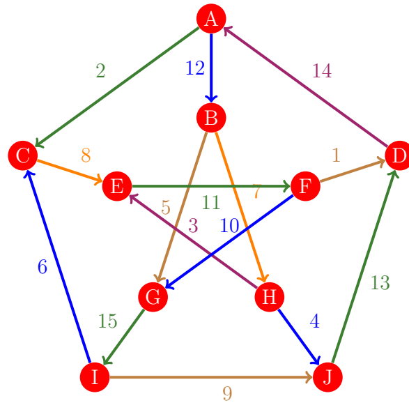
Figura 931: Flujo 923 de la gráfica de Petersen
