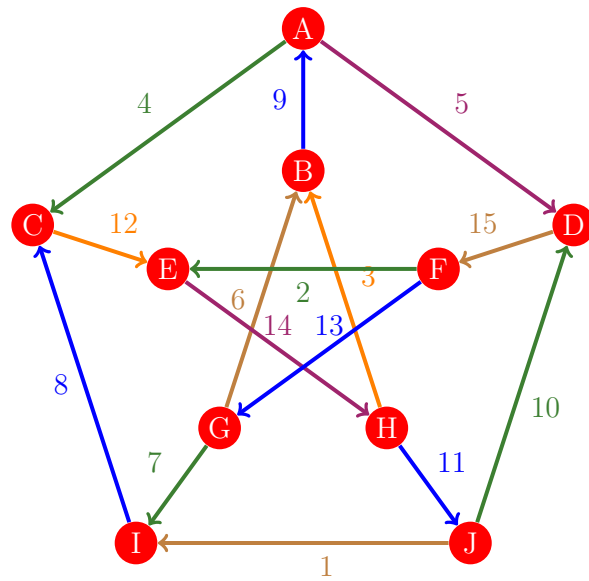
Figura 664: Flujo 656 de la gráfica de Petersen
