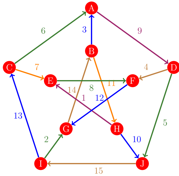
Figura 178: Flujo 170 de la gráfica de Petersen
