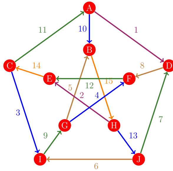
Figura 793: Flujo 785 de la gráfica de Petersen
