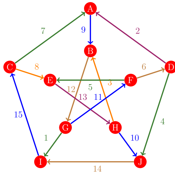
Figura 716: Flujo 708 de la gráfica de Petersen
