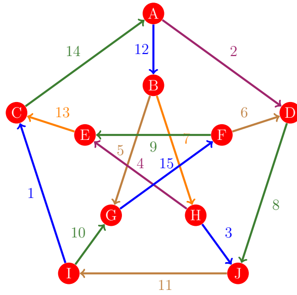
Figura 963: Flujo 955 de la gráfica de Petersen
