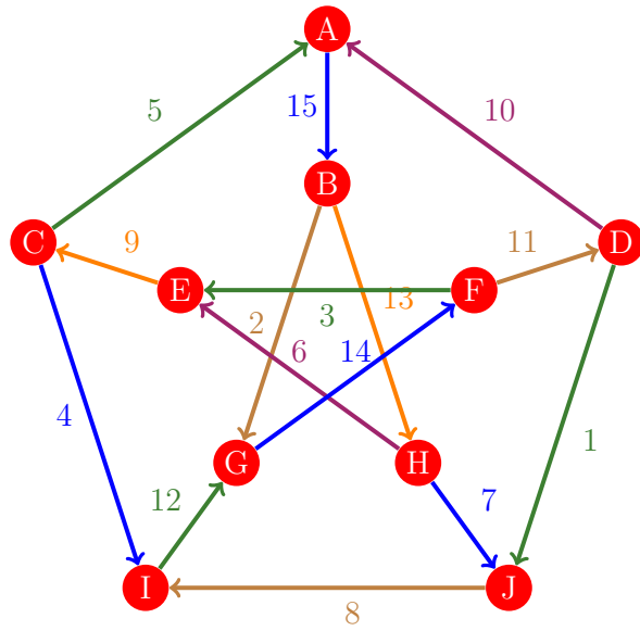
Figura 1173: Flujo 1165 de la gráfica de Petersen
