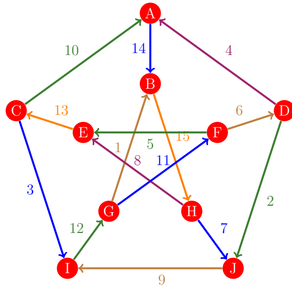
Figura 1109: Flujo 1101 de la gráfica de Petersen
