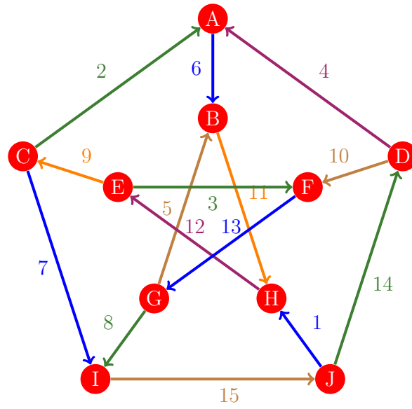
Figura 449: Flujo 441 de la gráfica de Petersen
