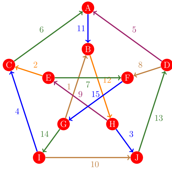
Figura 861: Flujo 853 de la gráfica de Petersen
