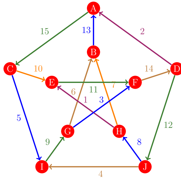
Figura 1007: Flujo 999 de la gráfica de Petersen
