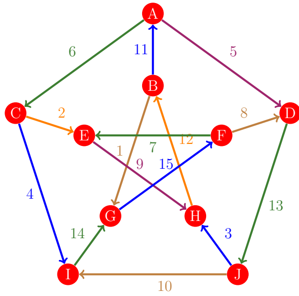
Figura 821: Flujo 813 de la gráfica de Petersen
