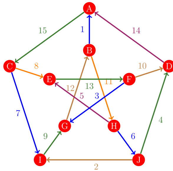
Figura 48: Flujo 40 de la gráfica de Petersen
