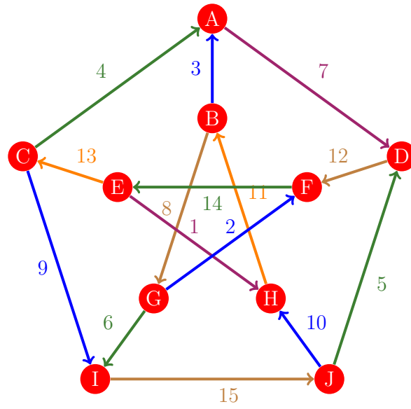
Figura 171: Flujo 163 de la gráfica de Petersen
