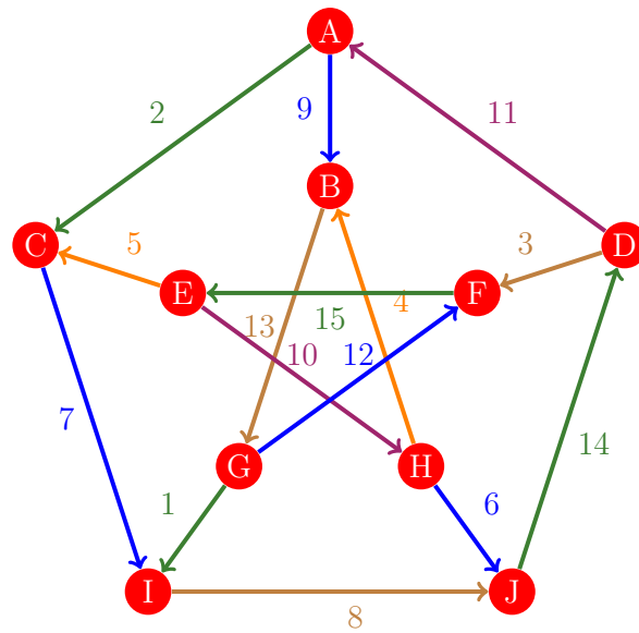
Figura 692: Flujo 684 de la gráfica de Petersen
