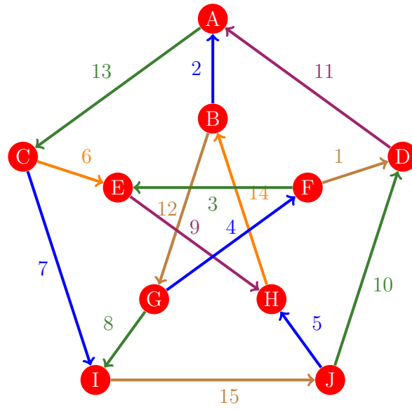
Figura 119: Flujo 111 de la gráfica de Petersen
