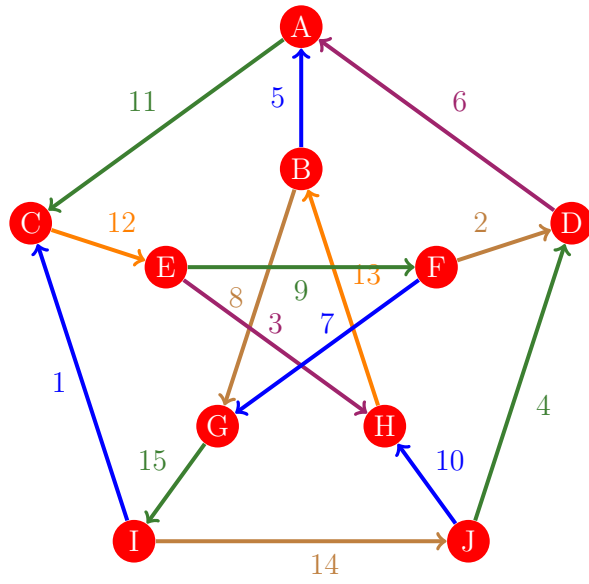
Figura 353: Flujo 345 de la gráfica de Petersen
