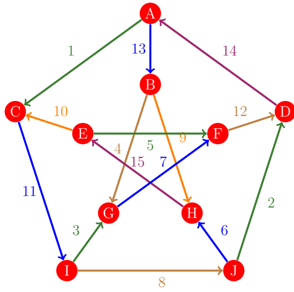
Figura 1043: Flujo 1035 de la gráfica de Petersen
