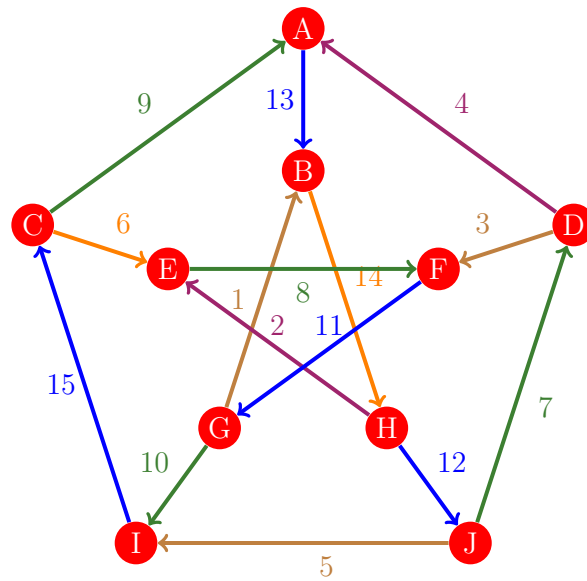
Figura 1032: Flujo 1024 de la gráfica de Petersen
