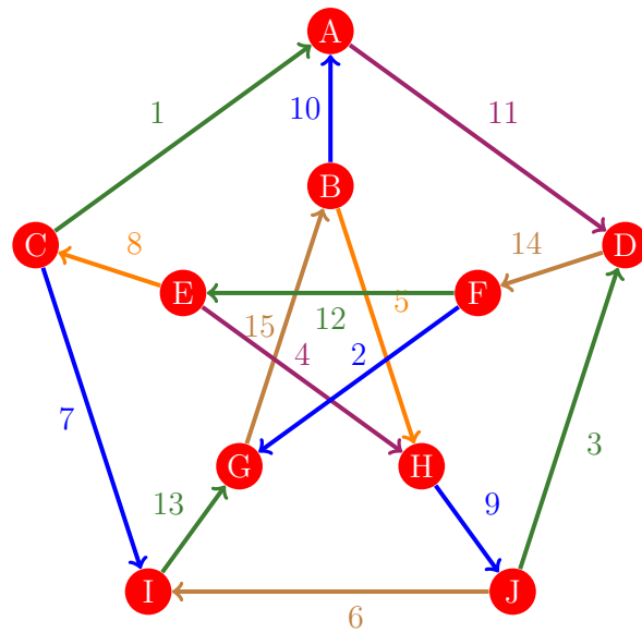
Figura 748: Flujo 740 de la gráfica de Petersen
