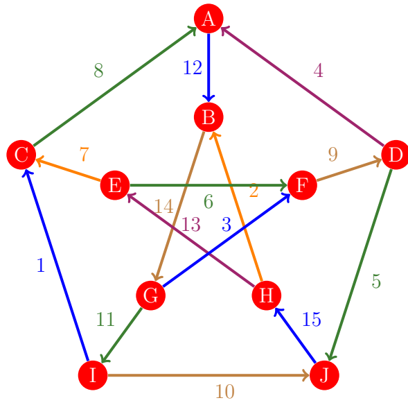
Figura 949: Flujo 941 de la gráfica de Petersen
