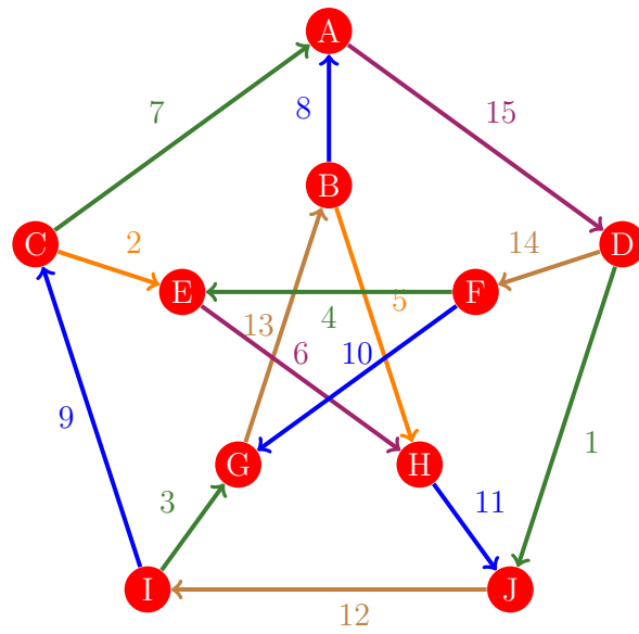
Figura 586: Flujo 578 de la gráfica de Petersen
