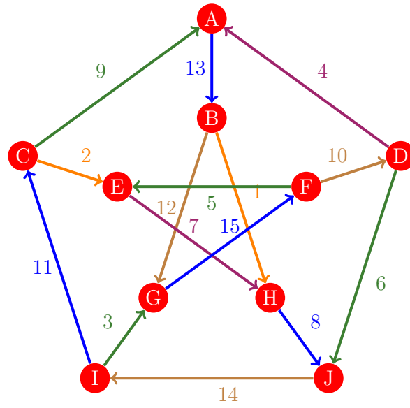
Figura 1031: Flujo 1023 de la gráfica de Petersen
