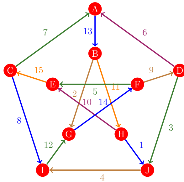
Figura 1026: Flujo 1018 de la gráfica de Petersen
