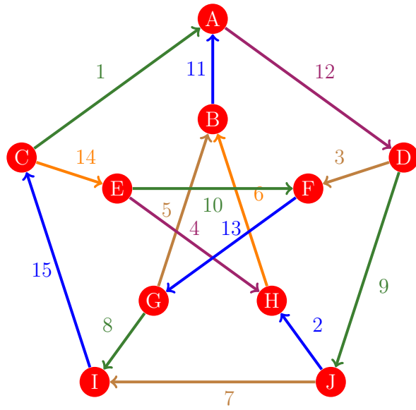
Figura 833: Flujo 825 de la gráfica de Petersen
