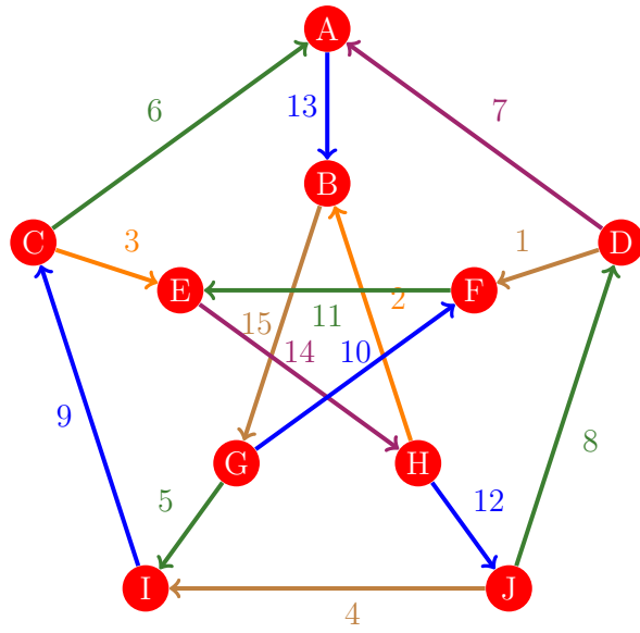
Figura 1024: Flujo 1016 de la gráfica de Petersen
