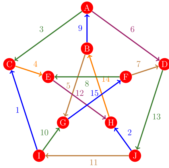
Figura 657: Flujo 649 de la gráfica de Petersen
