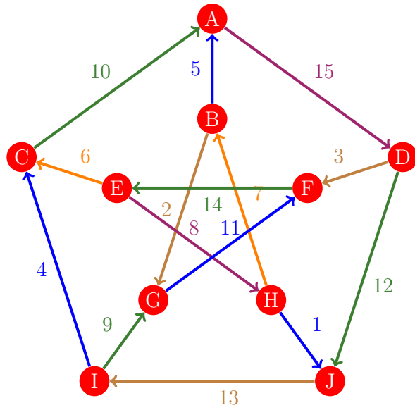
Figura 350: Flujo 342 de la gráfica de Petersen
