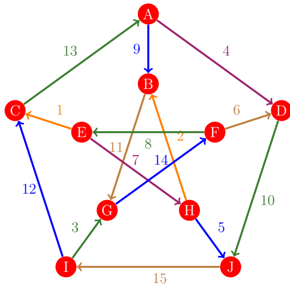
Figura 722: Flujo 714 de la gráfica de Petersen
