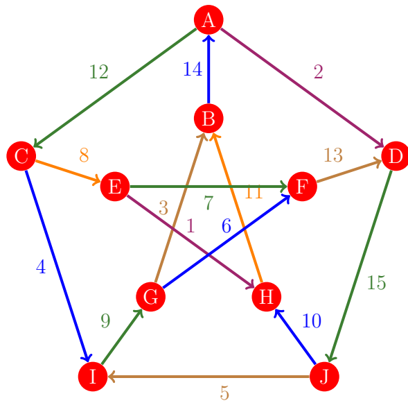
Figura 1078: Flujo 1070 de la gráfica de Petersen
