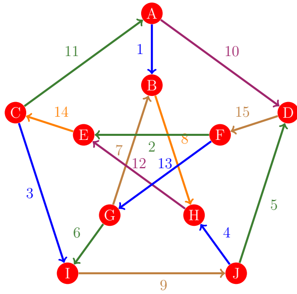
Figura 68: Flujo 60 de la gráfica de Petersen
