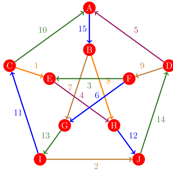
Figura 1195: Flujo 1187 de la gráfica de Petersen
