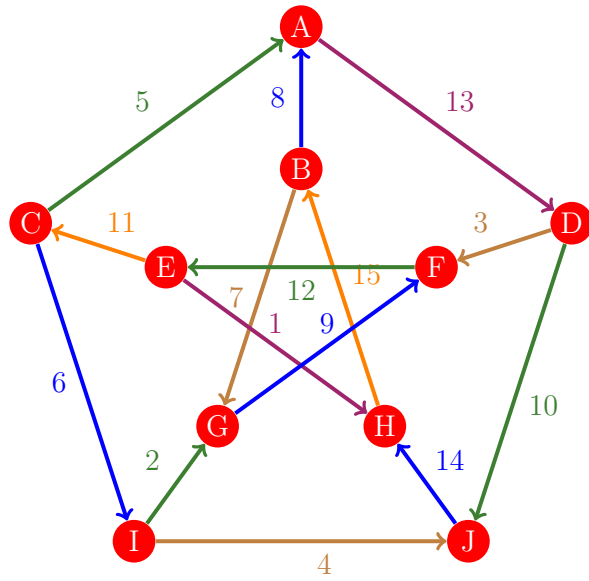
Figura 577: Flujo 569 de la gráfica de Petersen
