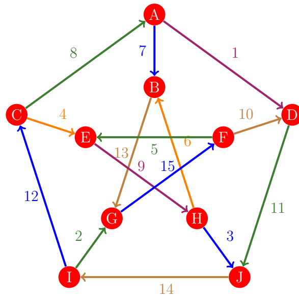
Figura 552: Flujo 544 de la gráfica de Petersen
