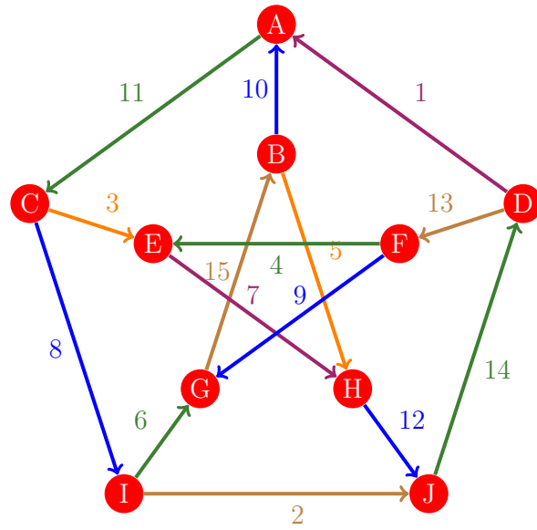
Figura 755: Flujo 747 de la gráfica de Petersen
