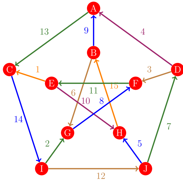
Figura 681: Flujo 673 de la gráfica de Petersen
