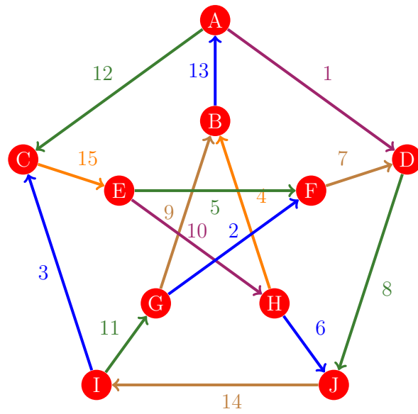
Figura 1000: Flujo 992 de la gráfica de Petersen
