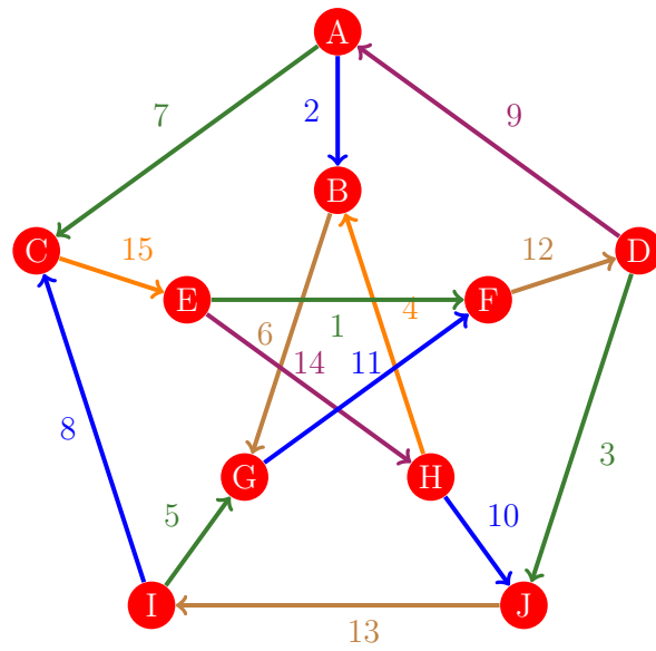
Figura 140: Flujo 132 de la gráfica de Petersen
