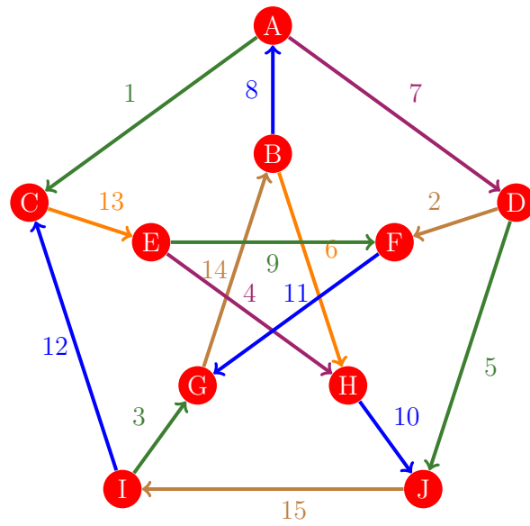
Figura 594: Flujo 586 de la gráfica de Petersen
