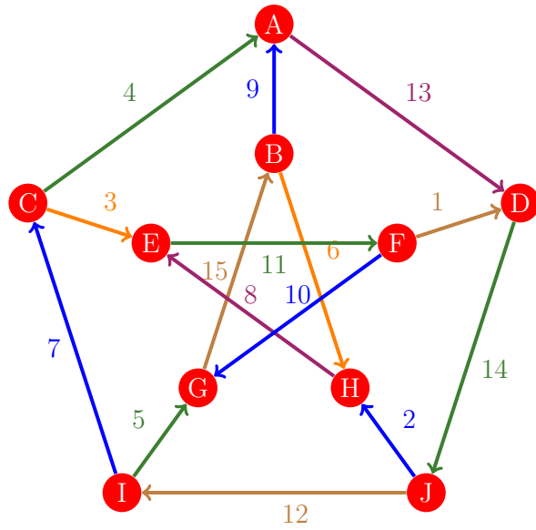
Figura 662: Flujo 654 de la gráfica de Petersen
