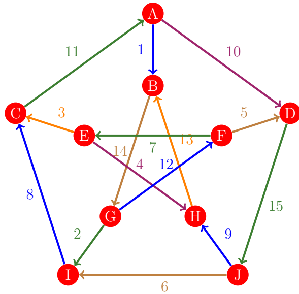
Figura 72: Flujo 64 de la gráfica de Petersen
