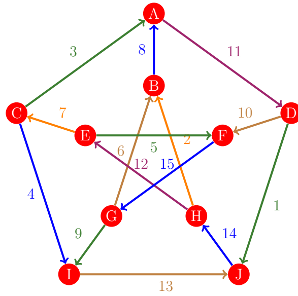
Figura 571: Flujo 563 de la gráfica de Petersen
