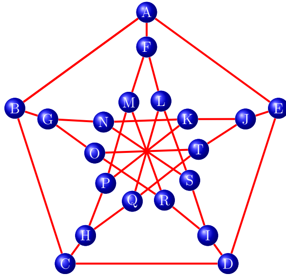
Figura 7: Gráfica G = (20, 30) .
