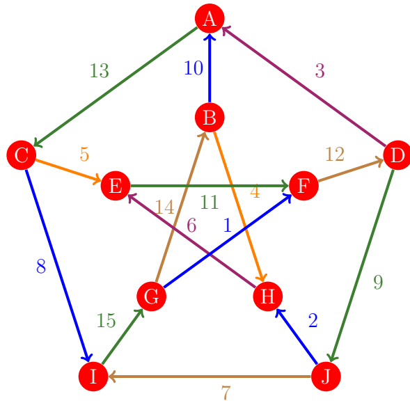
Figura 758: Flujo 750 de la gráfica de Petersen
