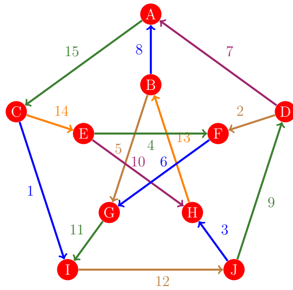
Figura 606: Flujo 598 de la gráfica de Petersen
