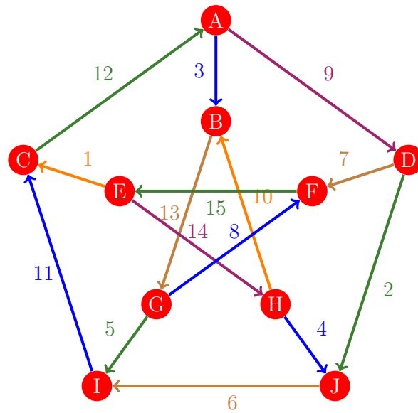
Figura 238: Flujo 230 de la gráfica de Petersen
