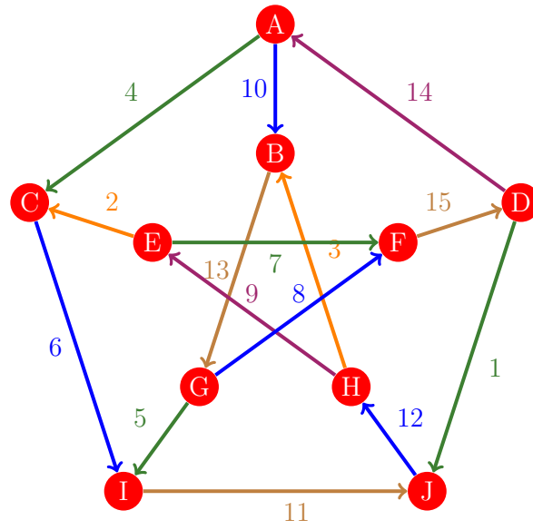
Figura 773: Flujo 765 de la gráfica de Petersen
