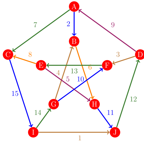
Figura 139: Flujo 131 de la gráfica de Petersen
