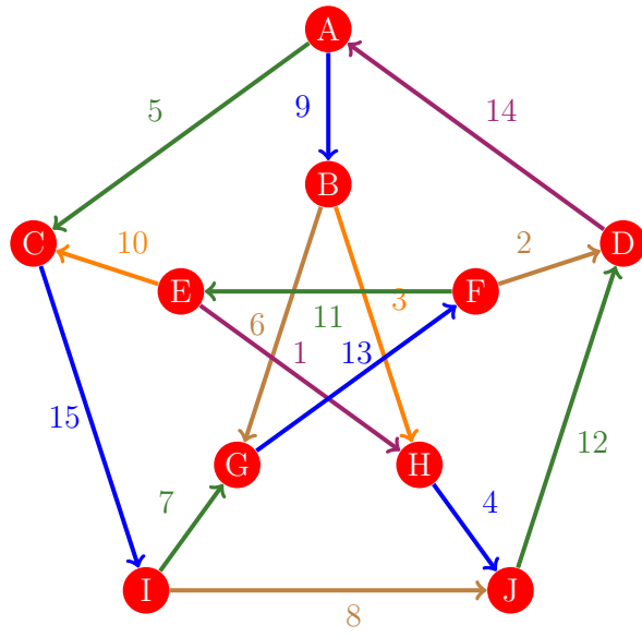
Figura 707: Flujo 699 de la gráfica de Petersen
