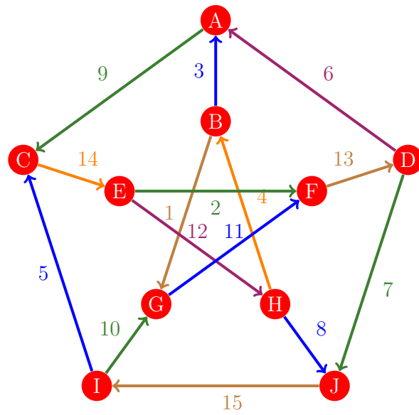
Figura 186: Flujo 178 de la gráfica de Petersen
