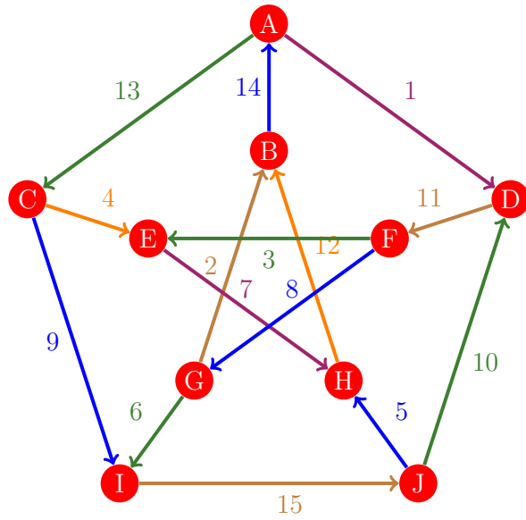
Figura 1082: Flujo 1074 de la gráfica de Petersen
