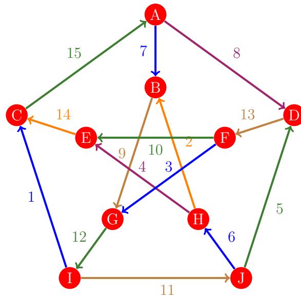
Figura 566: Flujo 558 de la gráfica de Petersen
