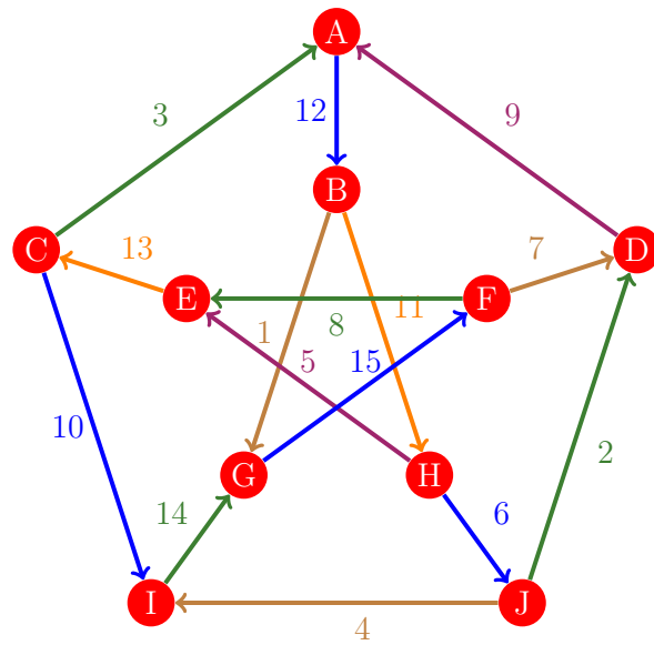
Figura 936: Flujo 928 de la gráfica de Petersen
