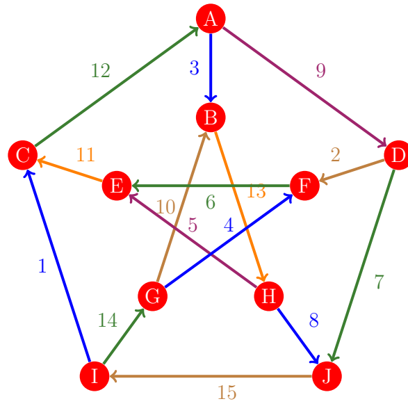
Figura 237: Flujo 229 de la gráfica de Petersen
