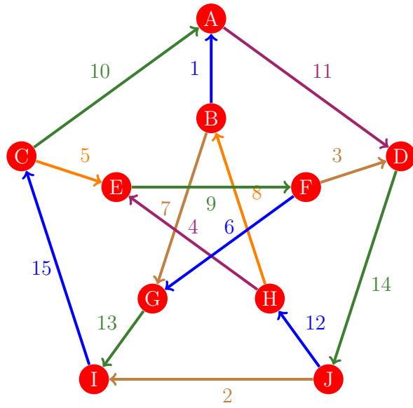
Figura 22: Flujo 14 de la gráfica de Petersen
