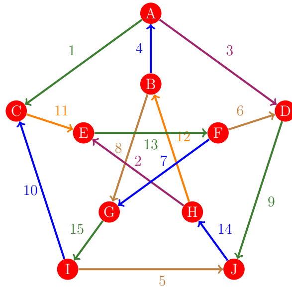
Figura 255: Flujo 247 de la gráfica de Petersen
