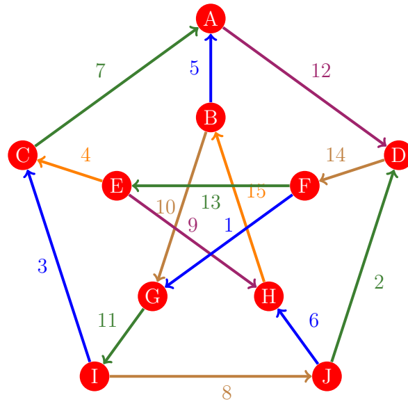
Figura 335: Flujo 327 de la gráfica de Petersen
