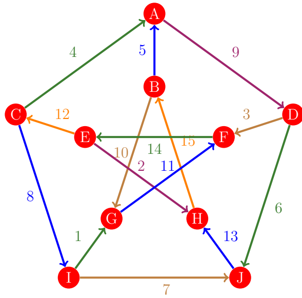
Figura 331: Flujo 323 de la gráfica de Petersen
