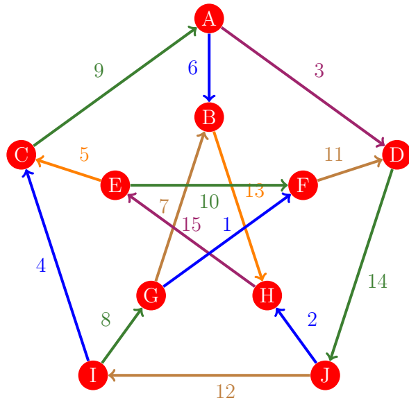
Figura 471: Flujo 463 de la gráfica de Petersen
