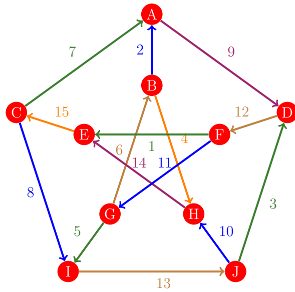
Figura 98: Flujo 90 de la gráfica de Petersen
