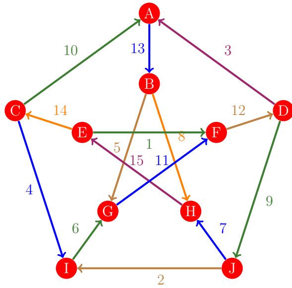
Figura 1035: Flujo 1027 de la gráfica de Petersen
