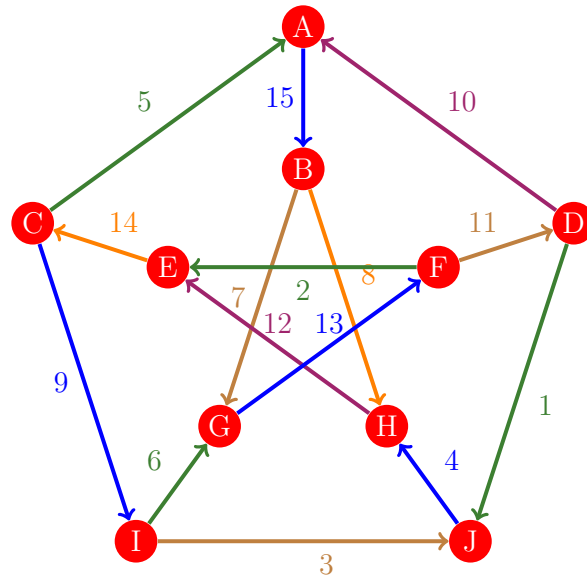
Figura 1175: Flujo 1167 de la gráfica de Petersen
