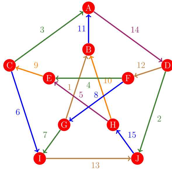
Figura 815: Flujo 807 de la gráfica de Petersen
