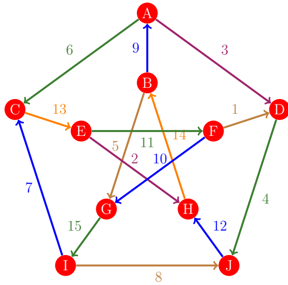
Figura 673: Flujo 665 de la gráfica de Petersen
