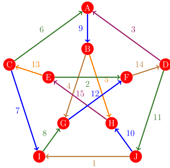
Figura 709: Flujo 701 de la gráfica de Petersen
