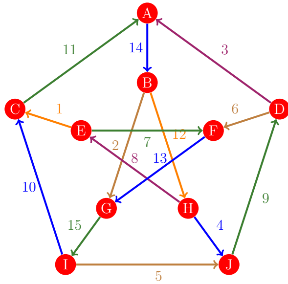
Figura 1113: Flujo 1105 de la gráfica de Petersen
