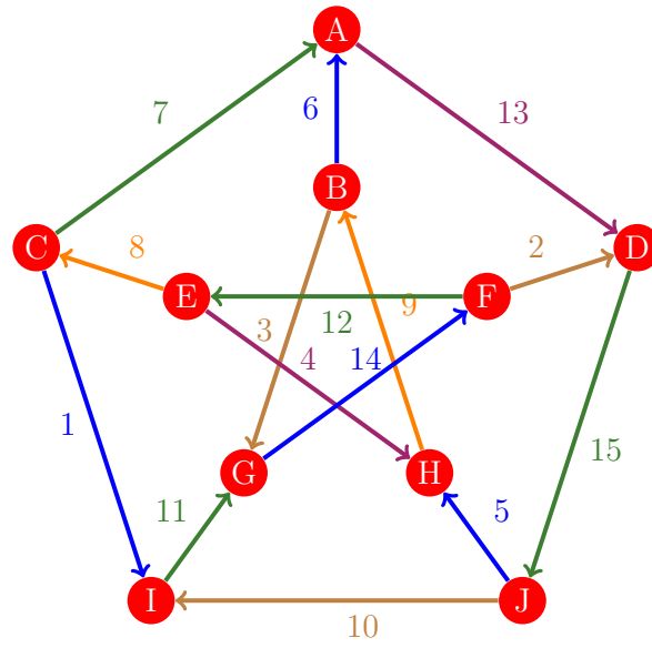
Figura 425: Flujo 417 de la gráfica de Petersen
