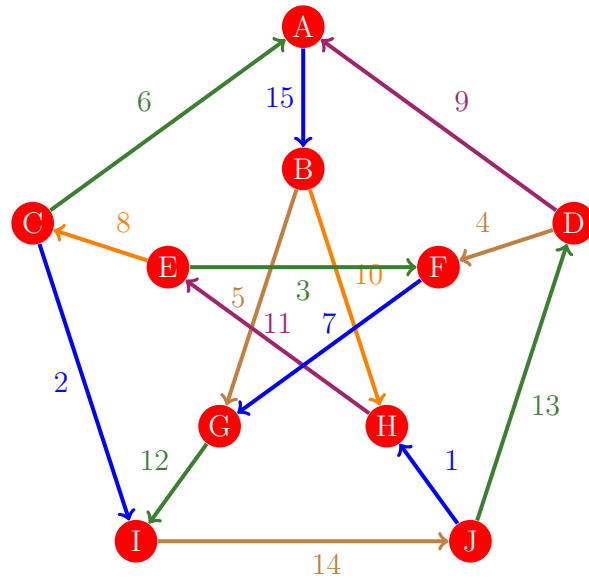
Figura 1181: Flujo 1173 de la gráfica de Petersen
