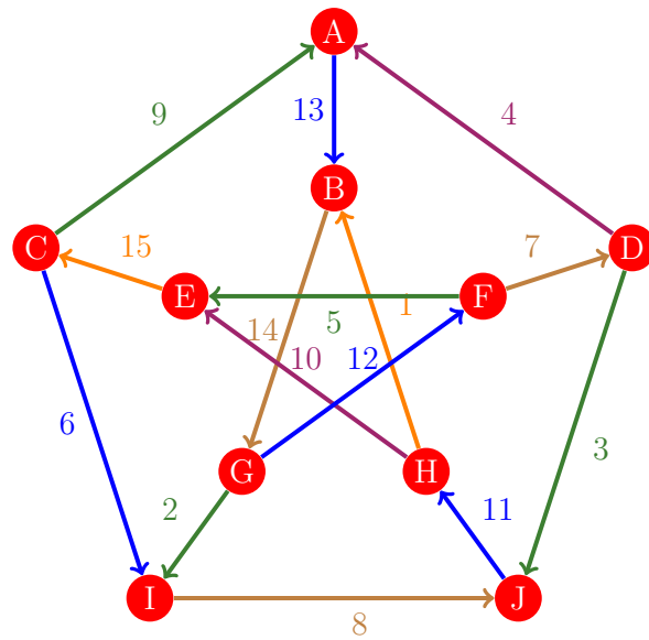
Figura 1034: Flujo 1026 de la gráfica de Petersen
