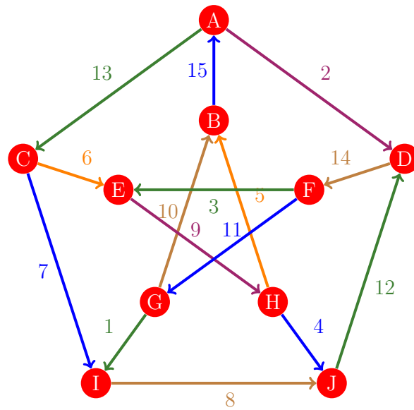
Figura 1164: Flujo 1156 de la gráfica de Petersen
