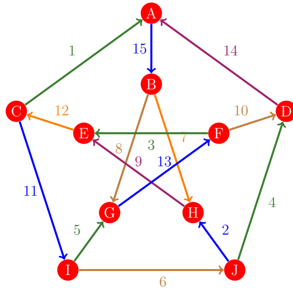
Figura 1208: Flujo 1200 de la gráfica de Petersen
