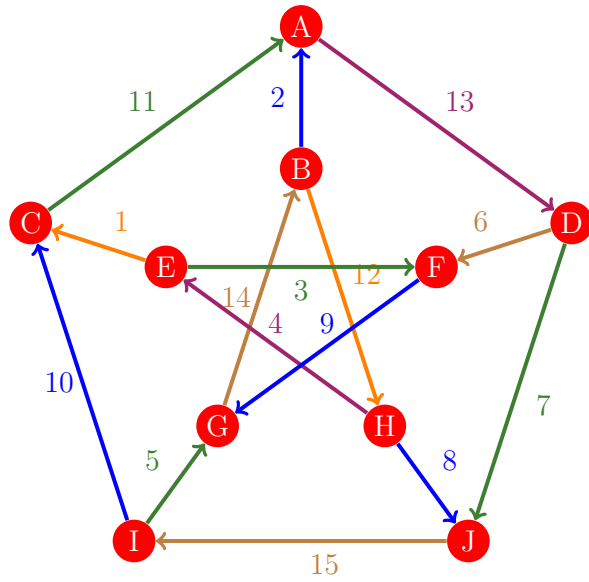
Figura 108: Flujo 100 de la gráfica de Petersen
