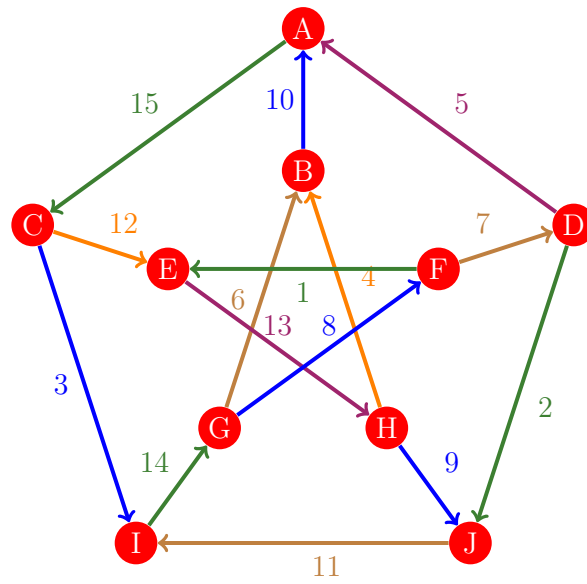
Figura 762: Flujo 754 de la gráfica de Petersen
