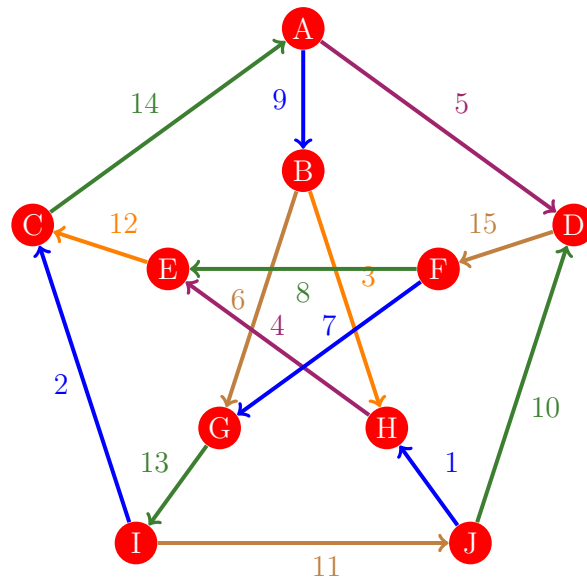
Figura 726: Flujo 718 de la gráfica de Petersen
