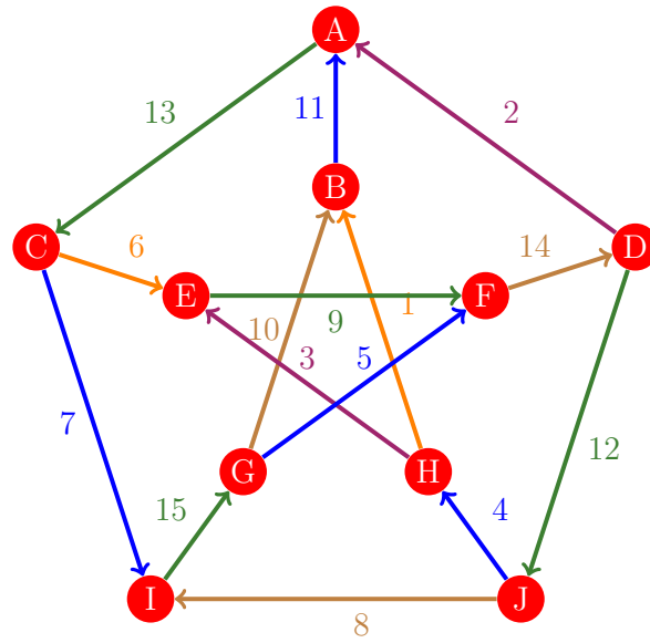
Figura 843: Flujo 835 de la gráfica de Petersen
