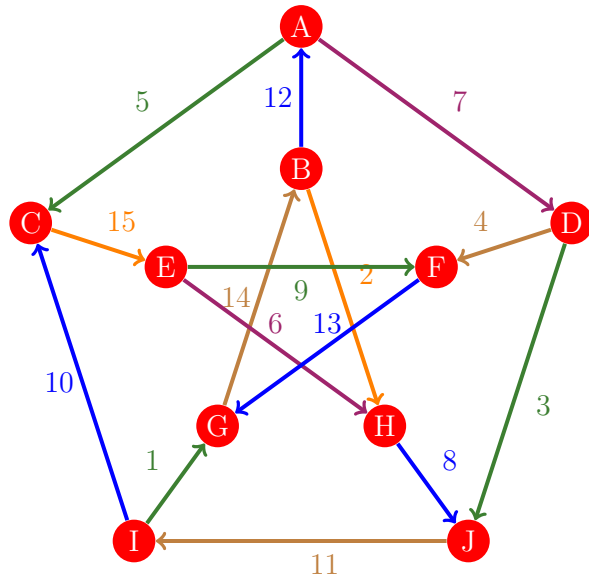
Figura 904: Flujo 896 de la gráfica de Petersen
