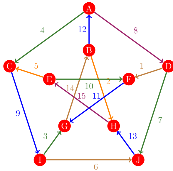
Figura 902: Flujo 894 de la gráfica de Petersen
