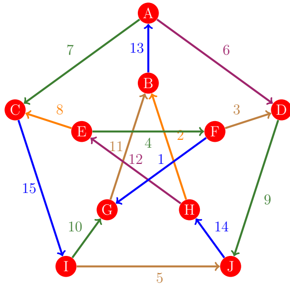
Figura 987: Flujo 979 de la gráfica de Petersen
