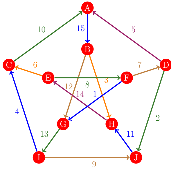
Figura 1199: Flujo 1191 de la gráfica de Petersen
