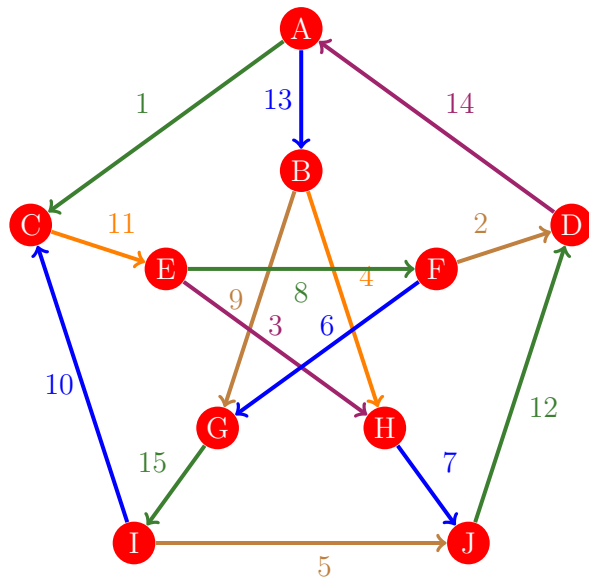
Figura 1044: Flujo 1036 de la gráfica de Petersen
