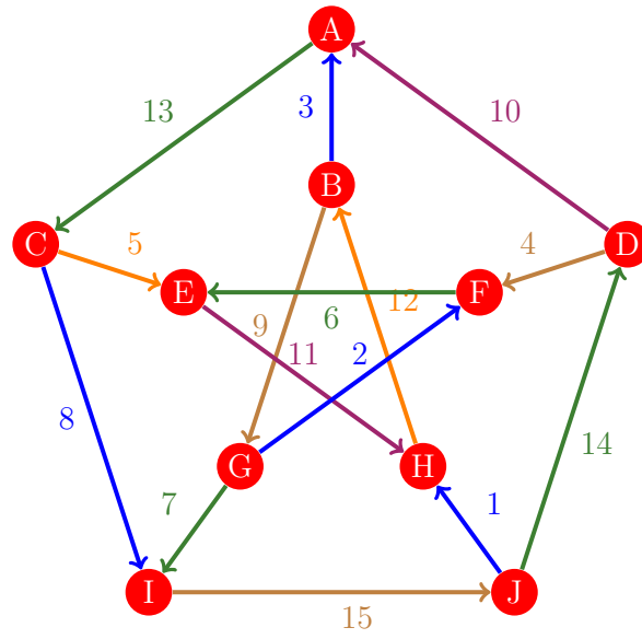
Figura 201: Flujo 193 de la gráfica de Petersen
