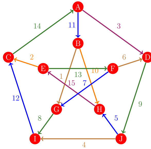
Figura 887: Flujo 879 de la gráfica de Petersen
