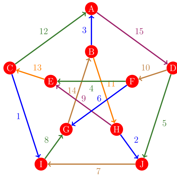
Figura 198: Flujo 190 de la gráfica de Petersen
