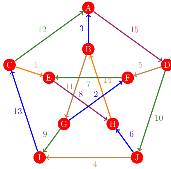
Figura 197: Flujo 189 de la gráfica de Petersen
