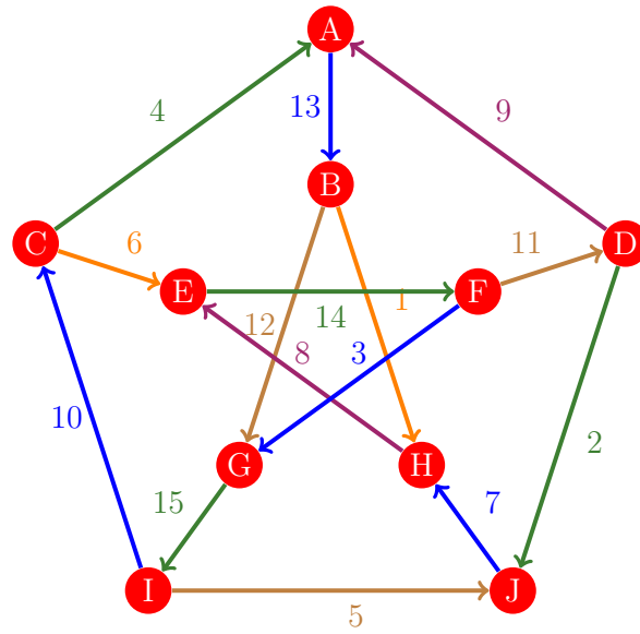
Figura 1015: Flujo 1007 de la gráfica de Petersen
