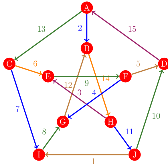
Figura 159: Flujo 151 de la gráfica de Petersen
