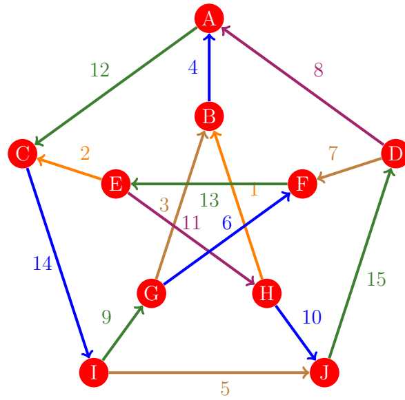
Figura 281: Flujo 273 de la gráfica de Petersen
