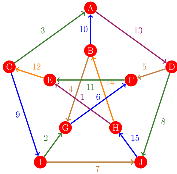
Figura 729: Flujo 721 de la gráfica de Petersen
