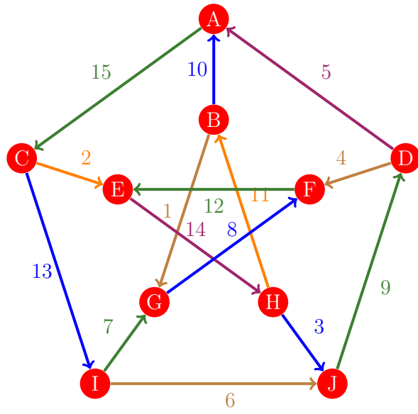
Figura 765: Flujo 757 de la gráfica de Petersen
