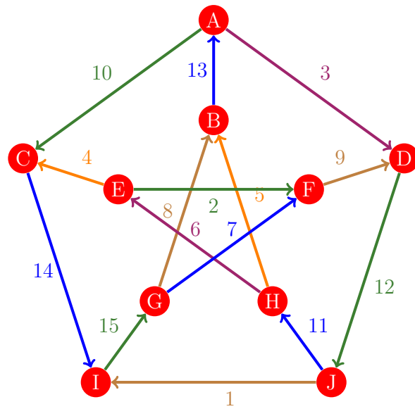
Figura 996: Flujo 988 de la gráfica de Petersen
