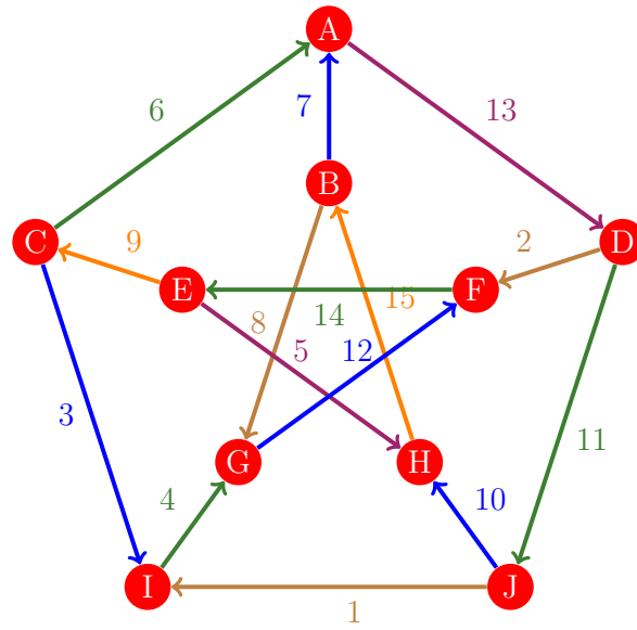
Figura 503: Flujo 495 de la gráfica de Petersen
