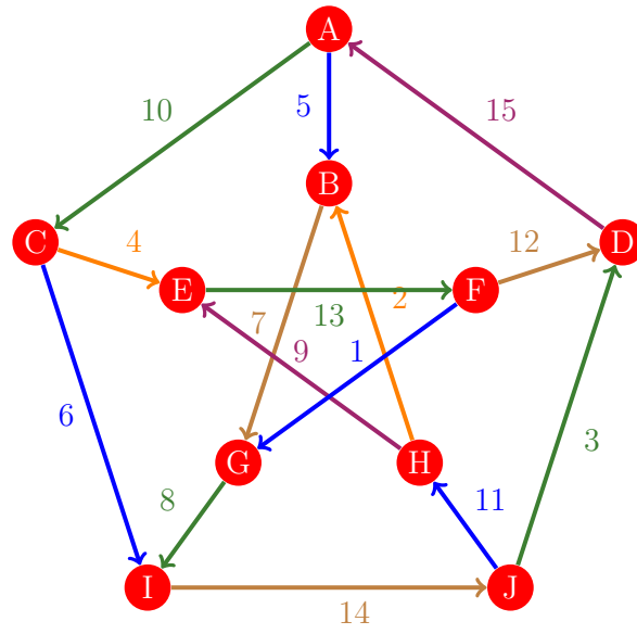
Figura 387: Flujo 379 de la gráfica de Petersen
