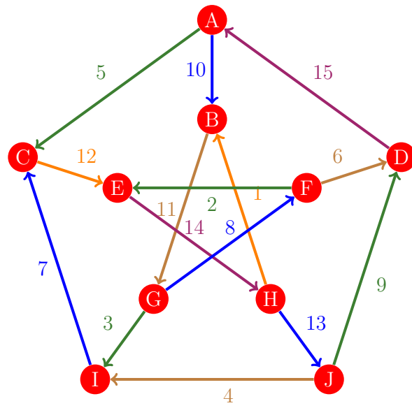
Figura 782: Flujo 774 de la gráfica de Petersen
