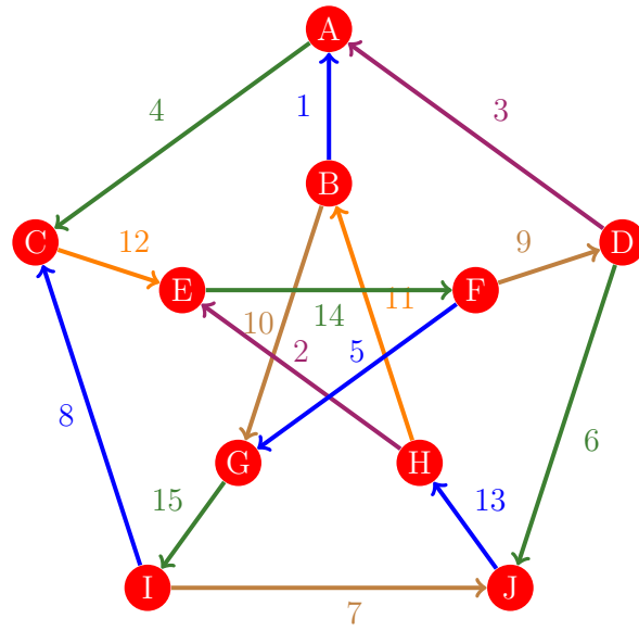
Figura 11: Flujo 3 de la gráfica de Petersen
