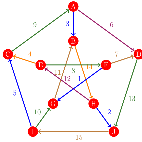
Figura 225: Flujo 217 de la gráfica de Petersen
