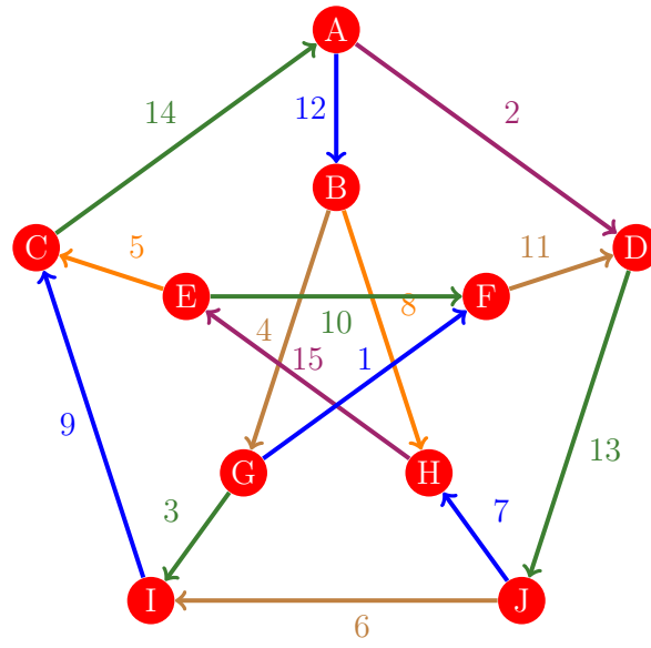
Figura 961: Flujo 953 de la gráfica de Petersen
