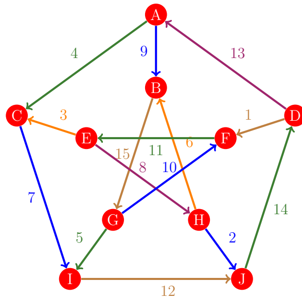
Figura 704: Flujo 696 de la gráfica de Petersen
