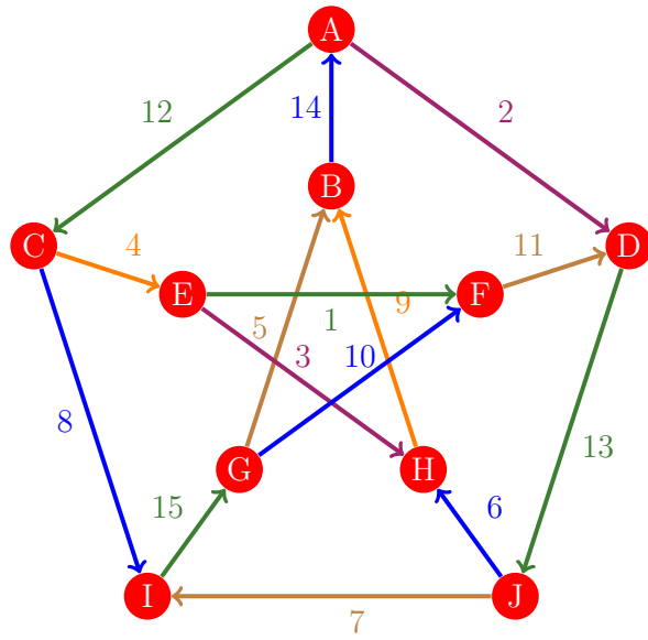
Figura 1075: Flujo 1067 de la gráfica de Petersen
