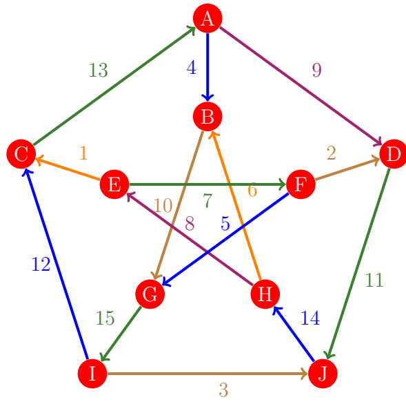
Figura 326: Flujo 318 de la gráfica de Petersen
