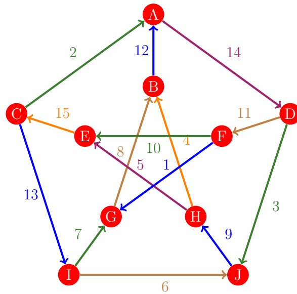
Figura 894: Flujo 886 de la gráfica de Petersen
