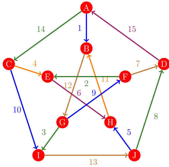
Figura 86: Flujo 78 de la gráfica de Petersen
