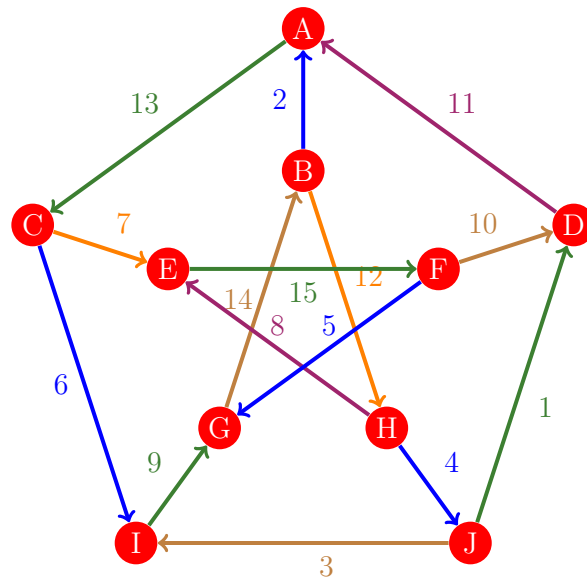
Figura 120: Flujo 112 de la gráfica de Petersen
