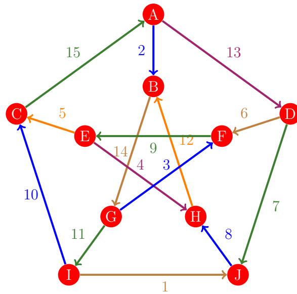
Figura 168: Flujo 160 de la gráfica de Petersen
