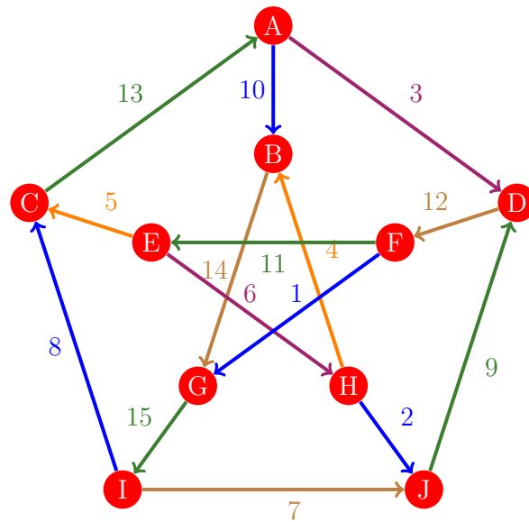
Figura 798: Flujo 790 de la gráfica de Petersen
