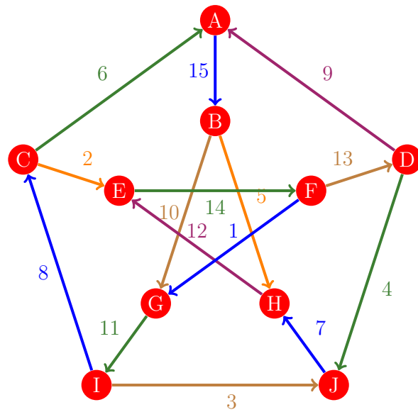
Figura 1182: Flujo 1174 de la gráfica de Petersen
