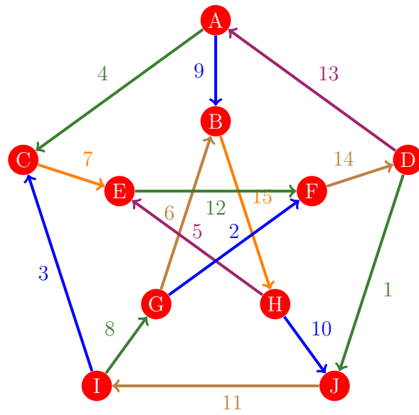
Figura 702: Flujo 694 de la gráfica de Petersen
