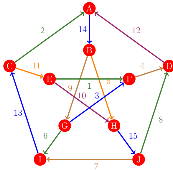
Figura 1090: Flujo 1082 de la gráfica de Petersen
