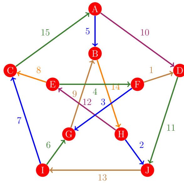
Figura 404: Flujo 396 de la gráfica de Petersen
