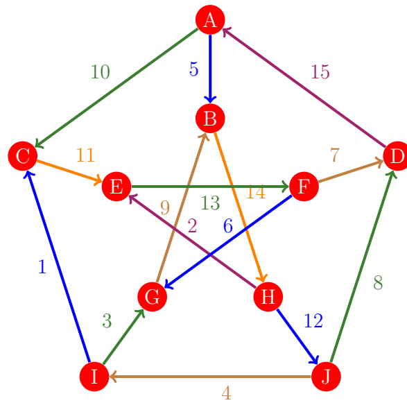
Figura 388: Flujo 380 de la gráfica de Petersen
