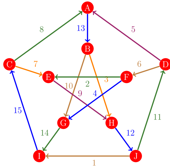
Figura 1030: Flujo 1022 de la gráfica de Petersen
