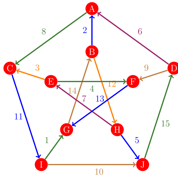
Figura 102: Flujo 94 de la gráfica de Petersen
