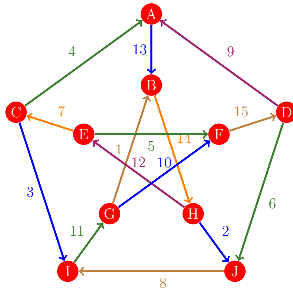
Figura 1016: Flujo 1008 de la gráfica de Petersen
