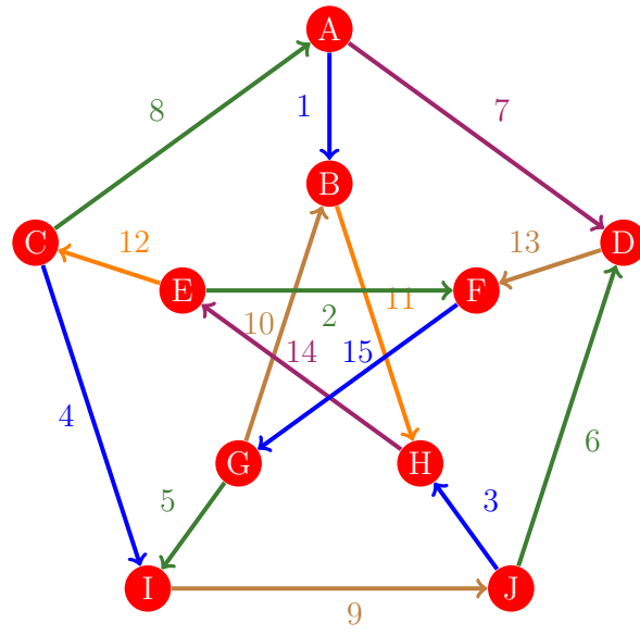
Figura 57: Flujo 49 de la gráfica de Petersen
