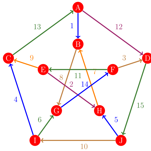
Figura 80: Flujo 72 de la gráfica de Petersen
