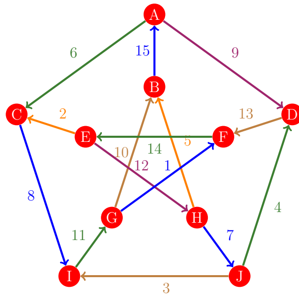
Figura 1142: Flujo 1134 de la gráfica de Petersen
