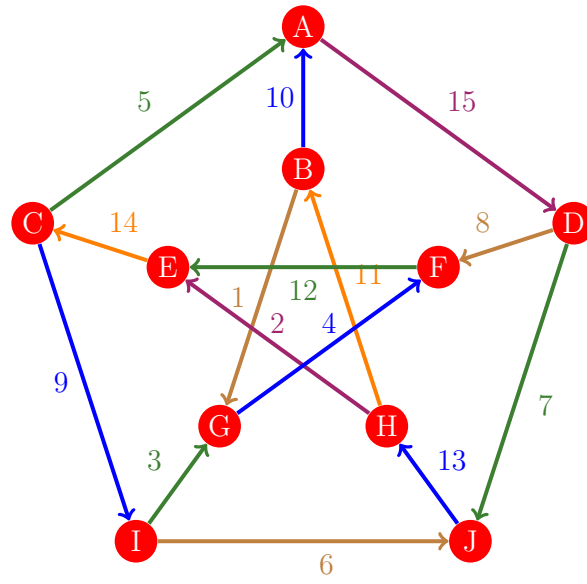
Figura 739: Flujo 731 de la gráfica de Petersen
