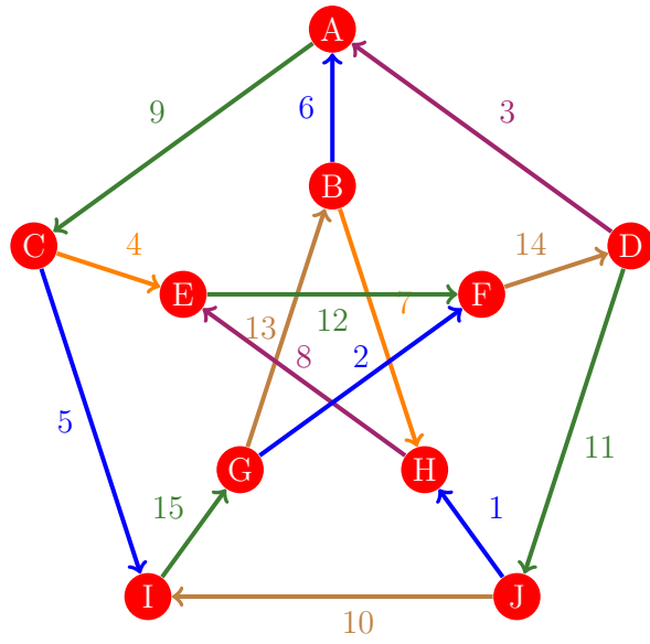
Figura 436: Flujo 428 de la gráfica de Petersen
