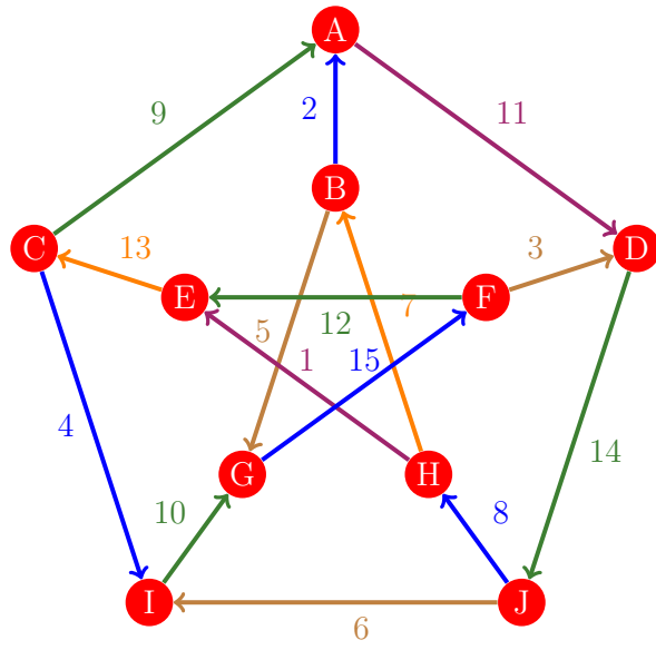
Figura 103: Flujo 95 de la gráfica de Petersen
