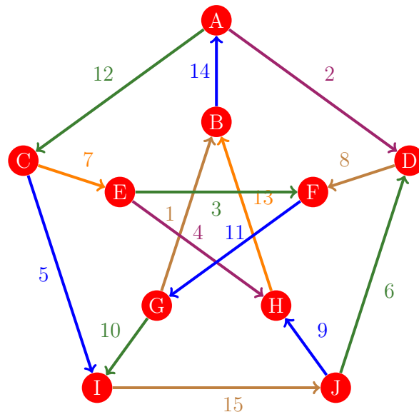
Figura 1080: Flujo 1072 de la gráfica de Petersen
