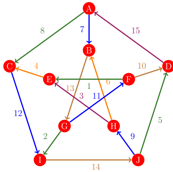
Figura 556: Flujo 548 de la gráfica de Petersen
