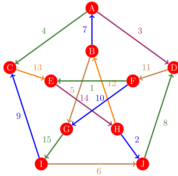
Figura 495: Flujo 487 de la gráfica de Petersen
