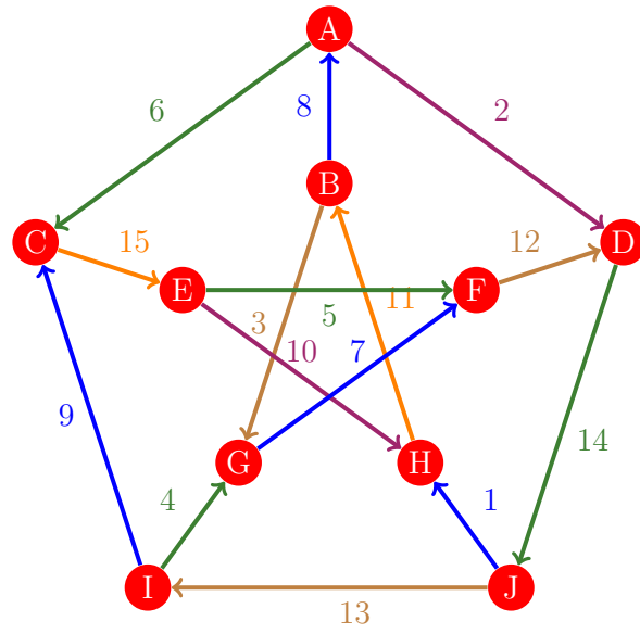
Figura 581: Flujo 573 de la gráfica de Petersen
