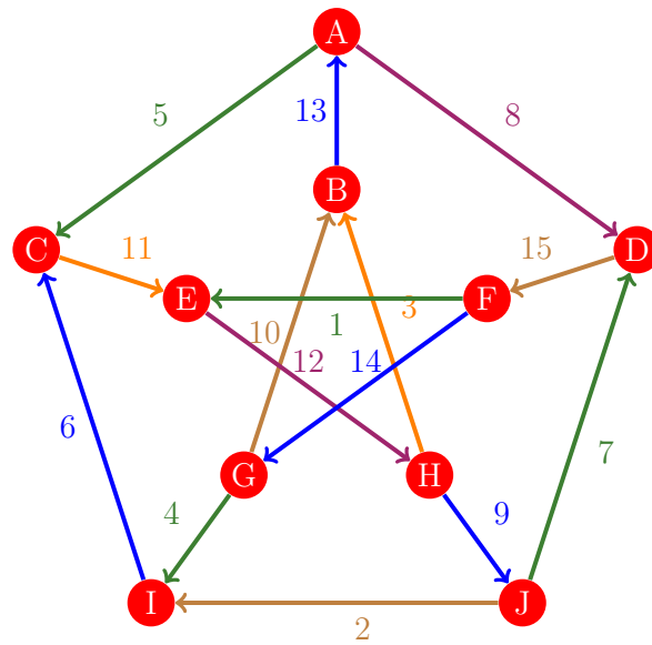
Figura 980: Flujo 972 de la gráfica de Petersen
