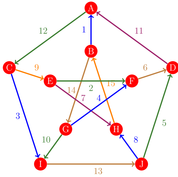
Figura 37: Flujo 29 de la gráfica de Petersen
