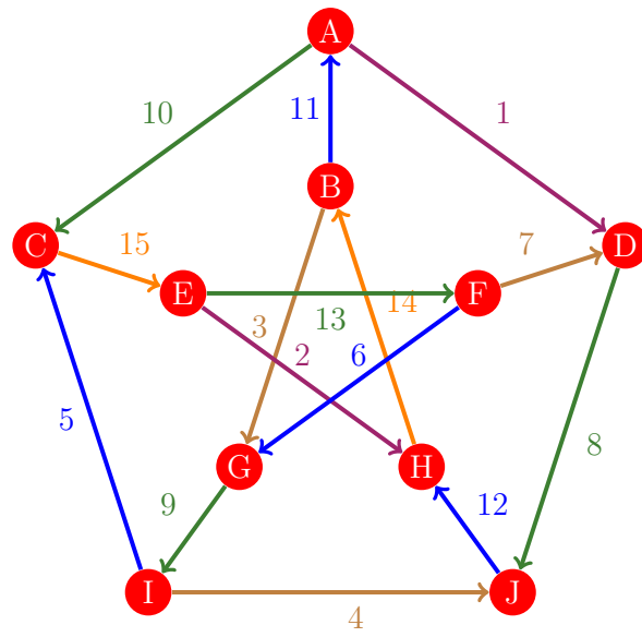
Figura 830: Flujo 822 de la gráfica de Petersen
