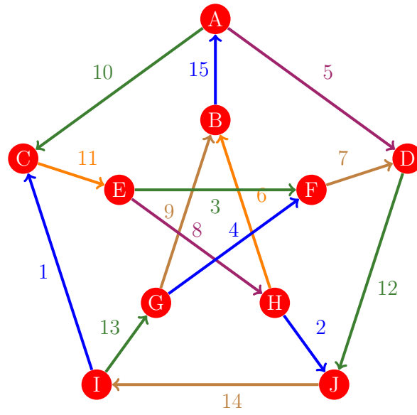
Figura 1157: Flujo 1149 de la gráfica de Petersen
