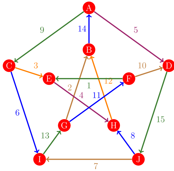
Figura 1067: Flujo 1059 de la gráfica de Petersen
