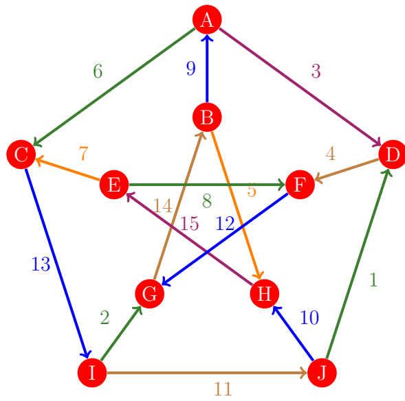
Figura 674: Flujo 666 de la gráfica de Petersen
