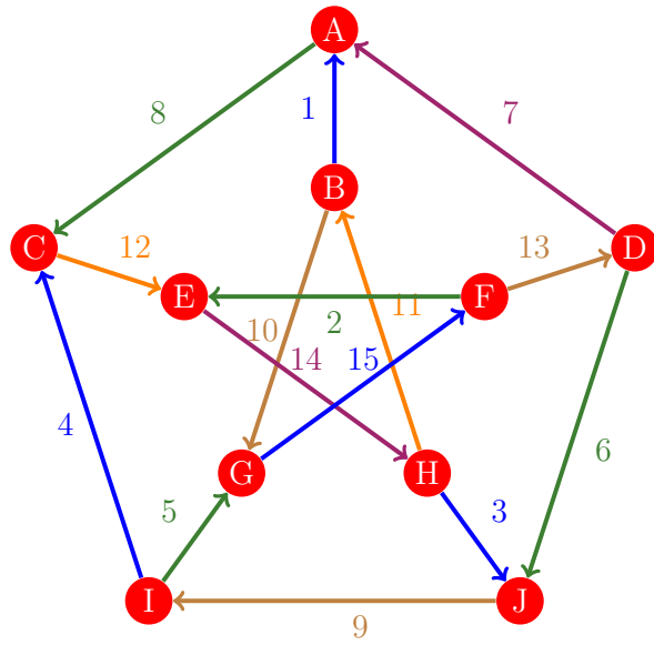
Figura 17: Flujo 9 de la gráfica de Petersen
