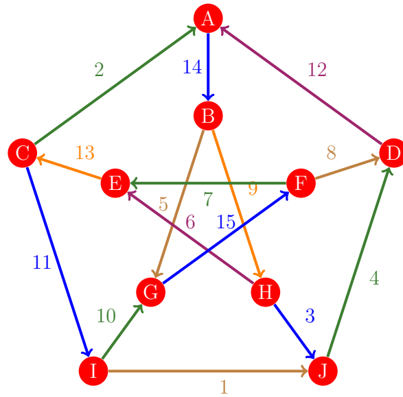
Figura 1089: Flujo 1081 de la gráfica de Petersen
