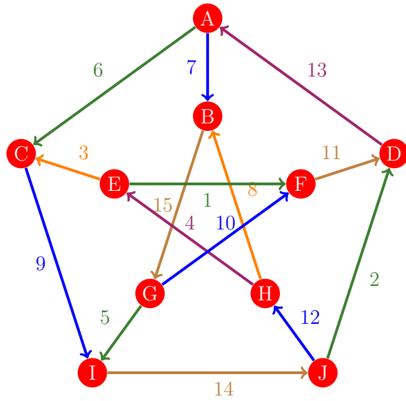
Figura 544: Flujo 536 de la gráfica de Petersen
