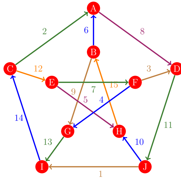
Figura 409: Flujo 401 de la gráfica de Petersen
