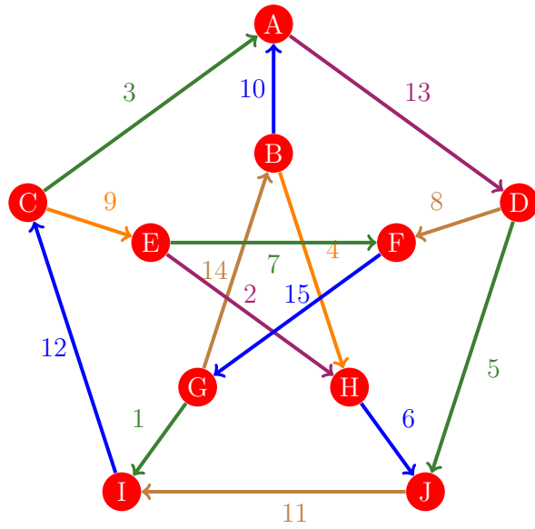
Figura 730: Flujo 722 de la gráfica de Petersen
