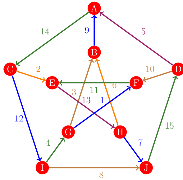
Figura 685: Flujo 677 de la gráfica de Petersen
