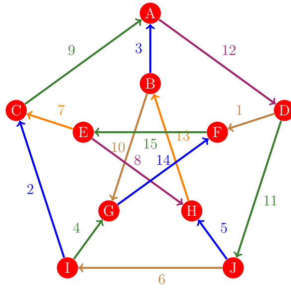
Figura 183: Flujo 175 de la gráfica de Petersen
