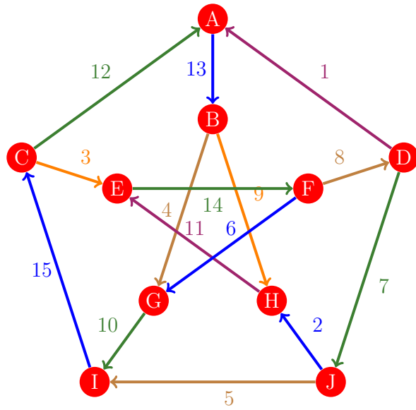
Figura 1039: Flujo 1031 de la gráfica de Petersen
