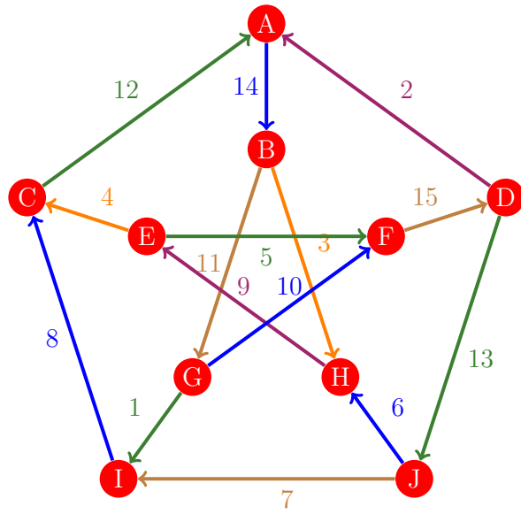
Figura 1117: Flujo 1109 de la gráfica de Petersen
