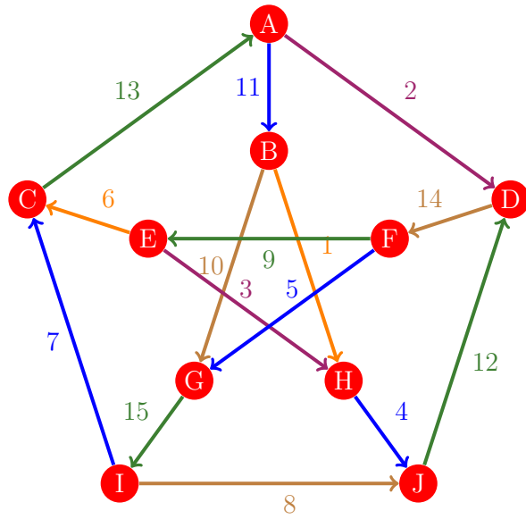
Figura 883: Flujo 875 de la gráfica de Petersen
