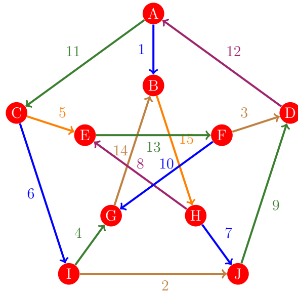
Figura 73: Flujo 65 de la gráfica de Petersen
