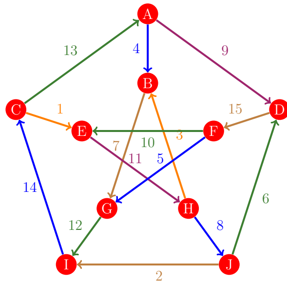
Figura 324: Flujo 316 de la gráfica de Petersen
