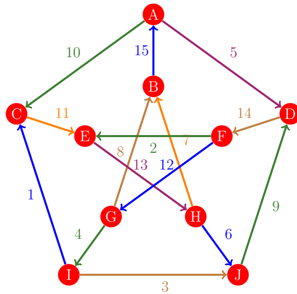
Figura 1156: Flujo 1148 de la gráfica de Petersen
