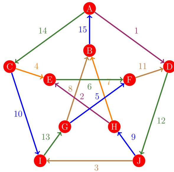
Figura 1166: Flujo 1158 de la gráfica de Petersen
