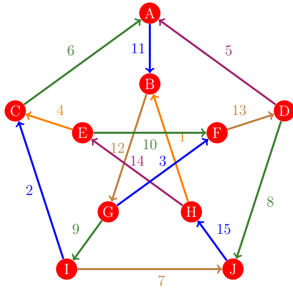
Figura 862: Flujo 854 de la gráfica de Petersen
