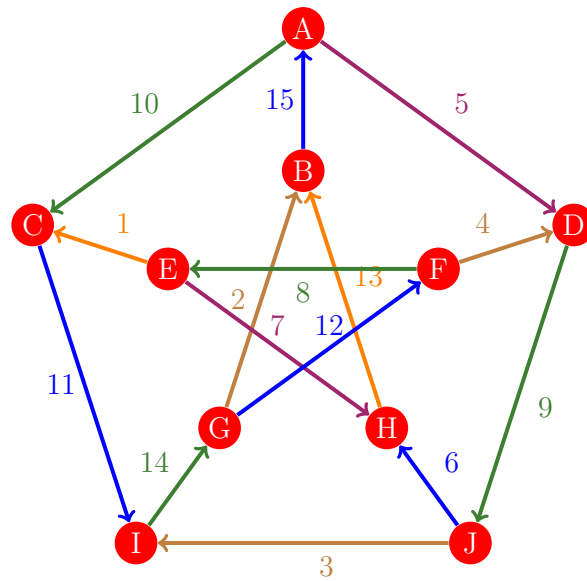
Figura 1158: Flujo 1150 de la gráfica de Petersen
