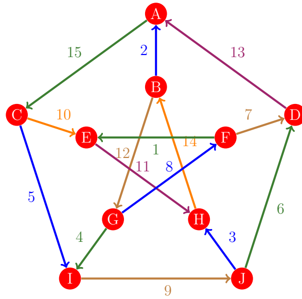
Figura 127: Flujo 119 de la gráfica de Petersen
