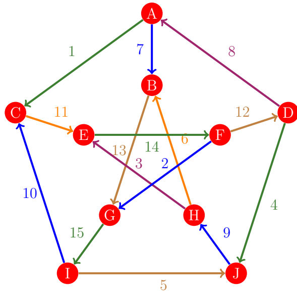
Figura 548: Flujo 540 de la gráfica de Petersen
