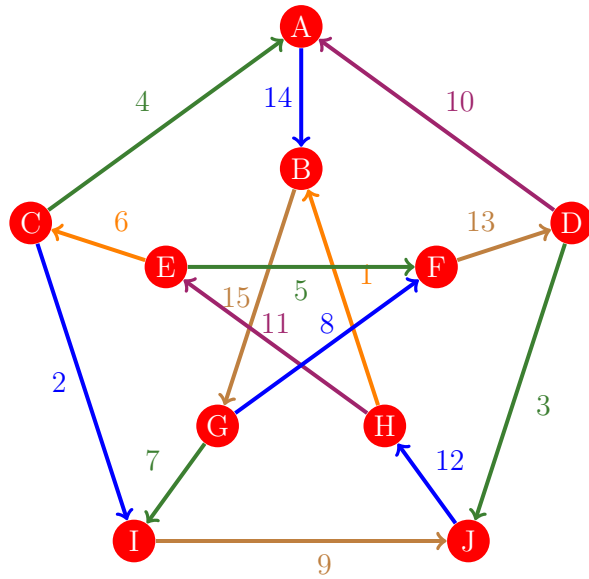
Figura 1100: Flujo 1092 de la gráfica de Petersen
