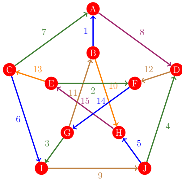
Figura 14: Flujo 6 de la gráfica de Petersen
