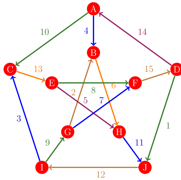
Figura 318: Flujo 310 de la gráfica de Petersen
