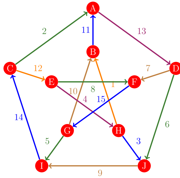
Figura 809: Flujo 801 de la gráfica de Petersen
