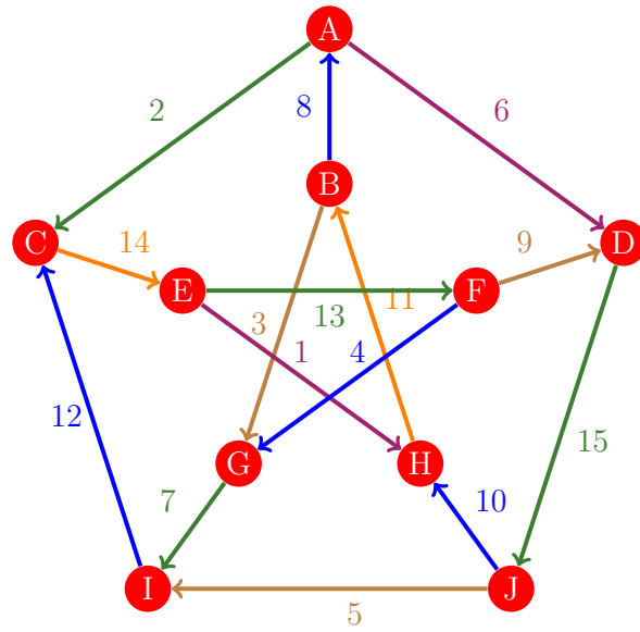
Figura 569: Flujo 561 de la gráfica de Petersen
