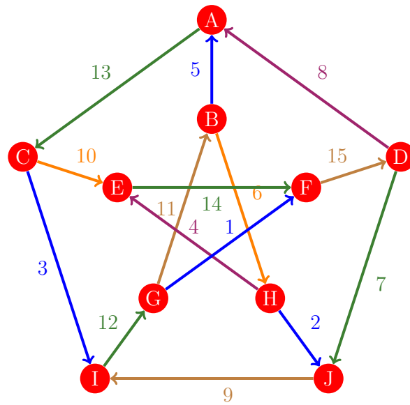
Figura 358: Flujo 350 de la gráfica de Petersen
