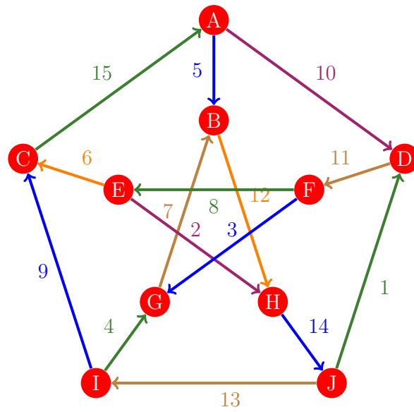
Figura 402: Flujo 394 de la gráfica de Petersen
