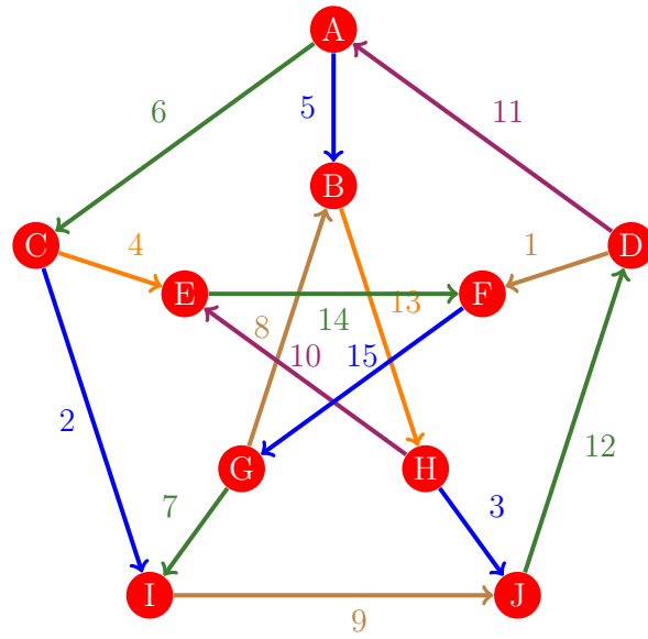
Figura 373: Flujo 365 de la gráfica de Petersen
