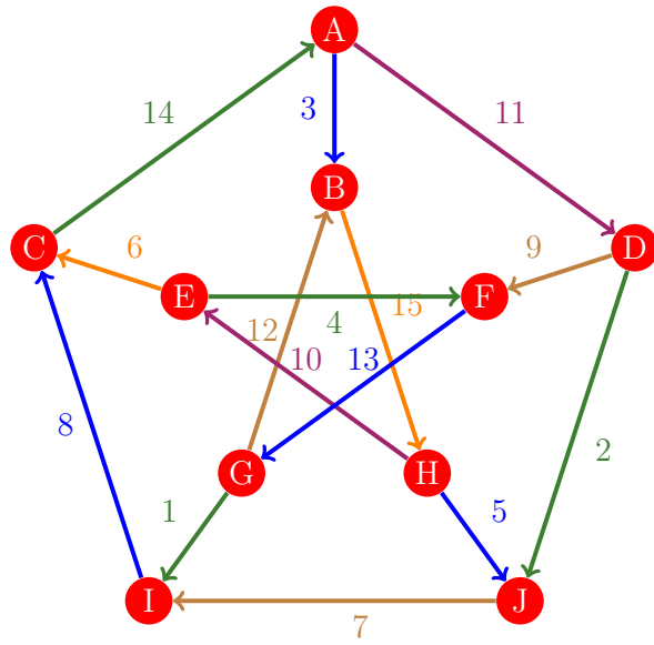
Figura 245: Flujo 237 de la gráfica de Petersen
