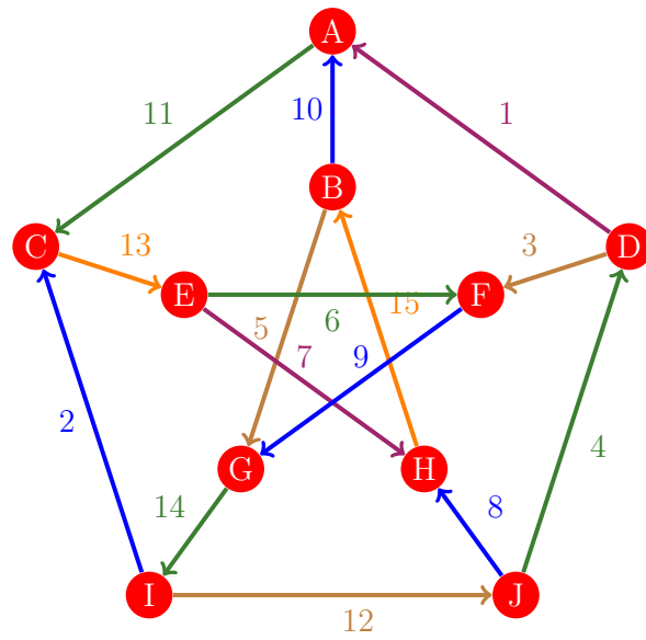
Figura 752: Flujo 744 de la gráfica de Petersen
