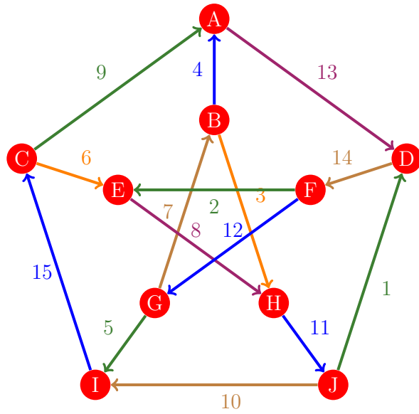
Figura 270: Flujo 262 de la gráfica de Petersen
