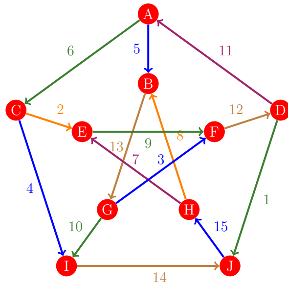
Figura 374: Flujo 366 de la gráfica de Petersen
