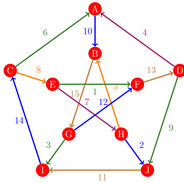
Figura 784: Flujo 776 de la gráfica de Petersen
