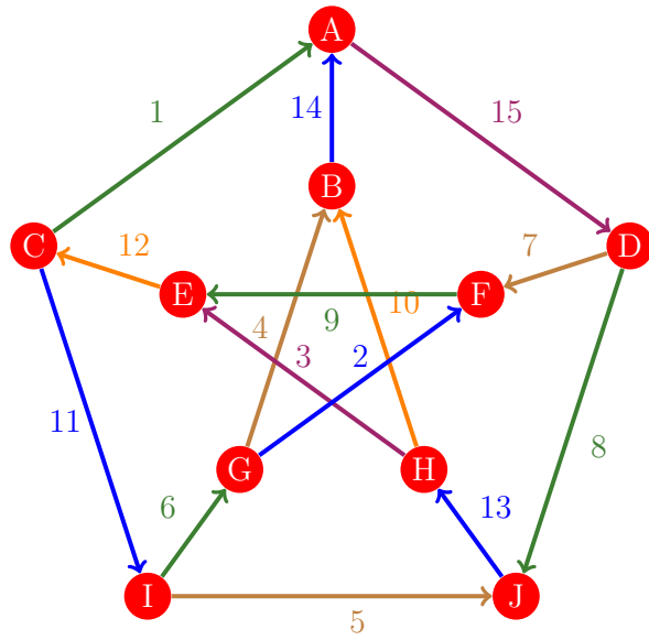
Figura 1083: Flujo 1075 de la gráfica de Petersen
