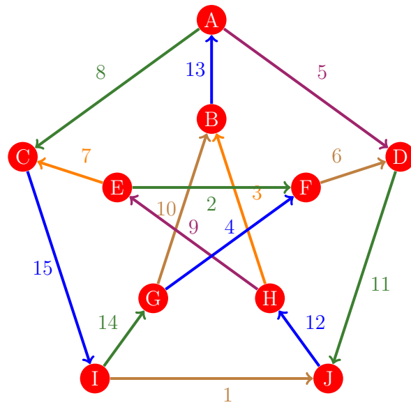
Figura 990: Flujo 982 de la gráfica de Petersen
