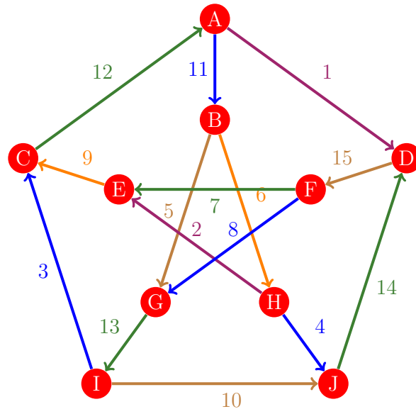
Figura 881: Flujo 873 de la gráfica de Petersen
