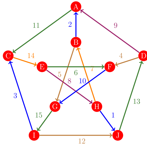
Figura 109: Flujo 101 de la gráfica de Petersen
