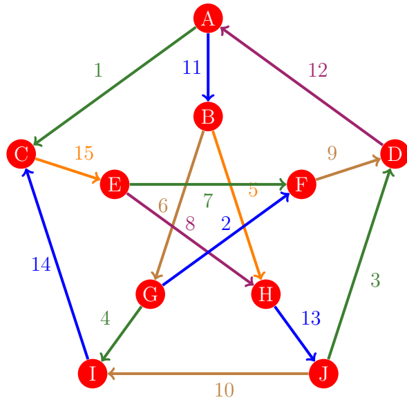
Figura 880: Flujo 872 de la gráfica de Petersen
