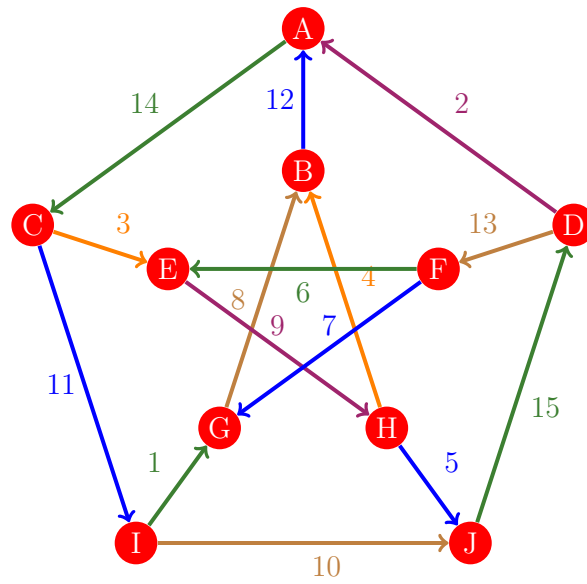
Figura 926: Flujo 918 de la gráfica de Petersen
