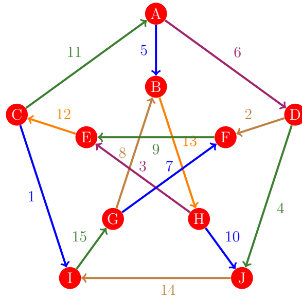
Figura 393: Flujo 385 de la gráfica de Petersen
