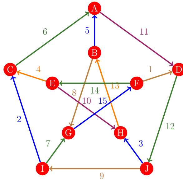
Figura 333: Flujo 325 de la gráfica de Petersen
