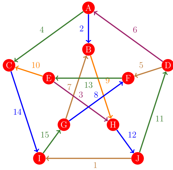
Figura 129: Flujo 121 de la gráfica de Petersen
