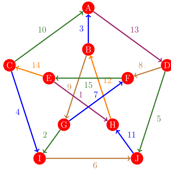
Figura 189: Flujo 181 de la gráfica de Petersen
