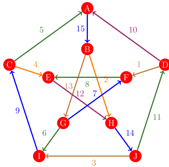
Figura 1180: Flujo 1172 de la gráfica de Petersen
