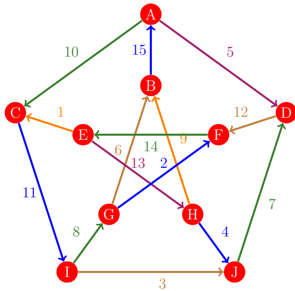
Figura 1154: Flujo 1146 de la gráfica de Petersen
