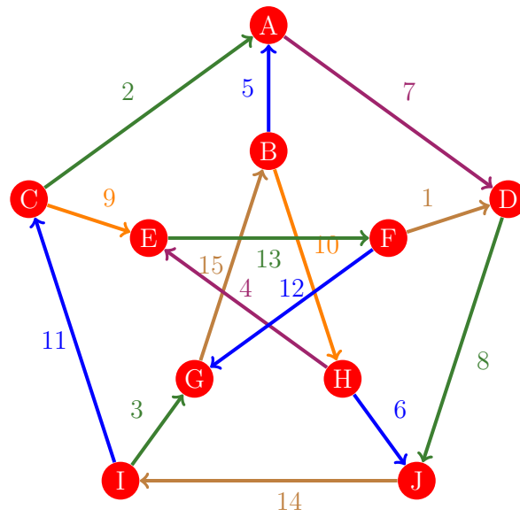
Figura 330: Flujo 322 de la gráfica de Petersen
