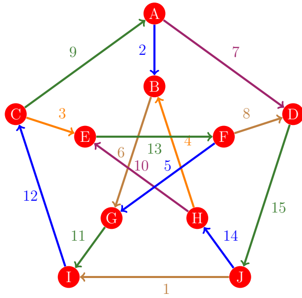
Figura 144: Flujo 136 de la gráfica de Petersen
