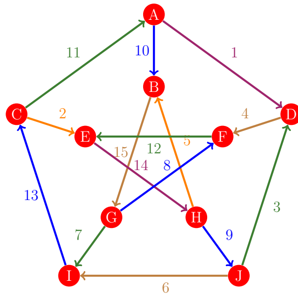
Figura 796: Flujo 788 de la gráfica de Petersen
