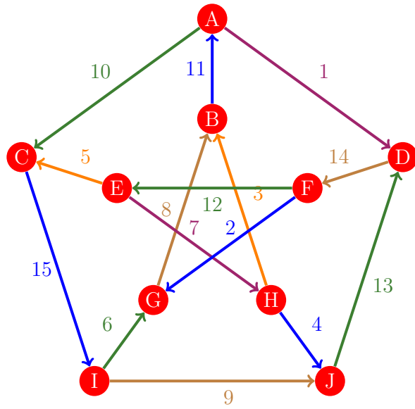
Figura 827: Flujo 819 de la gráfica de Petersen
