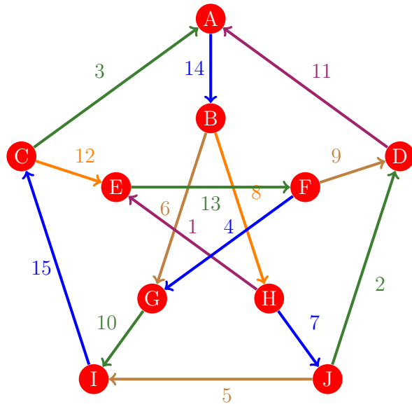
Figura 1095: Flujo 1087 de la gráfica de Petersen
