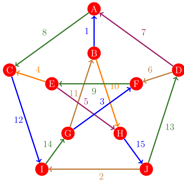
Figura 18: Flujo 10 de la gráfica de Petersen
