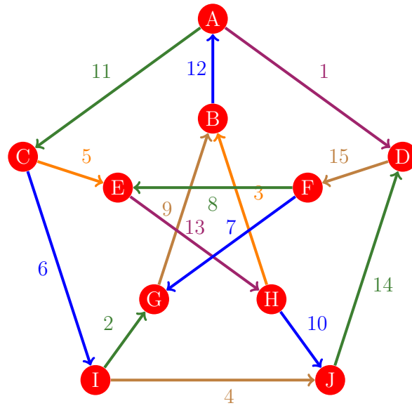
Figura 913: Flujo 905 de la gráfica de Petersen
