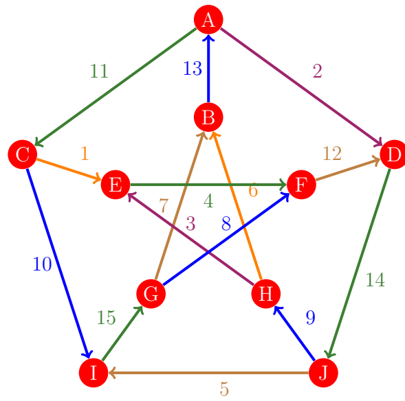
Figura 998: Flujo 990 de la gráfica de Petersen
