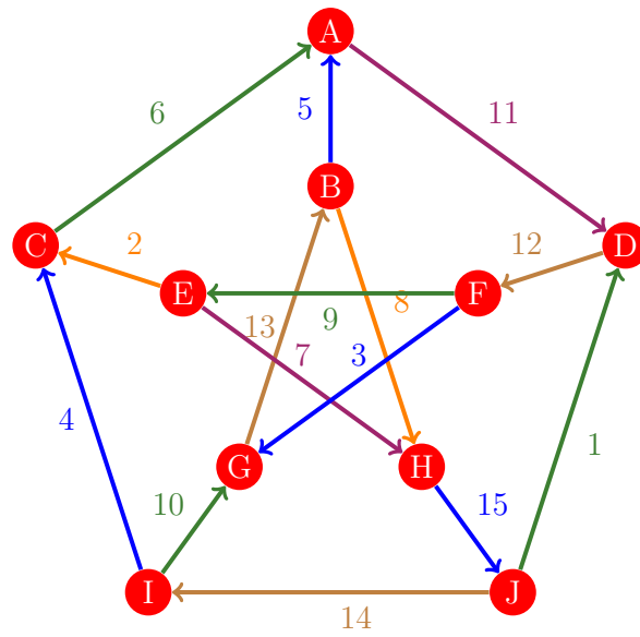
Figura 334: Flujo 326 de la gráfica de Petersen
