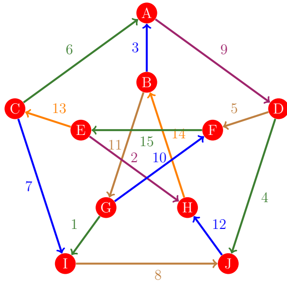
Figura 177: Flujo 169 de la gráfica de Petersen
