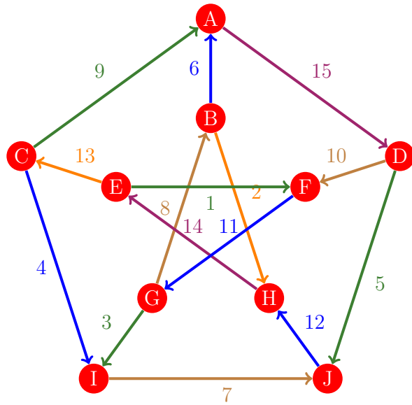
Figura 431: Flujo 423 de la gráfica de Petersen
