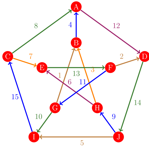
Figura 265: Flujo 257 de la gráfica de Petersen
