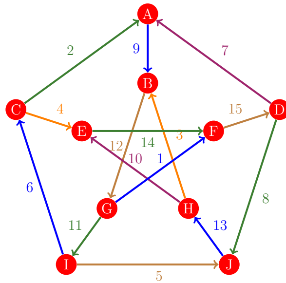
Figura 690: Flujo 682 de la gráfica de Petersen
