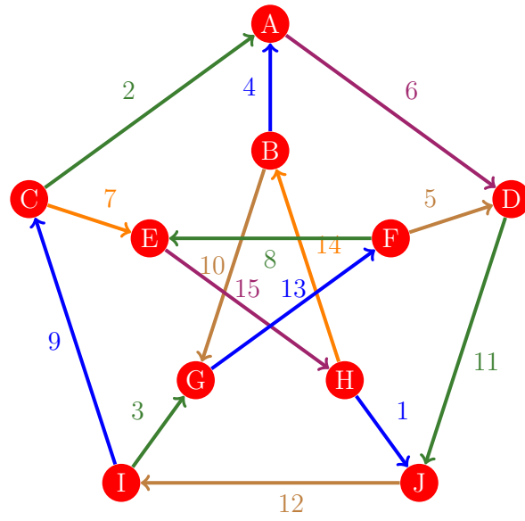
Figura 249: Flujo 241 de la gráfica de Petersen
