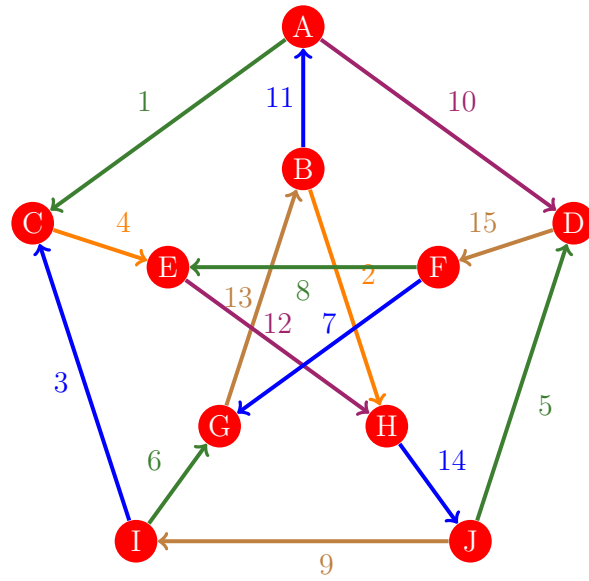
Figura 839: Flujo 831 de la gráfica de Petersen
