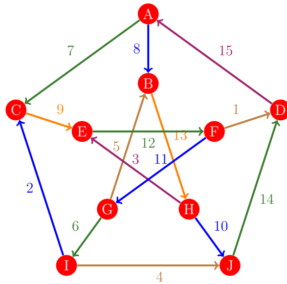
Figura 628: Flujo 620 de la gráfica de Petersen
