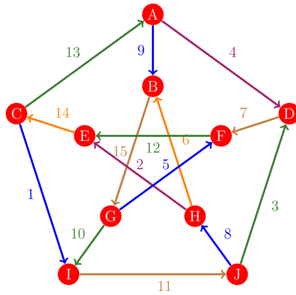
Figura 724: Flujo 716 de la gráfica de Petersen
