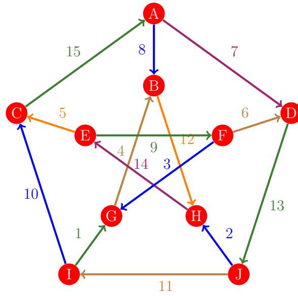
Figura 645: Flujo 637 de la gráfica de Petersen
