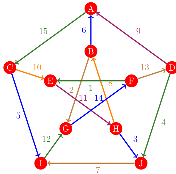
Figura 448: Flujo 440 de la gráfica de Petersen
