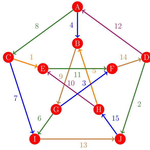
Figura 307: Flujo 299 de la gráfica de Petersen
