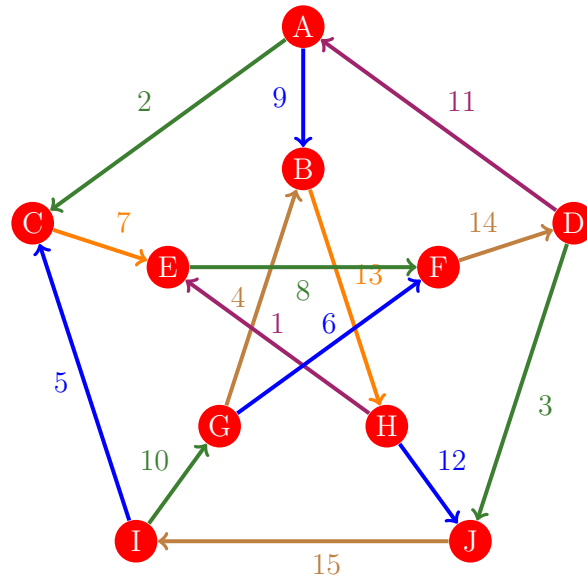
Figura 691: Flujo 683 de la gráfica de Petersen
