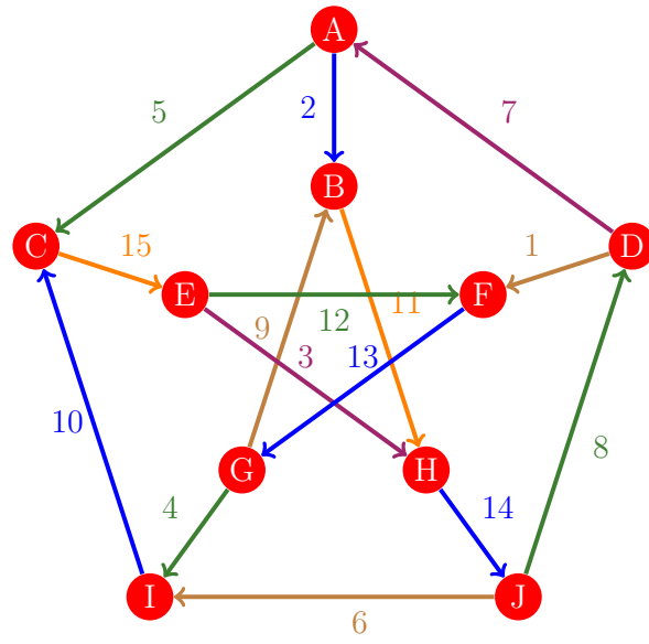
Figura 131: Flujo 123 de la gráfica de Petersen
