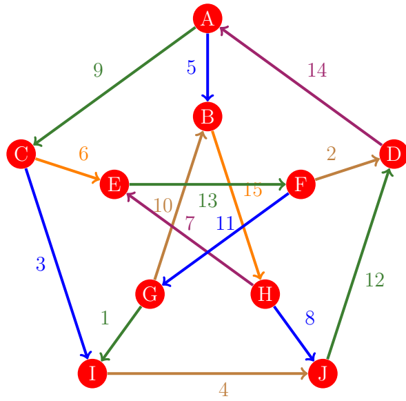
Figura 383: Flujo 375 de la gráfica de Petersen
