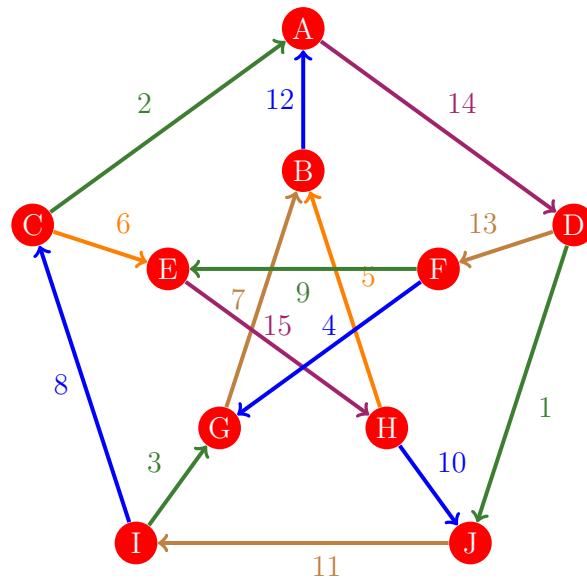
Figura 892: Flujo 884 de la gráfica de Petersen
