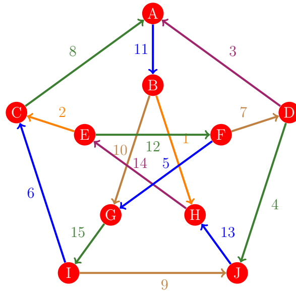
Figura 863: Flujo 855 de la gráfica de Petersen
