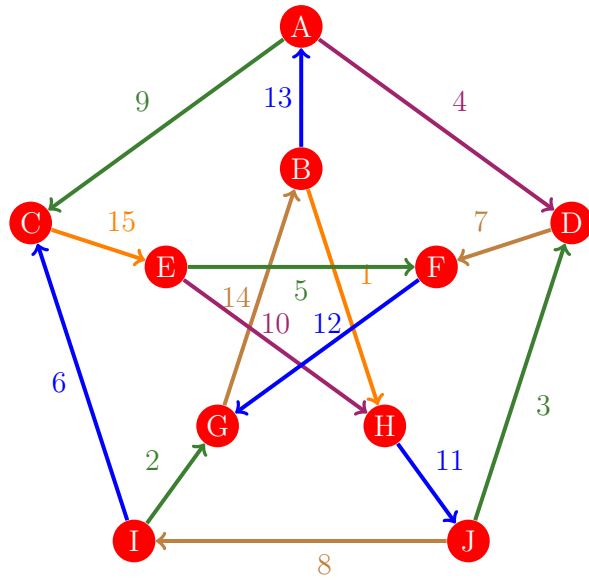
Figura 994: Flujo 986 de la gráfica de Petersen
