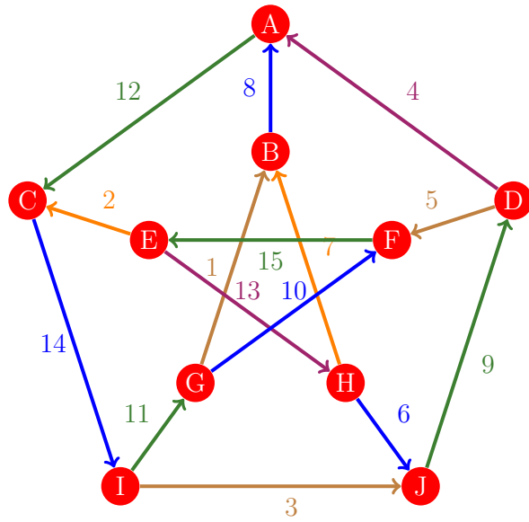
Figura 599: Flujo 591 de la gráfica de Petersen
