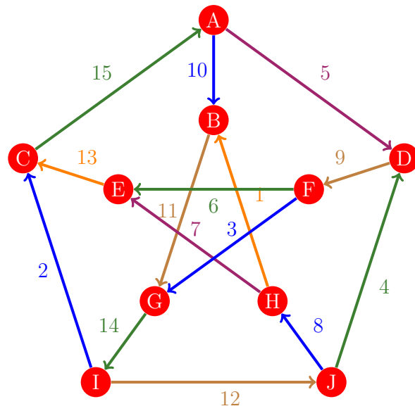
Figura 808: Flujo 800 de la gráfica de Petersen
