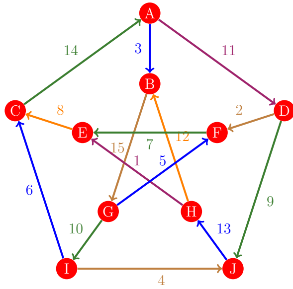
Figura 246: Flujo 238 de la gráfica de Petersen
