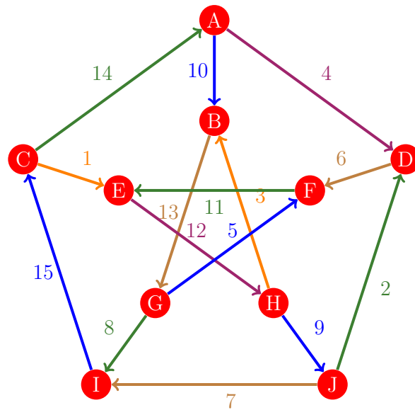
Figura 800: Flujo 792 de la gráfica de Petersen
