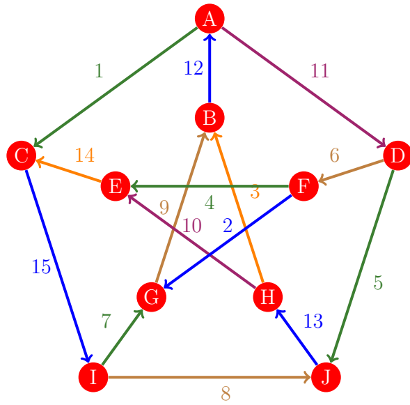
Figura 917: Flujo 909 de la gráfica de Petersen
