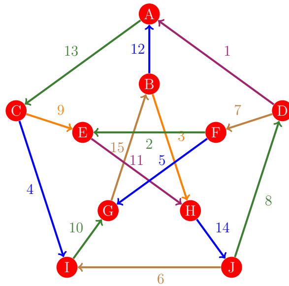
Figura 920: Flujo 912 de la gráfica de Petersen
