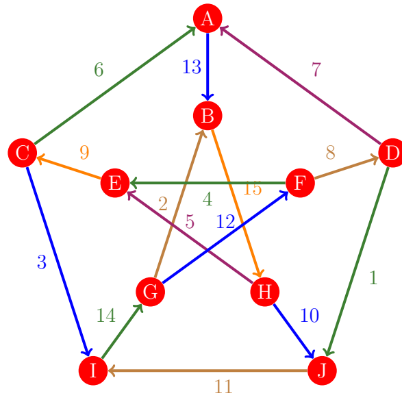
Figura 1021: Flujo 1013 de la gráfica de Petersen
