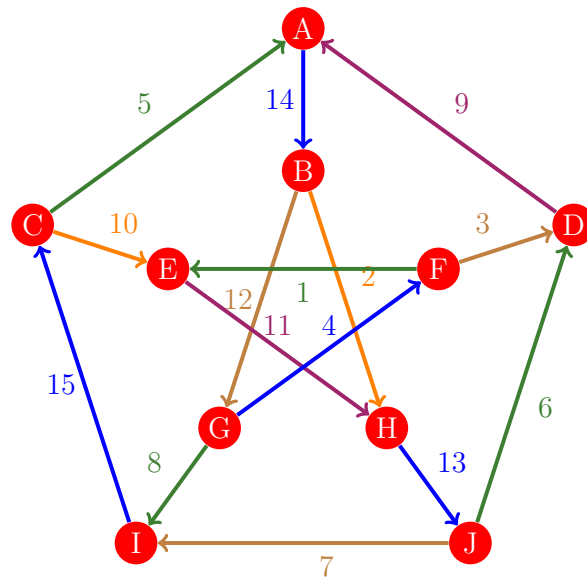
Figura 1102: Flujo 1094 de la gráfica de Petersen
