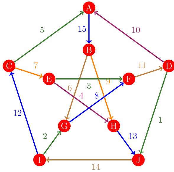
Figura 1174: Flujo 1166 de la gráfica de Petersen
