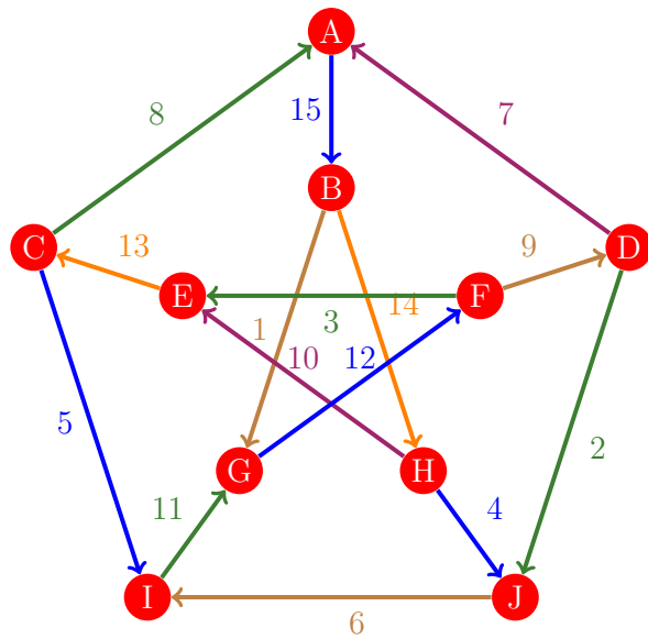
Figura 1190: Flujo 1182 de la gráfica de Petersen
