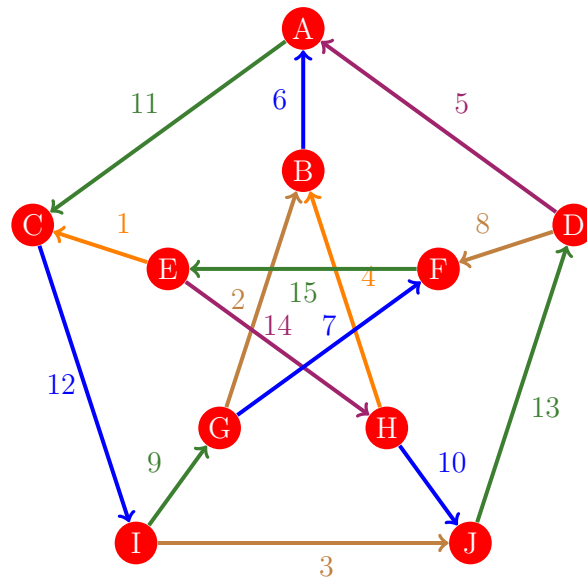
Figura 440: Flujo 432 de la gráfica de Petersen
