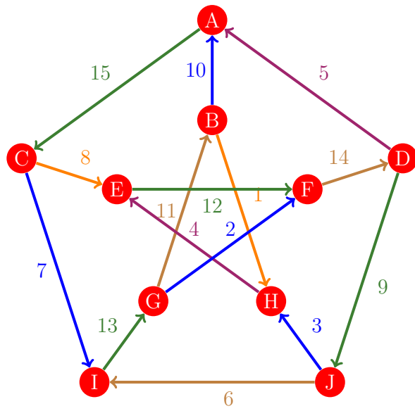
Figura 766: Flujo 758 de la gráfica de Petersen
