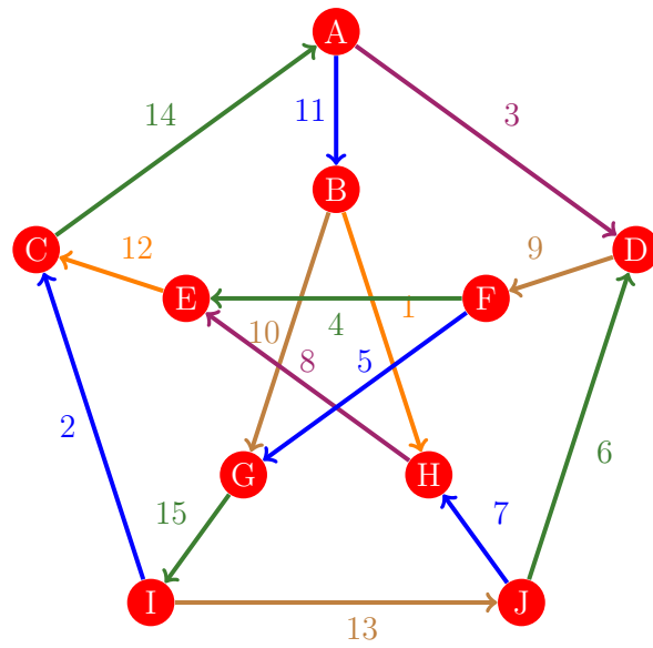
Figura 886: Flujo 878 de la gráfica de Petersen
