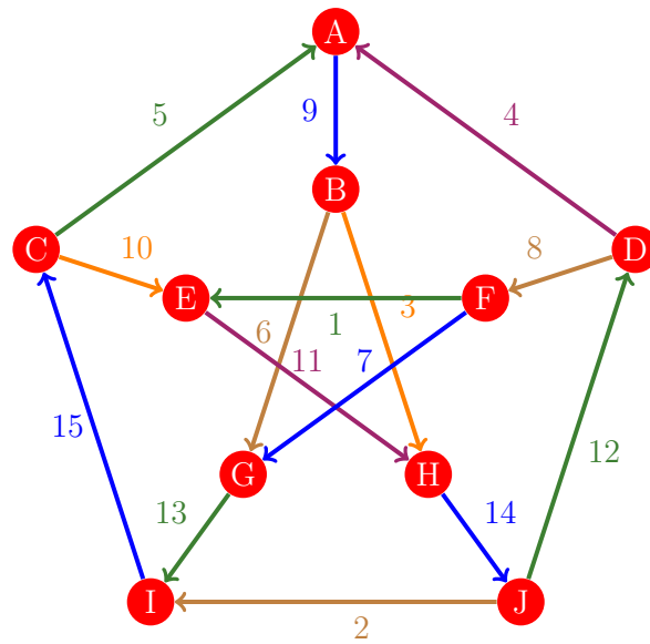
Figura 706: Flujo 698 de la gráfica de Petersen
