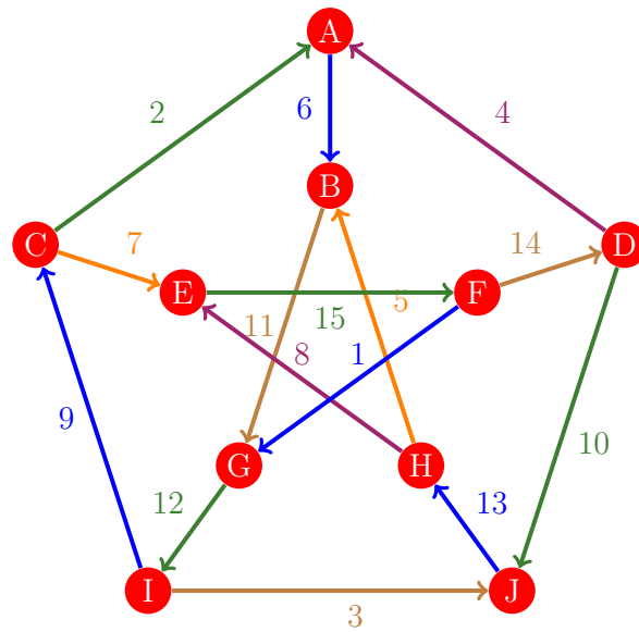
Figura 450: Flujo 442 de la gráfica de Petersen
