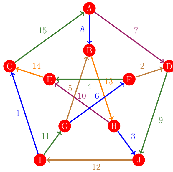
Figura 646: Flujo 638 de la gráfica de Petersen
