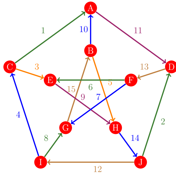
Figura 749: Flujo 741 de la gráfica de Petersen
