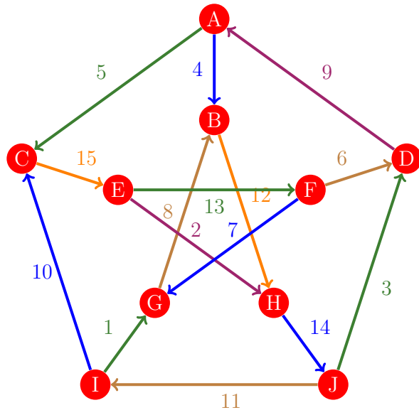
Figura 297: Flujo 289 de la gráfica de Petersen
