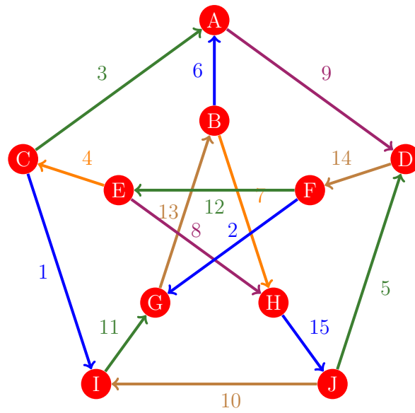
Figura 416: Flujo 408 de la gráfica de Petersen
