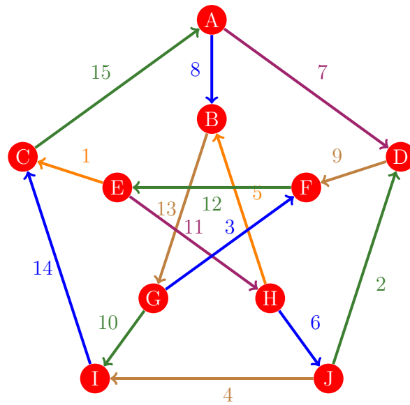
Figura 648: Flujo 640 de la gráfica de Petersen
