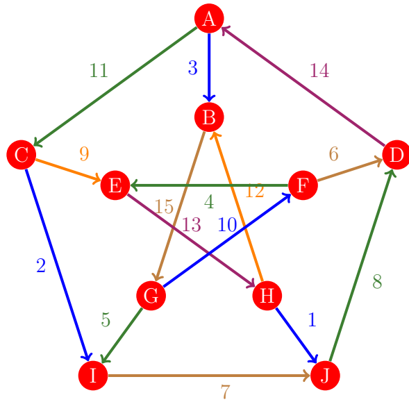
Figura 236: Flujo 228 de la gráfica de Petersen
