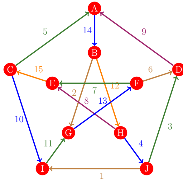
Figura 1101: Flujo 1093 de la gráfica de Petersen
