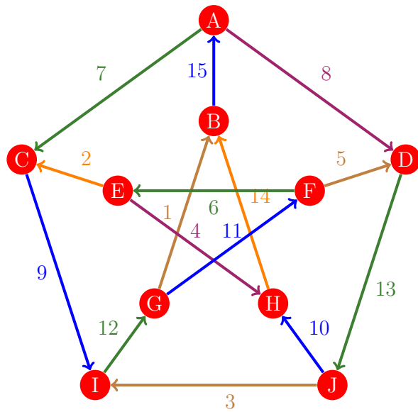
Figura 1146: Flujo 1138 de la gráfica de Petersen
