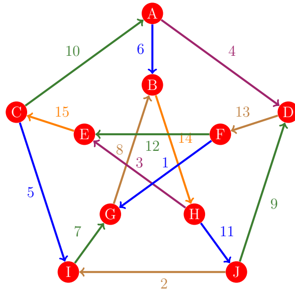
Figura 477: Flujo 469 de la gráfica de Petersen
