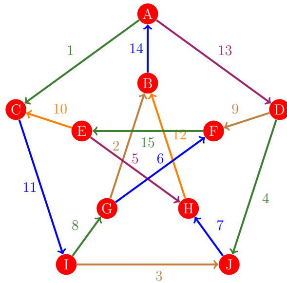
Figura 1086: Flujo 1078 de la gráfica de Petersen
