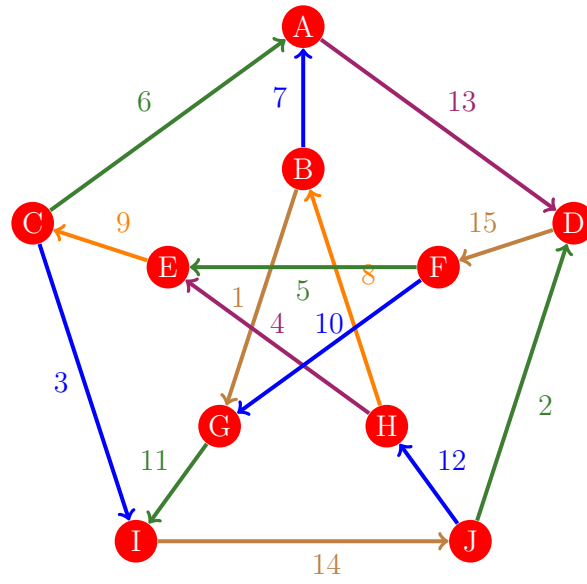
Figura 501: Flujo 493 de la gráfica de Petersen
