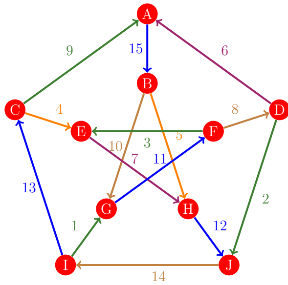
Figura 1192: Flujo 1184 de la gráfica de Petersen
