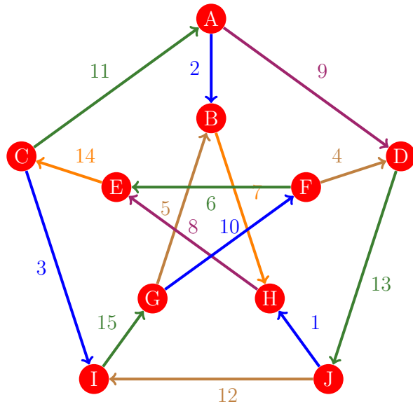
Figura 147: Flujo 139 de la gráfica de Petersen
