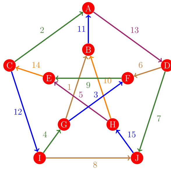
Figura 810: Flujo 802 de la gráfica de Petersen
