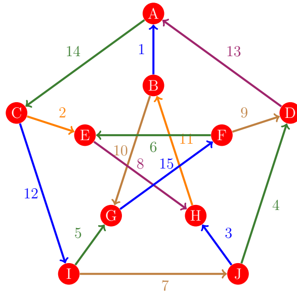
Figura 45: Flujo 37 de la gráfica de Petersen
