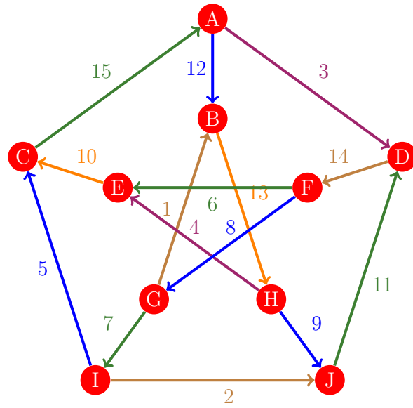
Figura 967: Flujo 959 de la gráfica de Petersen
