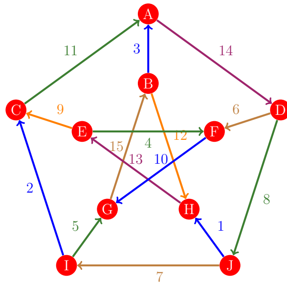
Figura 194: Flujo 186 de la gráfica de Petersen
