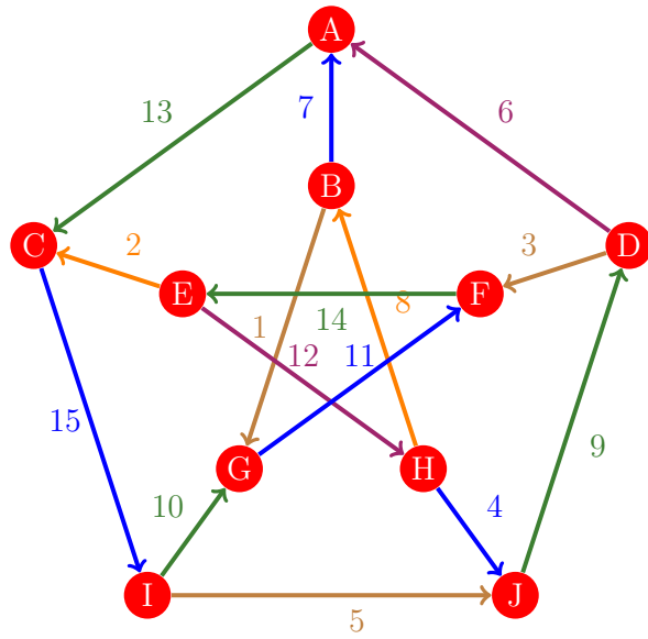
Figura 521: Flujo 513 de la gráfica de Petersen
