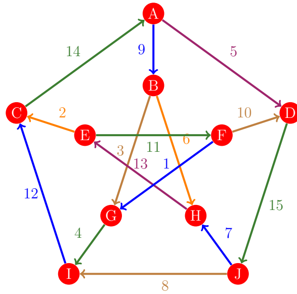
Figura 725: Flujo 717 de la gráfica de Petersen
