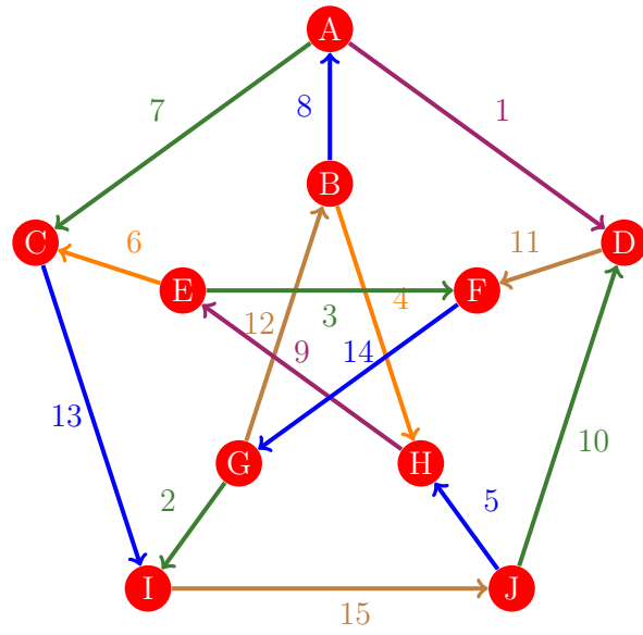
Figura 589: Flujo 581 de la gráfica de Petersen
