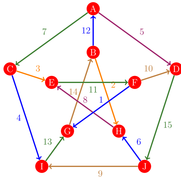
Figura 906: Flujo 898 de la gráfica de Petersen
