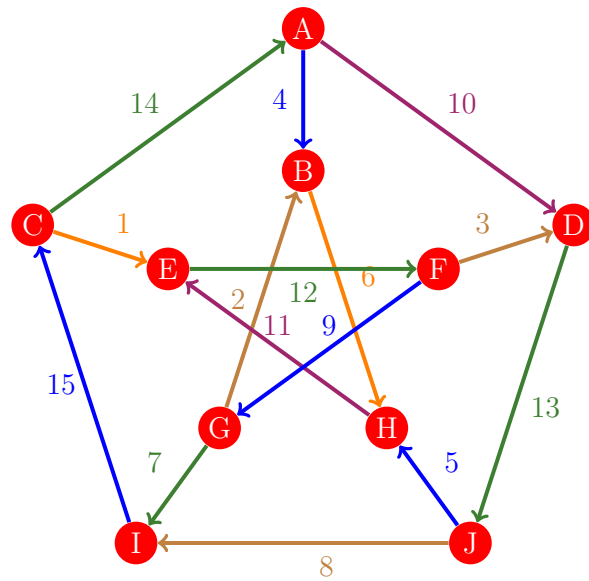
Figura 328: Flujo 320 de la gráfica de Petersen
