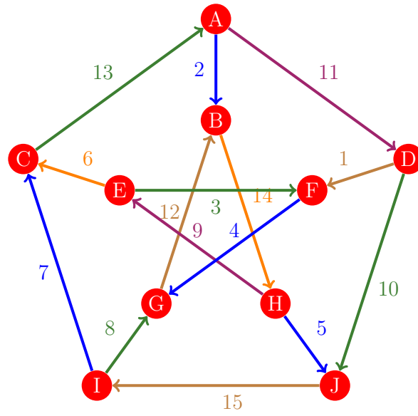
Figura 157: Flujo 149 de la gráfica de Petersen
