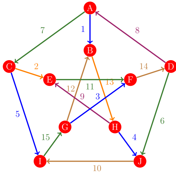
Figura 55: Flujo 47 de la gráfica de Petersen
