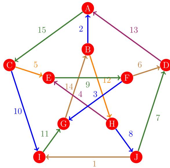
Figura 128: Flujo 120 de la gráfica de Petersen
