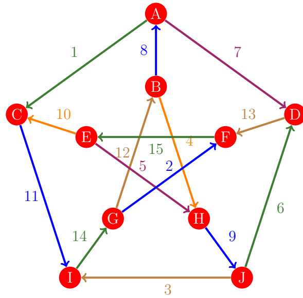
Figura 593: Flujo 585 de la gráfica de Petersen
