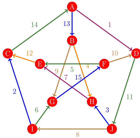
Figura 1046: Flujo 1038 de la gráfica de Petersen
