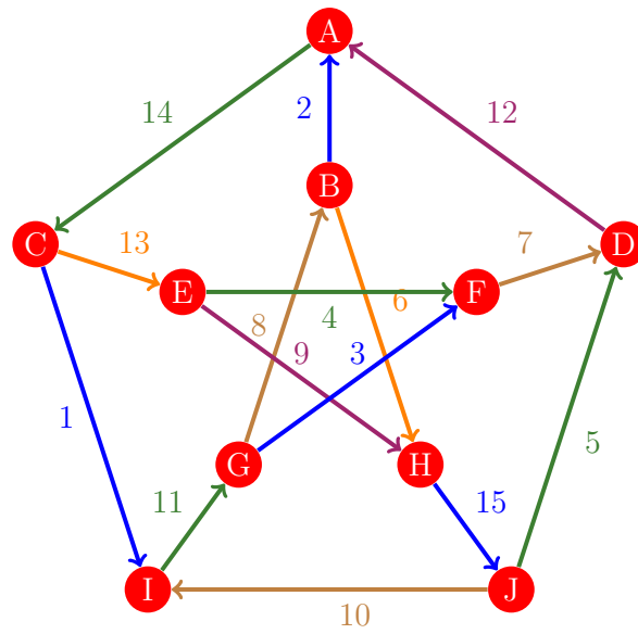
Figura 122: Flujo 114 de la gráfica de Petersen
