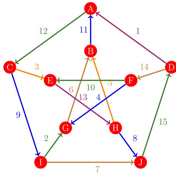
Figura 842: Flujo 834 de la gráfica de Petersen
