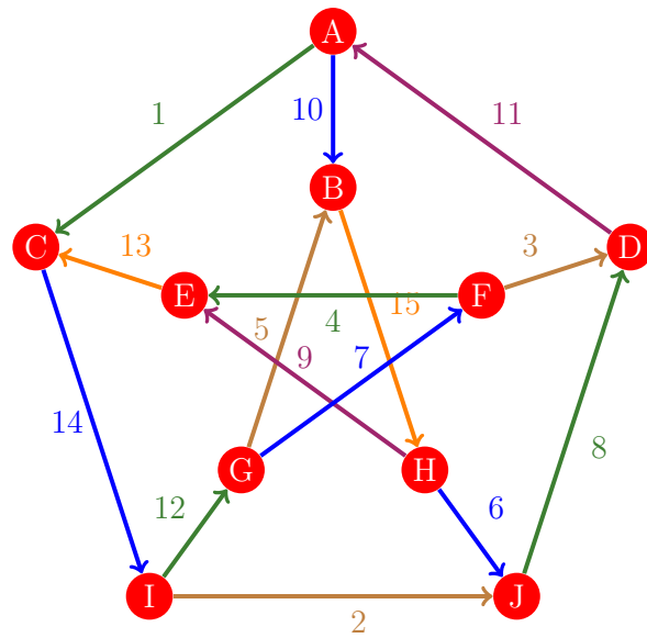
Figura 786: Flujo 778 de la gráfica de Petersen
