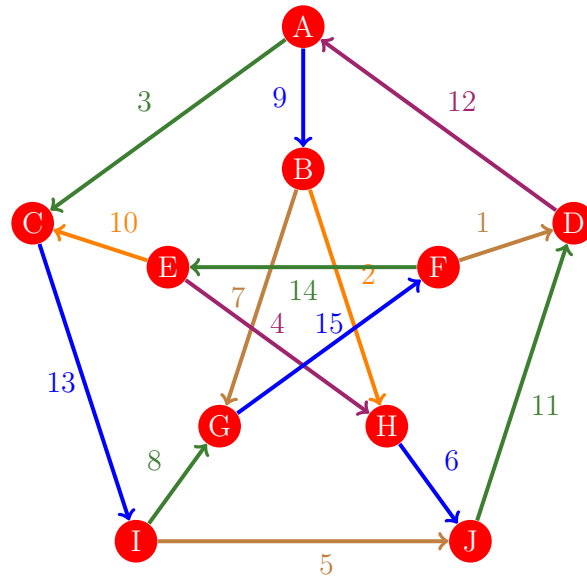
Figura 697: Flujo 689 de la gráfica de Petersen
