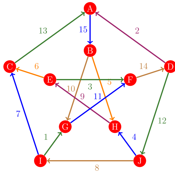
Figura 1204: Flujo 1196 de la gráfica de Petersen
