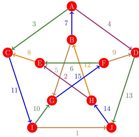
Figura 493: Flujo 485 de la gráfica de Petersen
