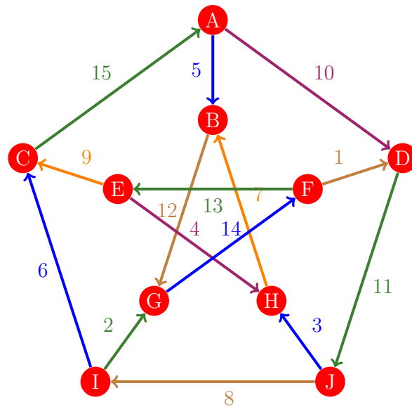
Figura 406: Flujo 398 de la gráfica de Petersen
