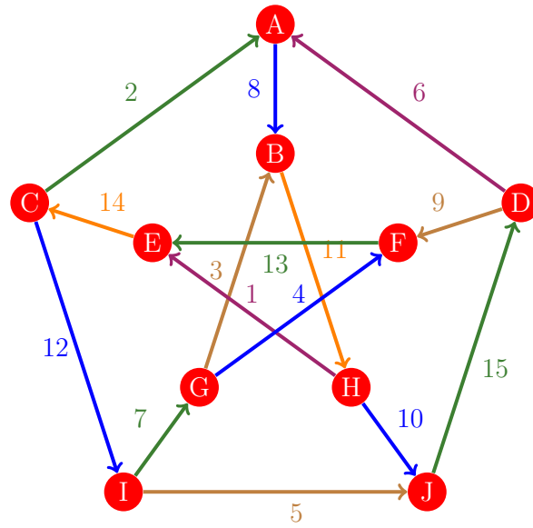
Figura 609: Flujo 601 de la gráfica de Petersen
