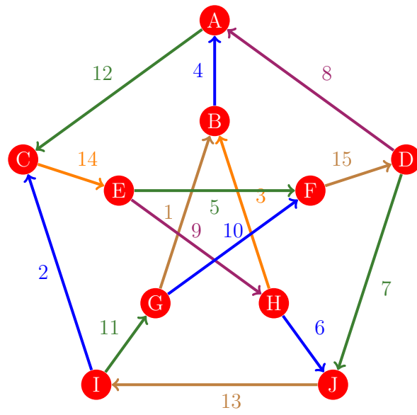
Figura 279: Flujo 271 de la gráfica de Petersen
