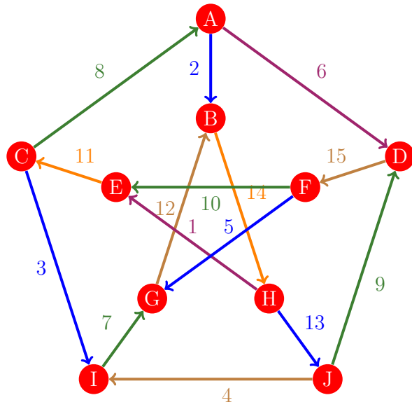
Figura 141: Flujo 133 de la gráfica de Petersen
