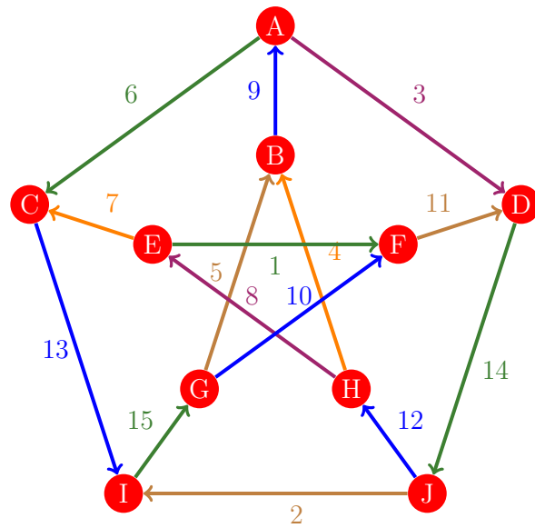
Figura 672: Flujo 664 de la gráfica de Petersen
