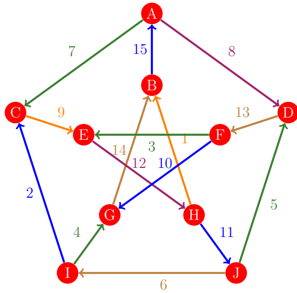
Figura 1145: Flujo 1137 de la gráfica de Petersen
