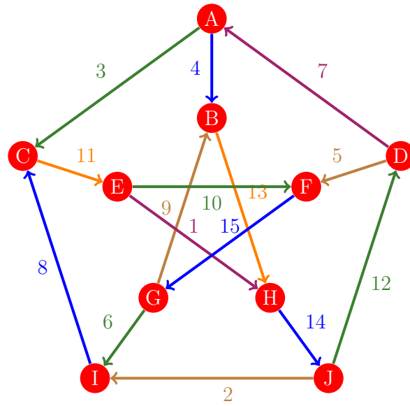
Figura 293: Flujo 285 de la gráfica de Petersen
