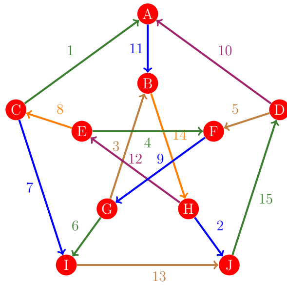
Figura 874: Flujo 866 de la gráfica de Petersen
