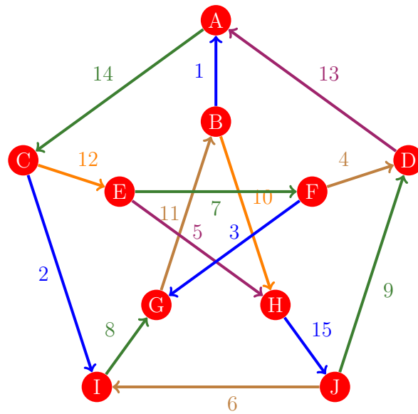
Figura 46: Flujo 38 de la gráfica de Petersen
