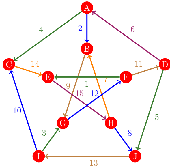
Figura 130: Flujo 122 de la gráfica de Petersen
