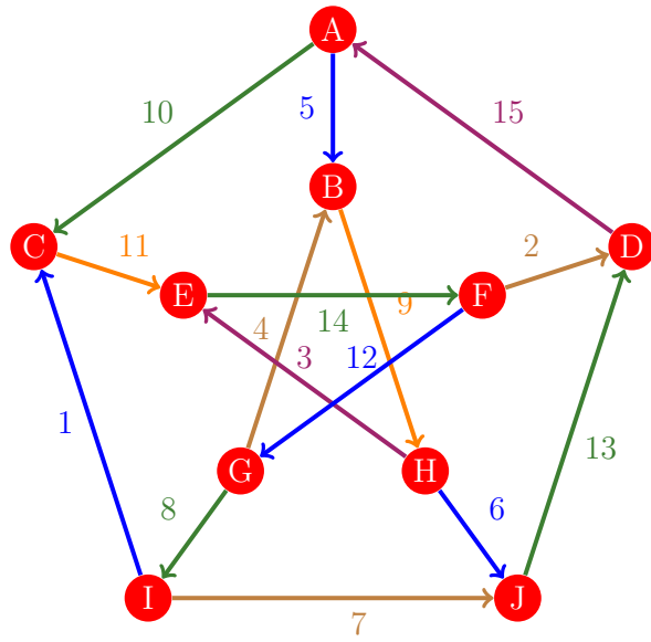
Figura 385: Flujo 377 de la gráfica de Petersen
