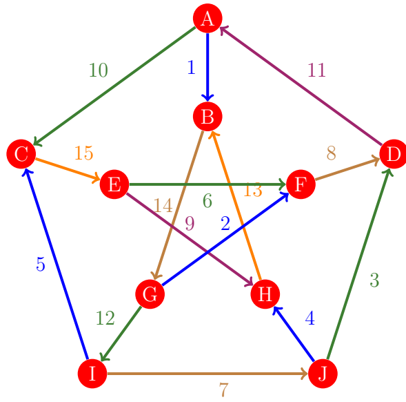
Figura 66: Flujo 58 de la gráfica de Petersen
