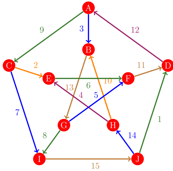
Figura 228: Flujo 220 de la gráfica de Petersen
