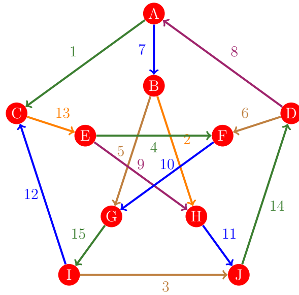
Figura 545: Flujo 537 de la gráfica de Petersen
