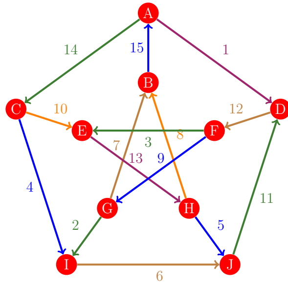
Figura 1165: Flujo 1157 de la gráfica de Petersen
