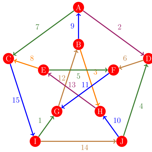
Figura 676: Flujo 668 de la gráfica de Petersen
