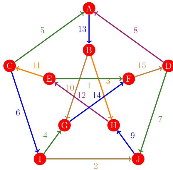
Figura 1020: Flujo 1012 de la gráfica de Petersen
