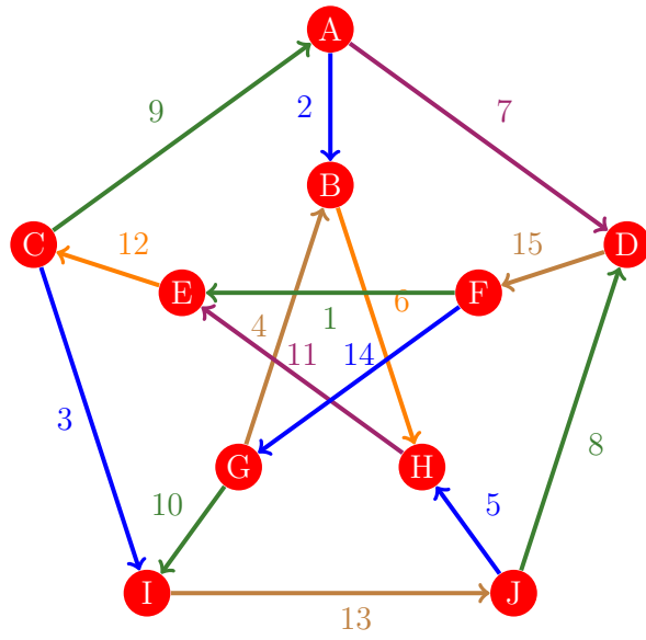
Figura 143: Flujo 135 de la gráfica de Petersen
