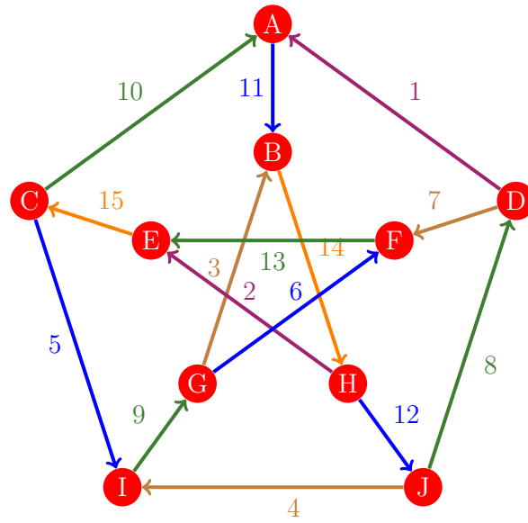
Figura 869: Flujo 861 de la gráfica de Petersen
