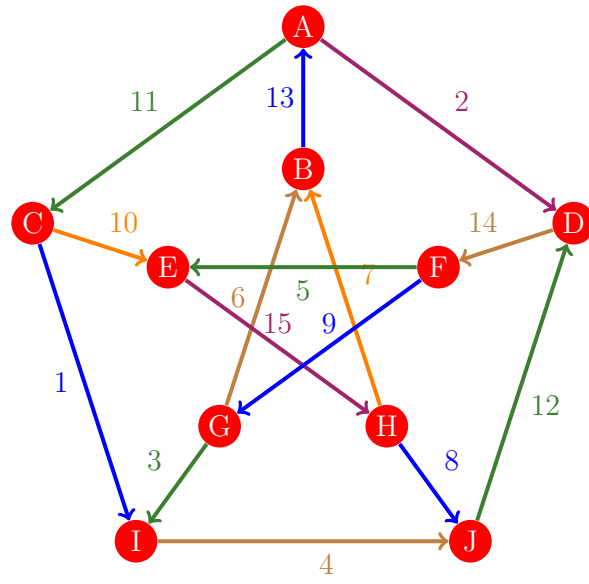
Figura 997: Flujo 989 de la gráfica de Petersen
