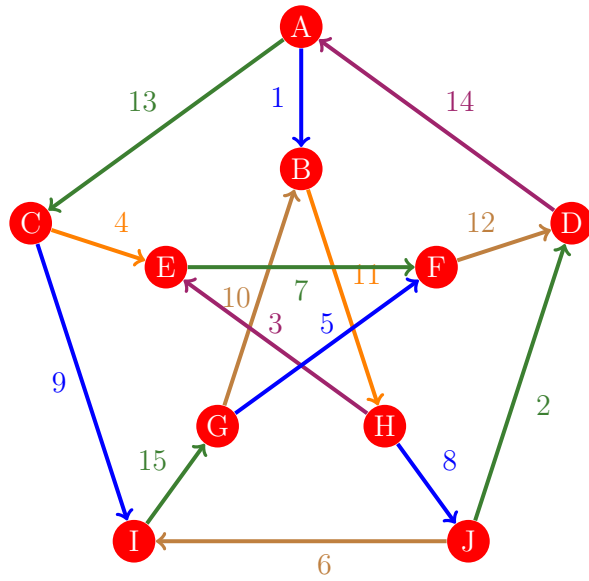
Figura 81: Flujo 73 de la gráfica de Petersen
