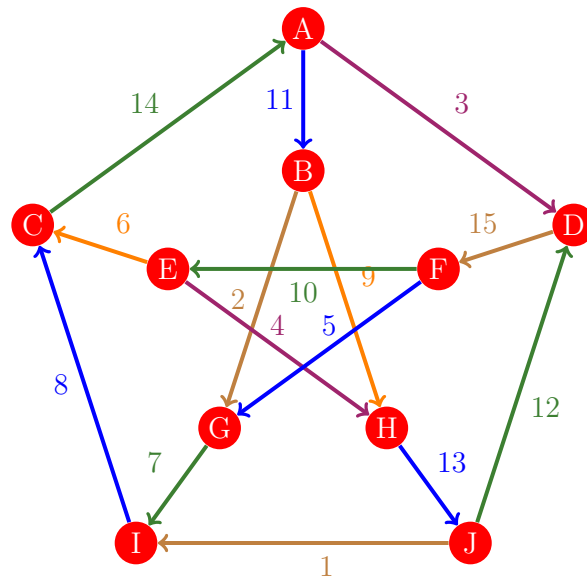
Figura 888: Flujo 880 de la gráfica de Petersen
