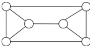
Figura 1: Gráfica 3-regular.
