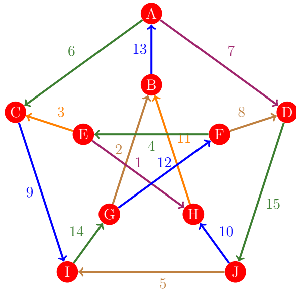
Figura 981: Flujo 973 de la gráfica de Petersen
