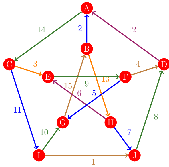
Figura 126: Flujo 118 de la gráfica de Petersen
