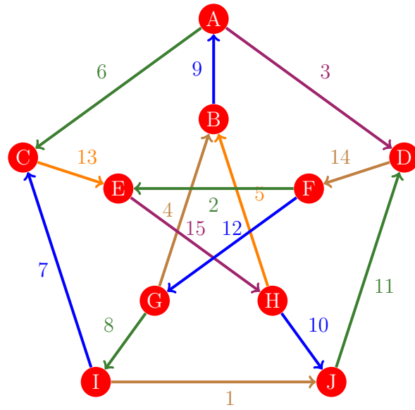
Figura 671: Flujo 663 de la gráfica de Petersen
