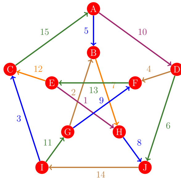
Figura 408: Flujo 400 de la gráfica de Petersen
