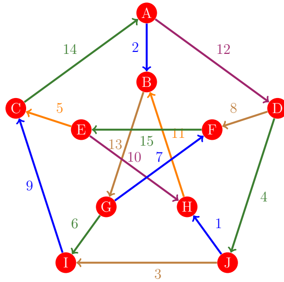
Figura 165: Flujo 157 de la gráfica de Petersen
