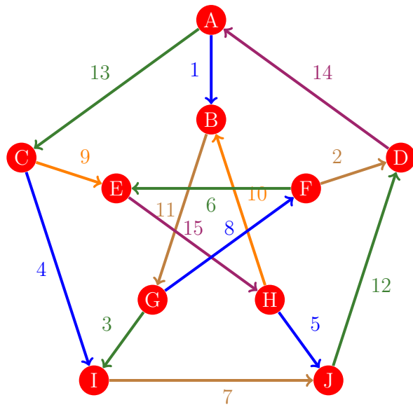
Figura 82: Flujo 74 de la gráfica de Petersen
