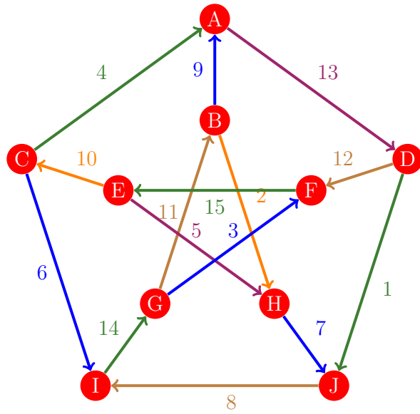
Figura 661: Flujo 653 de la gráfica de Petersen
