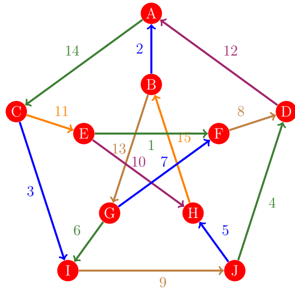
Figura 125: Flujo 117 de la gráfica de Petersen
