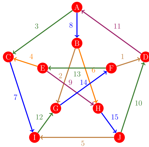
Figura 612: Flujo 604 de la gráfica de Petersen
