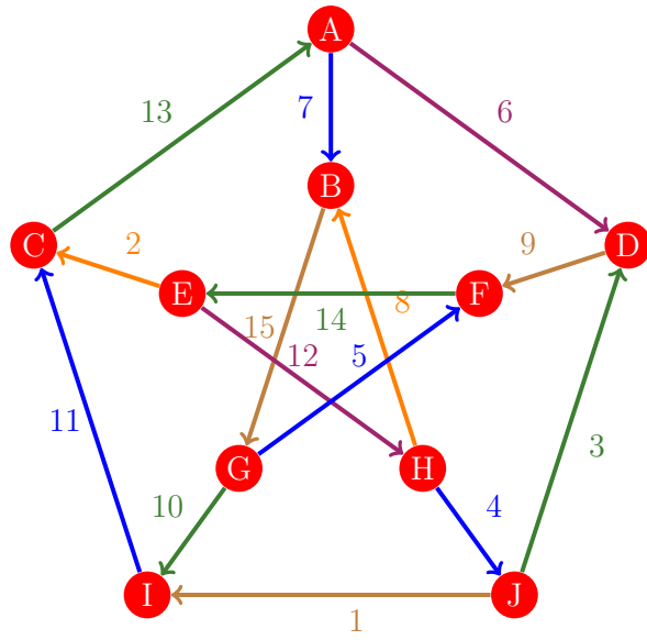
Figura 564: Flujo 556 de la gráfica de Petersen
