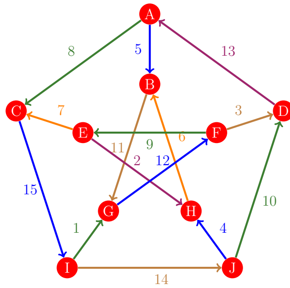
Figura 380: Flujo 372 de la gráfica de Petersen
