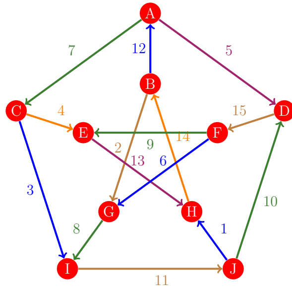
Figura 905: Flujo 897 de la gráfica de Petersen
