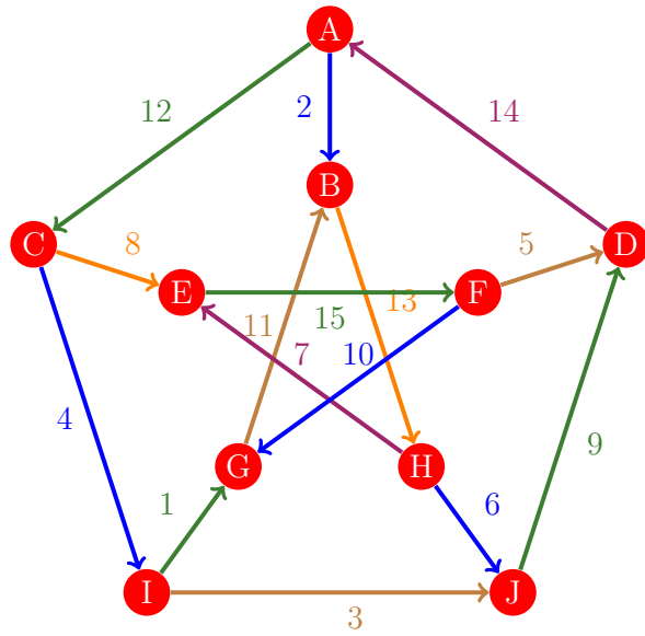
Figura 153: Flujo 145 de la gráfica de Petersen
