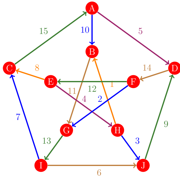
Figura 806: Flujo 798 de la gráfica de Petersen
