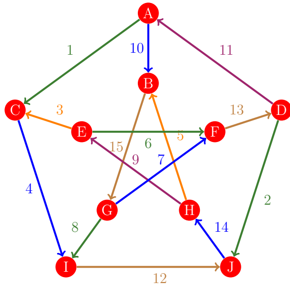
Figura 789: Flujo 781 de la gráfica de Petersen
