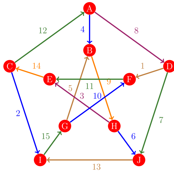
Figura 320: Flujo 312 de la gráfica de Petersen
