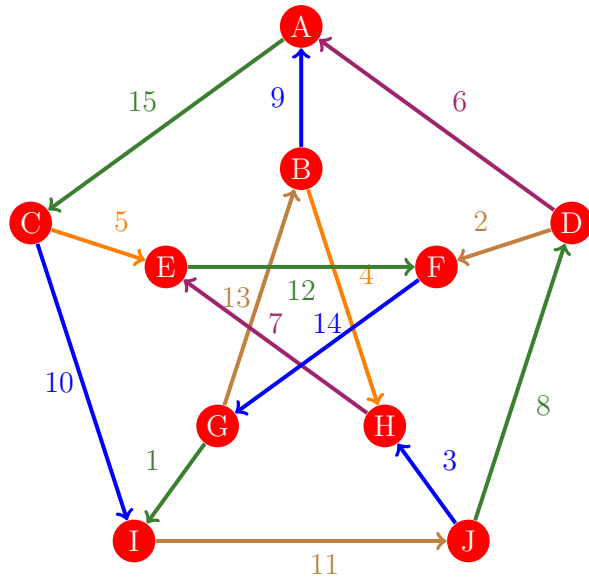
Figura 688: Flujo 680 de la gráfica de Petersen
