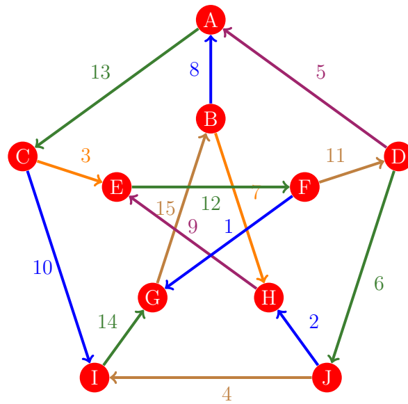
Figura 602: Flujo 594 de la gráfica de Petersen
