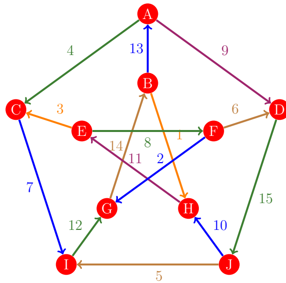
Figura 978: Flujo 970 de la gráfica de Petersen
