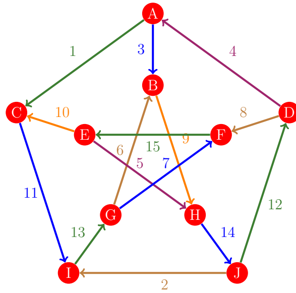
Figura 209: Flujo 201 de la gráfica de Petersen
