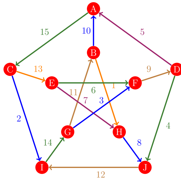
Figura 768: Flujo 760 de la gráfica de Petersen
