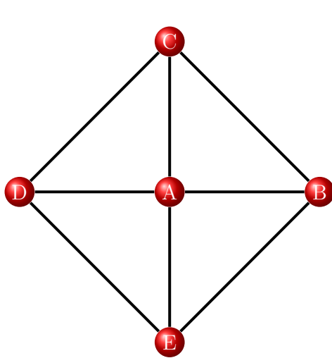
Figura 5: Gráfica G = (5, 8) .
