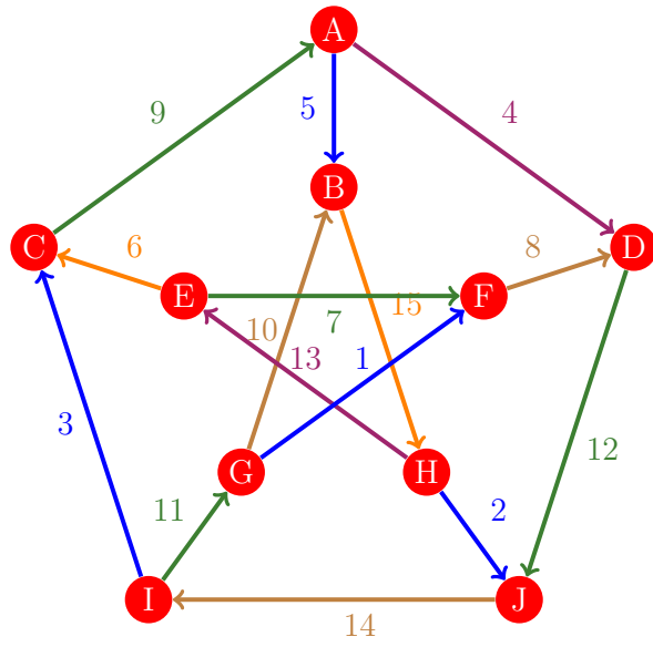
Figura 381: Flujo 373 de la gráfica de Petersen
