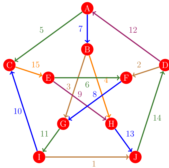
Figura 540: Flujo 532 de la gráfica de Petersen
