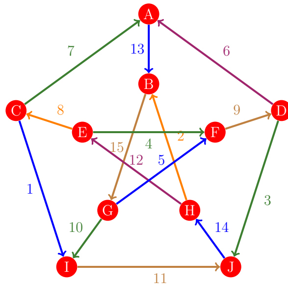
Figura 1028: Flujo 1020 de la gráfica de Petersen
