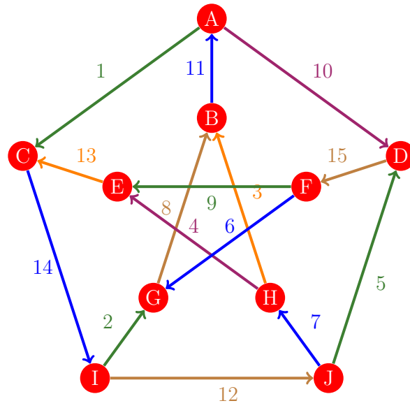
Figura 835: Flujo 827 de la gráfica de Petersen
