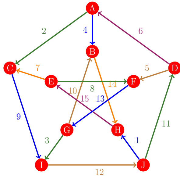
Figura 289: Flujo 281 de la gráfica de Petersen
