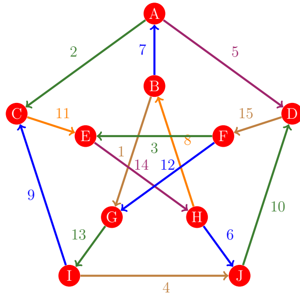
Figura 491: Flujo 483 de la gráfica de Petersen
