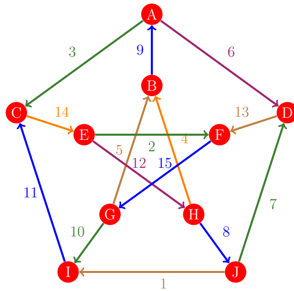
Figura 656: Flujo 648 de la gráfica de Petersen
