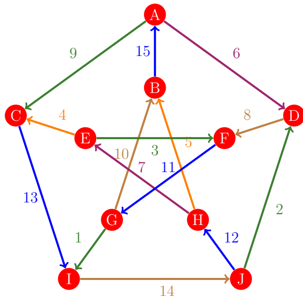
Figura 1152: Flujo 1144 de la gráfica de Petersen
