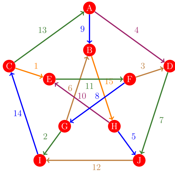
Figura 721: Flujo 713 de la gráfica de Petersen
