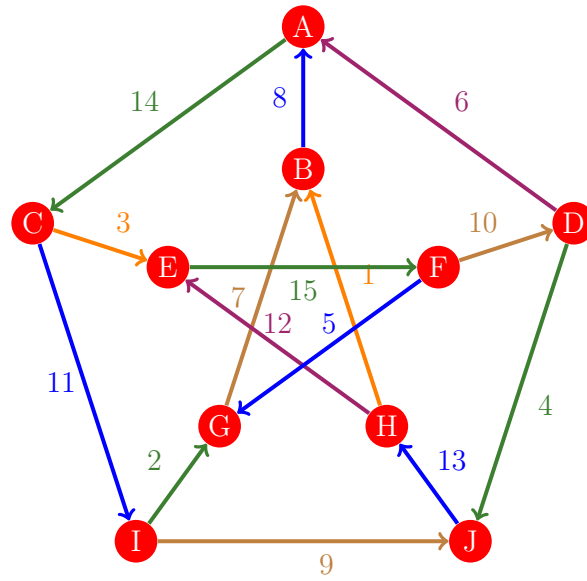
Figura 603: Flujo 595 de la gráfica de Petersen
