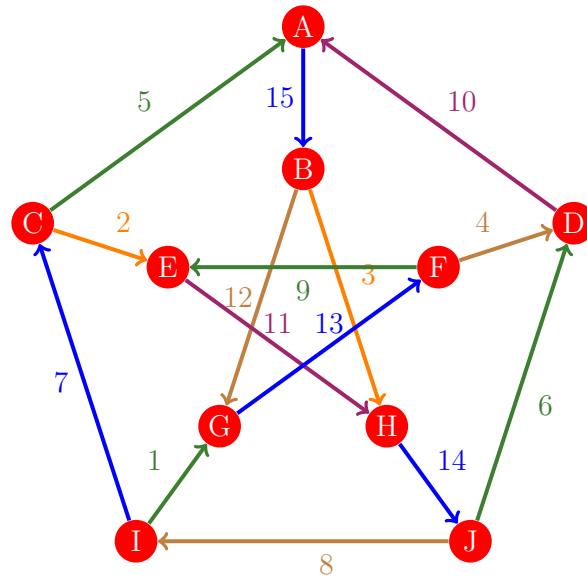
Figura 1179: Flujo 1171 de la gráfica de Petersen
