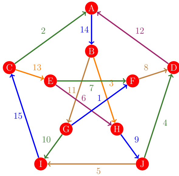
Figura 1091: Flujo 1083 de la gráfica de Petersen
