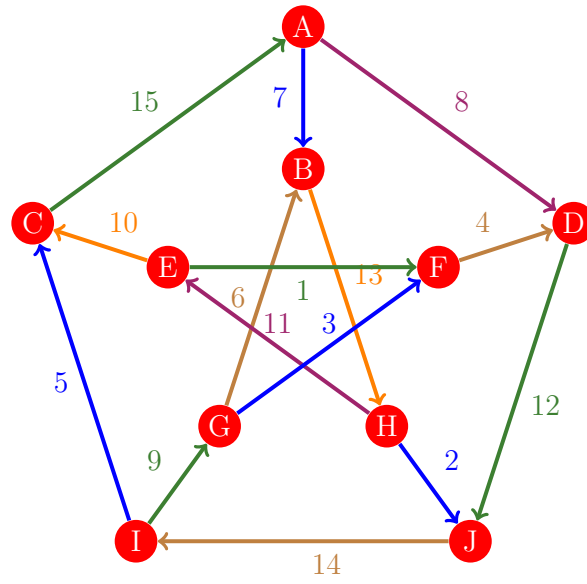
Figura 565: Flujo 557 de la gráfica de Petersen
