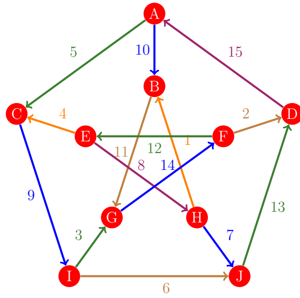
Figura 781: Flujo 773 de la gráfica de Petersen
