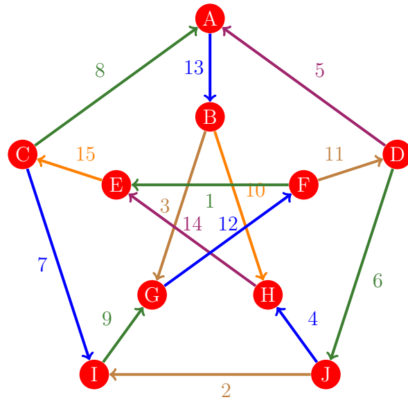
Figura 1029: Flujo 1021 de la gráfica de Petersen
