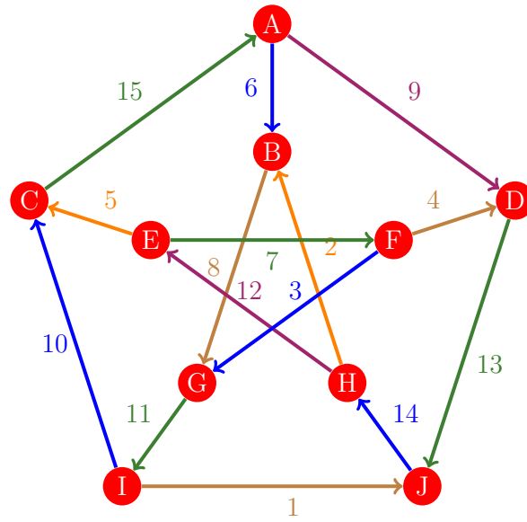
Figura 487: Flujo 479 de la gráfica de Petersen
