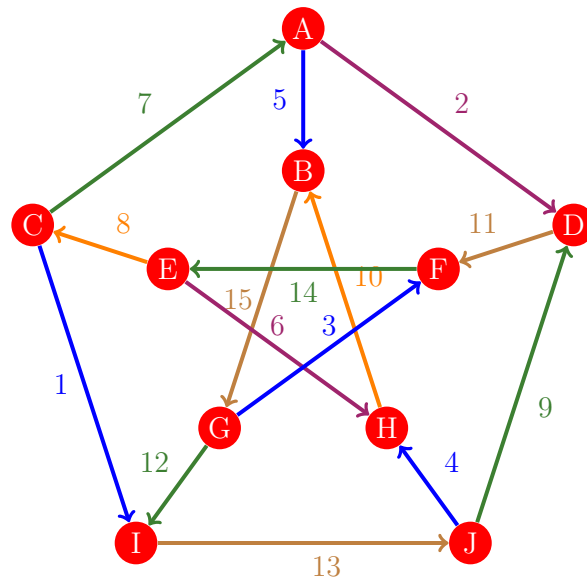
Figura 376: Flujo 368 de la gráfica de Petersen
