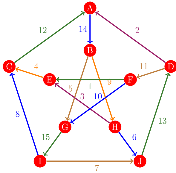
Figura 1115: Flujo 1107 de la gráfica de Petersen
