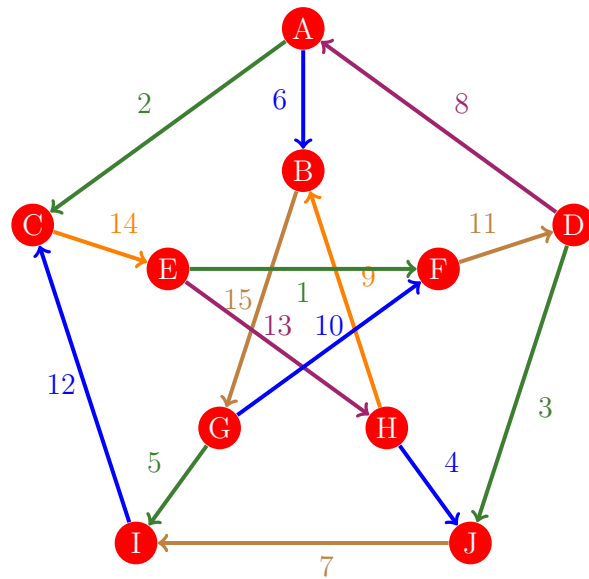
Figura 452: Flujo 444 de la gráfica de Petersen
