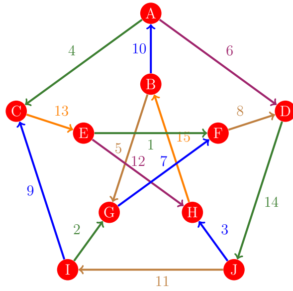
Figura 733: Flujo 725 de la gráfica de Petersen
