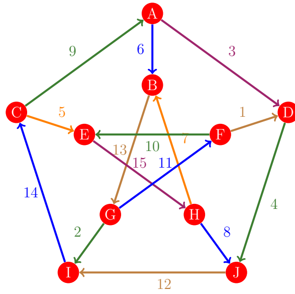
Figura 473: Flujo 465 de la gráfica de Petersen
