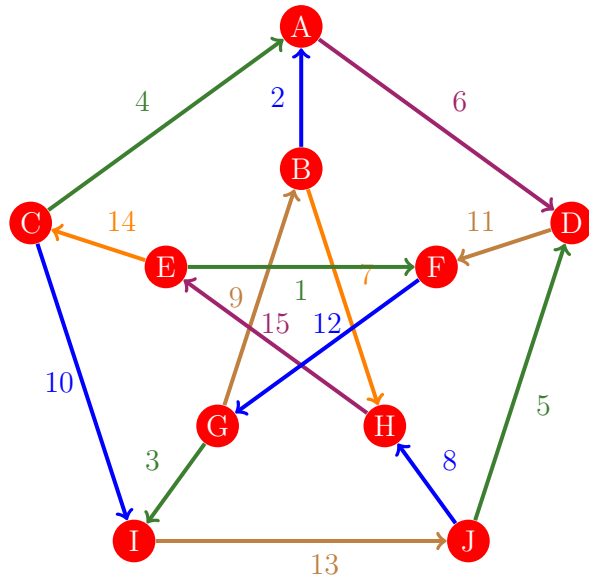
Figura 90: Flujo 82 de la gráfica de Petersen
