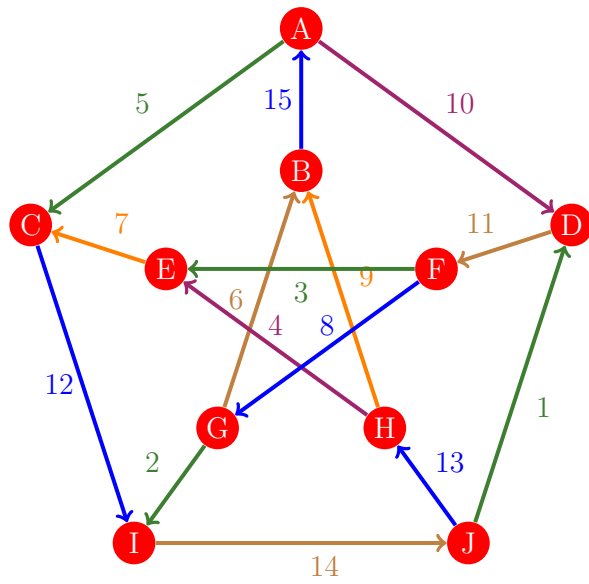
Figura 1134: Flujo 1126 de la gráfica de Petersen
