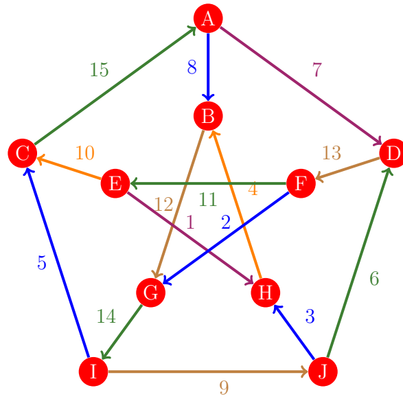
Figura 647: Flujo 639 de la gráfica de Petersen
