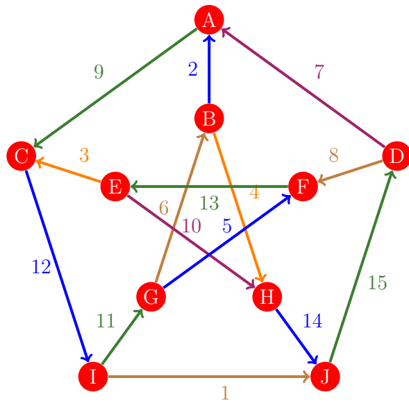
Figura 106: Flujo 98 de la gráfica de Petersen
