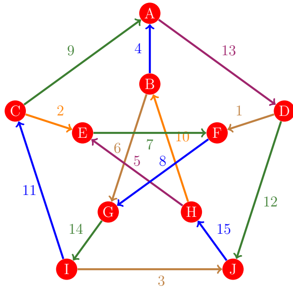
Figura 269: Flujo 261 de la gráfica de Petersen
