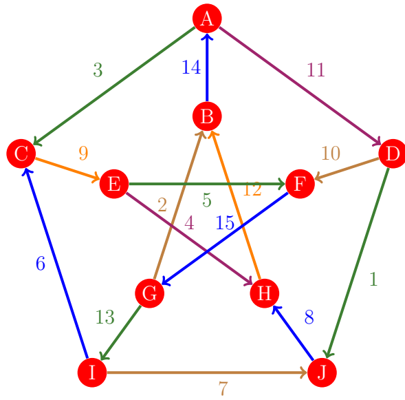
Figura 1057: Flujo 1049 de la gráfica de Petersen
