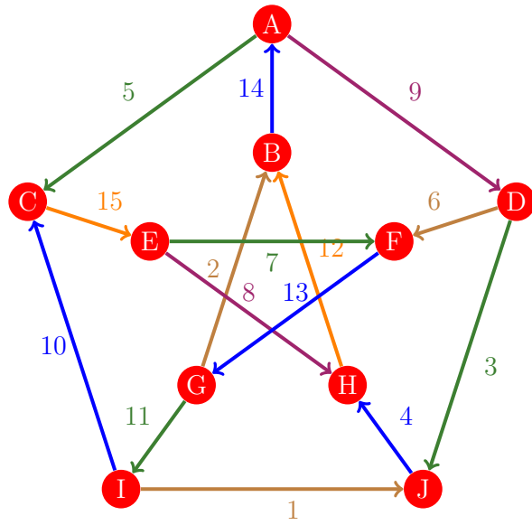
Figura 1061: Flujo 1053 de la gráfica de Petersen
