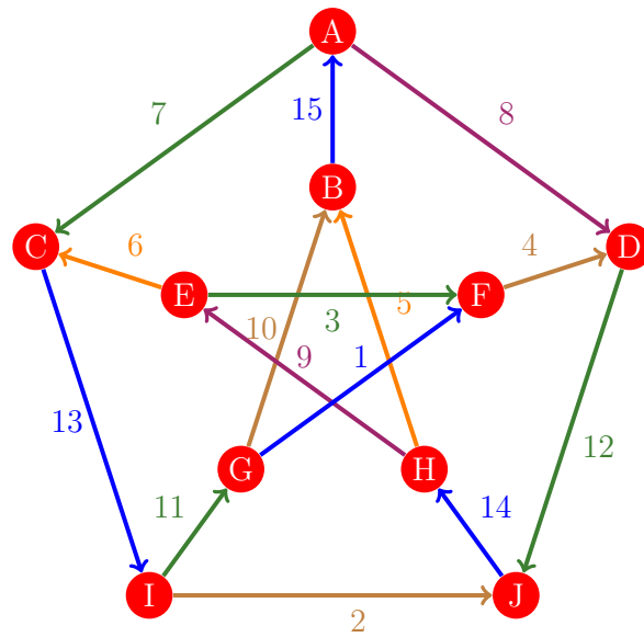
Figura 1144: Flujo 1136 de la gráfica de Petersen
