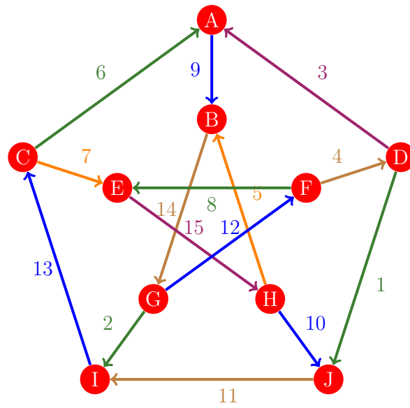
Figura 712: Flujo 704 de la gráfica de Petersen
