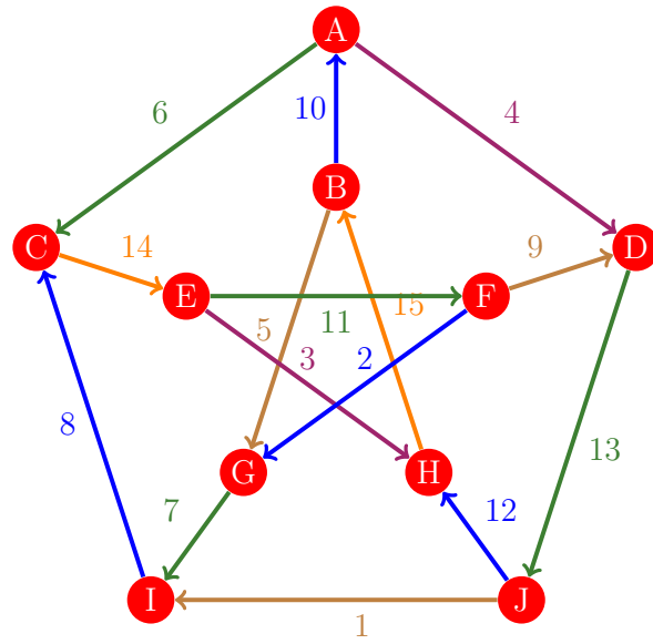
Figura 743: Flujo 735 de la gráfica de Petersen
