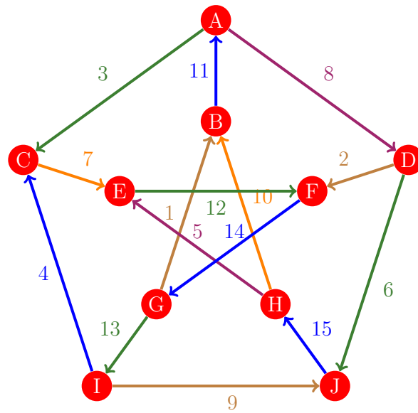
Figura 818: Flujo 810 de la gráfica de Petersen
