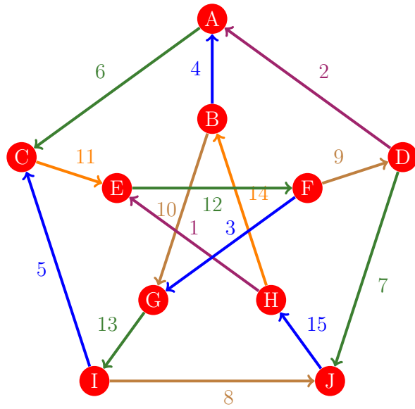
Figura 261: Flujo 253 de la gráfica de Petersen
