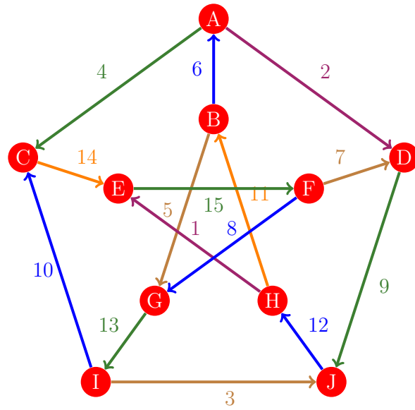
Figura 419: Flujo 411 de la gráfica de Petersen
