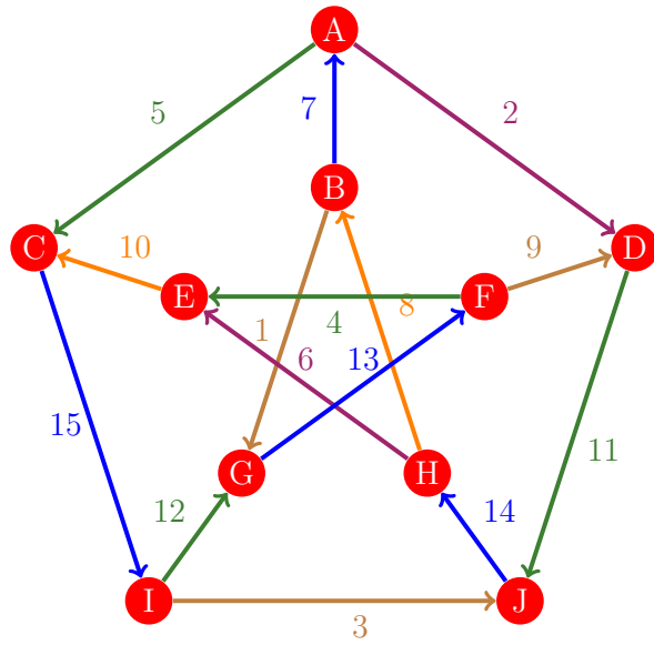
Figura 499: Flujo 491 de la gráfica de Petersen
