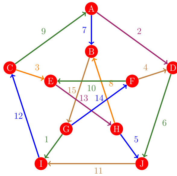
Figura 558: Flujo 550 de la gráfica de Petersen
