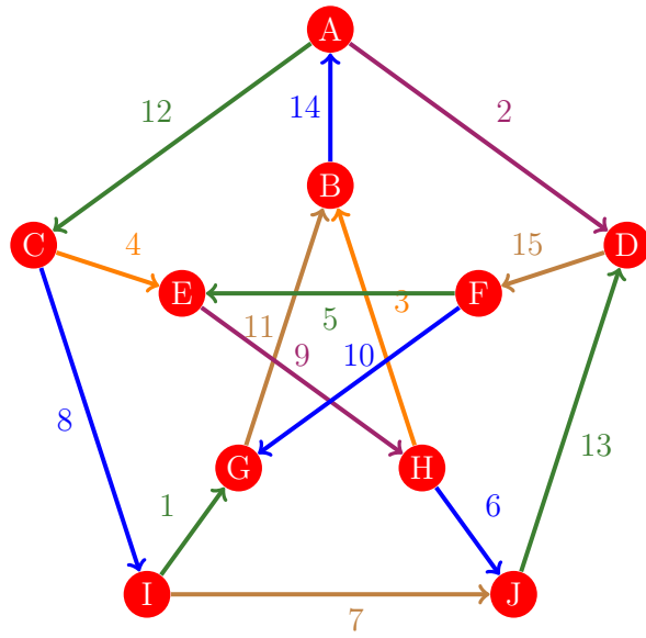
Figura 1077: Flujo 1069 de la gráfica de Petersen
