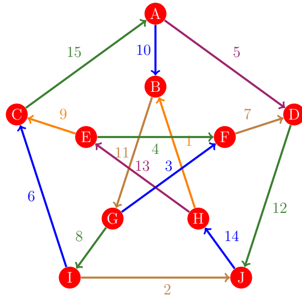
Figura 807: Flujo 799 de la gráfica de Petersen
