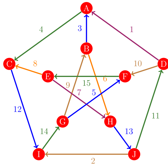
Figura 174: Flujo 166 de la gráfica de Petersen
