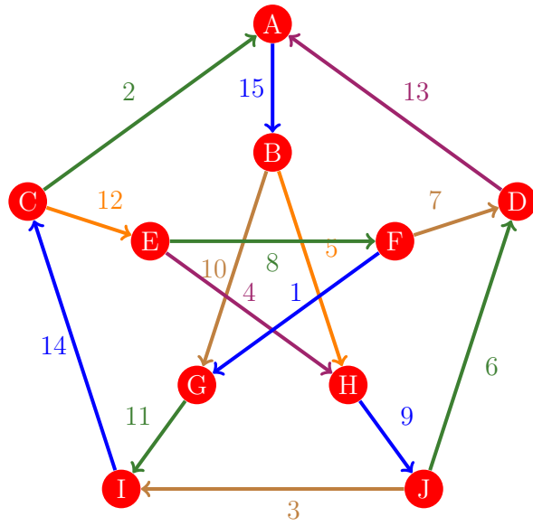
Figura 1170: Flujo 1162 de la gráfica de Petersen
