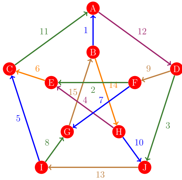
Figura 28: Flujo 20 de la gráfica de Petersen
