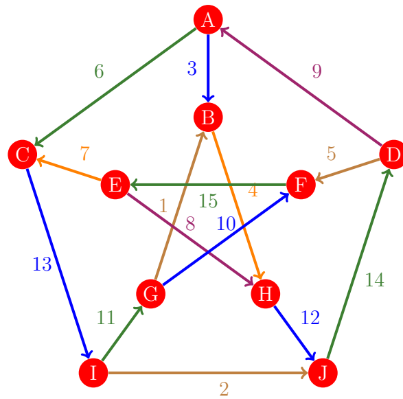
Figura 216: Flujo 208 de la gráfica de Petersen
