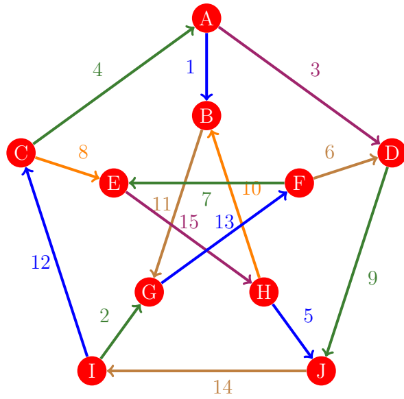
Figura 52: Flujo 44 de la gráfica de Petersen
