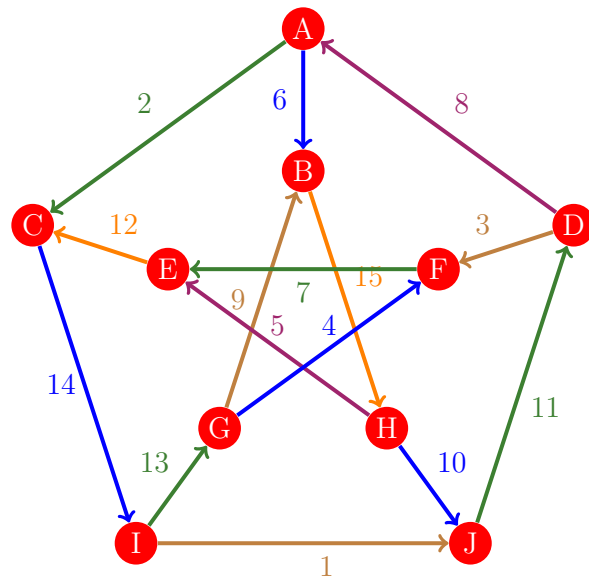
Figura 451: Flujo 443 de la gráfica de Petersen
