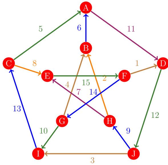
Figura 421: Flujo 413 de la gráfica de Petersen
