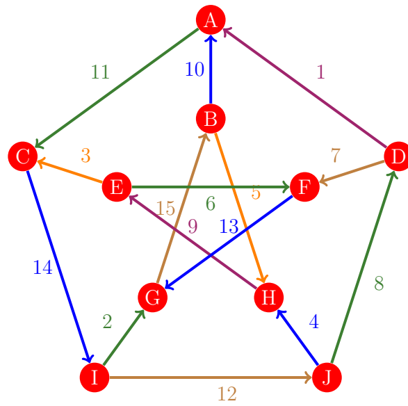
Figura 754: Flujo 746 de la gráfica de Petersen
