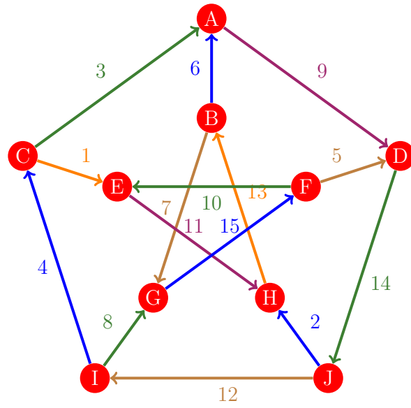
Figura 413: Flujo 405 de la gráfica de Petersen
