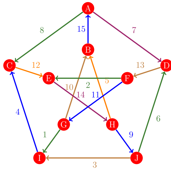
Figura 1148: Flujo 1140 de la gráfica de Petersen
