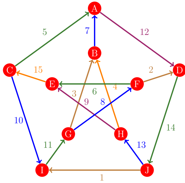
Figura 498: Flujo 490 de la gráfica de Petersen
