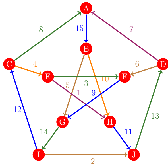
Figura 1187: Flujo 1179 de la gráfica de Petersen
