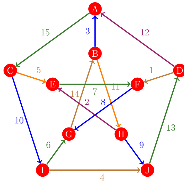
Figura 208: Flujo 200 de la gráfica de Petersen
