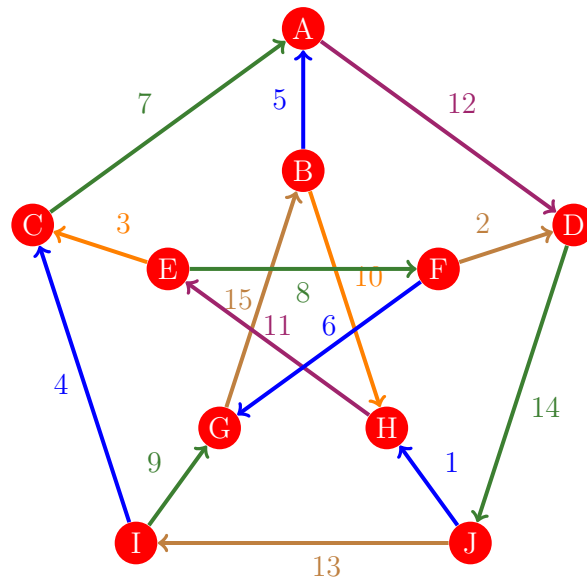
Figura 336: Flujo 328 de la gráfica de Petersen
