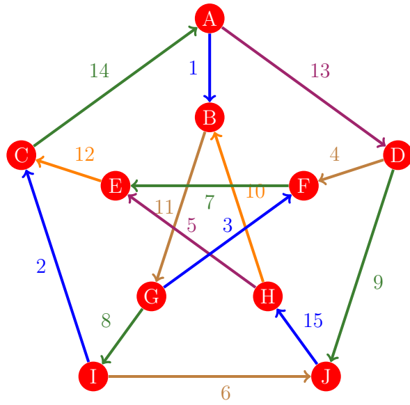
Figura 84: Flujo 76 de la gráfica de Petersen
