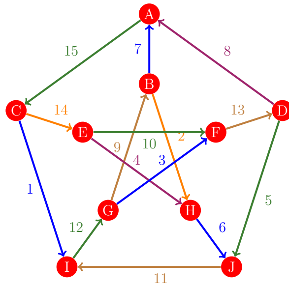
Figura 526: Flujo 518 de la gráfica de Petersen
