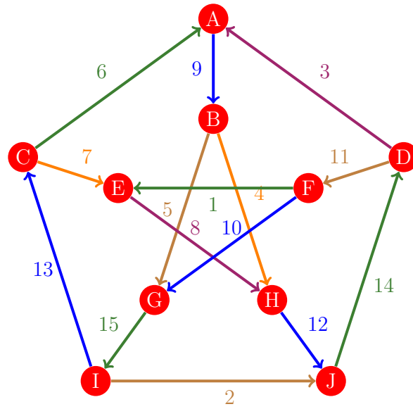
Figura 711: Flujo 703 de la gráfica de Petersen
