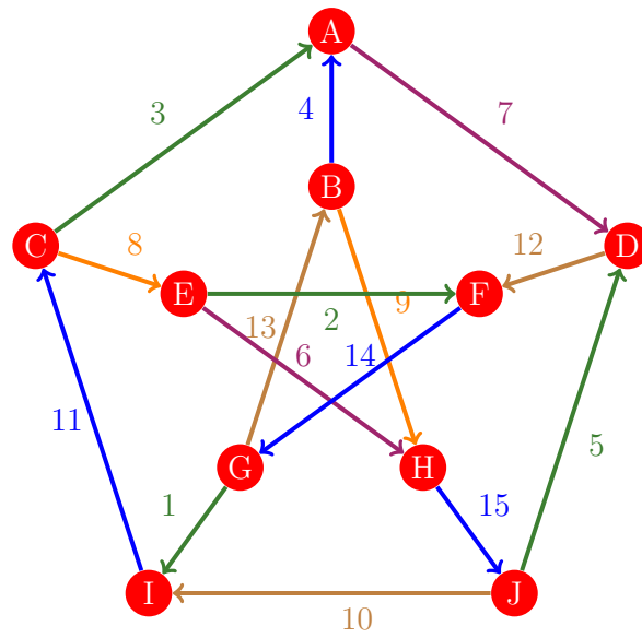
Figura 252: Flujo 244 de la gráfica de Petersen
