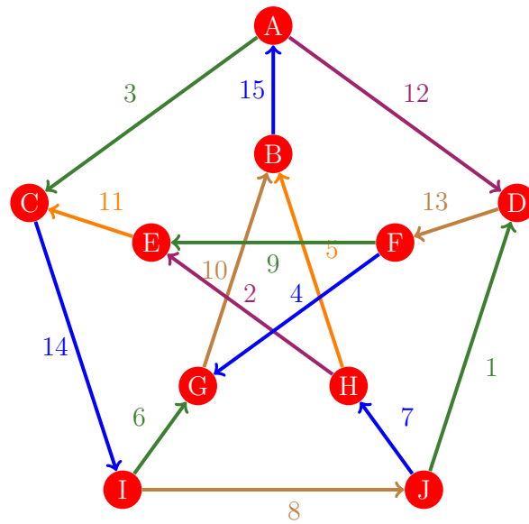
Figura 1132: Flujo 1124 de la gráfica de Petersen
