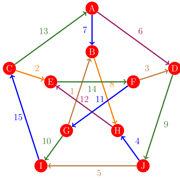
Figura 561: Flujo 553 de la gráfica de Petersen
