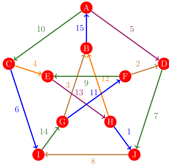
Figura 1153: Flujo 1145 de la gráfica de Petersen
