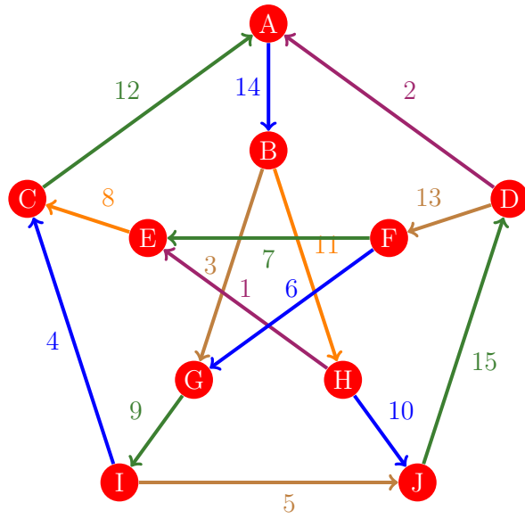
Figura 1118: Flujo 1110 de la gráfica de Petersen
