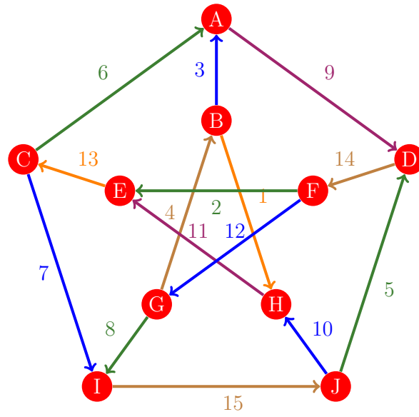
Figura 175: Flujo 167 de la gráfica de Petersen
