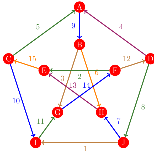
Figura 705: Flujo 697 de la gráfica de Petersen
