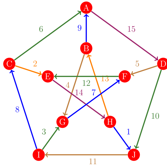
Figura 669: Flujo 661 de la gráfica de Petersen
