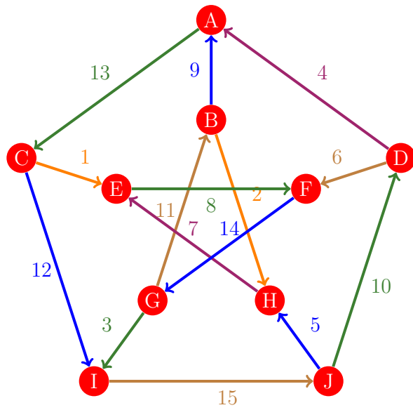
Figura 682: Flujo 674 de la gráfica de Petersen
