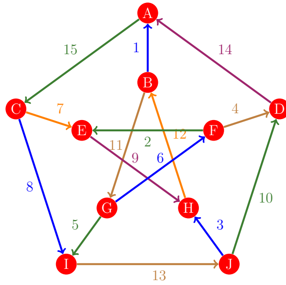
Figura 47: Flujo 39 de la gráfica de Petersen
