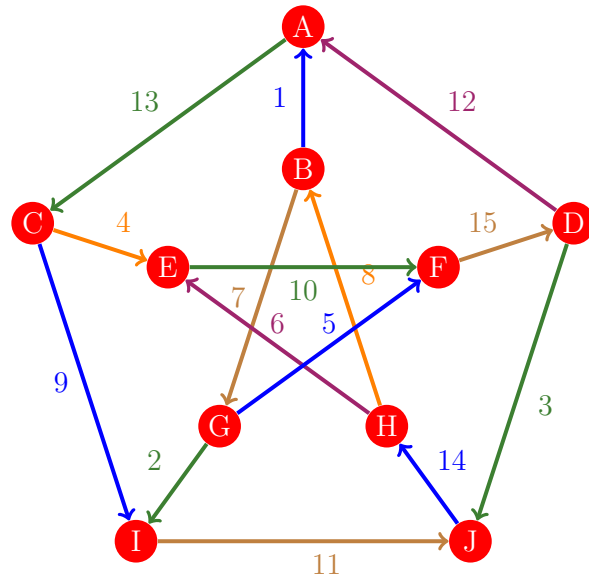
Figura 41: Flujo 33 de la gráfica de Petersen
