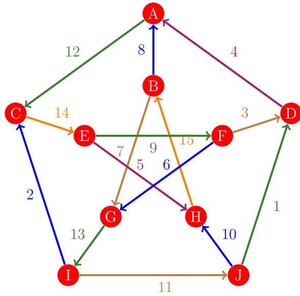
Figura 598: Flujo 590 de la gráfica de Petersen
