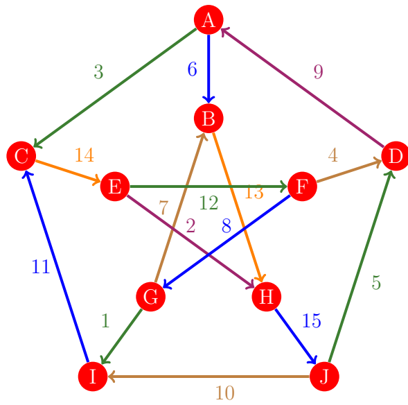
Figura 454: Flujo 446 de la gráfica de Petersen
