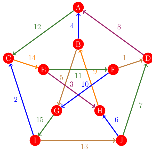
Figura 280: Flujo 272 de la gráfica de Petersen
