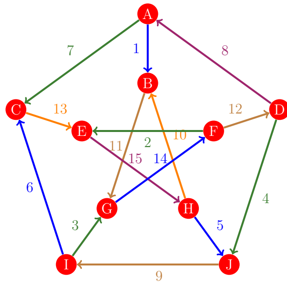
Figura 54: Flujo 46 de la gráfica de Petersen
