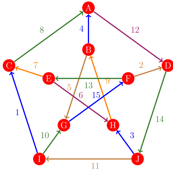
Figura 266: Flujo 258 de la gráfica de Petersen
