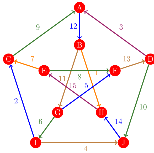
Figura 951: Flujo 943 de la gráfica de Petersen
