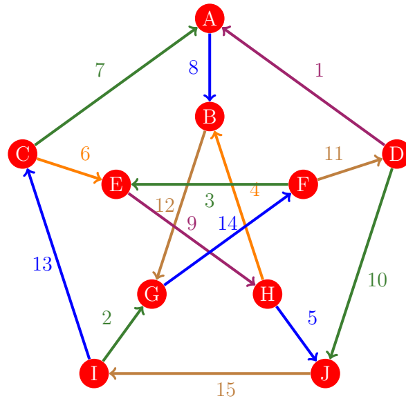
Figura 625: Flujo 617 de la gráfica de Petersen
