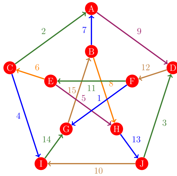
Figura 490: Flujo 482 de la gráfica de Petersen
