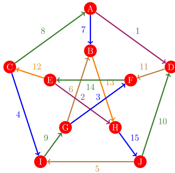
Figura 550: Flujo 542 de la gráfica de Petersen
