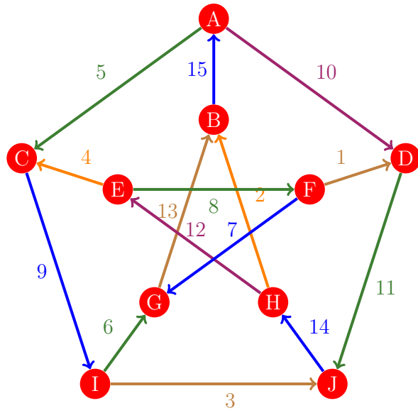
Figura 1140: Flujo 1132 de la gráfica de Petersen
