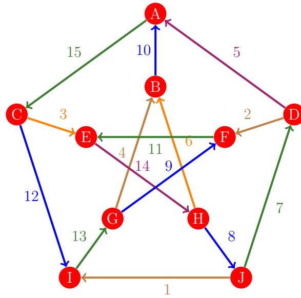
Figura 761: Flujo 753 de la gráfica de Petersen
