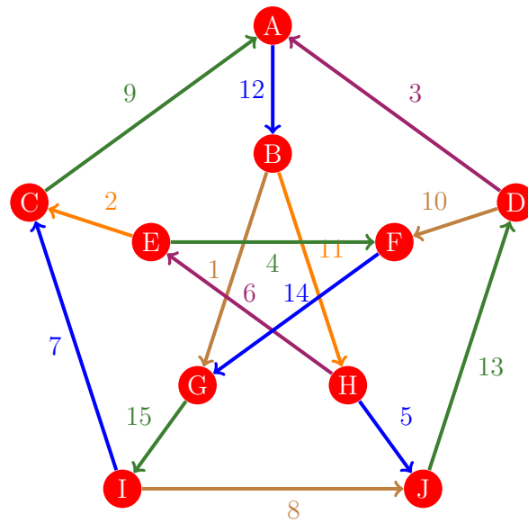
Figura 952: Flujo 944 de la gráfica de Petersen
