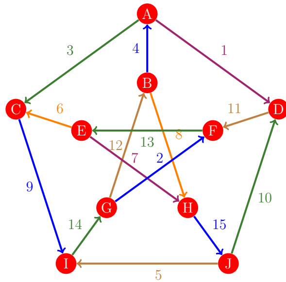
Figura 254: Flujo 246 de la gráfica de Petersen
