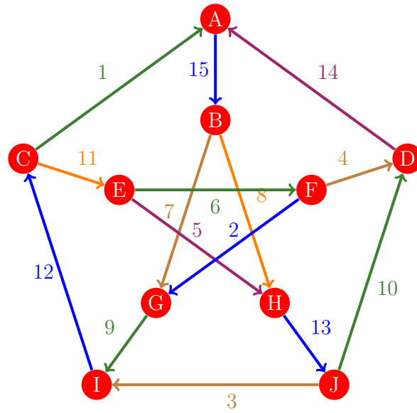
Figura 1207: Flujo 1199 de la gráfica de Petersen
