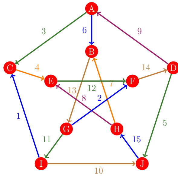
Figura 456: Flujo 448 de la gráfica de Petersen
