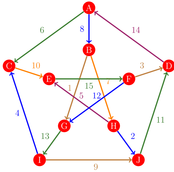
Figura 622: Flujo 614 de la gráfica de Petersen
