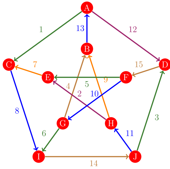
Figura 1003: Flujo 995 de la gráfica de Petersen
