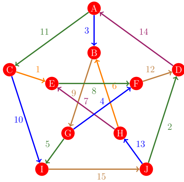
Figura 234: Flujo 226 de la gráfica de Petersen
