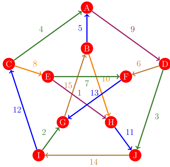
Figura 332: Flujo 324 de la gráfica de Petersen
