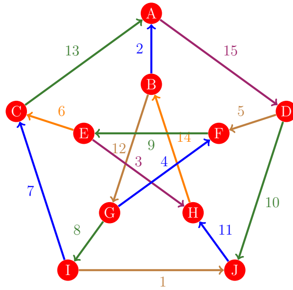
Figura 117: Flujo 109 de la gráfica de Petersen
