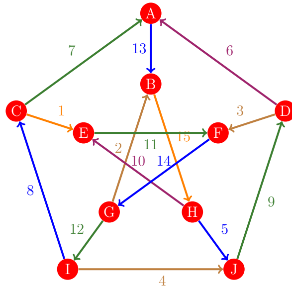
Figura 1025: Flujo 1017 de la gráfica de Petersen
