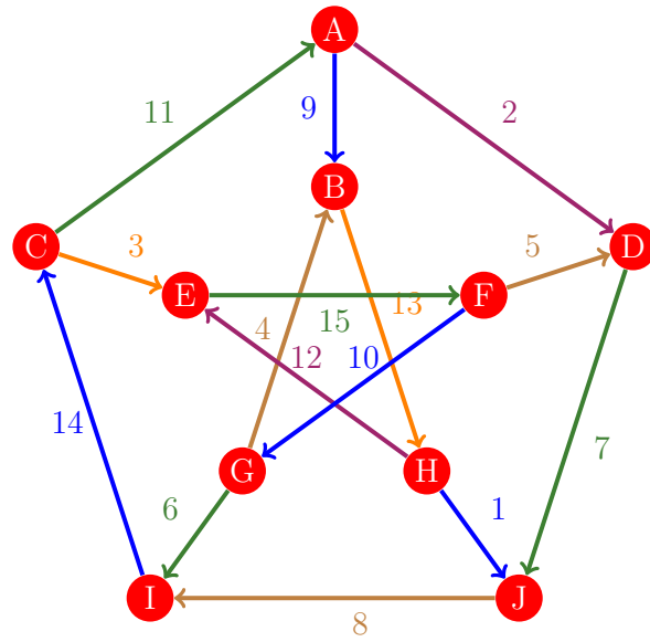
Figura 717: Flujo 709 de la gráfica de Petersen
