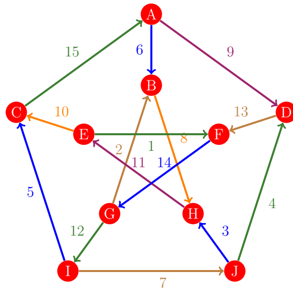
Figura 488: Flujo 480 de la gráfica de Petersen
