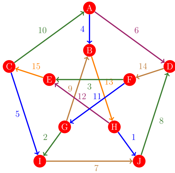
Figura 315: Flujo 307 de la gráfica de Petersen
