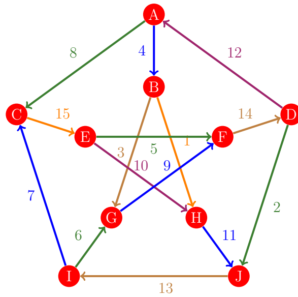
Figura 308: Flujo 300 de la gráfica de Petersen
