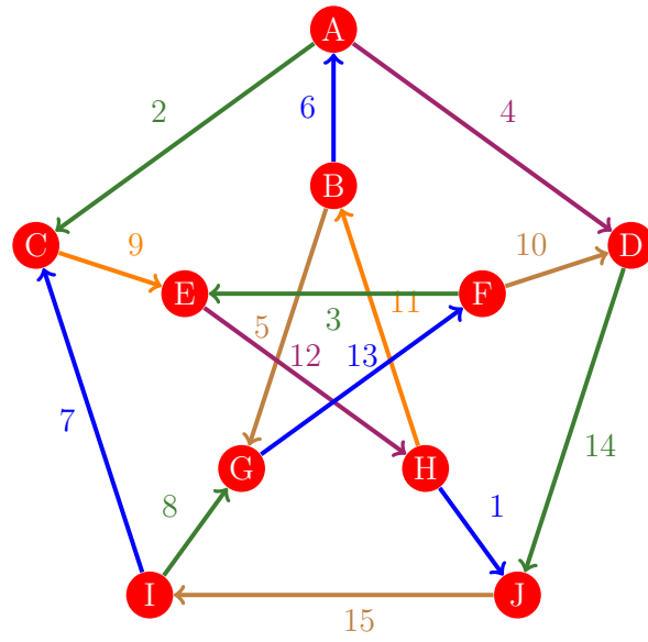
Figura 411: Flujo 403 de la gráfica de Petersen
