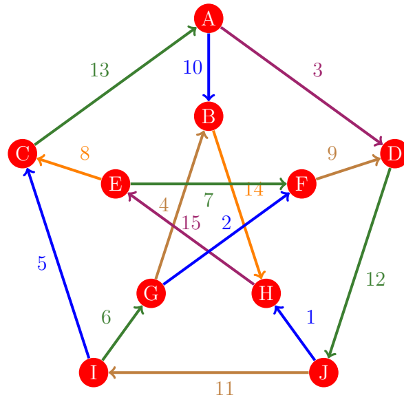
Figura 797: Flujo 789 de la gráfica de Petersen
