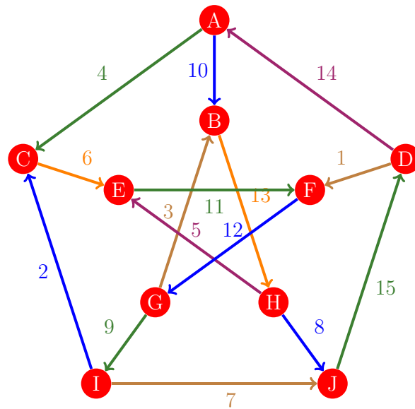
Figura 774: Flujo 766 de la gráfica de Petersen
