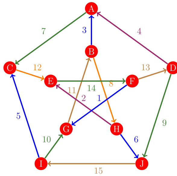
Figura 180: Flujo 172 de la gráfica de Petersen
