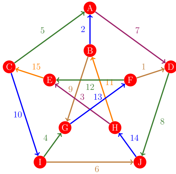
Figura 91: Flujo 83 de la gráfica de Petersen
