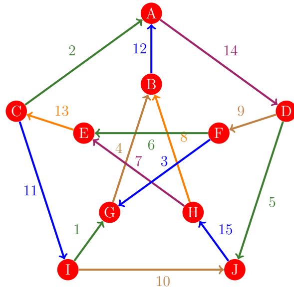
Figura 889: Flujo 881 de la gráfica de Petersen
