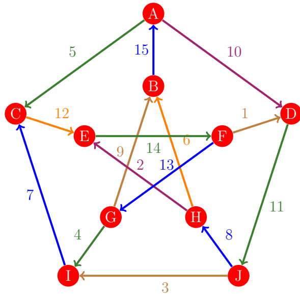
Figura 1137: Flujo 1129 de la gráfica de Petersen
