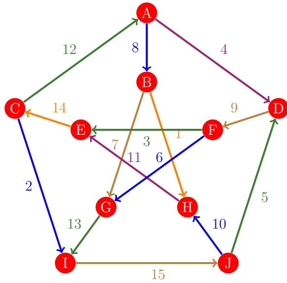
Figura 638: Flujo 630 de la gráfica de Petersen
