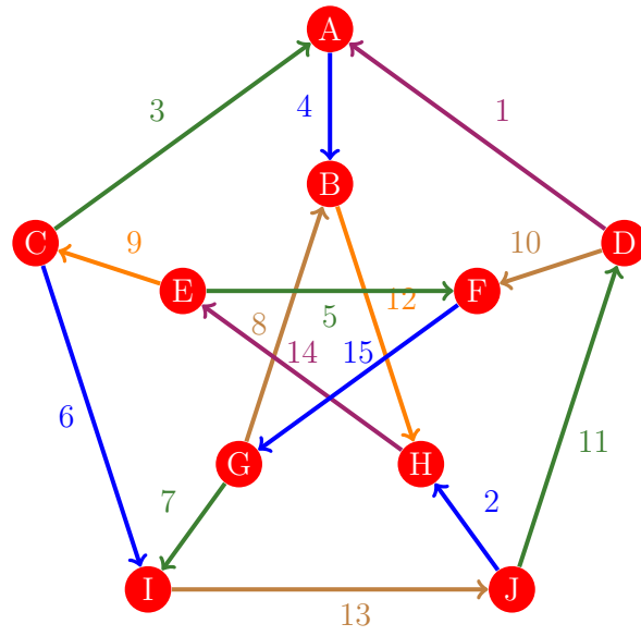
Figura 291: Flujo 283 de la gráfica de Petersen
