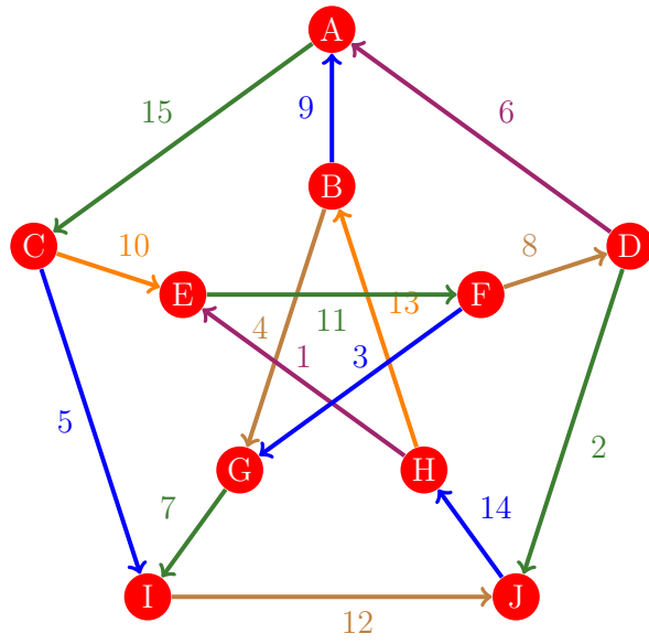
Figura 687: Flujo 679 de la gráfica de Petersen
