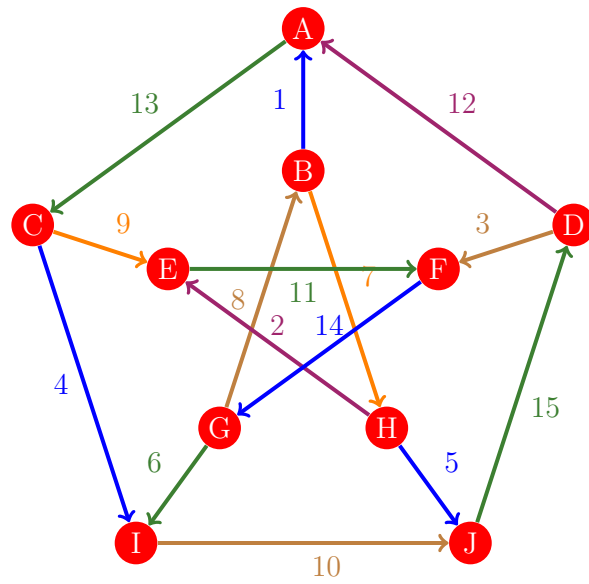
Figura 42: Flujo 34 de la gráfica de Petersen
