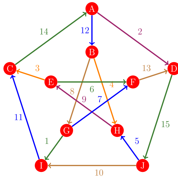
Figura 966: Flujo 958 de la gráfica de Petersen
