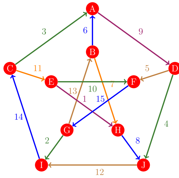
Figura 415: Flujo 407 de la gráfica de Petersen
