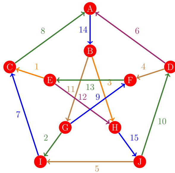
Figura 1106: Flujo 1098 de la gráfica de Petersen
