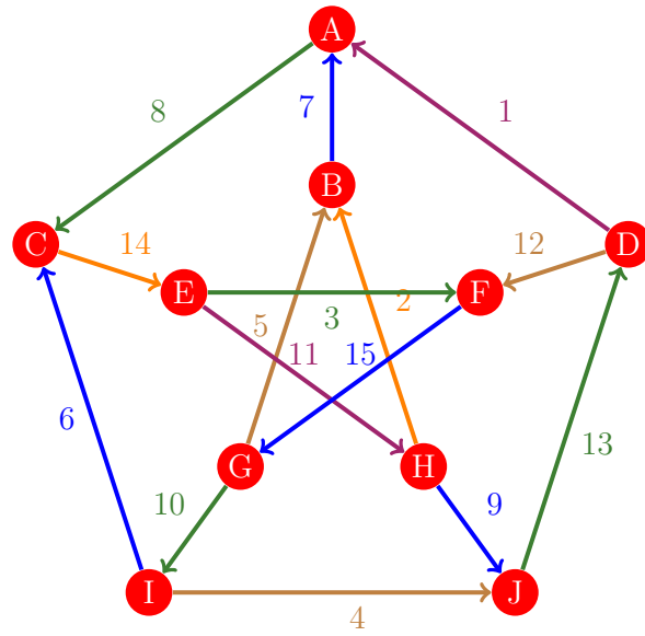
Figura 513: Flujo 505 de la gráfica de Petersen
