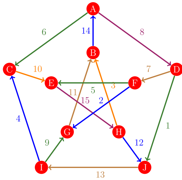
Figura 1064: Flujo 1056 de la gráfica de Petersen
