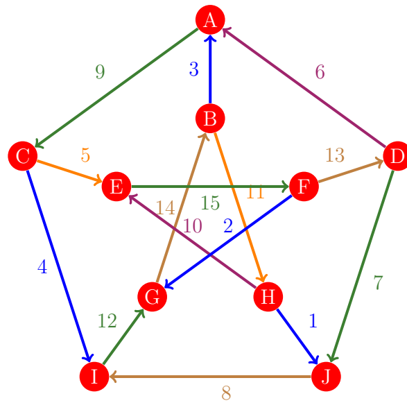
Figura 188: Flujo 180 de la gráfica de Petersen
