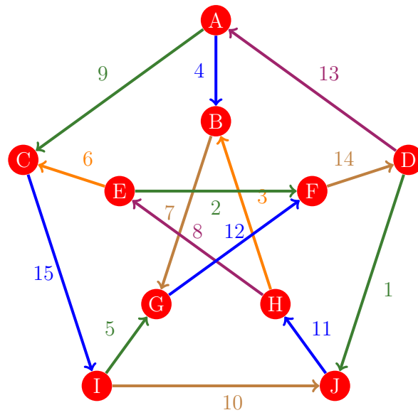
Figura 312: Flujo 304 de la gráfica de Petersen
