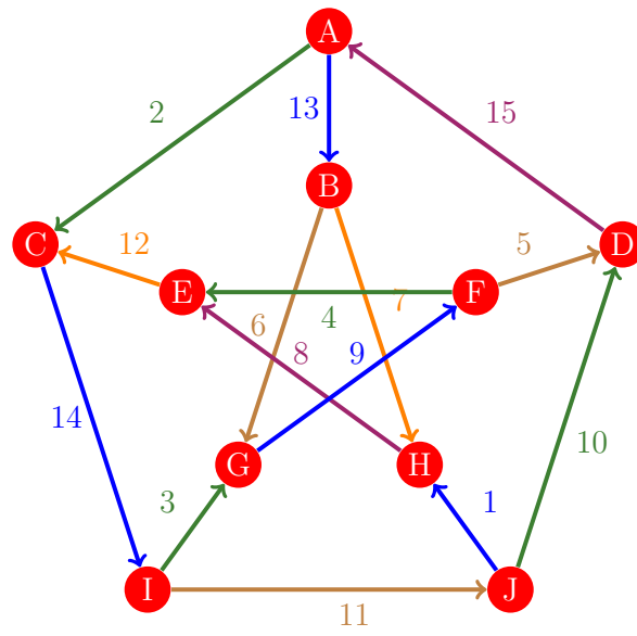
Figura 1011: Flujo 1003 de la gráfica de Petersen
