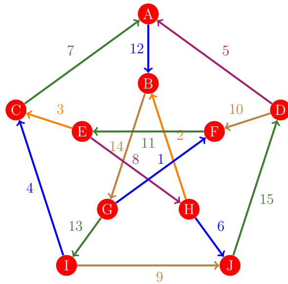
Figura 946: Flujo 938 de la gráfica de Petersen
