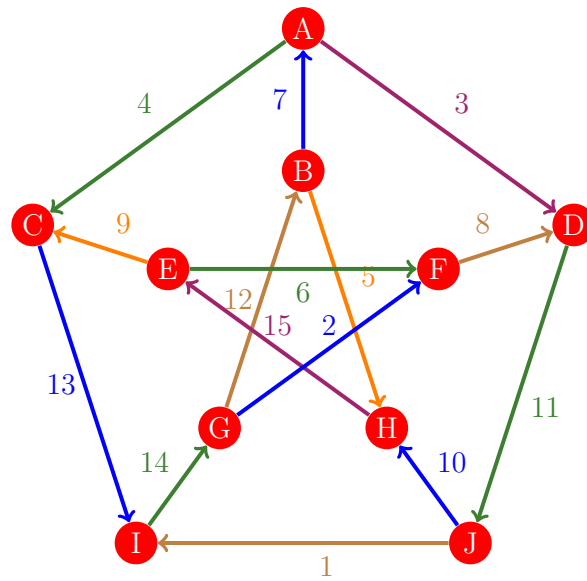
Figura 496: Flujo 488 de la gráfica de Petersen
