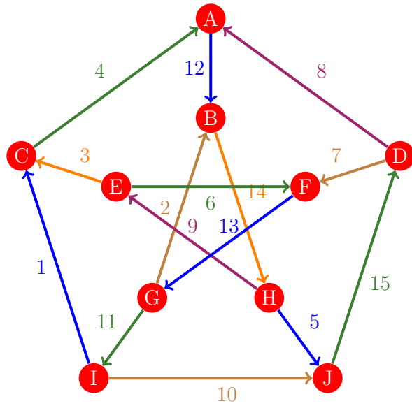
Figura 939: Flujo 931 de la gráfica de Petersen
