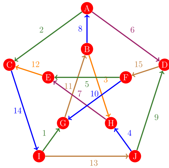
Figura 570: Flujo 562 de la gráfica de Petersen
