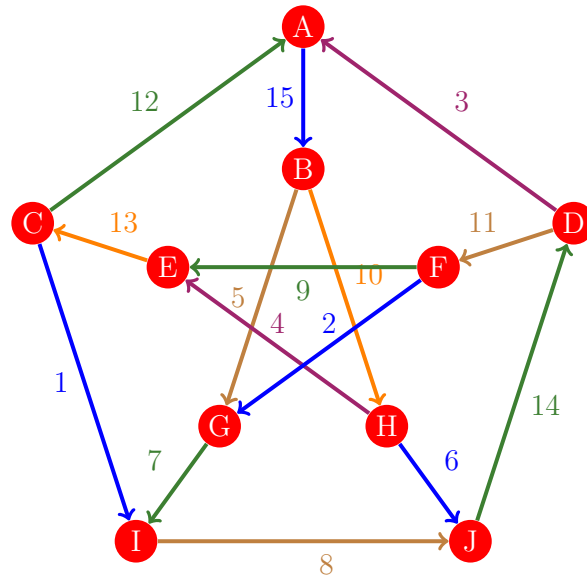
Figura 1201: Flujo 1193 de la gráfica de Petersen
