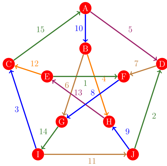
Figura 802: Flujo 794 de la gráfica de Petersen
