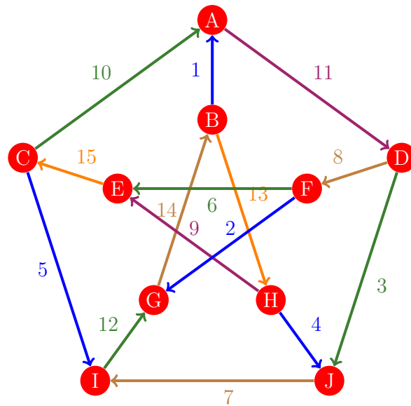
Figura 26: Flujo 18 de la gráfica de Petersen
