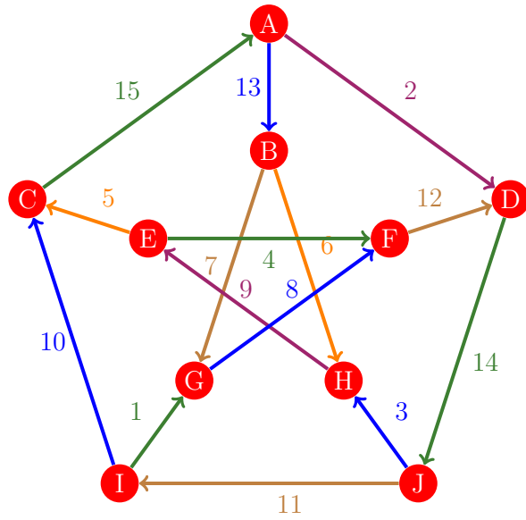
Figura 1048: Flujo 1040 de la gráfica de Petersen
