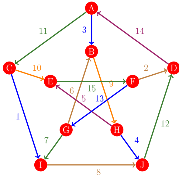
Figura 233: Flujo 225 de la gráfica de Petersen
