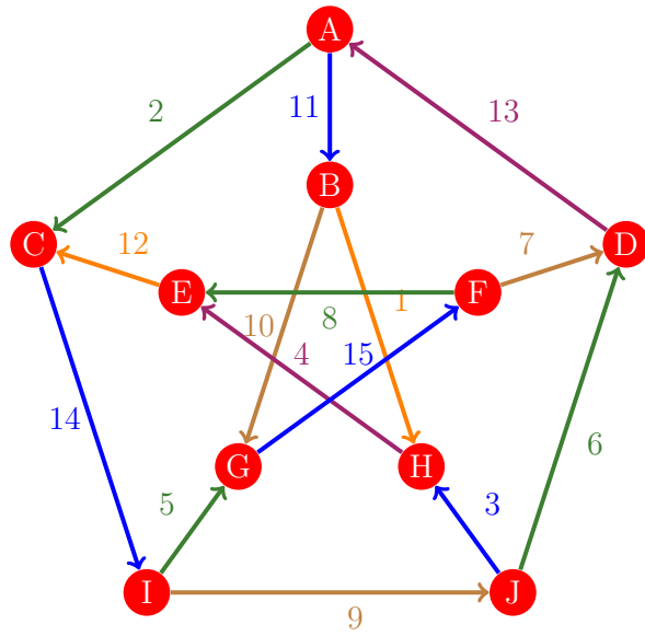
Figura 851: Flujo 843 de la gráfica de Petersen
