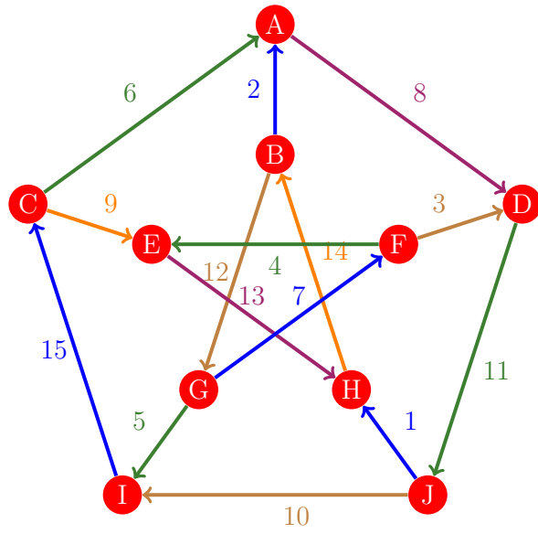
Figura 93: Flujo 85 de la gráfica de Petersen
