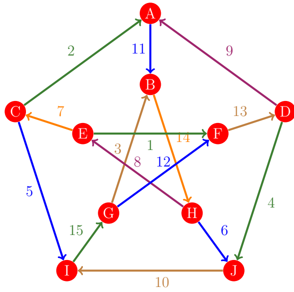
Figura 849: Flujo 841 de la gráfica de Petersen
