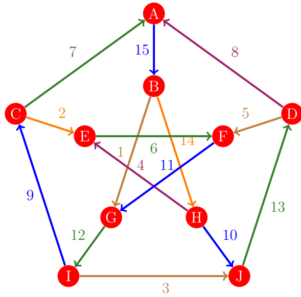
Figura 1186: Flujo 1178 de la gráfica de Petersen
