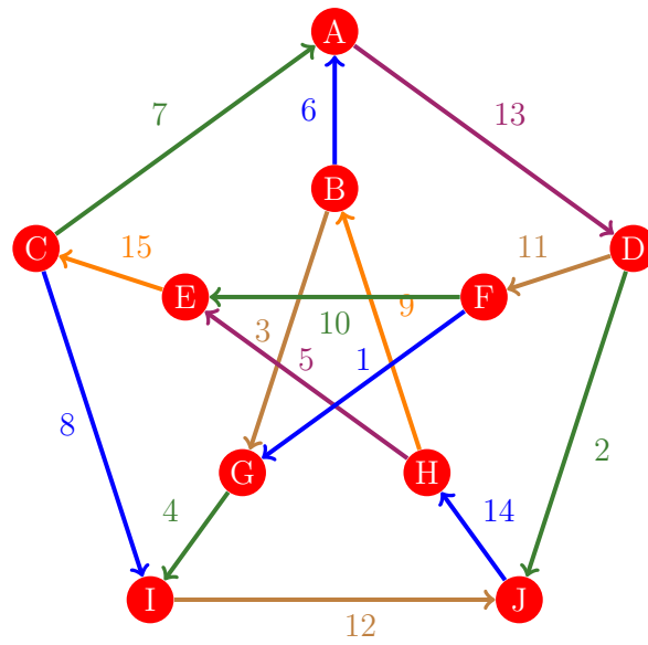
Figura 426: Flujo 418 de la gráfica de Petersen
