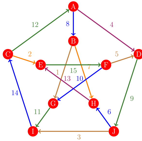
Figura 639: Flujo 631 de la gráfica de Petersen
