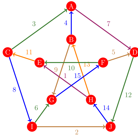
Figura 251: Flujo 243 de la gráfica de Petersen
