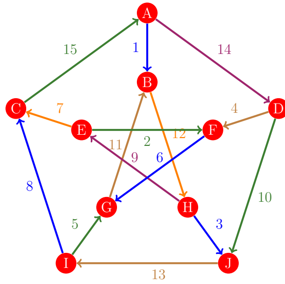
Figura 87: Flujo 79 de la gráfica de Petersen
