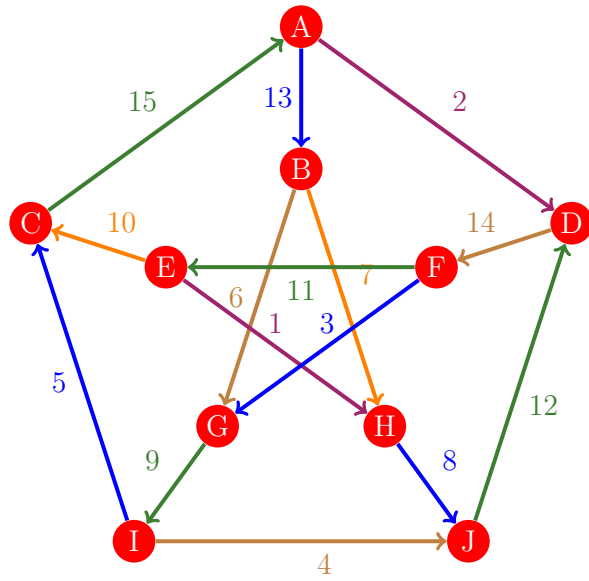
Figura 1047: Flujo 1039 de la gráfica de Petersen
