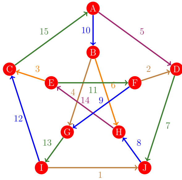
Figura 801: Flujo 793 de la gráfica de Petersen
