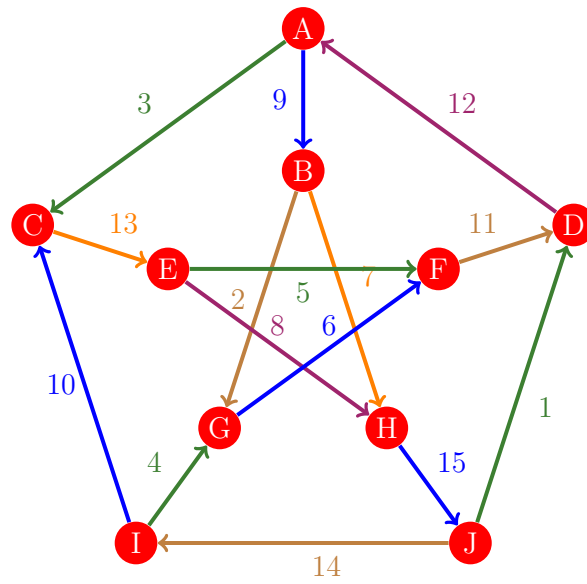
Figura 698: Flujo 690 de la gráfica de Petersen
