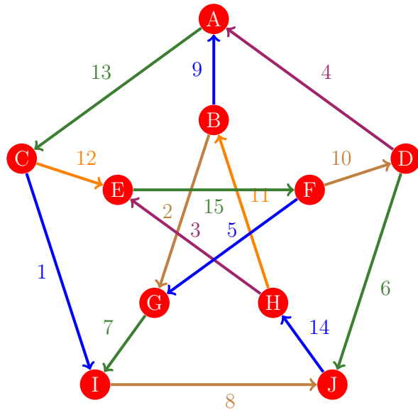
Figura 683: Flujo 675 de la gráfica de Petersen
