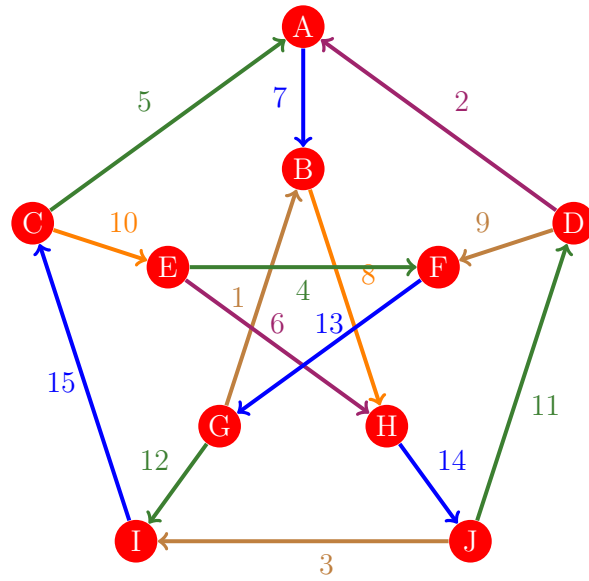
Figura 537: Flujo 529 de la gráfica de Petersen
