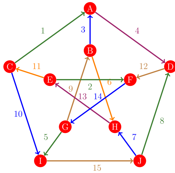
Figura 170: Flujo 162 de la gráfica de Petersen
