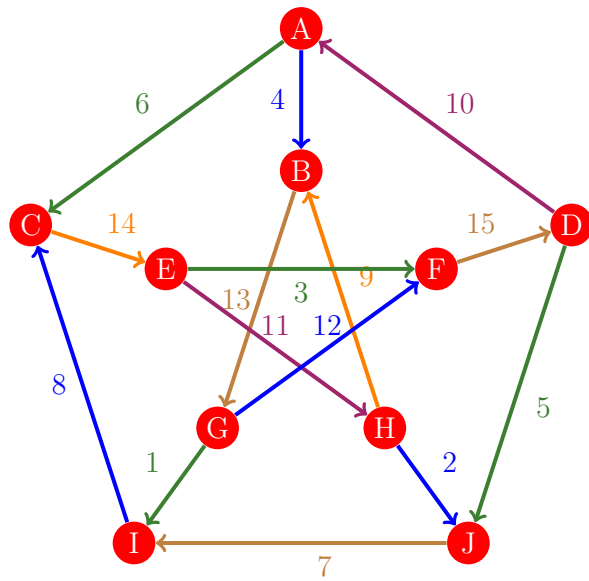
Figura 302: Flujo 294 de la gráfica de Petersen
