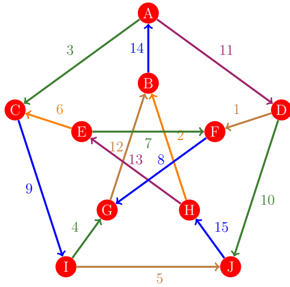
Figura 1058: Flujo 1050 de la gráfica de Petersen
