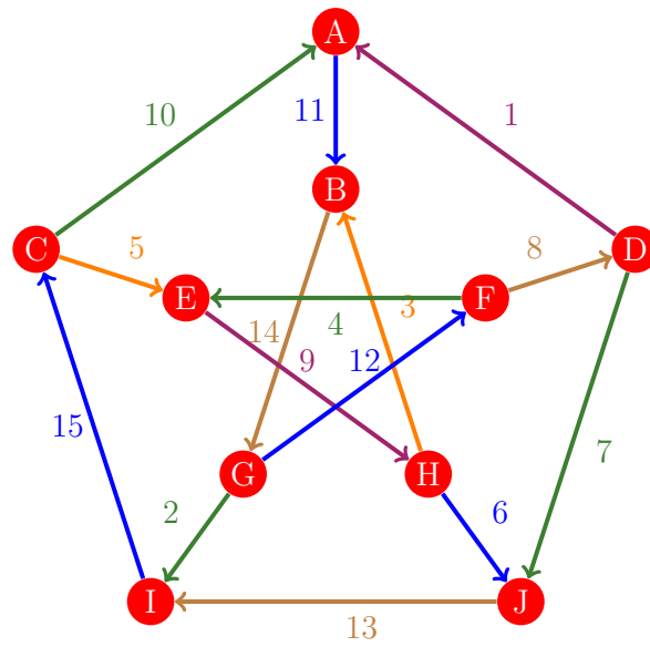
Figura 872: Flujo 864 de la gráfica de Petersen
