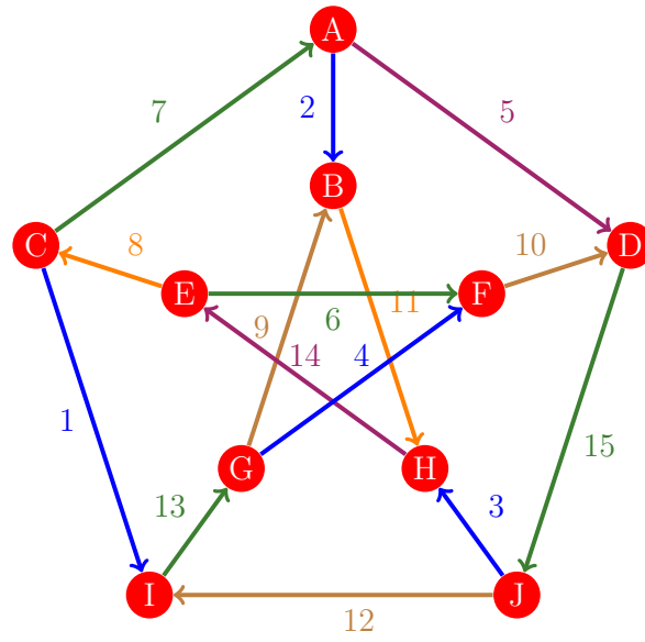
Figura 137: Flujo 129 de la gráfica de Petersen
