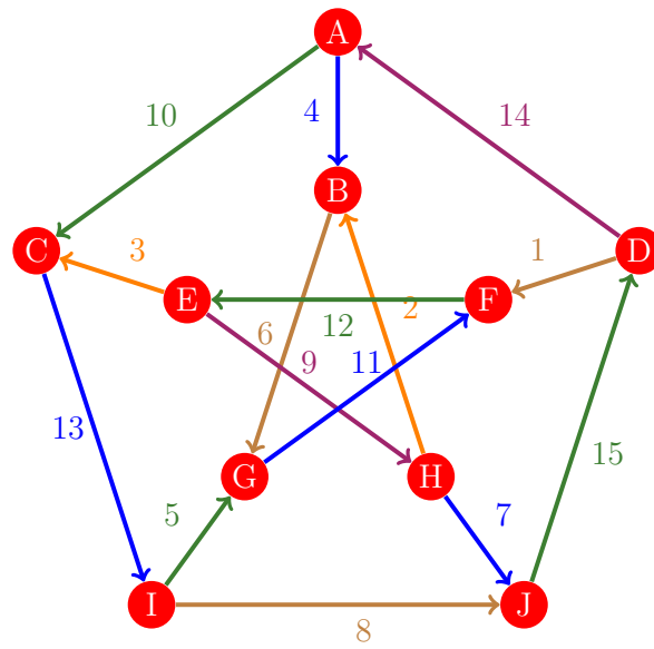
Figura 317: Flujo 309 de la gráfica de Petersen
