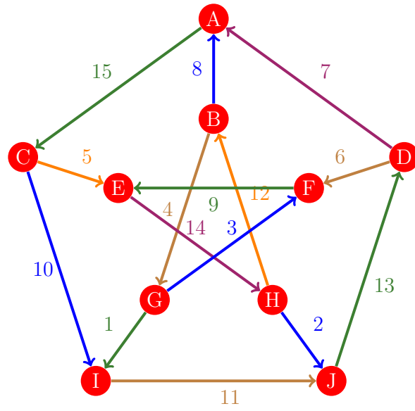
Figura 605: Flujo 597 de la gráfica de Petersen
