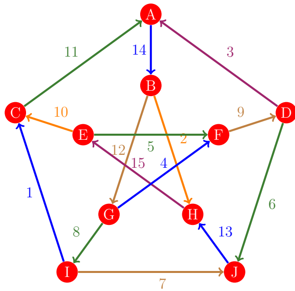
Figura 1114: Flujo 1106 de la gráfica de Petersen
