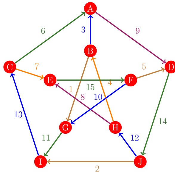
Figura 176: Flujo 168 de la gráfica de Petersen
