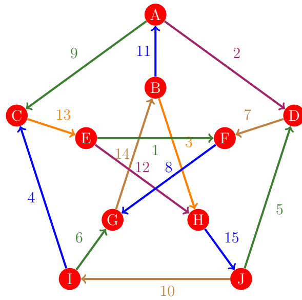
Figura 826: Flujo 818 de la gráfica de Petersen
