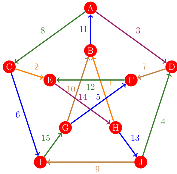
Figura 823: Flujo 815 de la gráfica de Petersen
