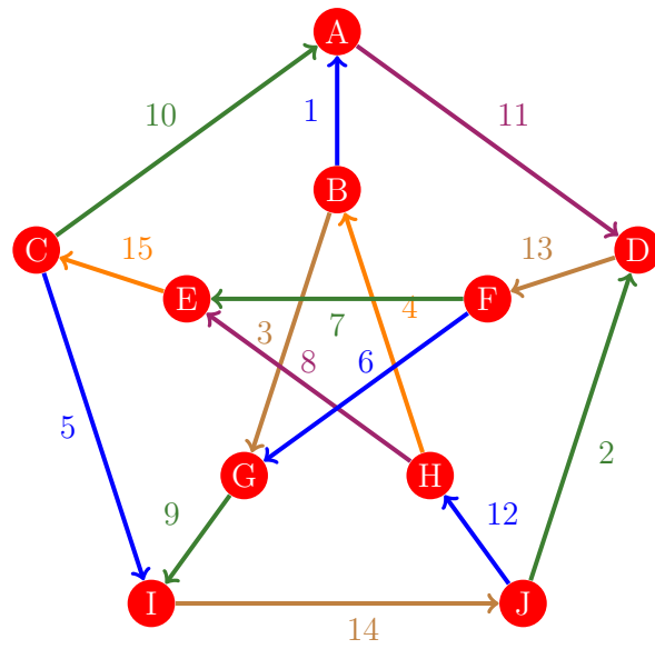
Figura 24: Flujo 16 de la gráfica de Petersen
