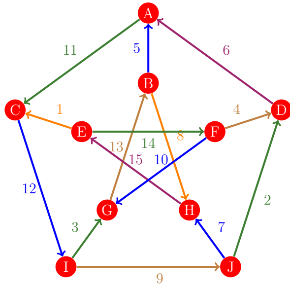
Figura 354: Flujo 346 de la gráfica de Petersen
