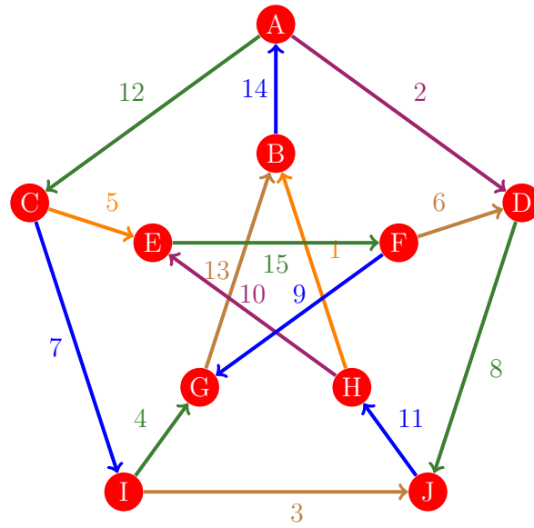
Figura 1079: Flujo 1071 de la gráfica de Petersen
