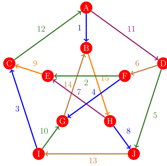
Figura 75: Flujo 67 de la gráfica de Petersen
