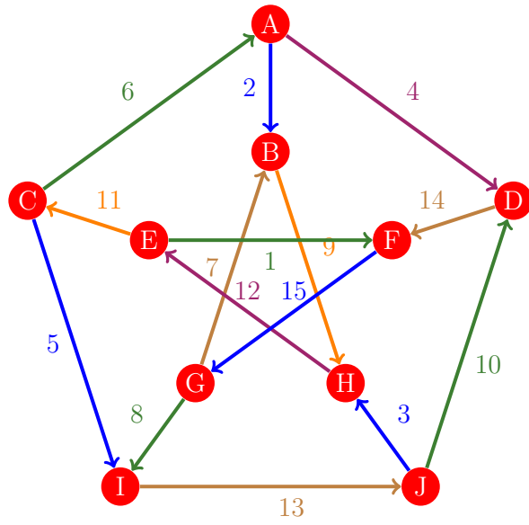
Figura 133: Flujo 125 de la gráfica de Petersen
