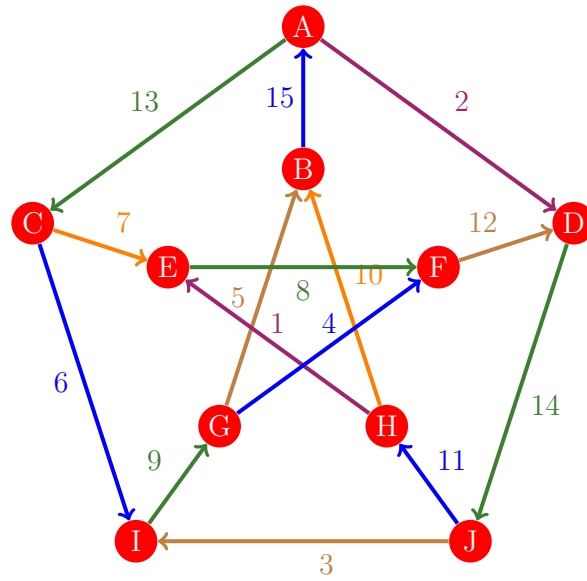
Figura 1163: Flujo 1155 de la gráfica de Petersen
