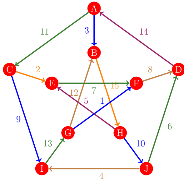
Figura 235: Flujo 227 de la gráfica de Petersen
