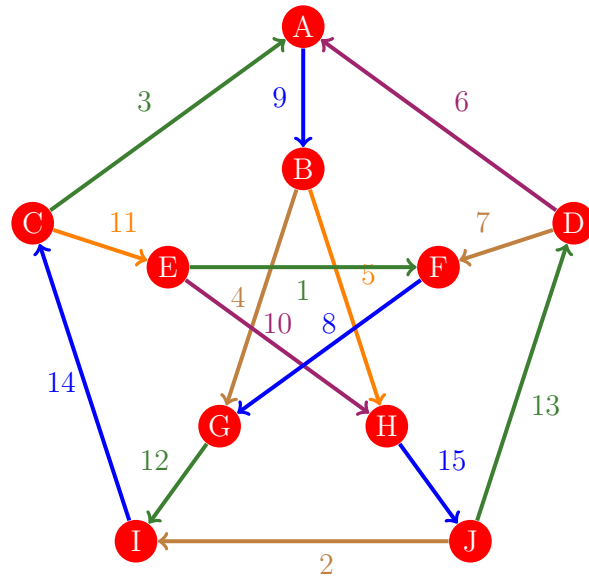
Figura 693: Flujo 685 de la gráfica de Petersen
