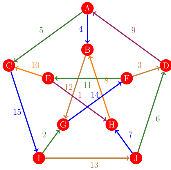
Figura 298: Flujo 290 de la gráfica de Petersen
