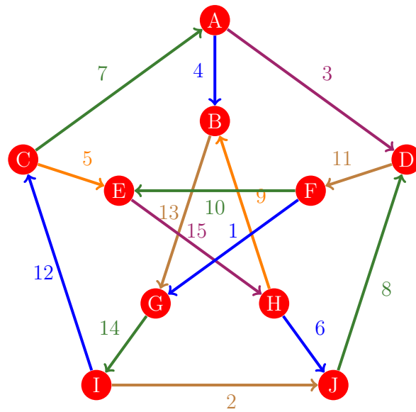
Figura 304: Flujo 296 de la gráfica de Petersen
