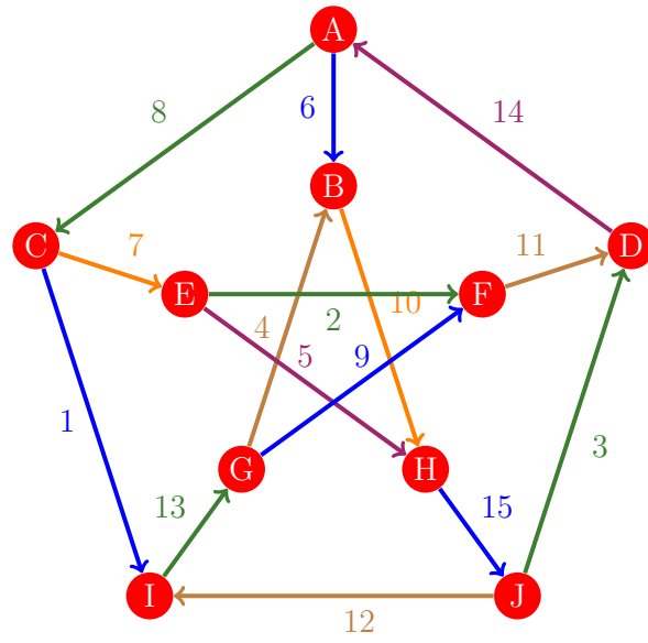
Figura 469: Flujo 461 de la gráfica de Petersen
