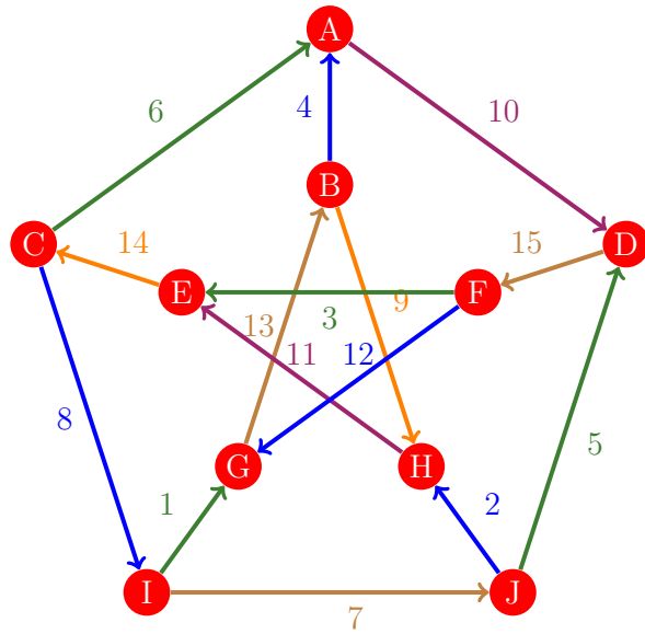
Figura 260: Flujo 252 de la gráfica de Petersen
