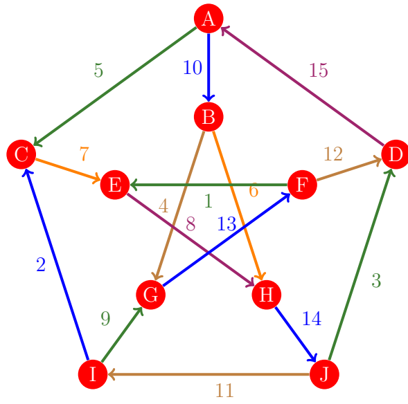
Figura 775: Flujo 767 de la gráfica de Petersen
