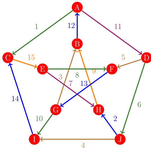
Figura 918: Flujo 910 de la gráfica de Petersen
