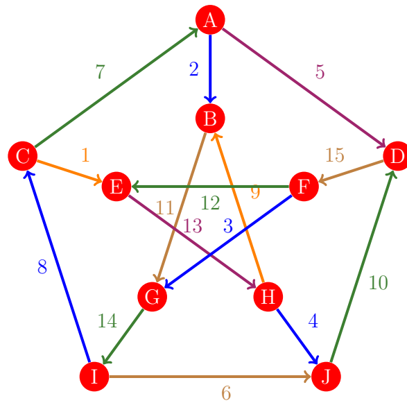
Figura 138: Flujo 130 de la gráfica de Petersen
