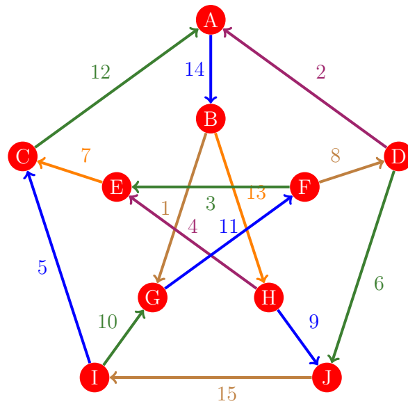
Figura 1120: Flujo 1112 de la gráfica de Petersen
