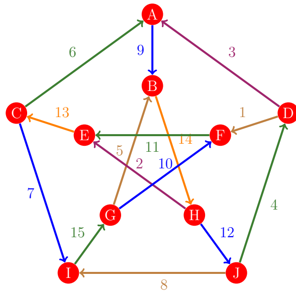
Figura 710: Flujo 702 de la gráfica de Petersen
