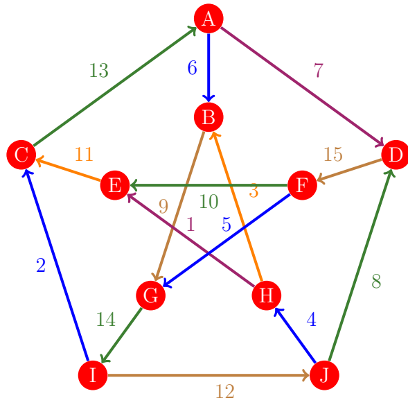
Figura 483: Flujo 475 de la gráfica de Petersen
