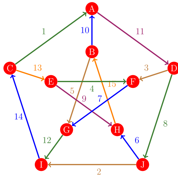
Figura 746: Flujo 738 de la gráfica de Petersen
