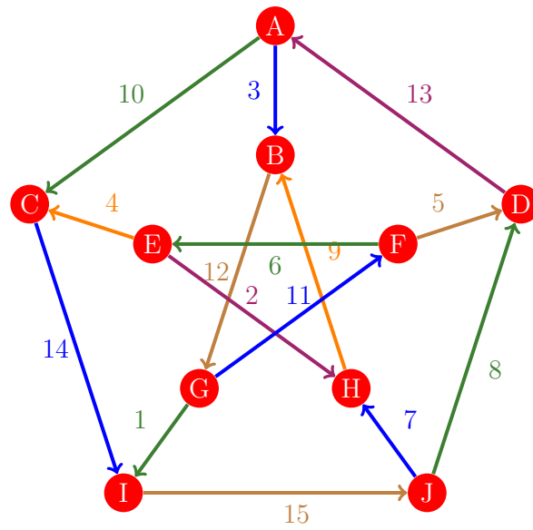
Figura 230: Flujo 222 de la gráfica de Petersen
