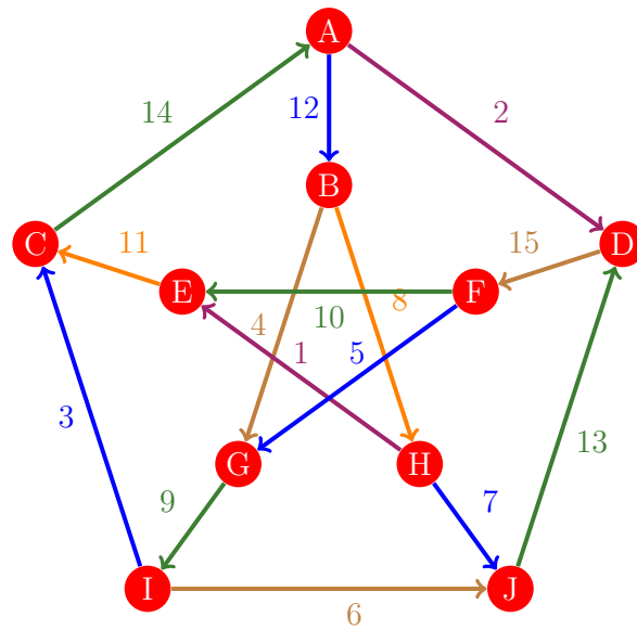
Figura 962: Flujo 954 de la gráfica de Petersen
