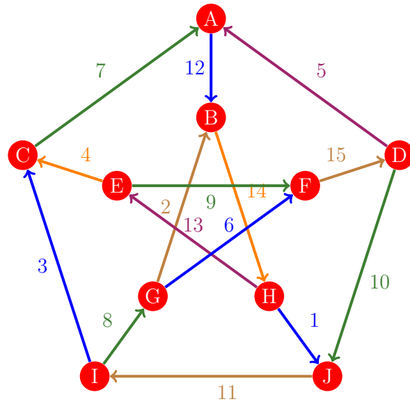
Figura 945: Flujo 937 de la gráfica de Petersen
