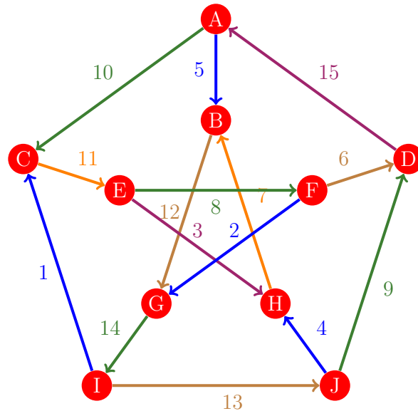
Figura 391: Flujo 383 de la gráfica de Petersen
