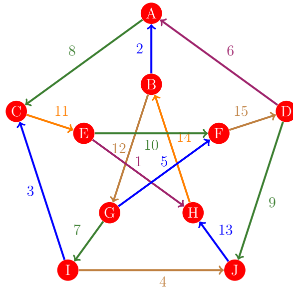
Figura 101: Flujo 93 de la gráfica de Petersen
