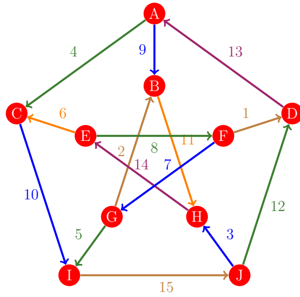
Figura 701: Flujo 693 de la gráfica de Petersen
