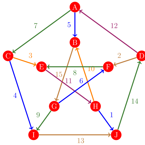
Figura 378: Flujo 370 de la gráfica de Petersen
