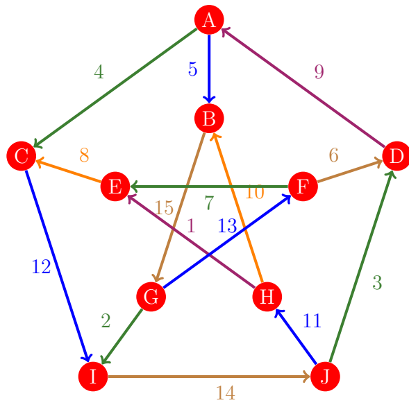
Figura 372: Flujo 364 de la gráfica de Petersen
