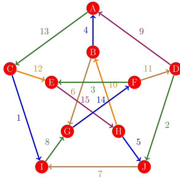
Figura 283: Flujo 275 de la gráfica de Petersen
