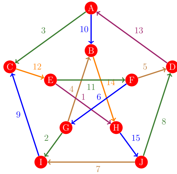
Figura 769: Flujo 761 de la gráfica de Petersen
