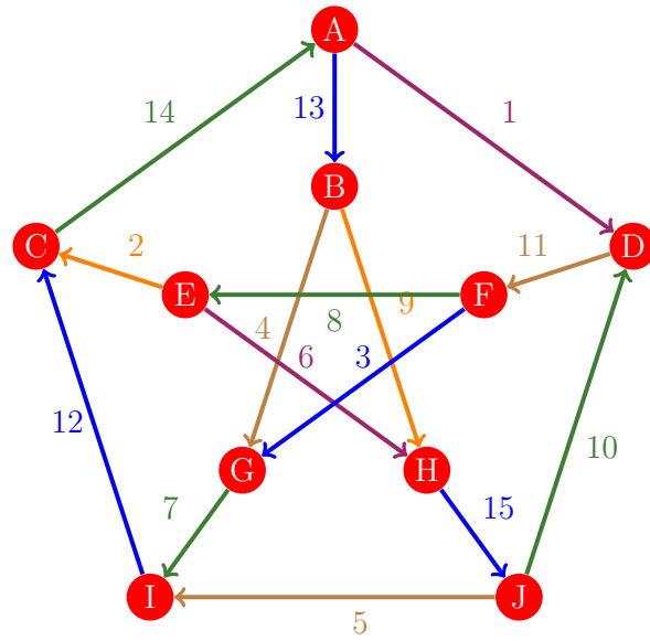
Figura 1045: Flujo 1037 de la gráfica de Petersen
