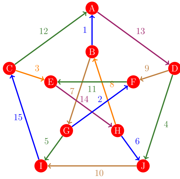
Figura 35: Flujo 27 de la gráfica de Petersen
