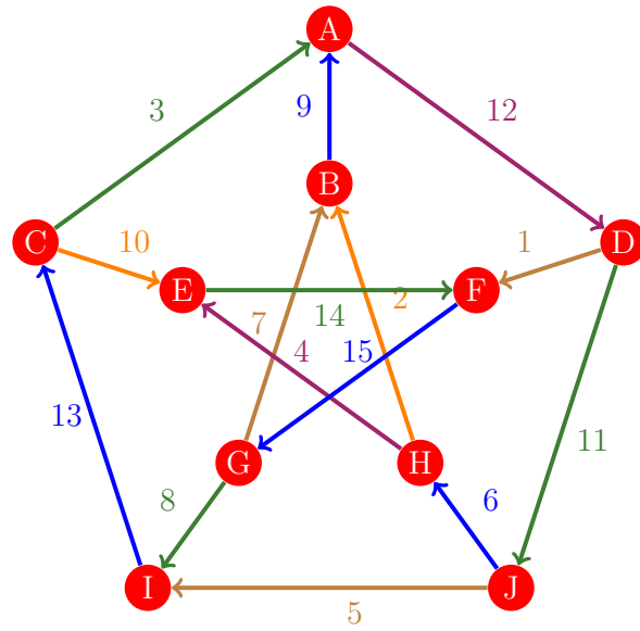
Figura 653: Flujo 645 de la gráfica de Petersen
