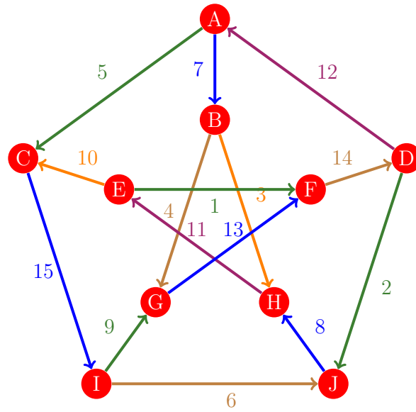
Figura 539: Flujo 531 de la gráfica de Petersen
