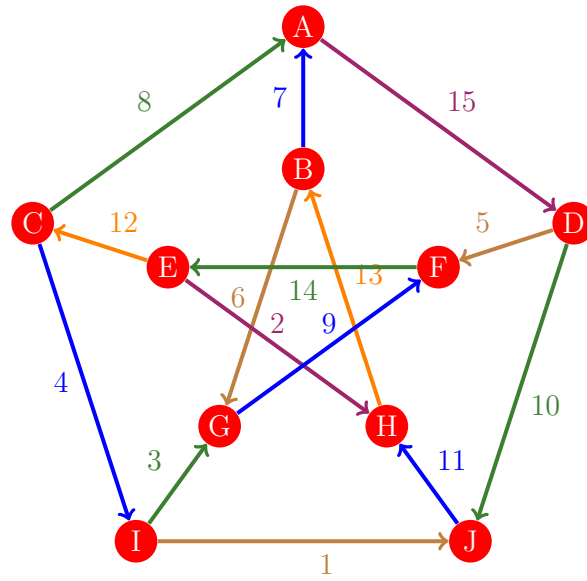
Figura 509: Flujo 501 de la gráfica de Petersen
