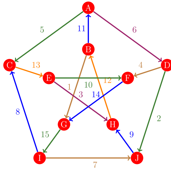
Figura 819: Flujo 811 de la gráfica de Petersen
