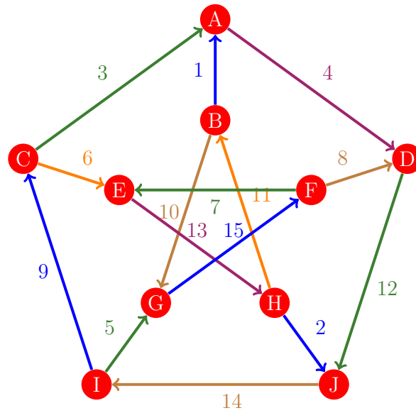
Figura 9: Flujo 1 de la gráfica de Petersen
