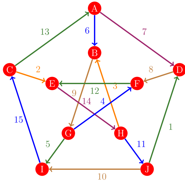
Figura 484: Flujo 476 de la gráfica de Petersen
