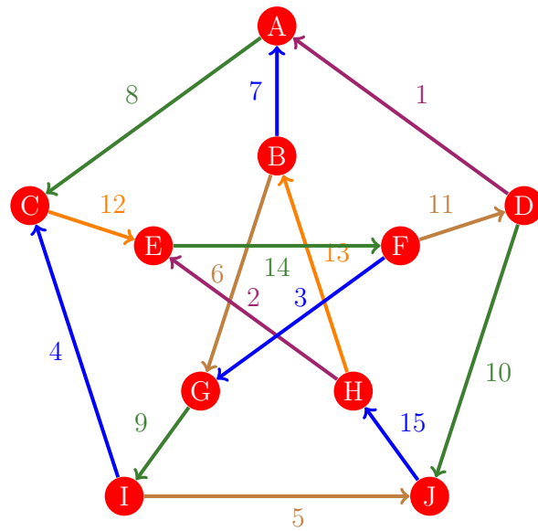
Figura 514: Flujo 506 de la gráfica de Petersen
