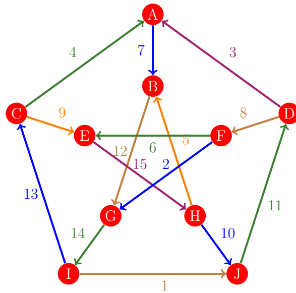
Figura 536: Flujo 528 de la gráfica de Petersen
