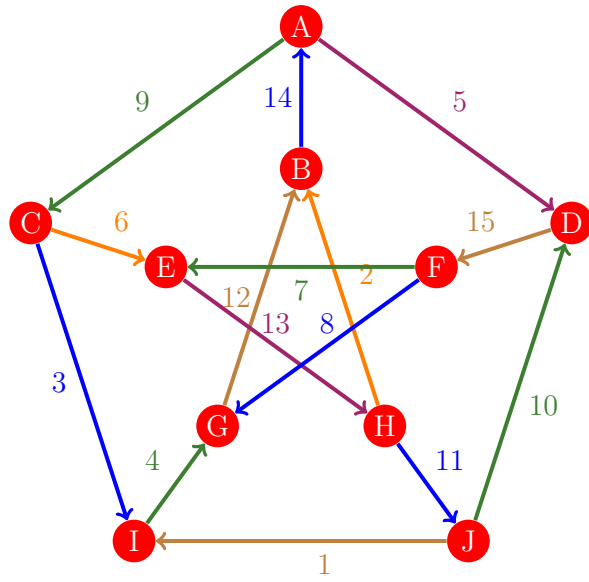
Figura 1068: Flujo 1060 de la gráfica de Petersen
