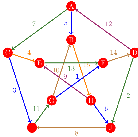
Figura 377: Flujo 369 de la gráfica de Petersen
