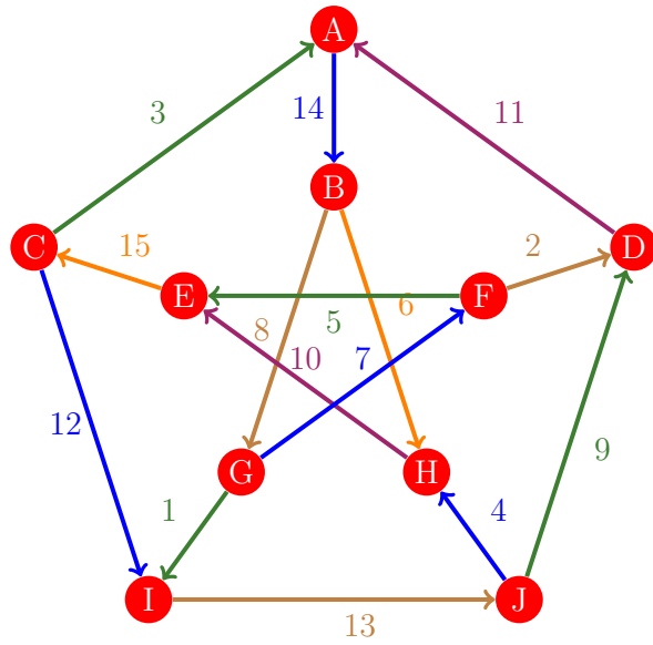
Figura 1096: Flujo 1088 de la gráfica de Petersen
