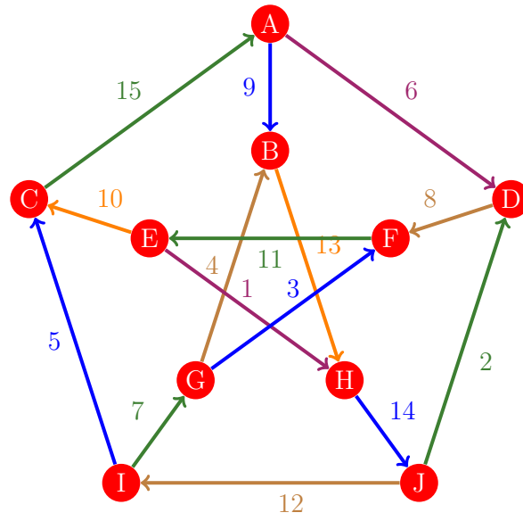
Figura 727: Flujo 719 de la gráfica de Petersen
