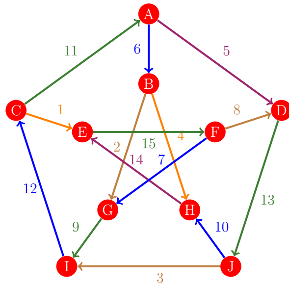
Figura 480: Flujo 472 de la gráfica de Petersen
