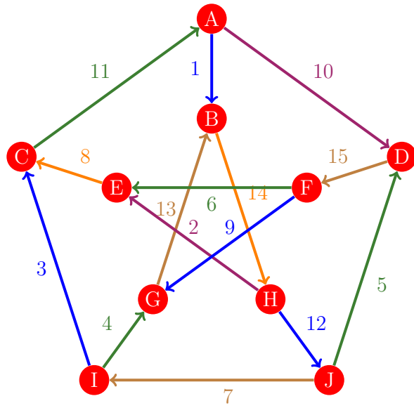
Figura 71: Flujo 63 de la gráfica de Petersen
