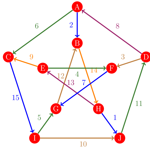
Figura 135: Flujo 127 de la gráfica de Petersen
