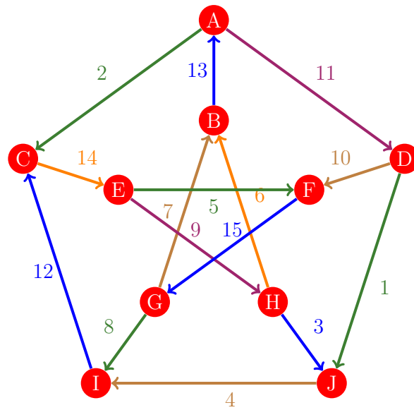
Figura 972: Flujo 964 de la gráfica de Petersen
