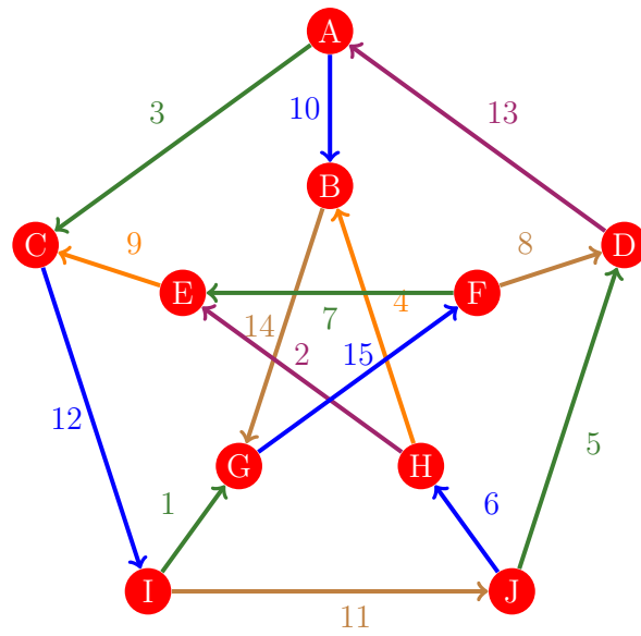
Figura 770: Flujo 762 de la gráfica de Petersen
