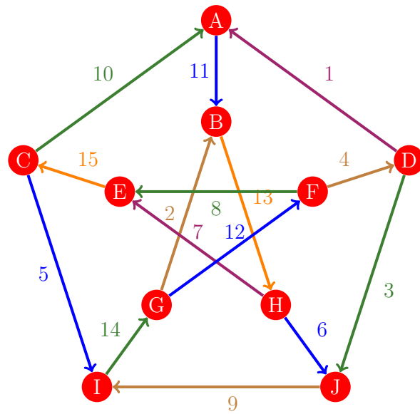
Figura 868: Flujo 860 de la gráfica de Petersen
