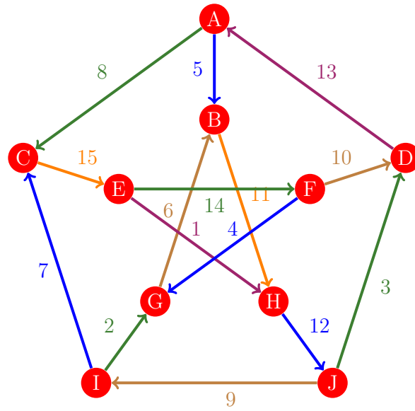
Figura 379: Flujo 371 de la gráfica de Petersen
