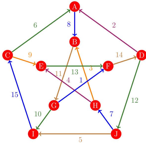
Figura 620: Flujo 612 de la gráfica de Petersen
