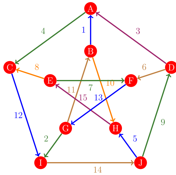
Figura 12: Flujo 4 de la gráfica de Petersen
