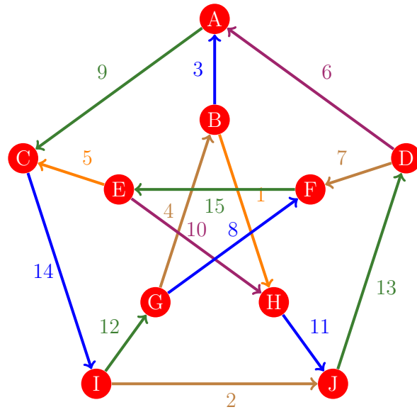
Figura 185: Flujo 177 de la gráfica de Petersen
