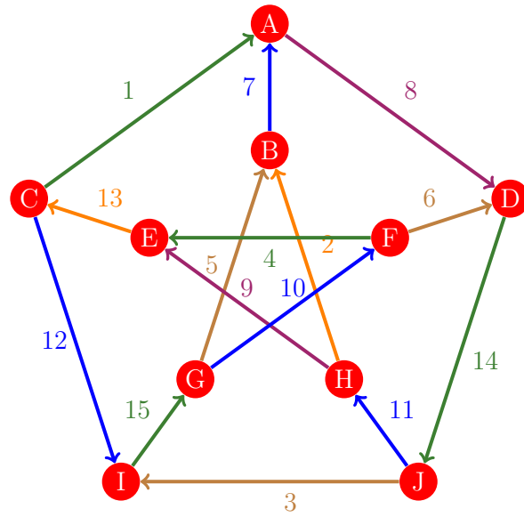
Figura 505: Flujo 497 de la gráfica de Petersen
