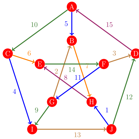
Figura 390: Flujo 382 de la gráfica de Petersen
