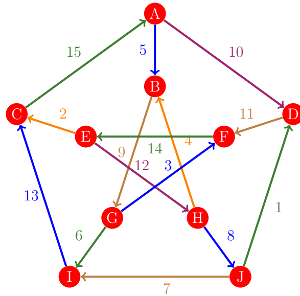
Figura 405: Flujo 397 de la gráfica de Petersen
