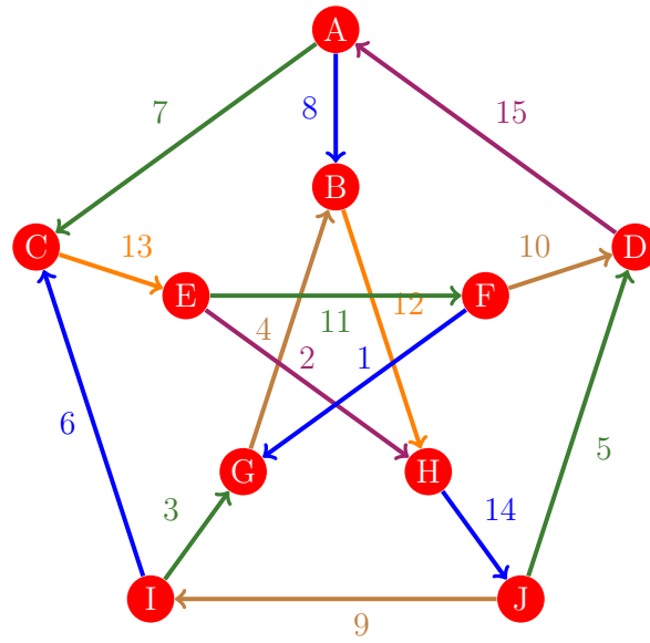
Figura 627: Flujo 619 de la gráfica de Petersen
