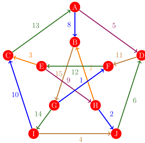
Figura 642: Flujo 634 de la gráfica de Petersen
