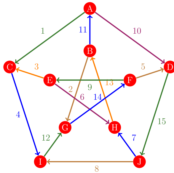
Figura 838: Flujo 830 de la gráfica de Petersen
