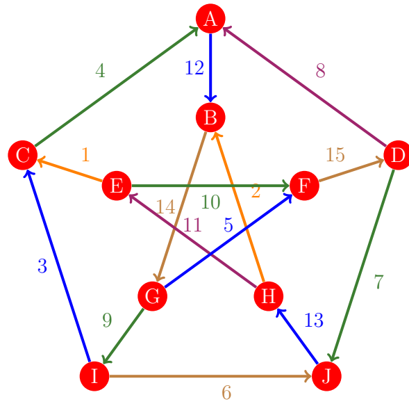
Figura 941: Flujo 933 de la gráfica de Petersen
