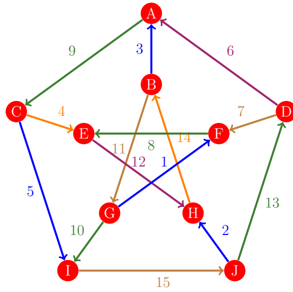
Figura 187: Flujo 179 de la gráfica de Petersen
