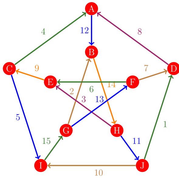
Figura 940: Flujo 932 de la gráfica de Petersen
