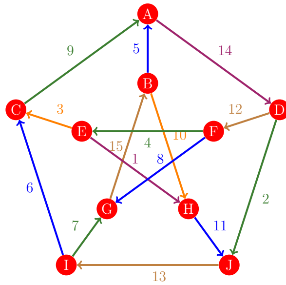
Figura 342: Flujo 334 de la gráfica de Petersen
