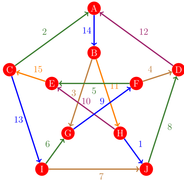
Figura 1092: Flujo 1084 de la gráfica de Petersen
