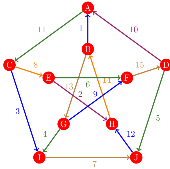
Figura 33: Flujo 25 de la gráfica de Petersen
