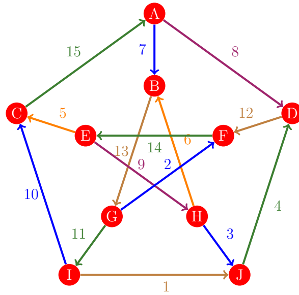
Figura 567: Flujo 559 de la gráfica de Petersen
