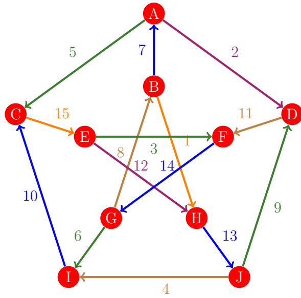
Figura 500: Flujo 492 de la gráfica de Petersen
