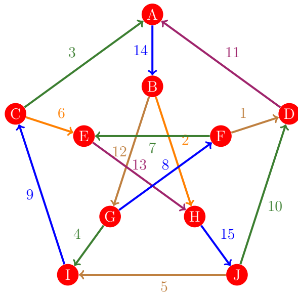
Figura 1098: Flujo 1090 de la gráfica de Petersen
