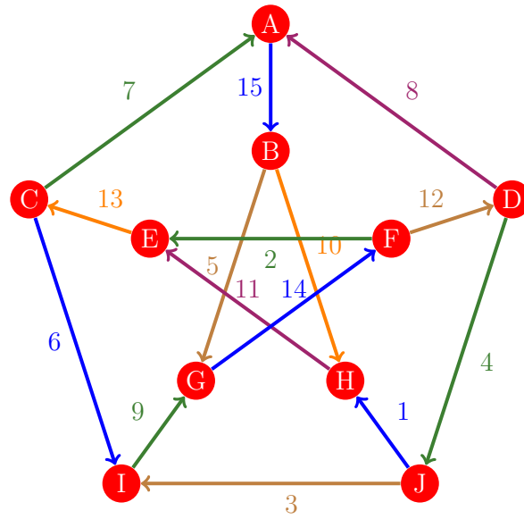
Figura 1183: Flujo 1175 de la gráfica de Petersen
