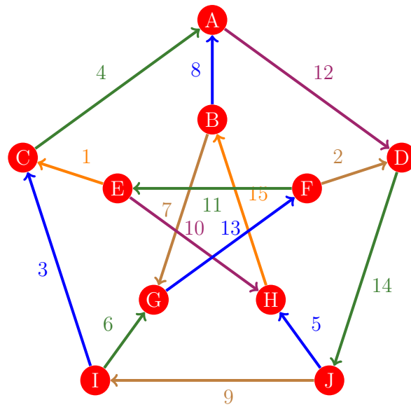
Figura 574: Flujo 566 de la gráfica de Petersen
