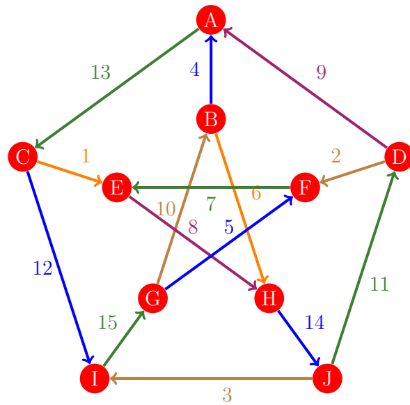
Figura 286: Flujo 278 de la gráfica de Petersen
