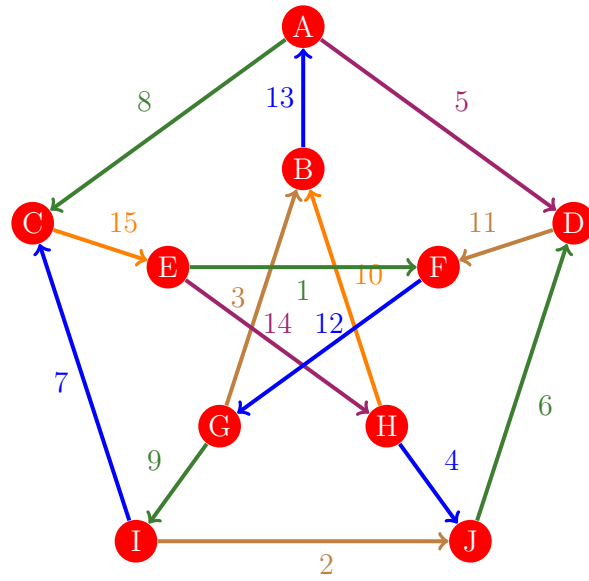
Figura 989: Flujo 981 de la gráfica de Petersen
