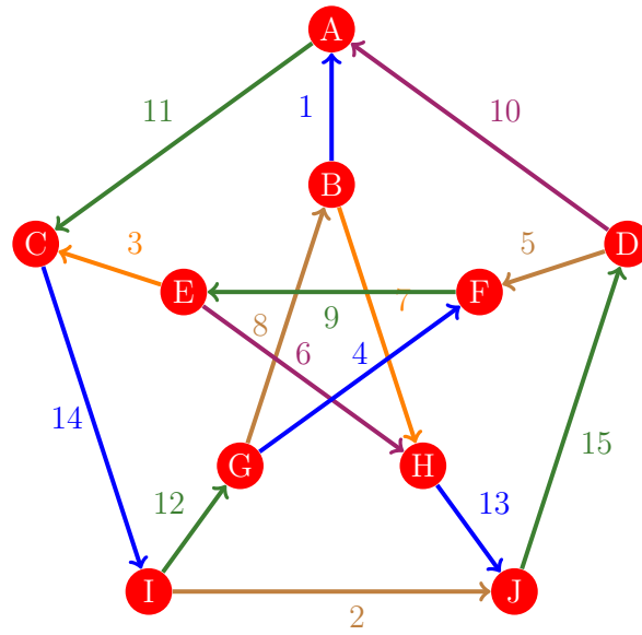
Figura 31: Flujo 23 de la gráfica de Petersen
