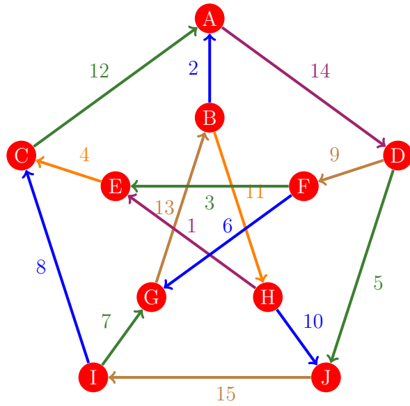
Figura 114: Flujo 106 de la gráfica de Petersen
