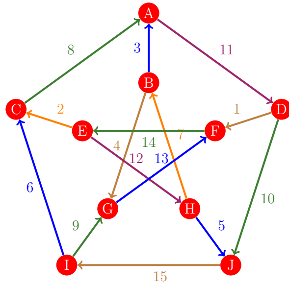
Figura 181: Flujo 173 de la gráfica de Petersen
