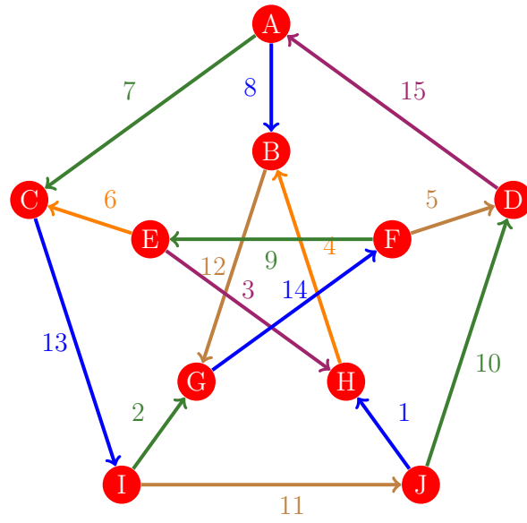
Figura 629: Flujo 621 de la gráfica de Petersen
