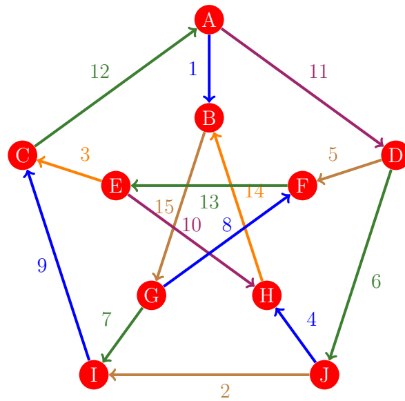
Figura 76: Flujo 68 de la gráfica de Petersen
