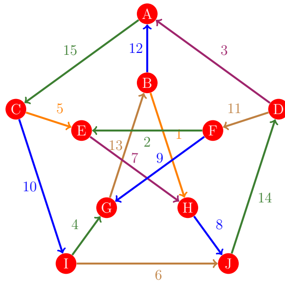
Figura 928: Flujo 920 de la gráfica de Petersen
