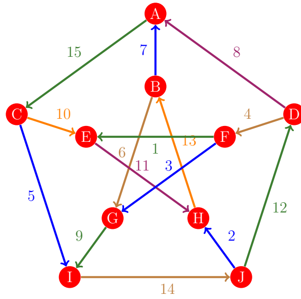
Figura 525: Flujo 517 de la gráfica de Petersen
