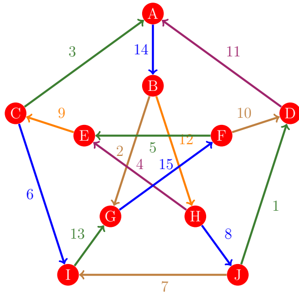
Figura 1097: Flujo 1089 de la gráfica de Petersen
