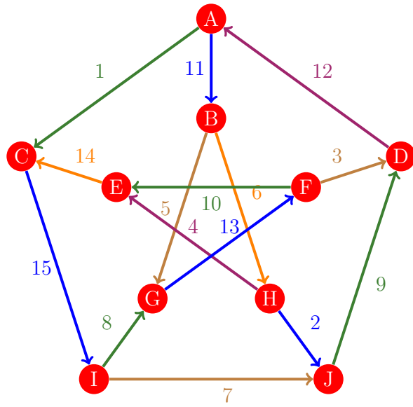
Figura 879: Flujo 871 de la gráfica de Petersen
