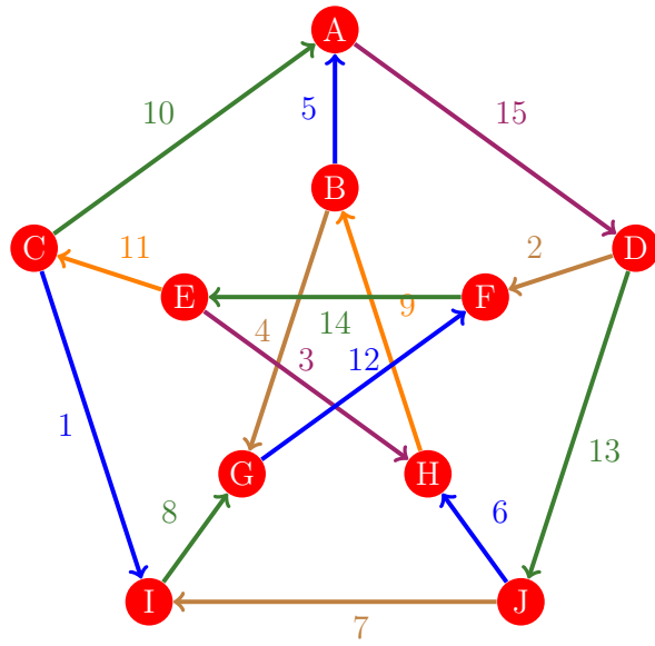
Figura 345: Flujo 337 de la gráfica de Petersen
