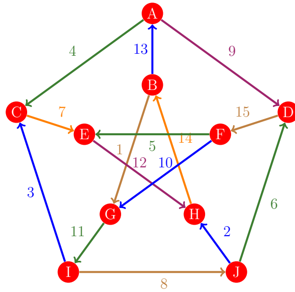
Figura 977: Flujo 969 de la gráfica de Petersen
