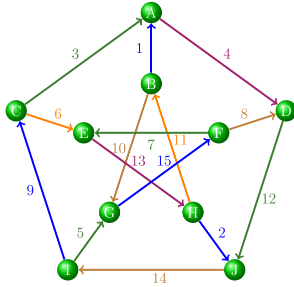
Figura 4: Gráfica de Petersen con flujo elegante.
