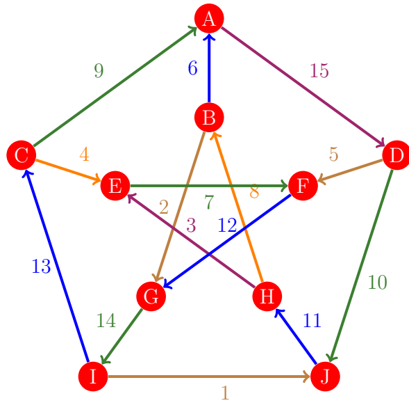
Figura 432: Flujo 424 de la gráfica de Petersen
