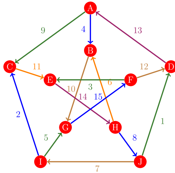
Figura 313: Flujo 305 de la gráfica de Petersen
