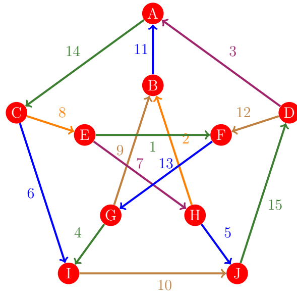
Figura 845: Flujo 837 de la gráfica de Petersen
