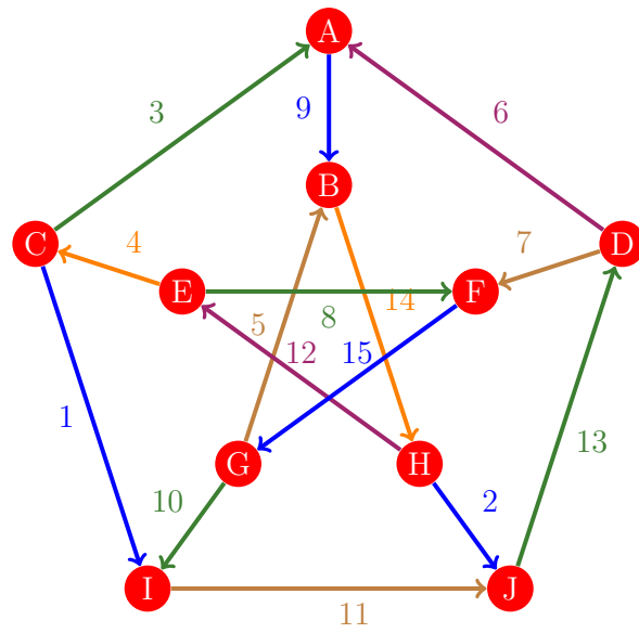
Figura 694: Flujo 686 de la gráfica de Petersen
