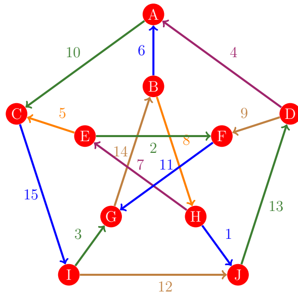
Figura 438: Flujo 430 de la gráfica de Petersen
