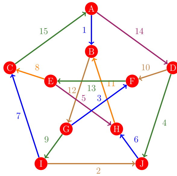
Figura 88: Flujo 80 de la gráfica de Petersen
