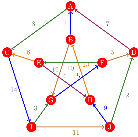
Figura 19: Flujo 11 de la gráfica de Petersen
