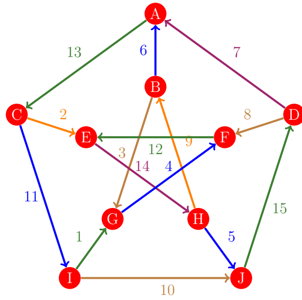
Figura 441: Flujo 433 de la gráfica de Petersen
