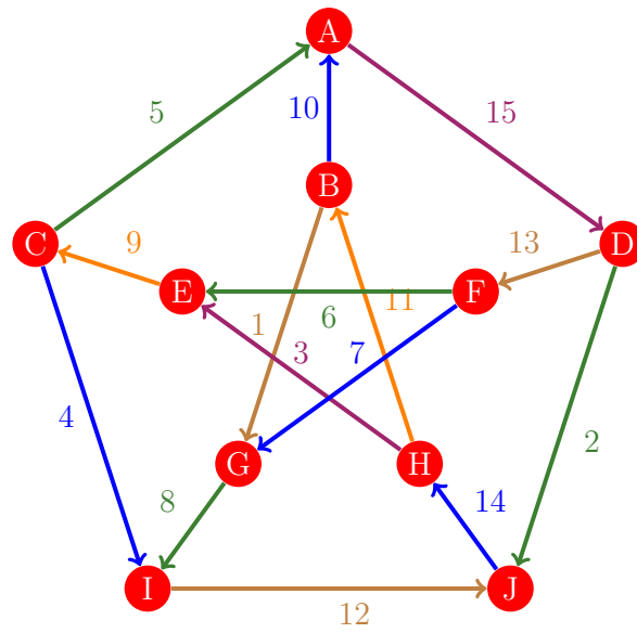
Figura 738: Flujo 730 de la gráfica de Petersen
