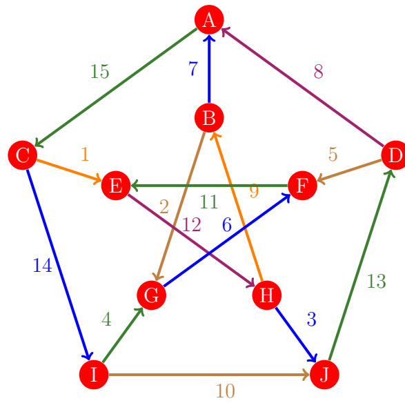
Figura 528: Flujo 520 de la gráfica de Petersen
