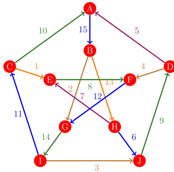
Figura 1198: Flujo 1190 de la gráfica de Petersen
