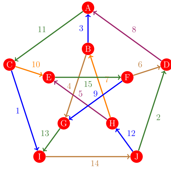
Figura 195: Flujo 187 de la gráfica de Petersen
