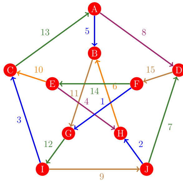
Figura 398: Flujo 390 de la gráfica de Petersen
