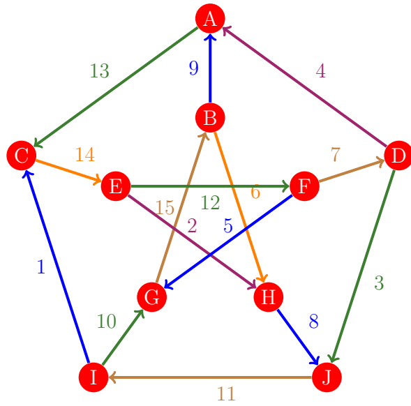
Figura 684: Flujo 676 de la gráfica de Petersen
