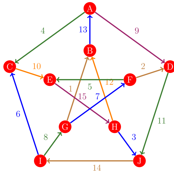
Figura 976: Flujo 968 de la gráfica de Petersen
