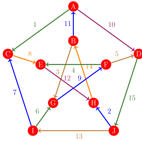
Figura 837: Flujo 829 de la gráfica de Petersen
