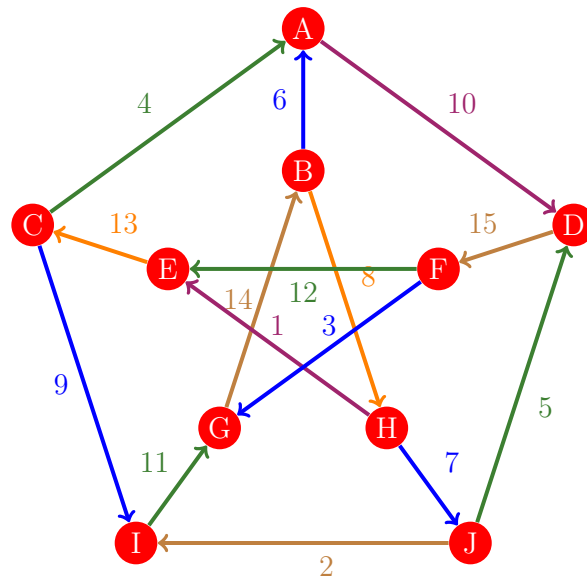
Figura 418: Flujo 410 de la gráfica de Petersen
