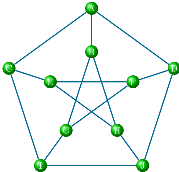
Figura 3: Gráfica de Petersen.
