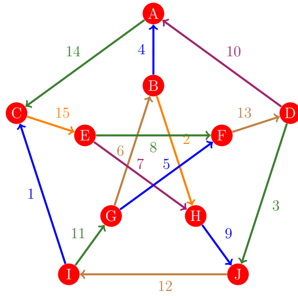
Figura 287: Flujo 279 de la gráfica de Petersen
