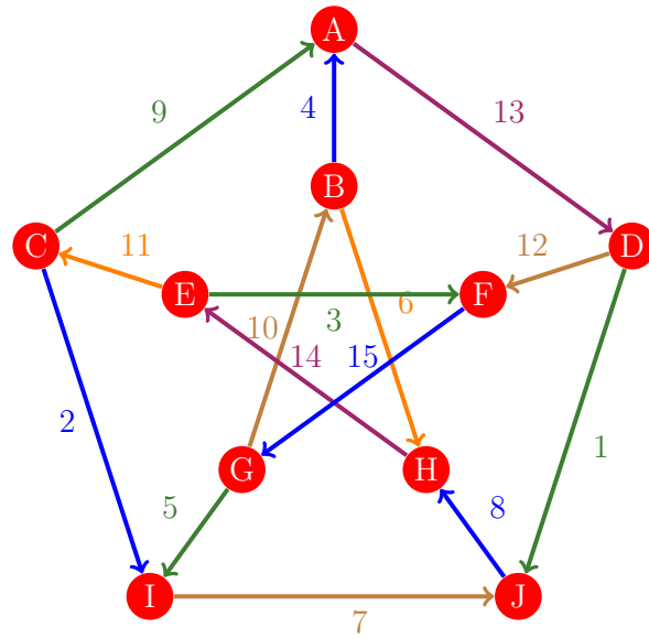
Figura 271: Flujo 263 de la gráfica de Petersen
