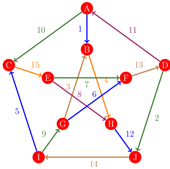
Figura 64: Flujo 56 de la gráfica de Petersen
