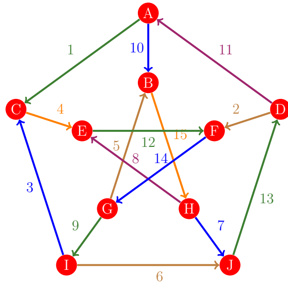
Figura 787: Flujo 779 de la gráfica de Petersen
