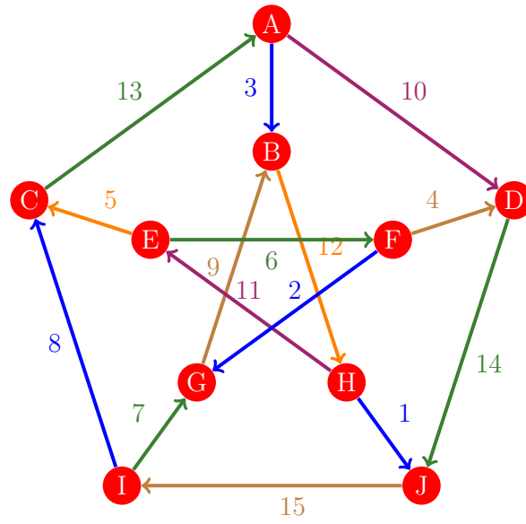
Figura 241: Flujo 233 de la gráfica de Petersen
