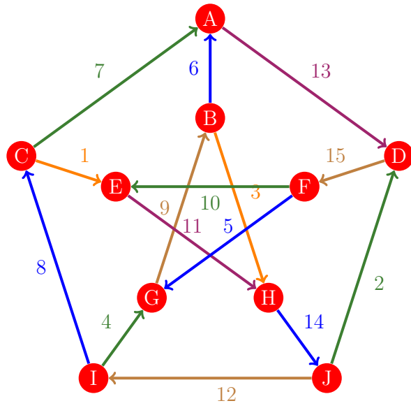
Figura 423: Flujo 415 de la gráfica de Petersen
