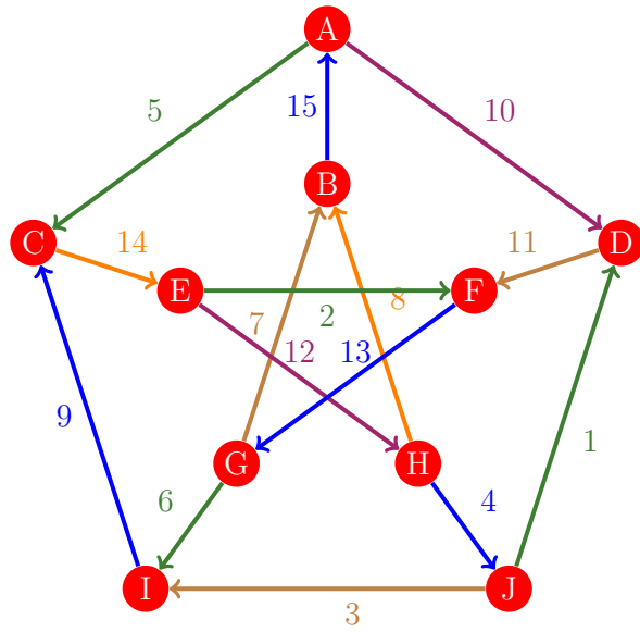
Figura 1135: Flujo 1127 de la gráfica de Petersen
