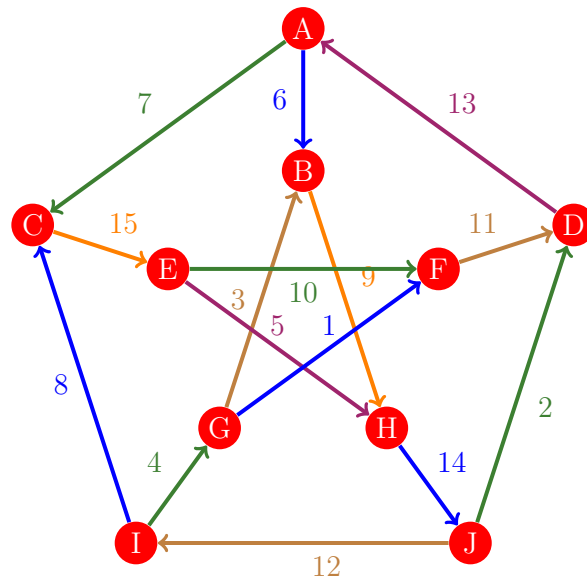
Figura 466: Flujo 458 de la gráfica de Petersen
