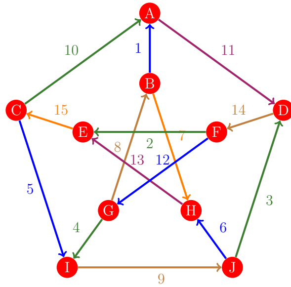
Figura 23: Flujo 15 de la gráfica de Petersen
