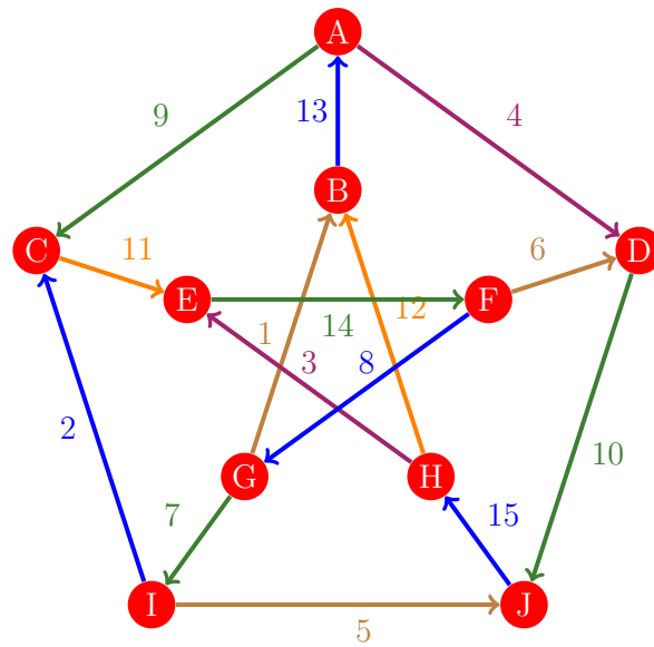
Figura 992: Flujo 984 de la gráfica de Petersen
