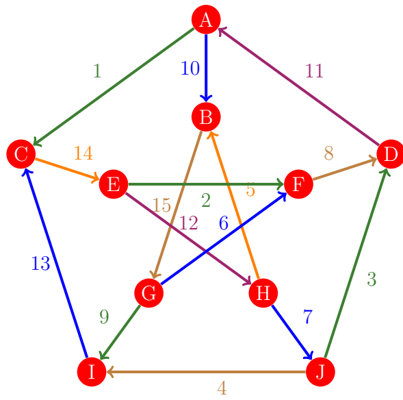
Figura 790: Flujo 782 de la gráfica de Petersen
