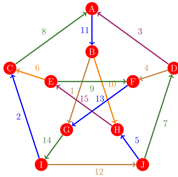
Figura 864: Flujo 856 de la gráfica de Petersen
