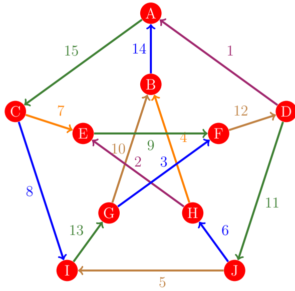
Figura 1088: Flujo 1080 de la gráfica de Petersen
