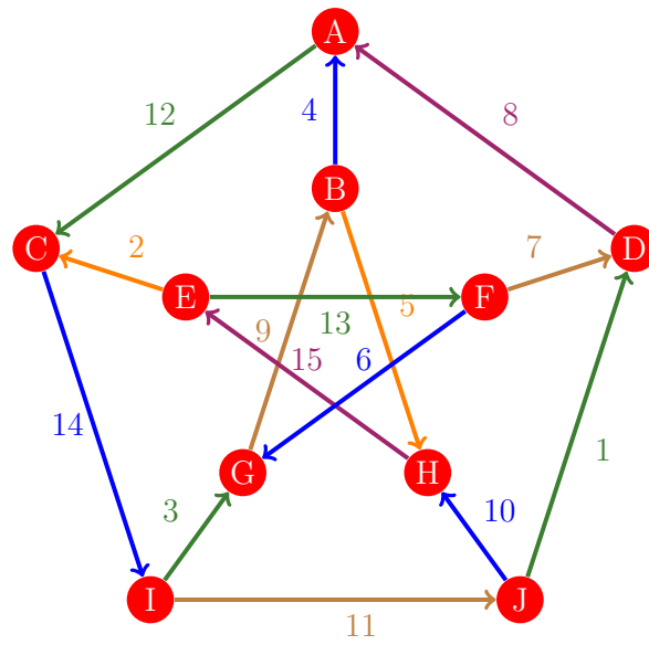
Figura 282: Flujo 274 de la gráfica de Petersen
