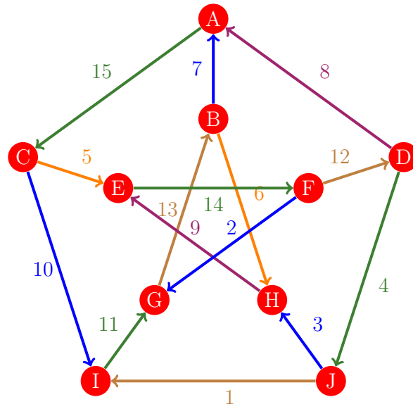
Figura 527: Flujo 519 de la gráfica de Petersen
