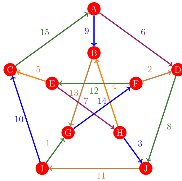
Figura 728: Flujo 720 de la gráfica de Petersen
