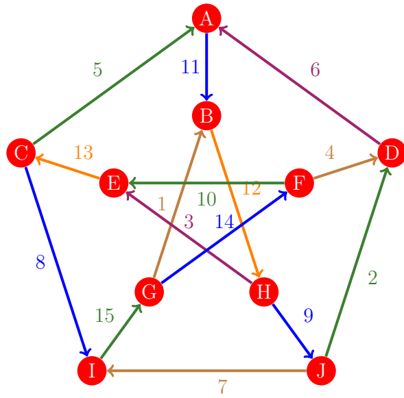
Figura 859: Flujo 851 de la gráfica de Petersen
