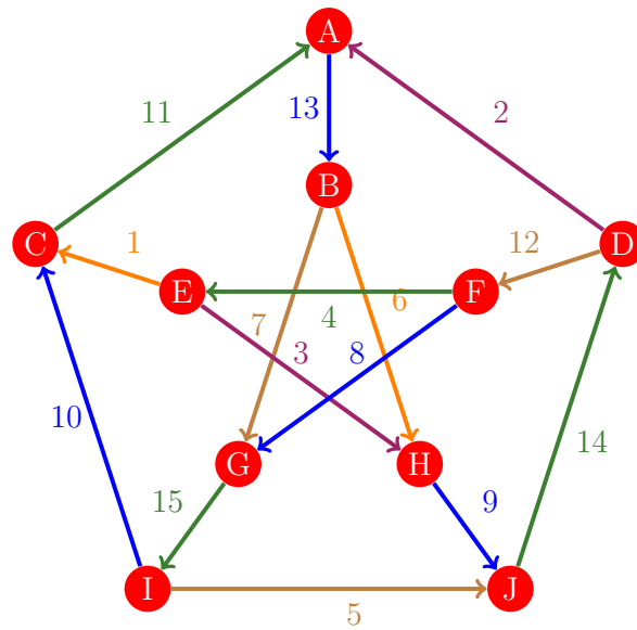
Figura 1038: Flujo 1030 de la gráfica de Petersen
