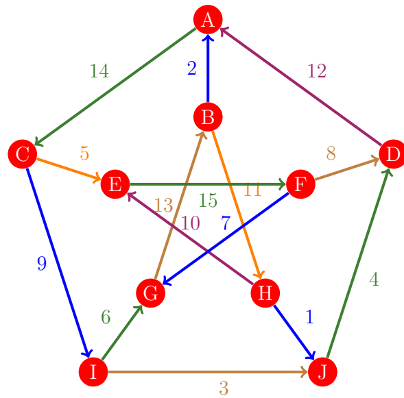
Figura 124: Flujo 116 de la gráfica de Petersen
