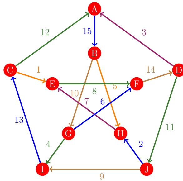
Figura 1202: Flujo 1194 de la gráfica de Petersen
