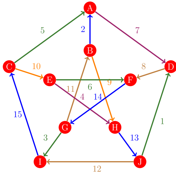
Figura 92: Flujo 84 de la gráfica de Petersen
