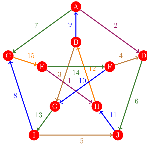
Figura 675: Flujo 667 de la gráfica de Petersen
