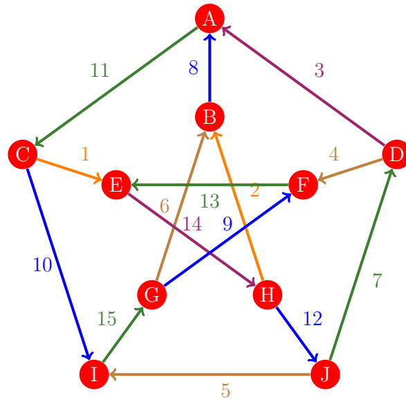
Figura 595: Flujo 587 de la gráfica de Petersen
