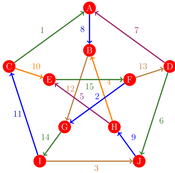
Figura 633: Flujo 625 de la gráfica de Petersen
