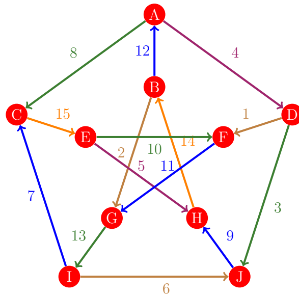
Figura 908: Flujo 900 de la gráfica de Petersen
