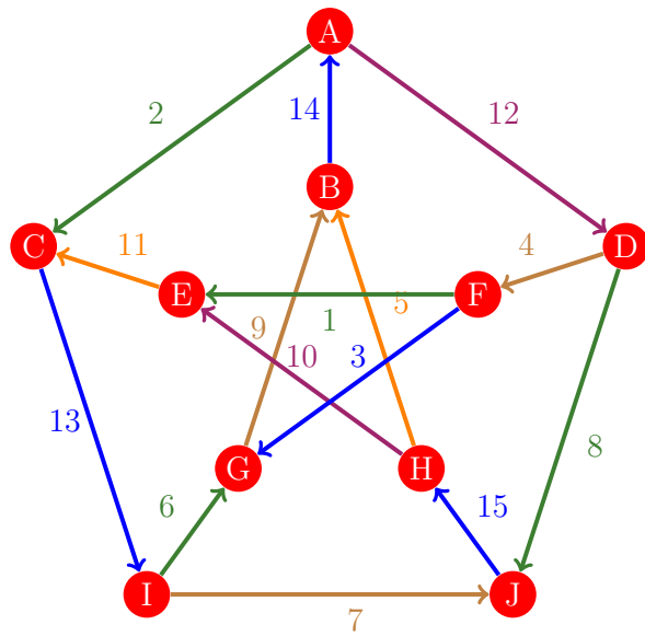
Figura 1050: Flujo 1042 de la gráfica de Petersen
