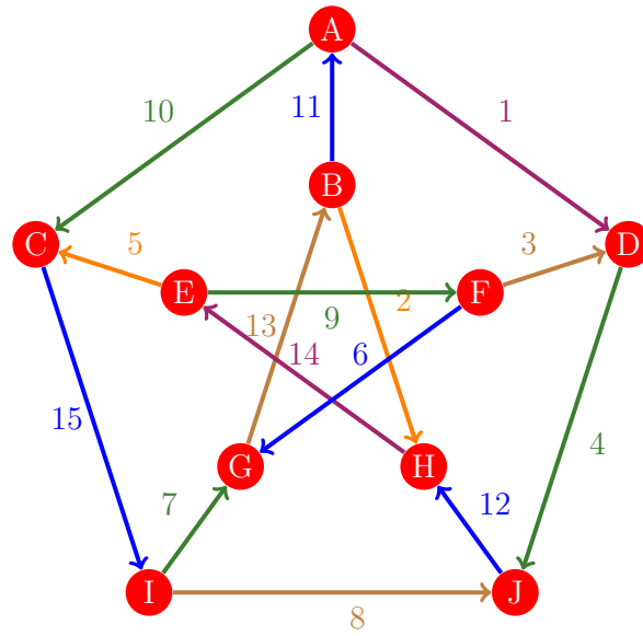
Figura 831: Flujo 823 de la gráfica de Petersen
