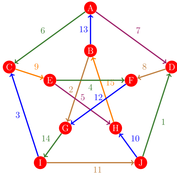
Figura 982: Flujo 974 de la gráfica de Petersen
