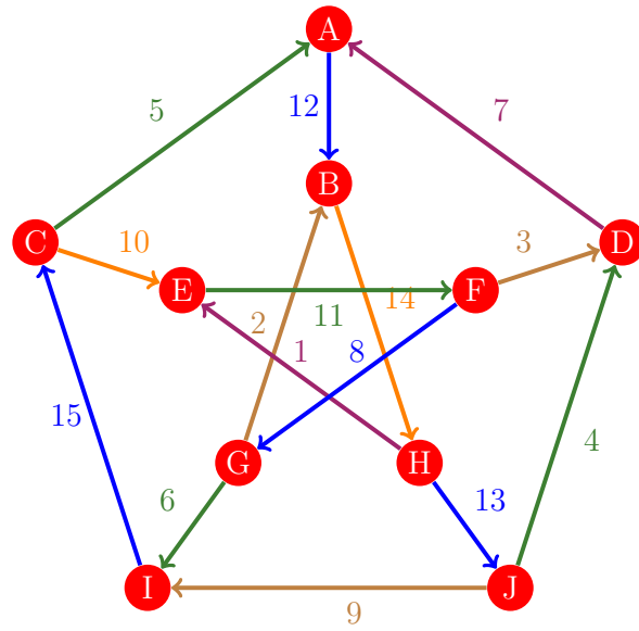
Figura 943: Flujo 935 de la gráfica de Petersen
