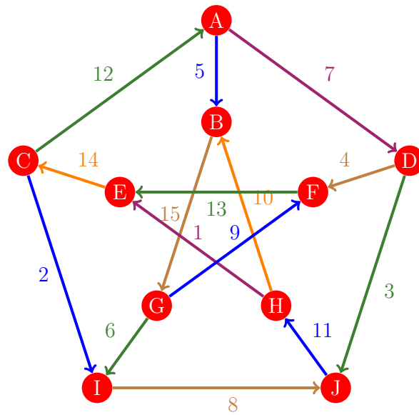
Figura 396: Flujo 388 de la gráfica de Petersen
