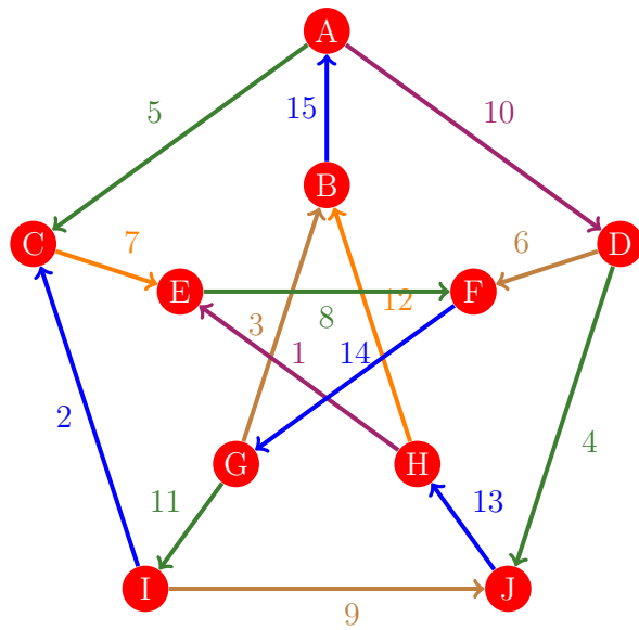
Figura 1138: Flujo 1130 de la gráfica de Petersen
