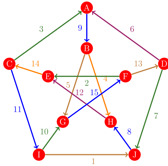
Figura 695: Flujo 687 de la gráfica de Petersen
