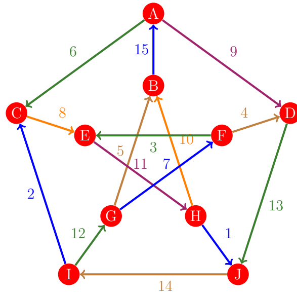
Figura 1141: Flujo 1133 de la gráfica de Petersen
