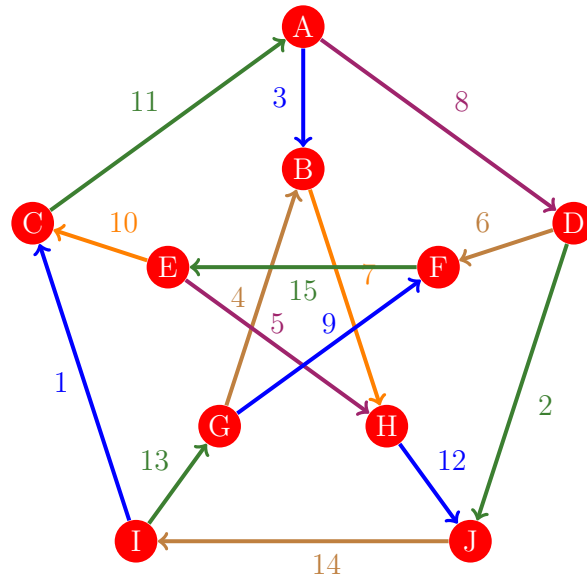
Figura 231: Flujo 223 de la gráfica de Petersen
