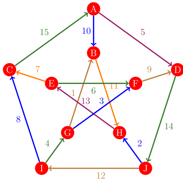
Figura 804: Flujo 796 de la gráfica de Petersen
