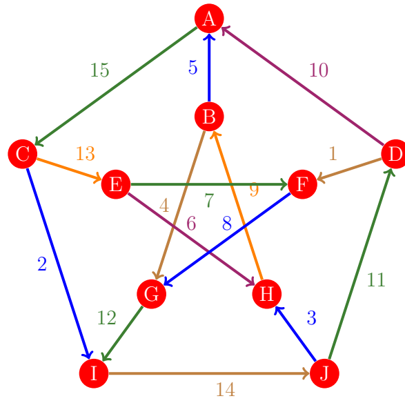
Figura 361: Flujo 353 de la gráfica de Petersen
