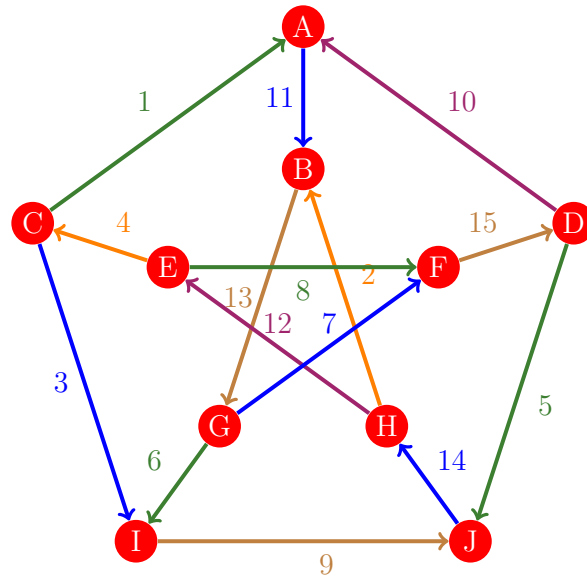
Figura 877: Flujo 869 de la gráfica de Petersen
