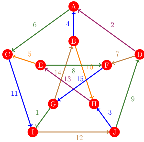
Figura 262: Flujo 254 de la gráfica de Petersen
