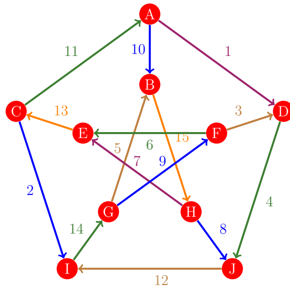
Figura 792: Flujo 784 de la gráfica de Petersen
