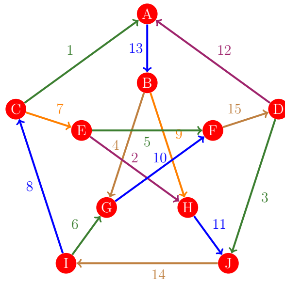
Figura 1041: Flujo 1033 de la gráfica de Petersen
