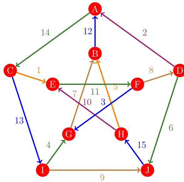
Figura 924: Flujo 916 de la gráfica de Petersen
