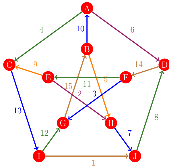
Figura 734: Flujo 726 de la gráfica de Petersen
