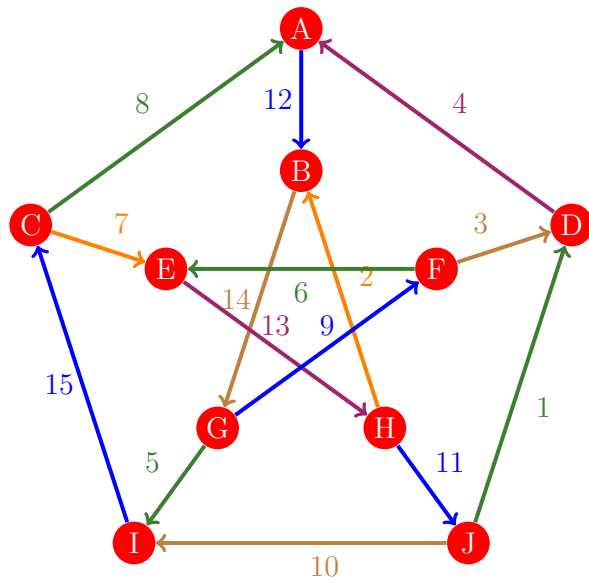
Figura 950: Flujo 942 de la gráfica de Petersen
