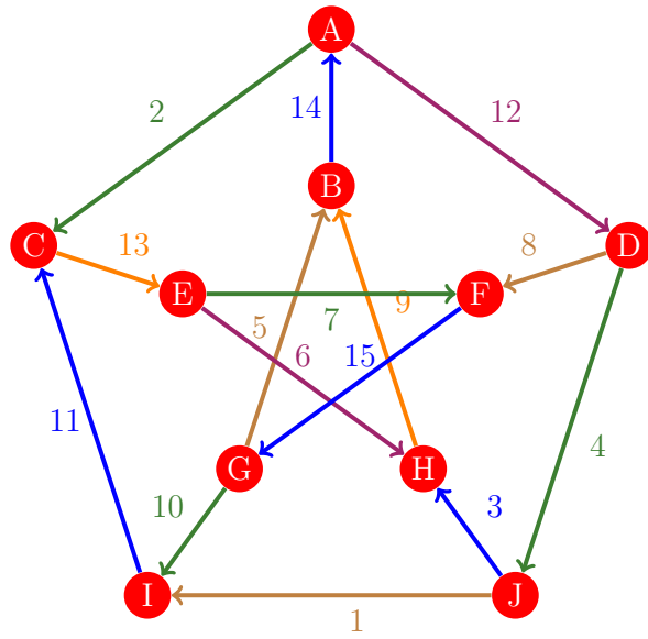
Figura 1049: Flujo 1041 de la gráfica de Petersen
