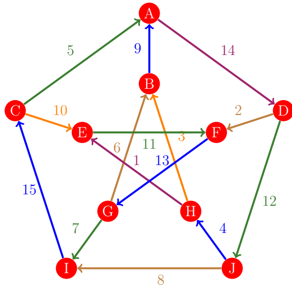
Figura 665: Flujo 657 de la gráfica de Petersen
