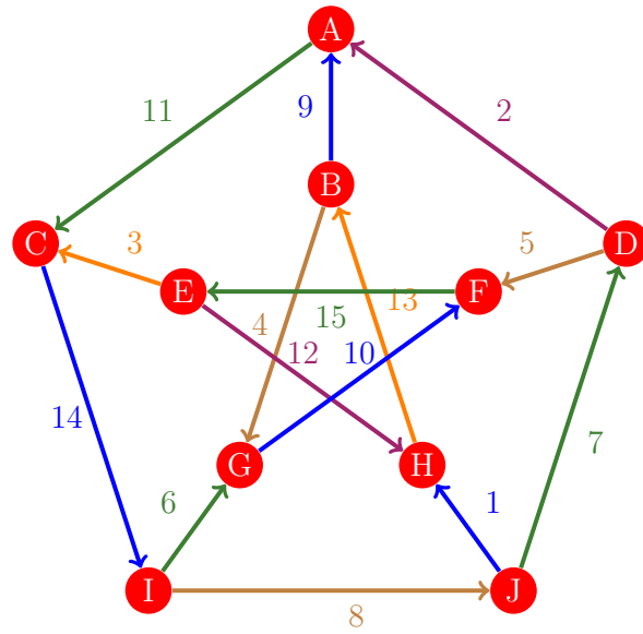
Figura 677: Flujo 669 de la gráfica de Petersen
