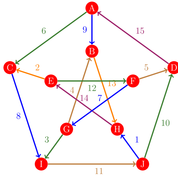
Figura 713: Flujo 705 de la gráfica de Petersen
