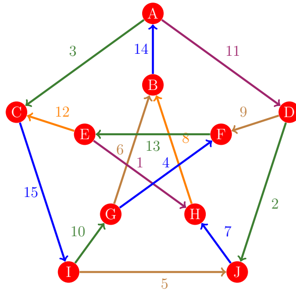
Figura 1055: Flujo 1047 de la gráfica de Petersen
