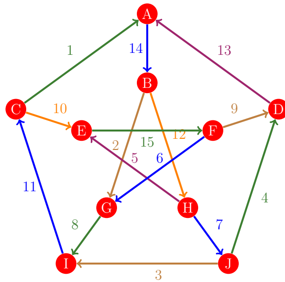
Figura 1124: Flujo 1116 de la gráfica de Petersen
