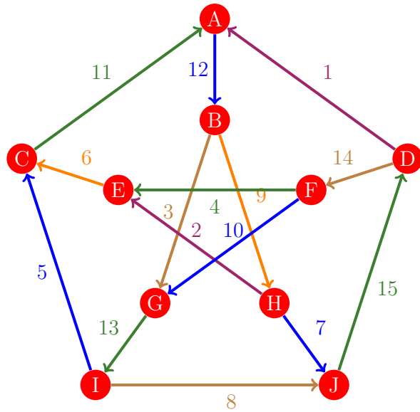
Figura 954: Flujo 946 de la gráfica de Petersen
