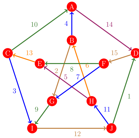
Figura 276: Flujo 268 de la gráfica de Petersen
