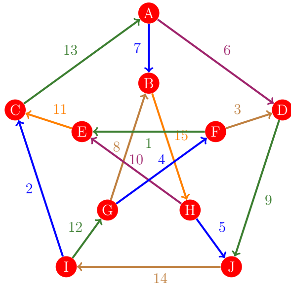
Figura 562: Flujo 554 de la gráfica de Petersen
