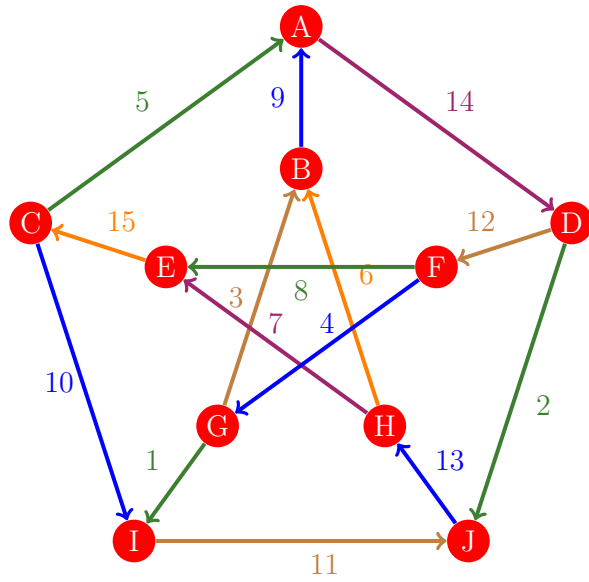
Figura 666: Flujo 658 de la gráfica de Petersen
