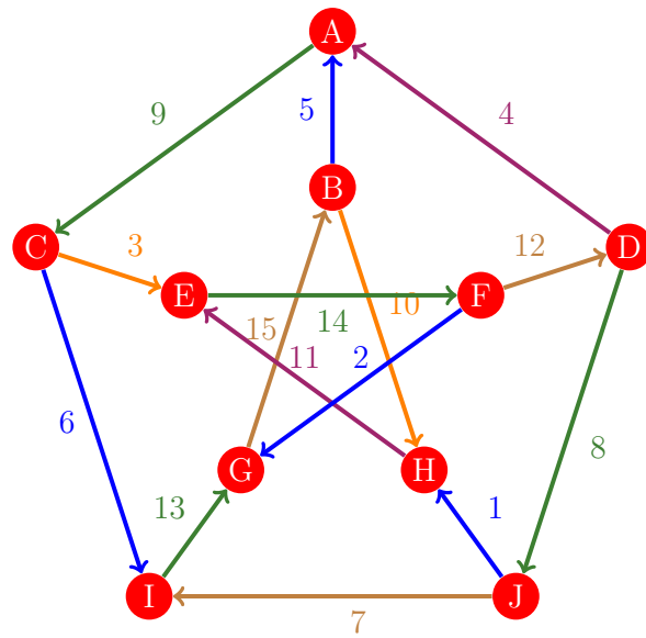
Figura 344: Flujo 336 de la gráfica de Petersen
