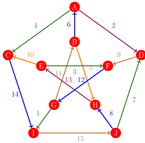
Figura 420: Flujo 412 de la gráfica de Petersen
