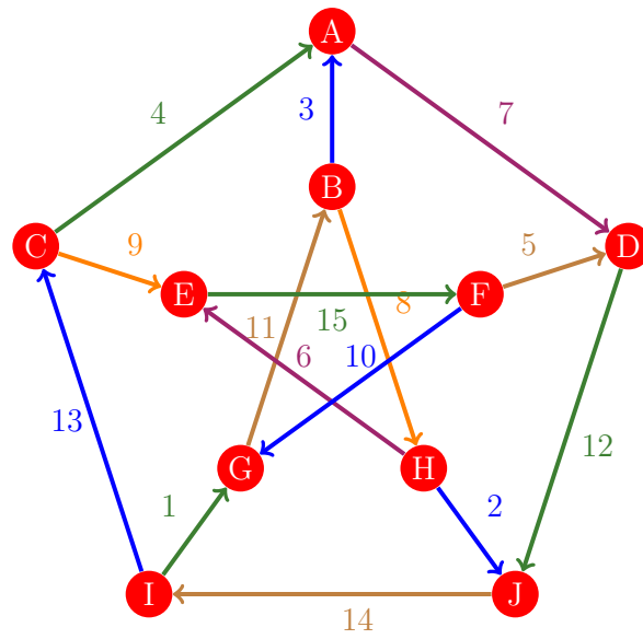
Figura 172: Flujo 164 de la gráfica de Petersen
