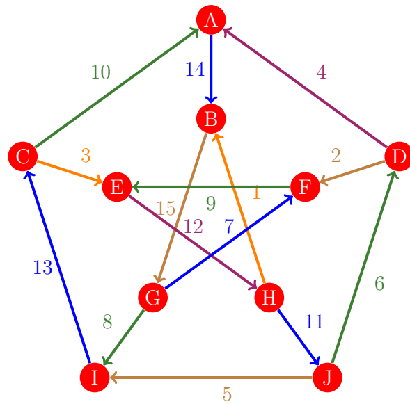
Figura 1110: Flujo 1102 de la gráfica de Petersen
