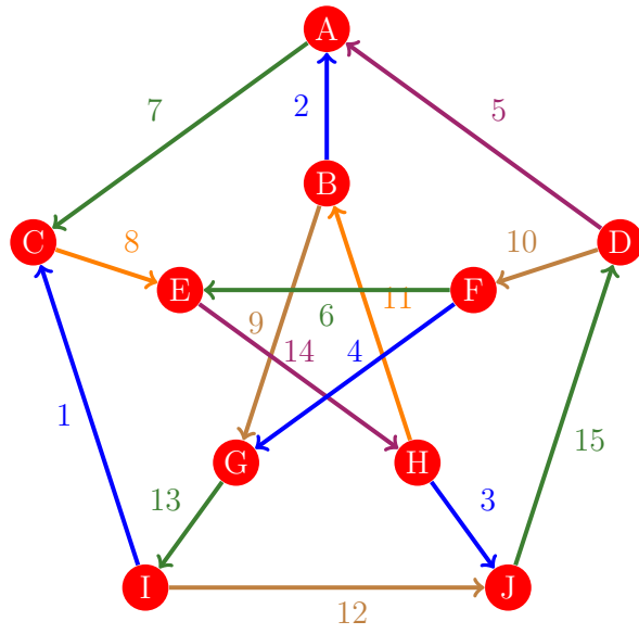
Figura 99: Flujo 91 de la gráfica de Petersen
