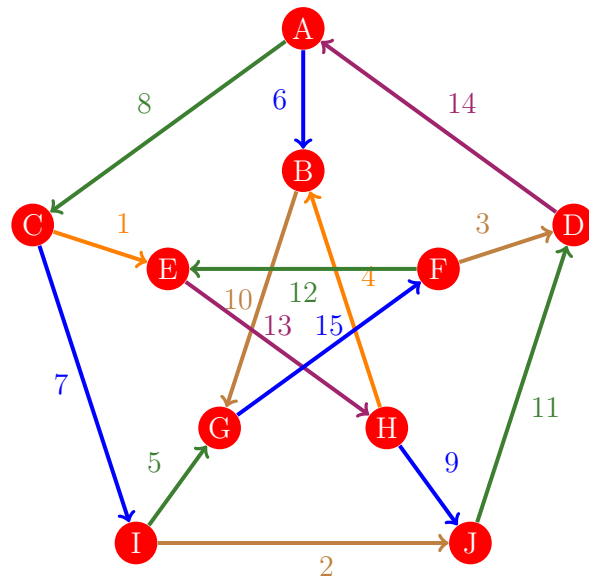
Figura 470: Flujo 462 de la gráfica de Petersen
