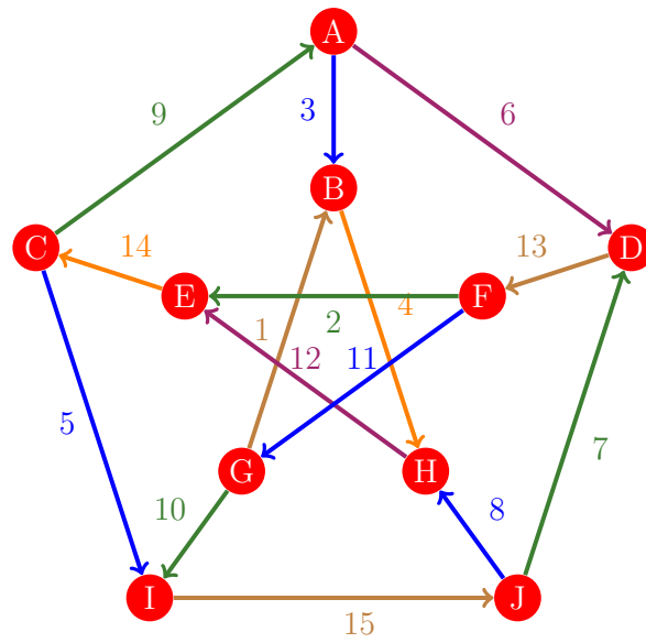
Figura 224: Flujo 216 de la gráfica de Petersen
