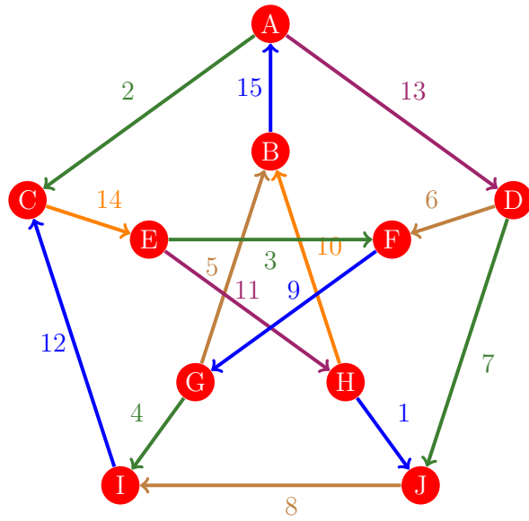
Figura 1129: Flujo 1121 de la gráfica de Petersen
