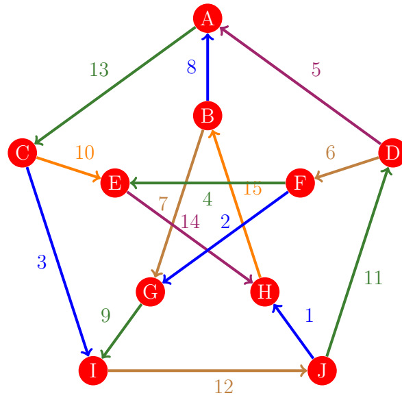
Figura 601: Flujo 593 de la gráfica de Petersen
