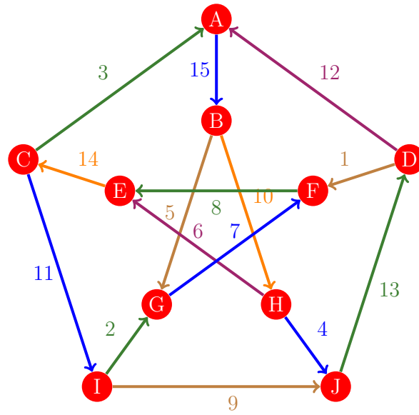
Figura 1171: Flujo 1163 de la gráfica de Petersen
