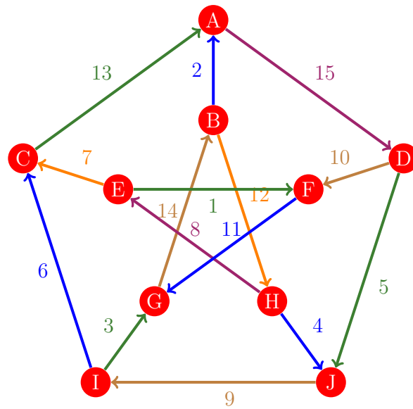
Figura 118: Flujo 110 de la gráfica de Petersen
