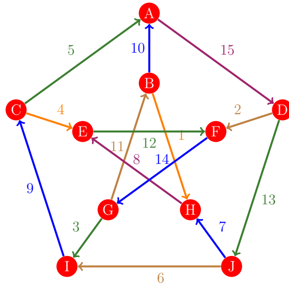
Figura 741: Flujo 733 de la gráfica de Petersen
