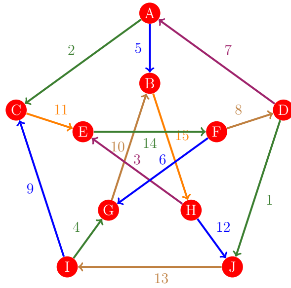
Figura 369: Flujo 361 de la gráfica de Petersen
