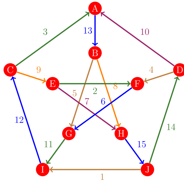
Figura 1013: Flujo 1005 de la gráfica de Petersen
