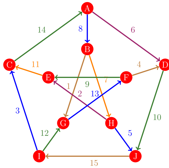
Figura 644: Flujo 636 de la gráfica de Petersen
