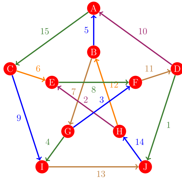
Figura 363: Flujo 355 de la gráfica de Petersen
