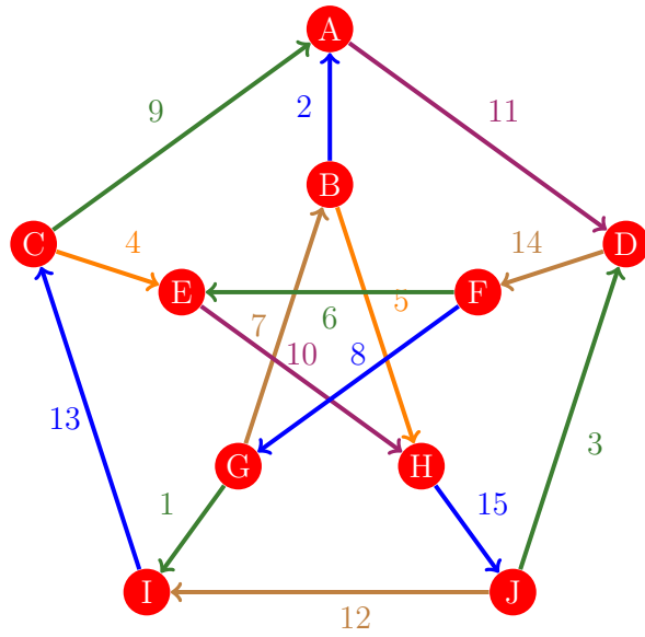
Figura 104: Flujo 96 de la gráfica de Petersen
