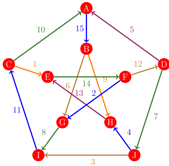
Figura 1194: Flujo 1186 de la gráfica de Petersen
