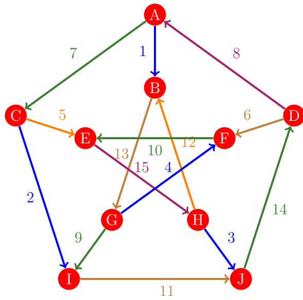
Figura 56: Flujo 48 de la gráfica de Petersen
