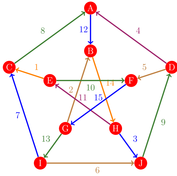
Figura 947: Flujo 939 de la gráfica de Petersen
