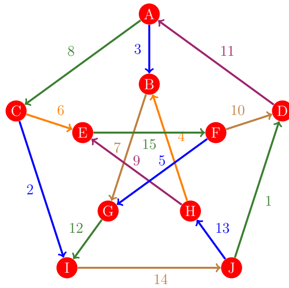
Figura 222: Flujo 214 de la gráfica de Petersen
