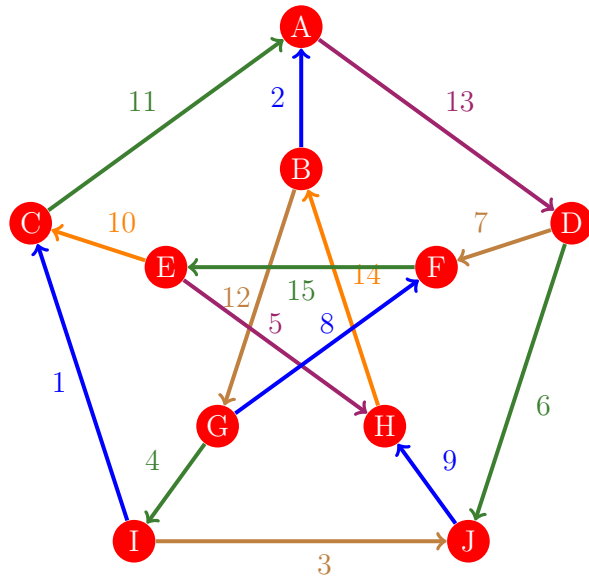
Figura 107: Flujo 99 de la gráfica de Petersen
