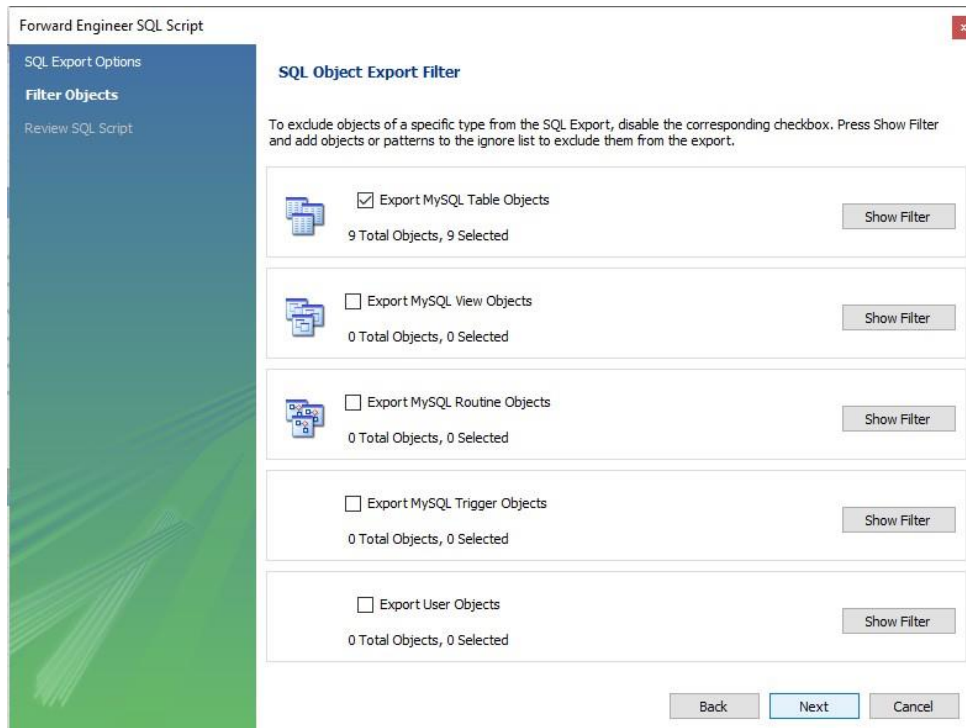
Figura 11. Generación de script parte uno.
