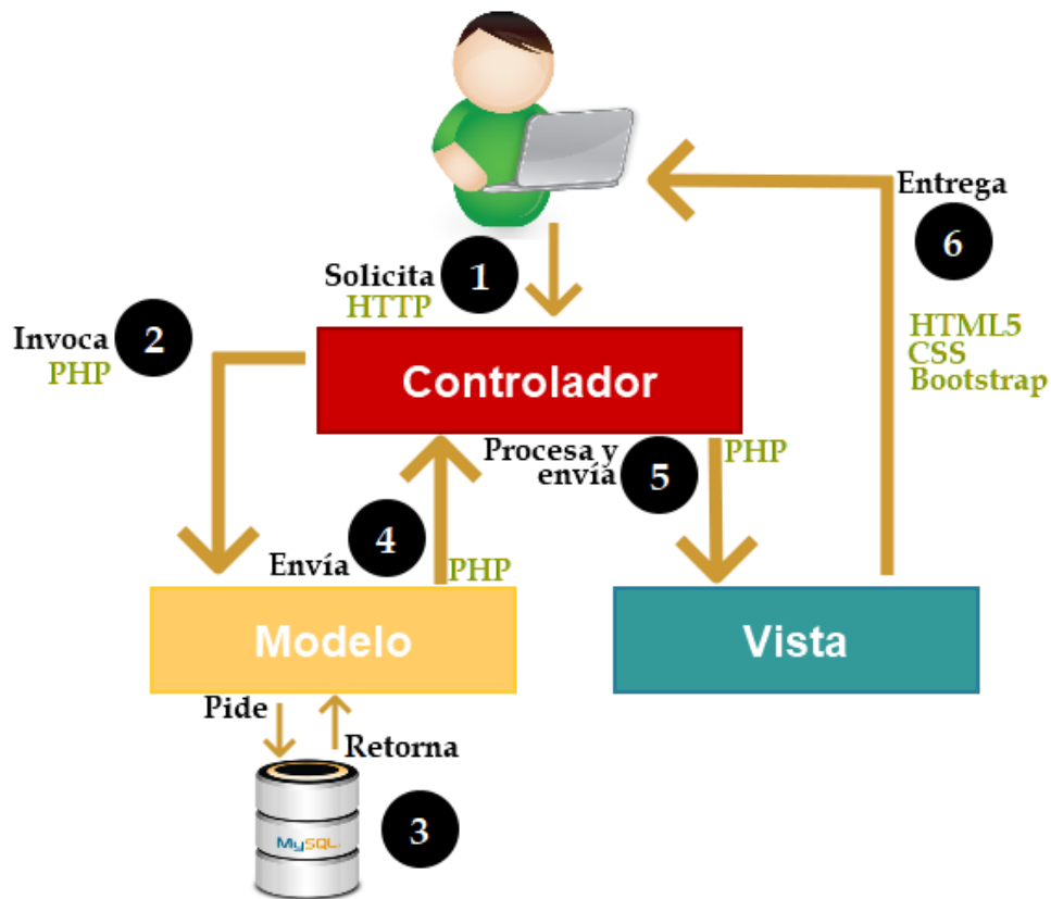
Figura 4. Patrón Modelo Vista Controlador
