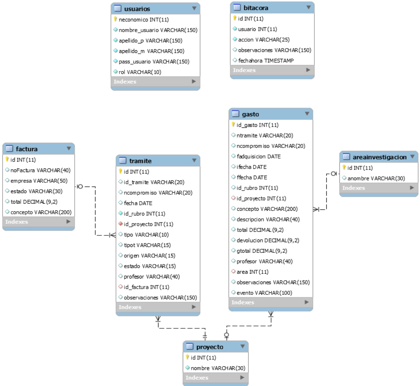
Figura 3. Diagrama entidad-relación.
