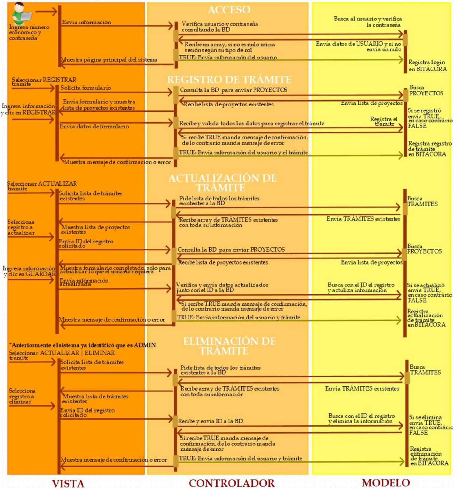
Figura 7. Diagramas de secuencia de registrar, actualizar y eliminar trámite.
