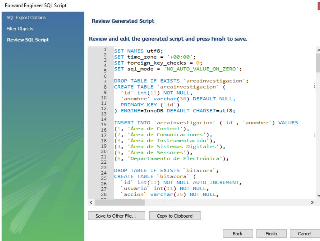
Figura 12. Generación de script parte dos.
