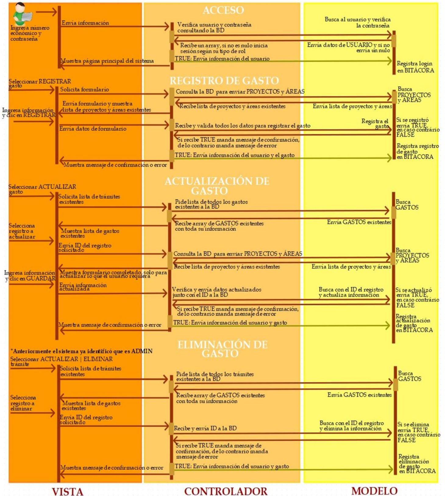
Figura 8. Diagramas de secuencia de registrar, actualizar y eliminar gasto.
